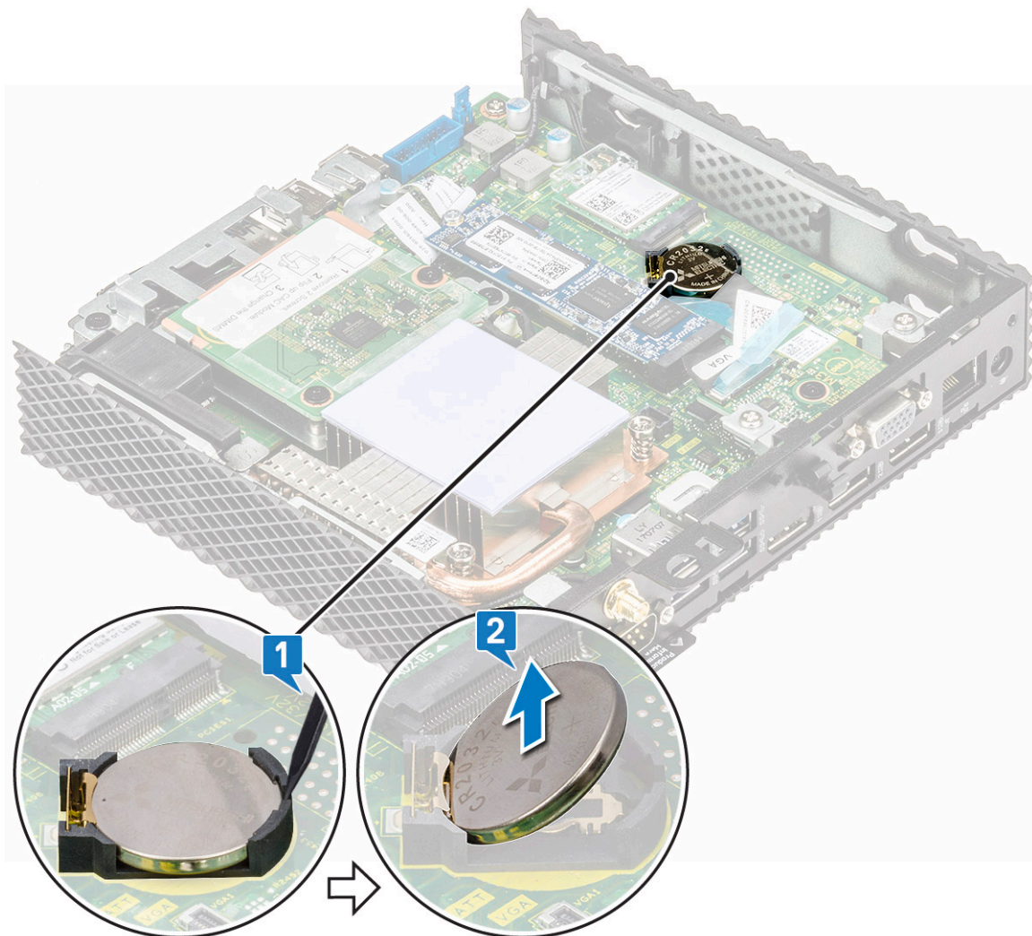
Figur 19. Ta bort knappcellsbatteriet
