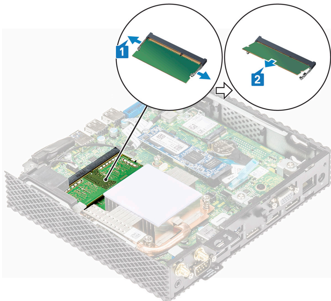
Figur 33. Ta bort minneskortet
