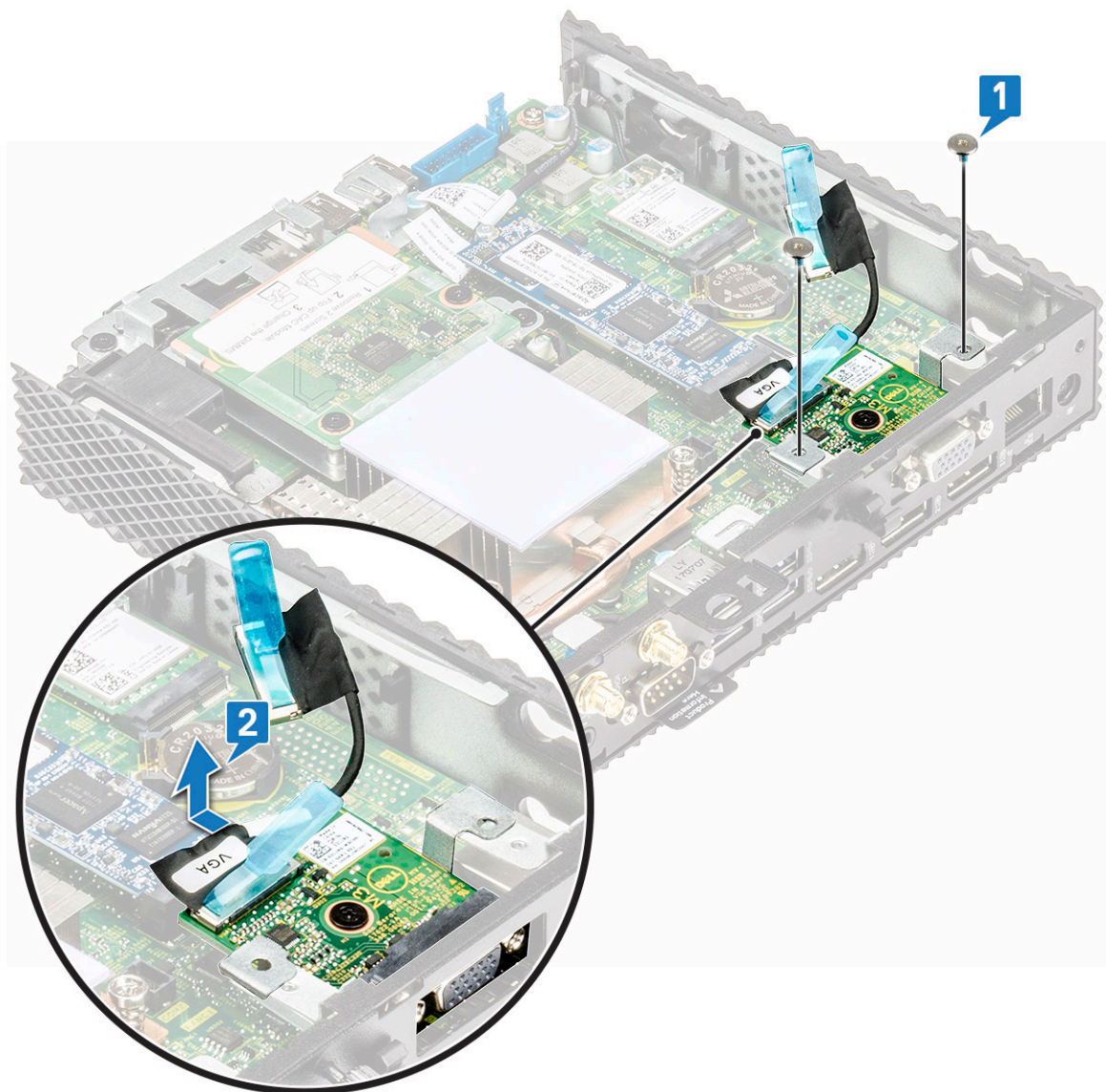
Figur 22. Ta bort expansionsplatsen
