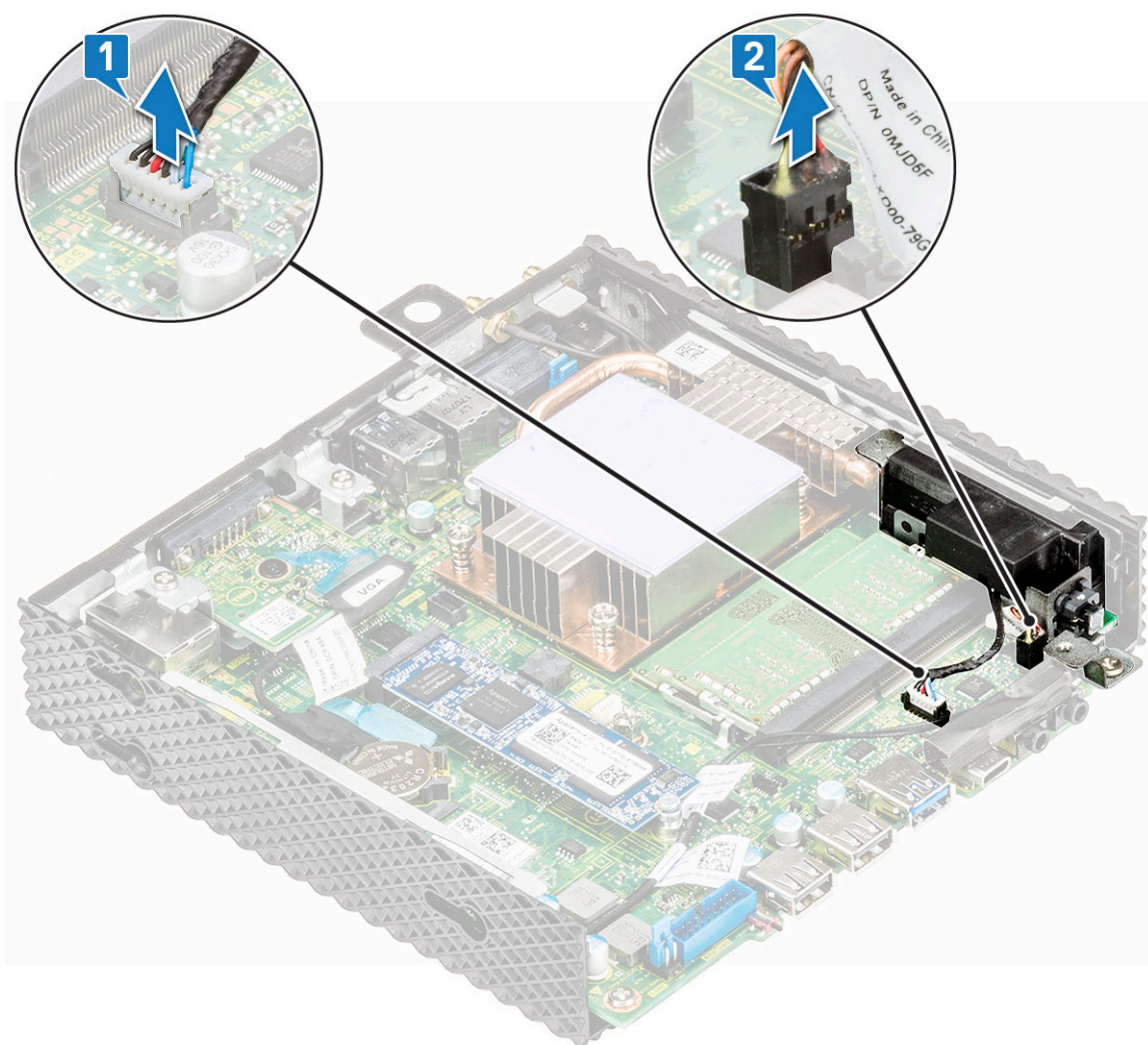
Figura 31. Desconecte os cabos
