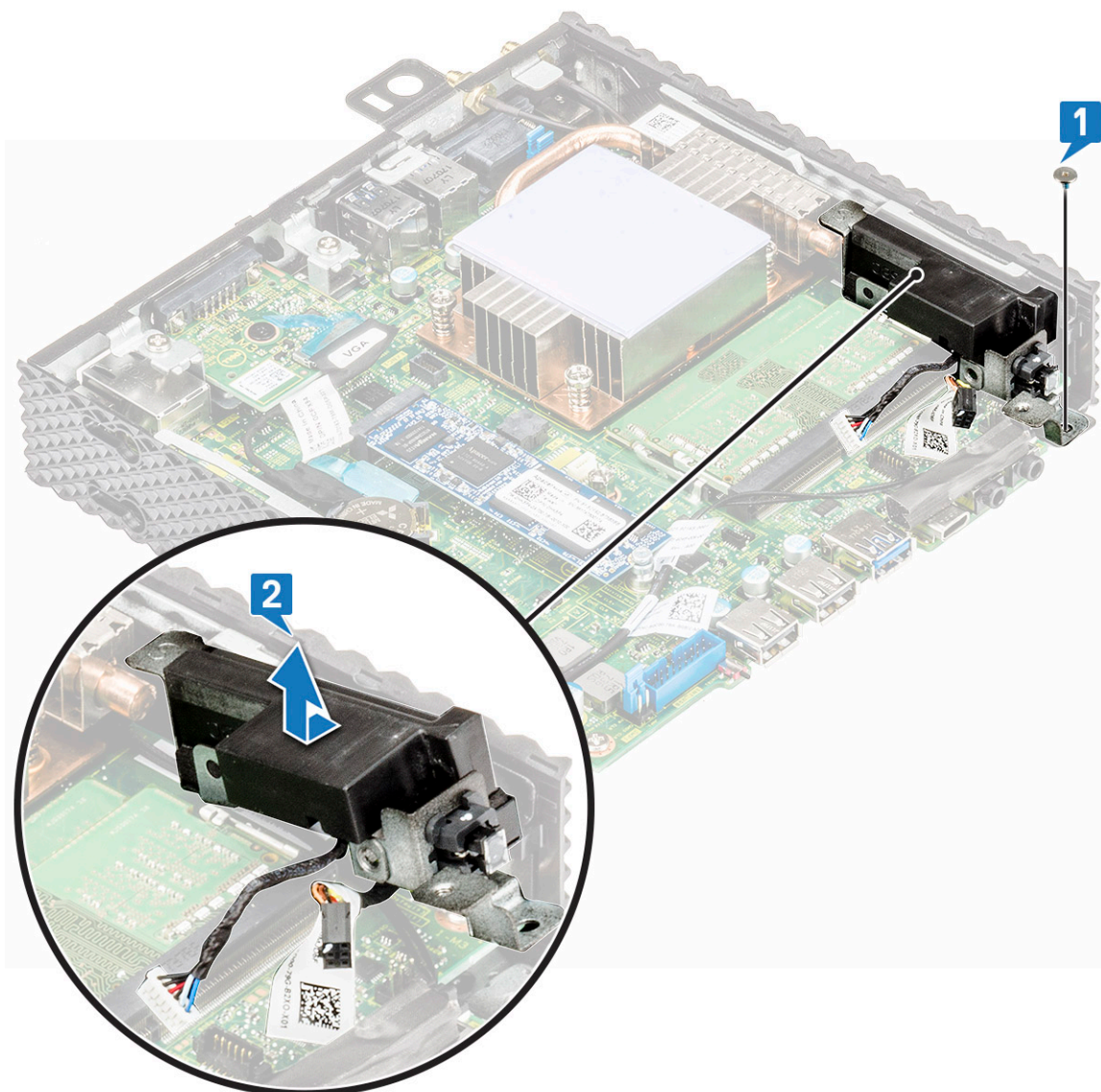
Figura 32. Remova o alto-falante/botão liga/desliga
