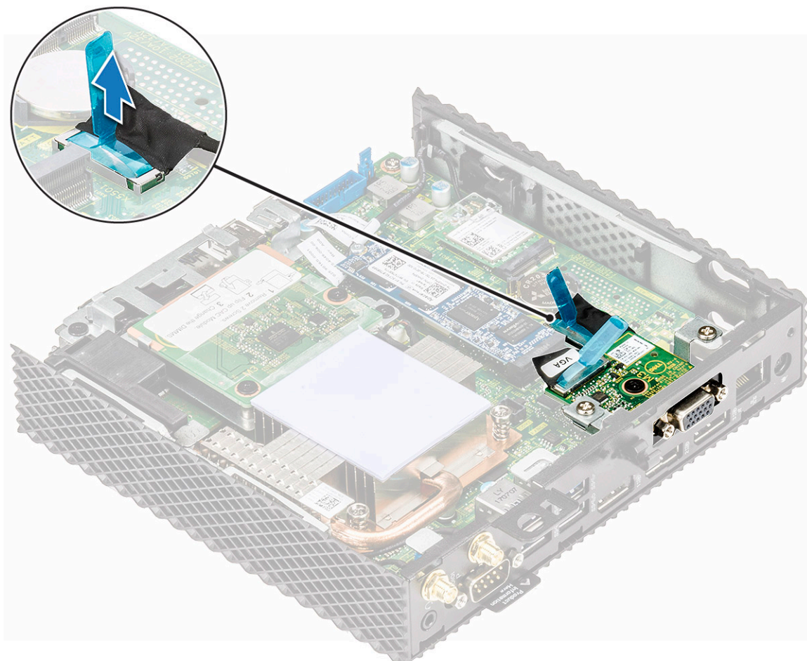
Figura 21. Desconecte o cabo Serial/VGA/SFP/RJ45
