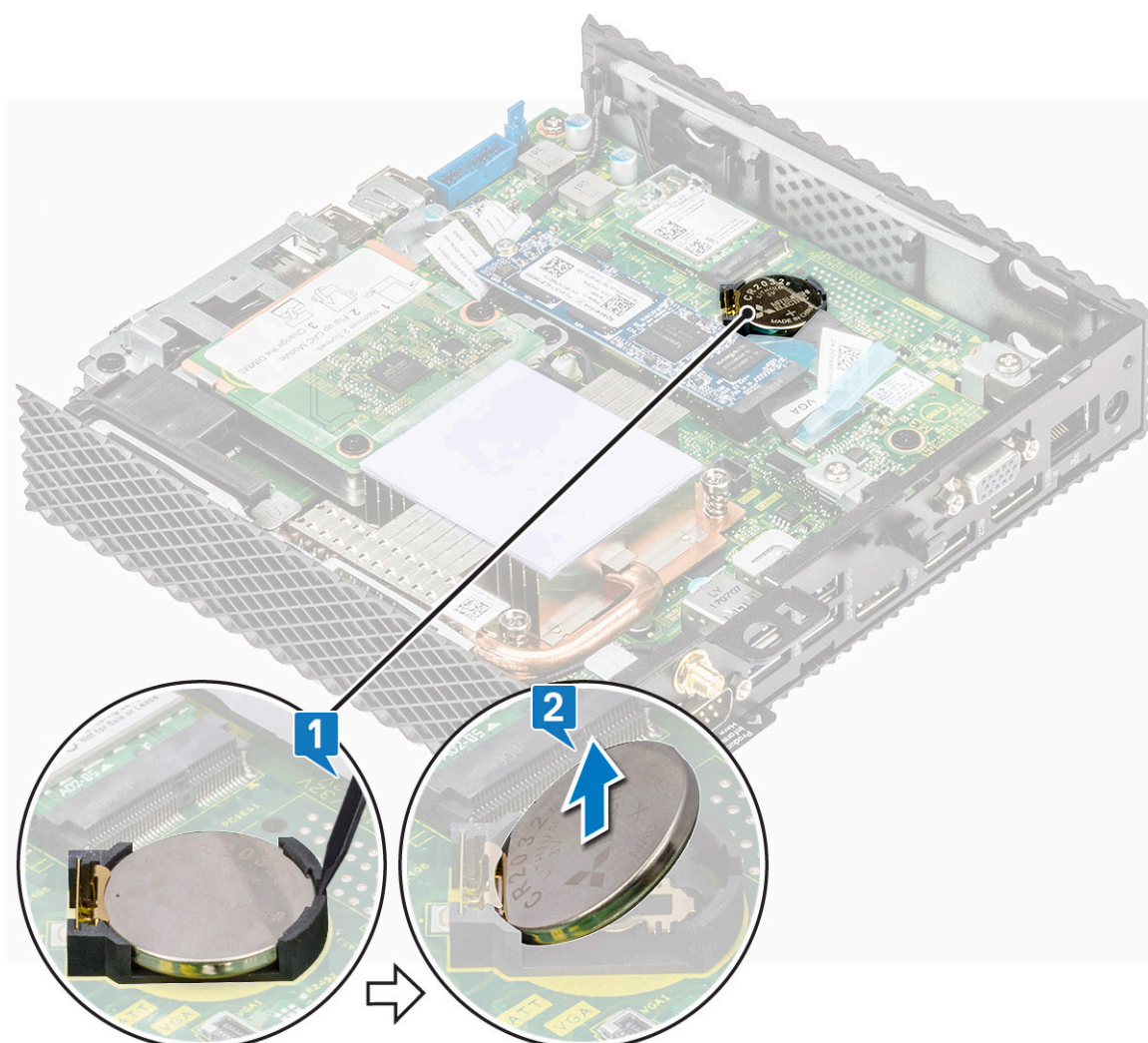
Figura 19. Remova a bateria de célula tipo moeda
