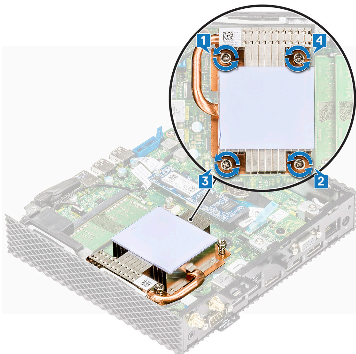
Figura 28. Remova os quatro parafusos
