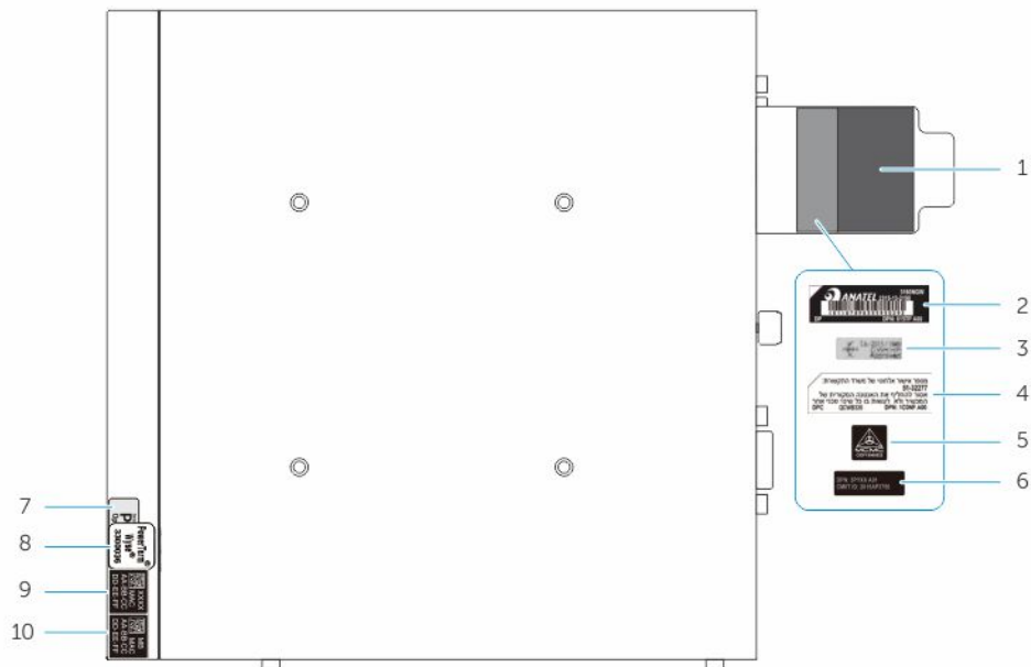
Afbeelding 4. Wyse 5070 thin client-labels
