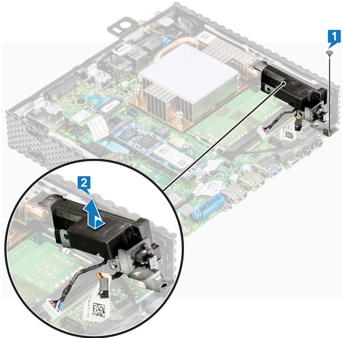
Afbeelding 32. Verwijder de luidspreker / aan/uit-knop
