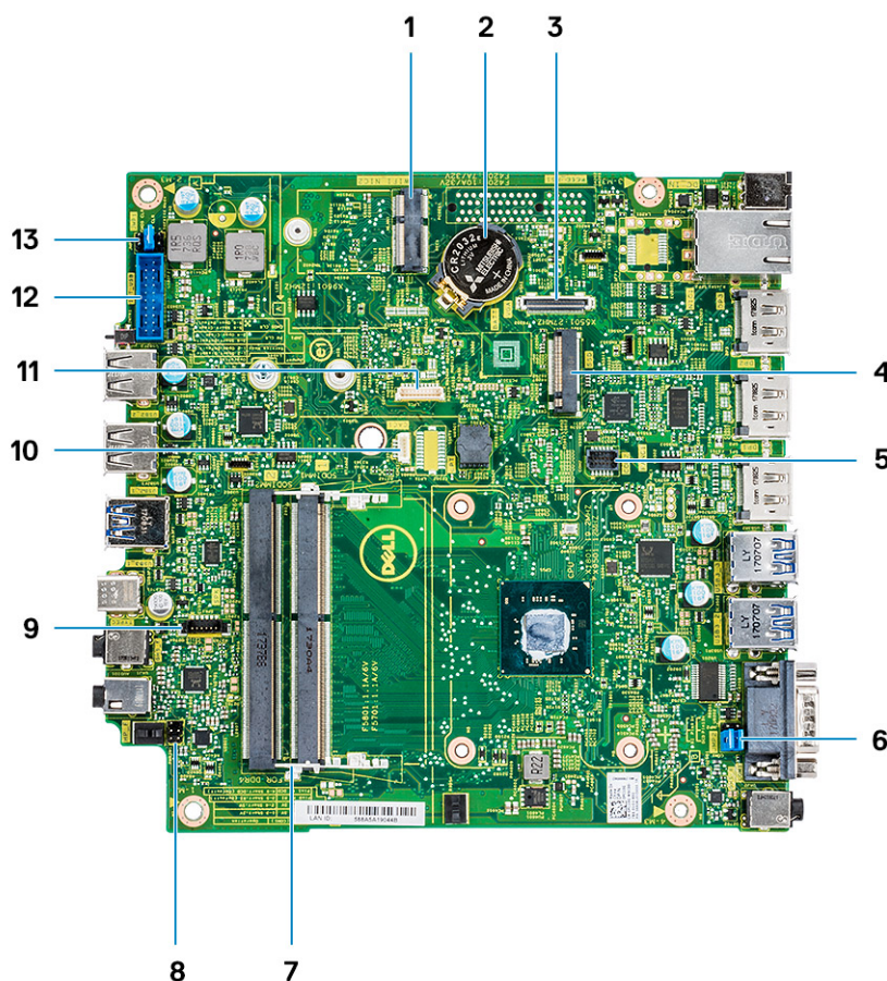
Afbeelding 6. Componenten op de systeemkaart
