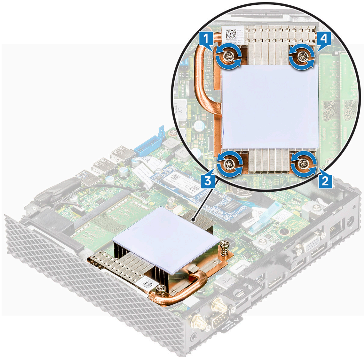
Afbeelding 28. Verwijder de vier schroeven
