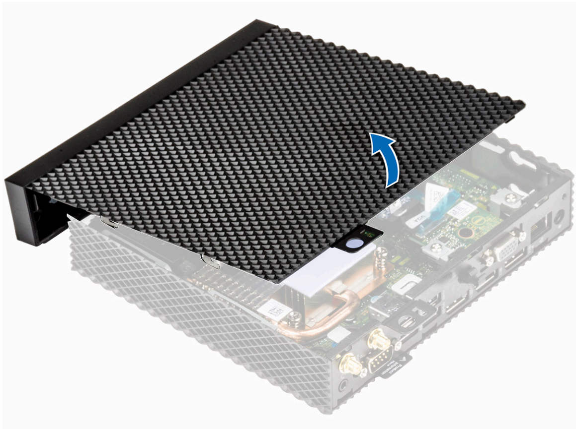
Afbeelding 14. Til de kap op
