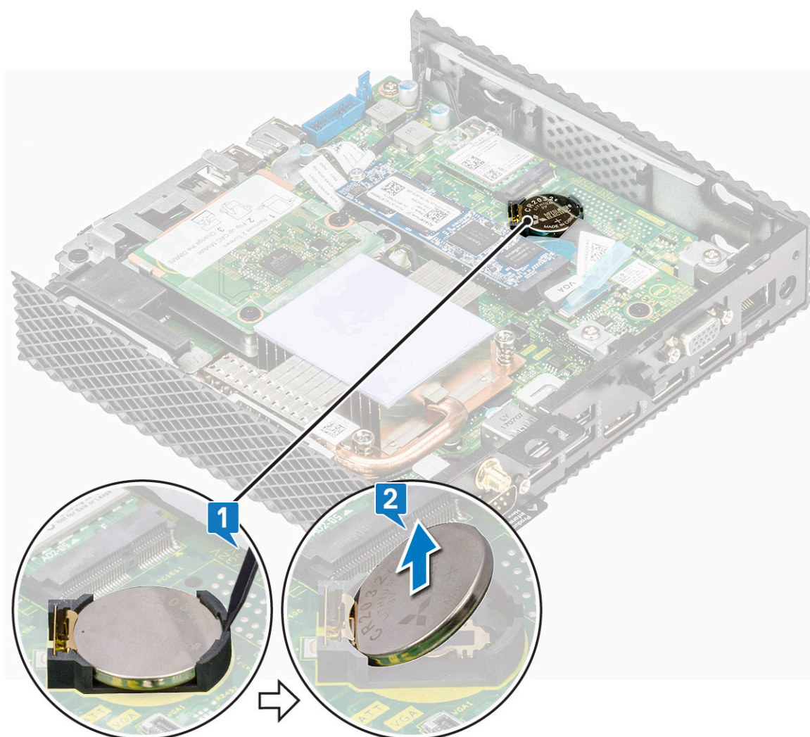
Figura 19. Rimuovere la batteria a bottone
