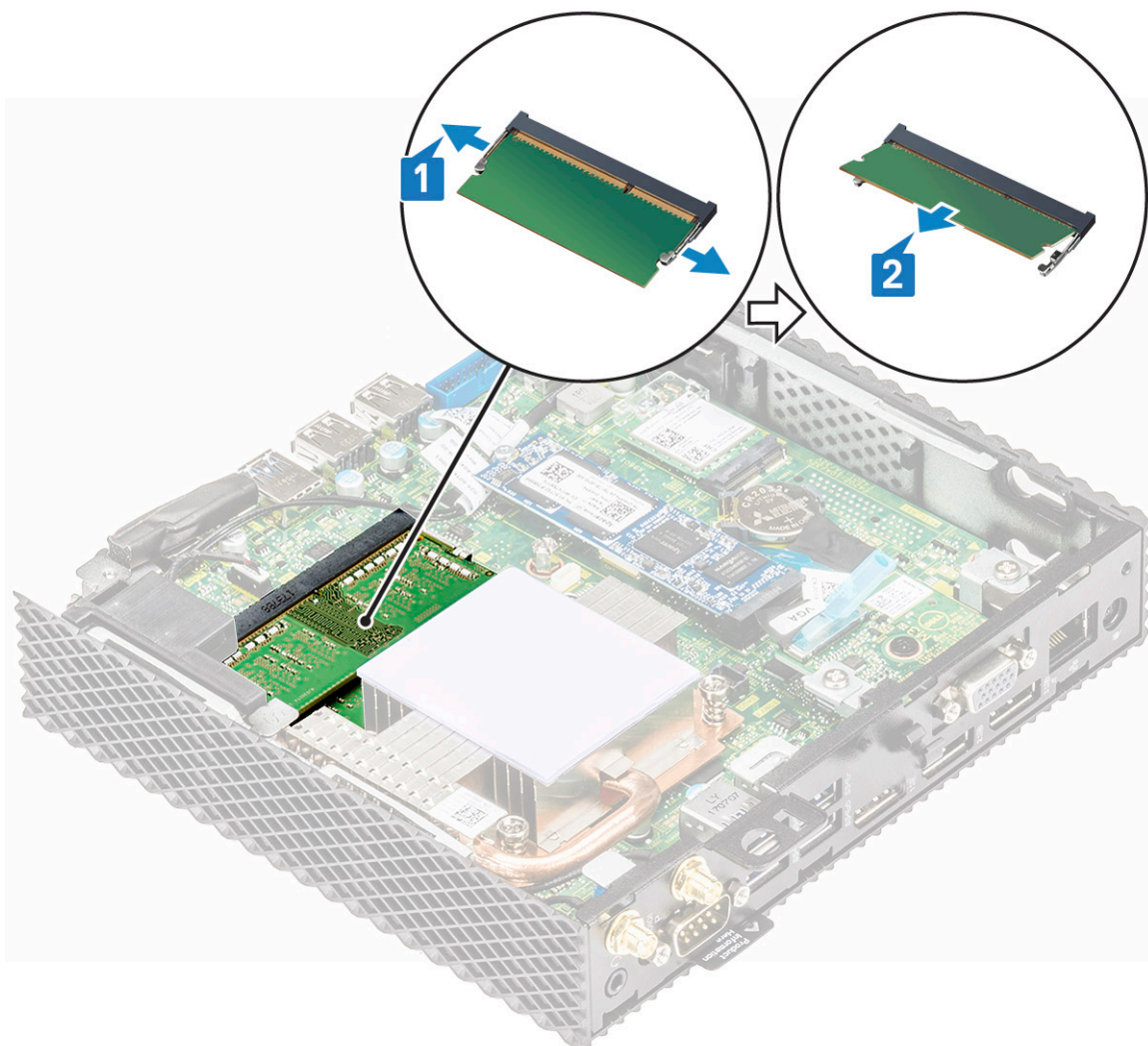
Figura 33. Rimuovere le schede di memoria
