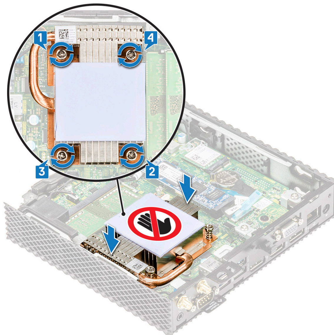
Figura 30. Installazione del dissipatore di calore
