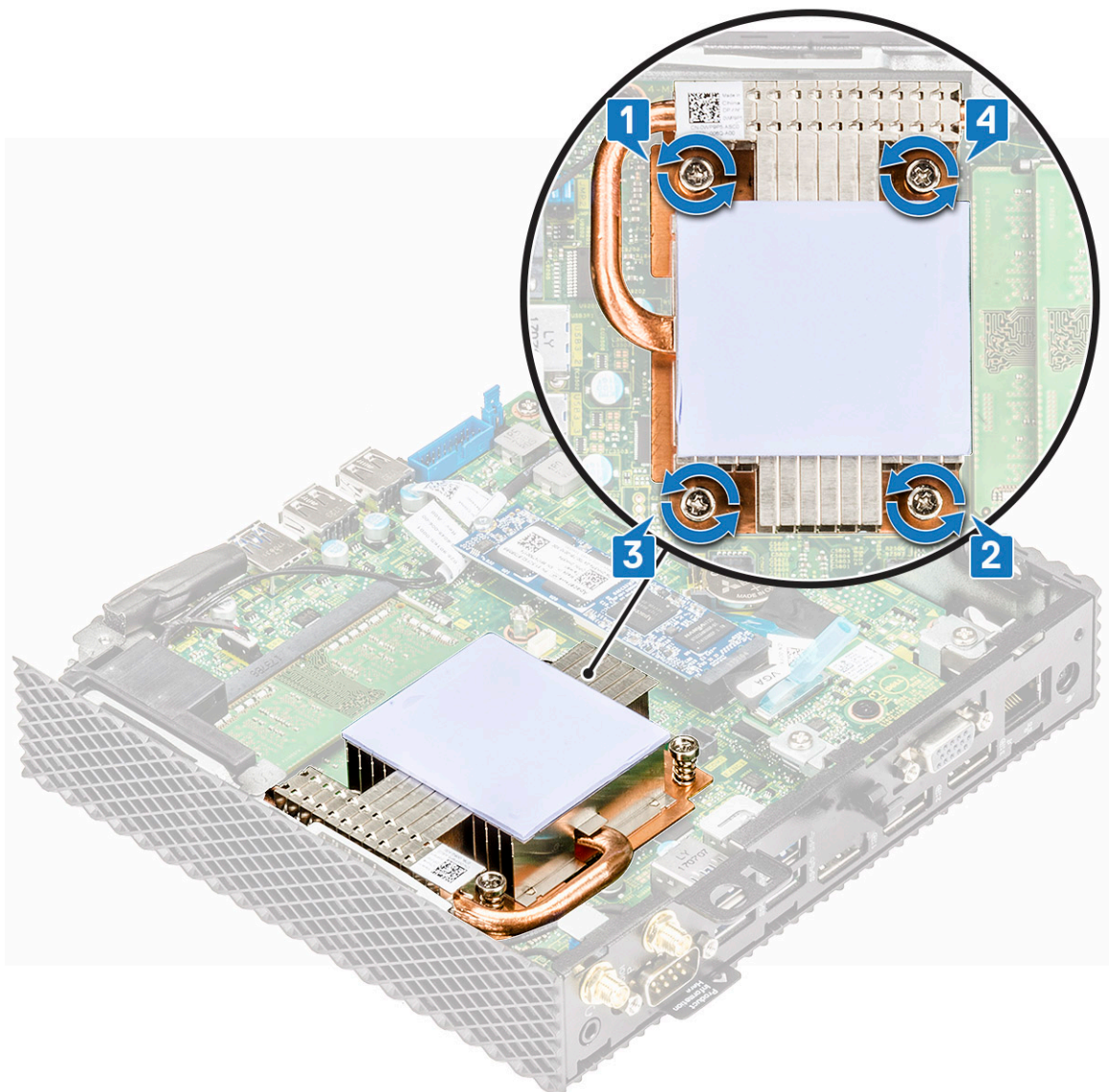
Figura 28. Rimuovere le quattro viti
