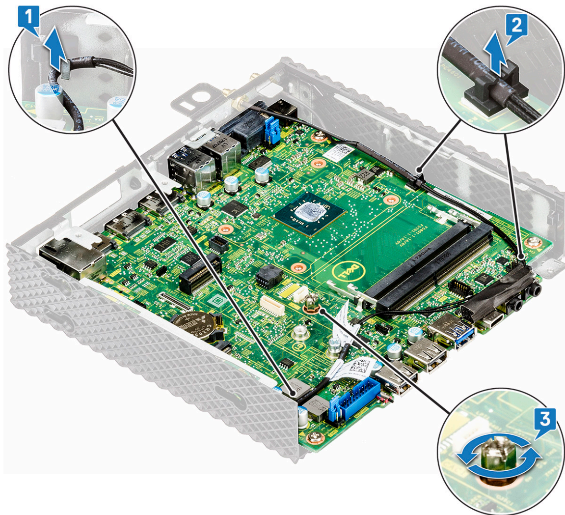
Figura 36. Rimuovere il cavo e la vite
