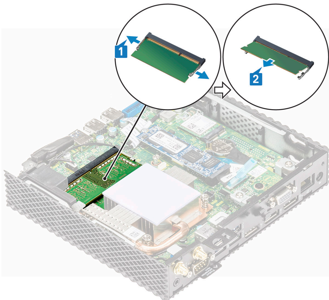
33. ábra. Távolítsa el a memóriakártyákat
