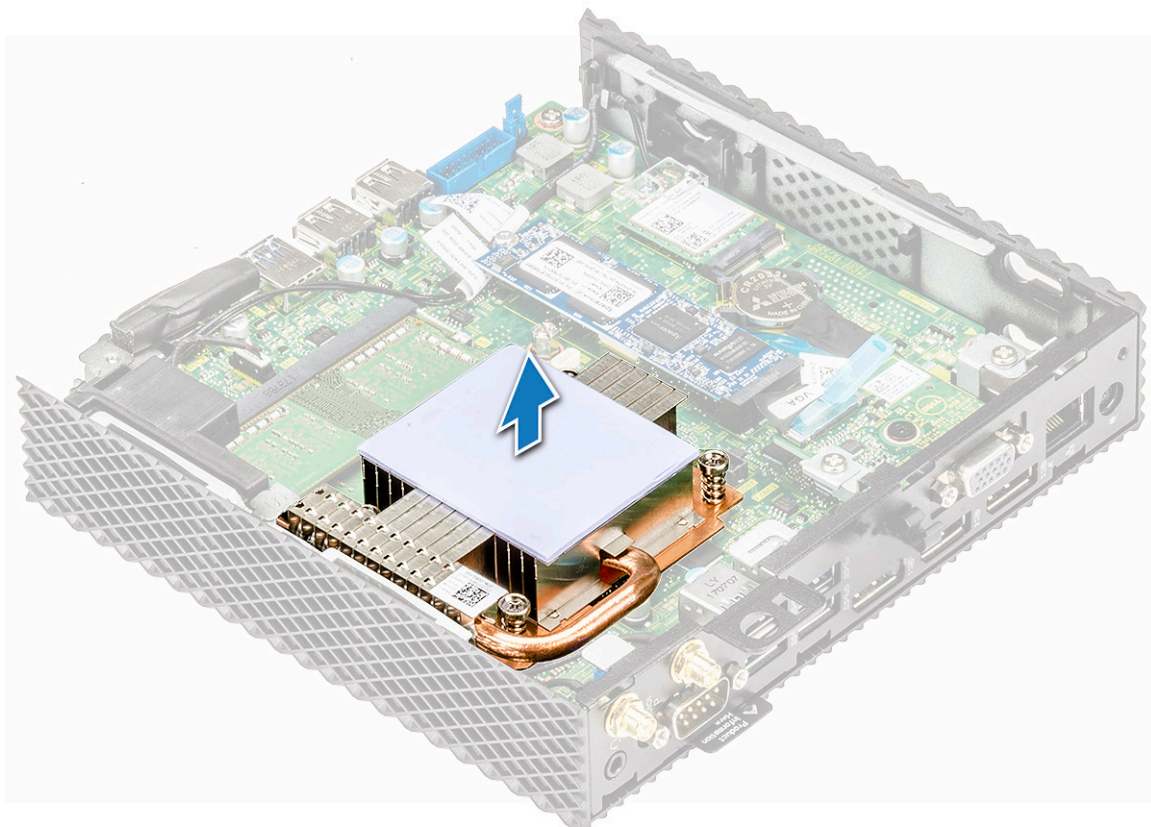
29. ábra. A hűtőborda leemelése
