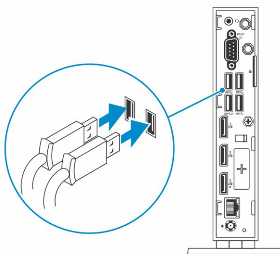
8. ábra. A billentyűzet és az egér üzembe helyezése
