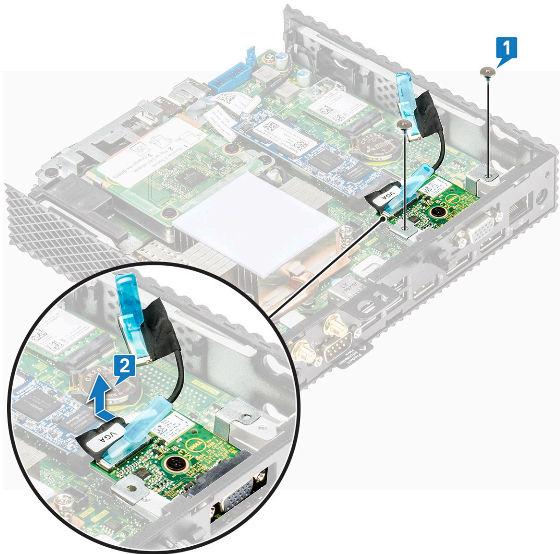
איור 22. הסר את כרטיס ההרחבה
