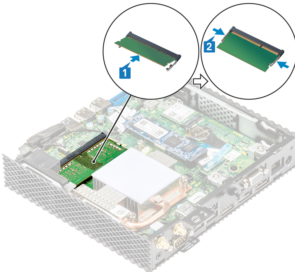
איור 35. התקנת מודול זיכרון
