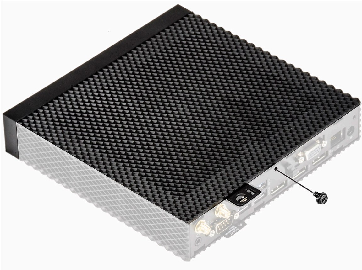
איור 12. שחרר את הבורג הידני
