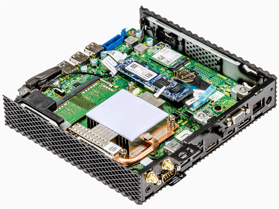
איור 25. תושבת קורא כרטיסי CAC הוסרה
