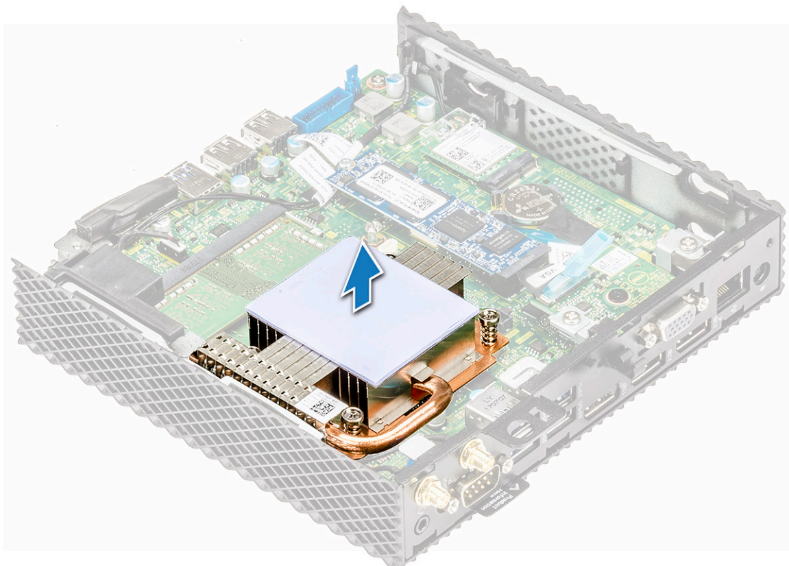
איור 29. הרם את גוף הקירור
