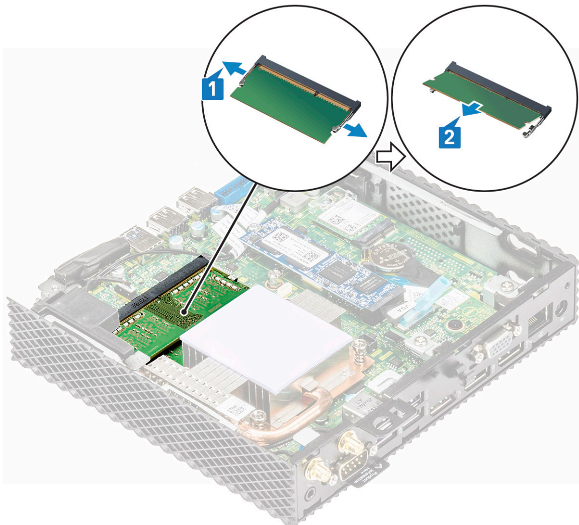
איור 33. הסר את כרטיסי הזיכרון
