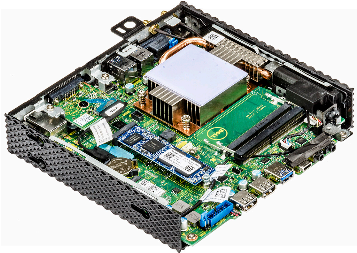
איור 34. כרטיסי הזיכרון הוסרו
