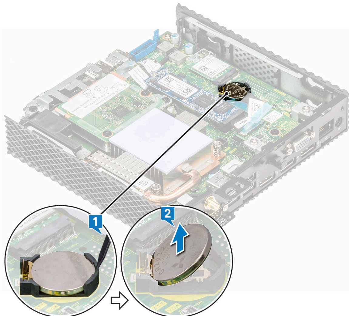
איור 19. הסר את סוללת המטבע
