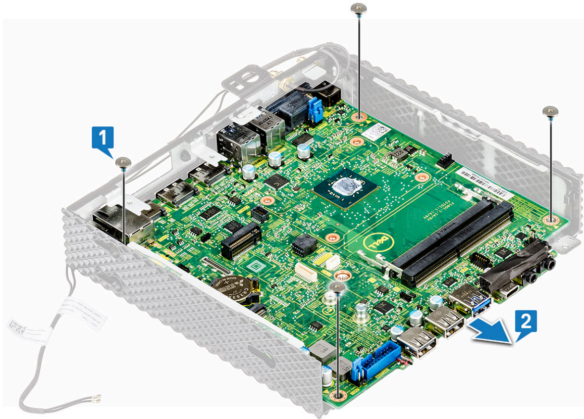
איור 37. הסר את ארבעת הברגים
