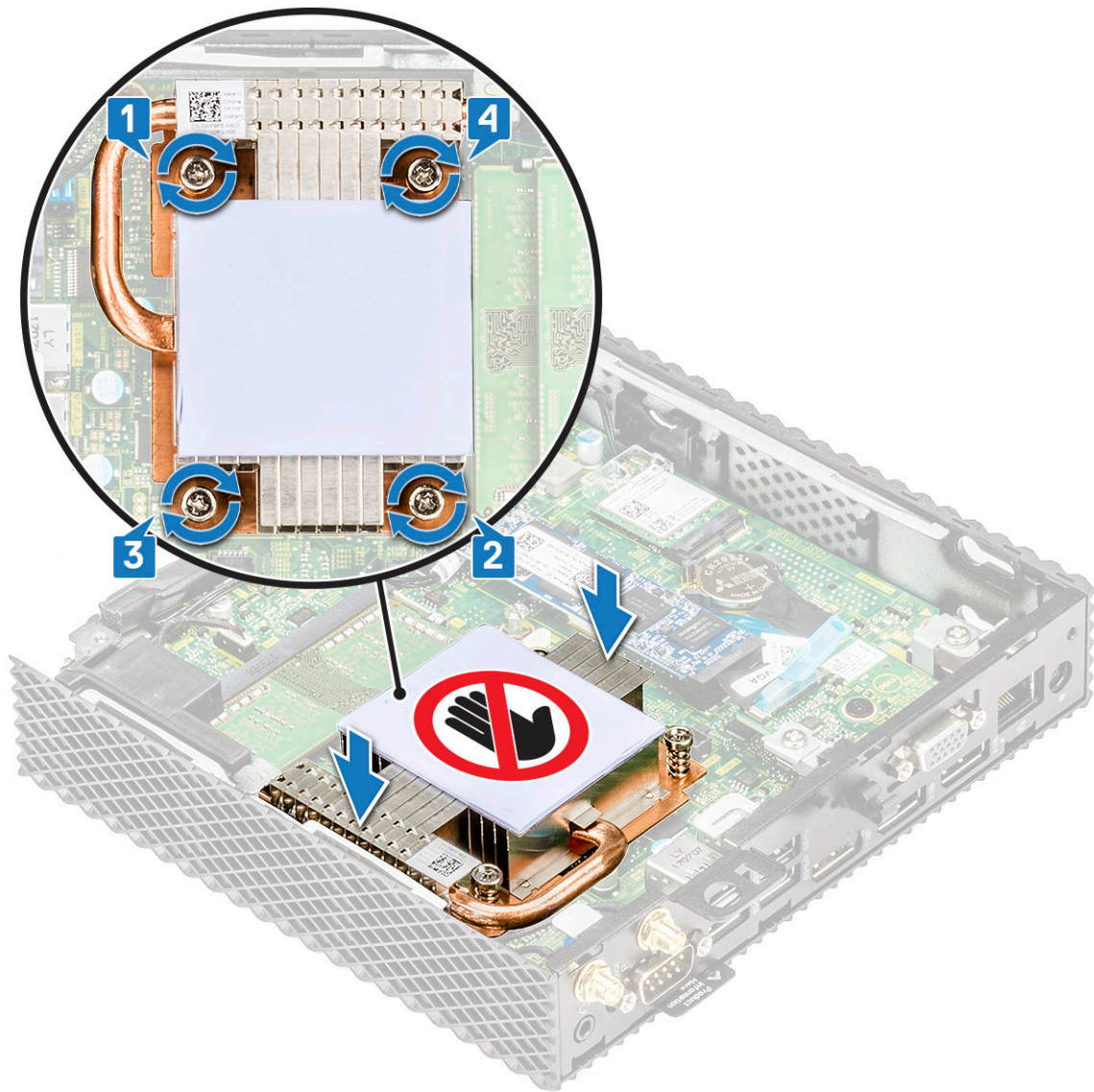
איור 30. התקנת גוף הקירור
