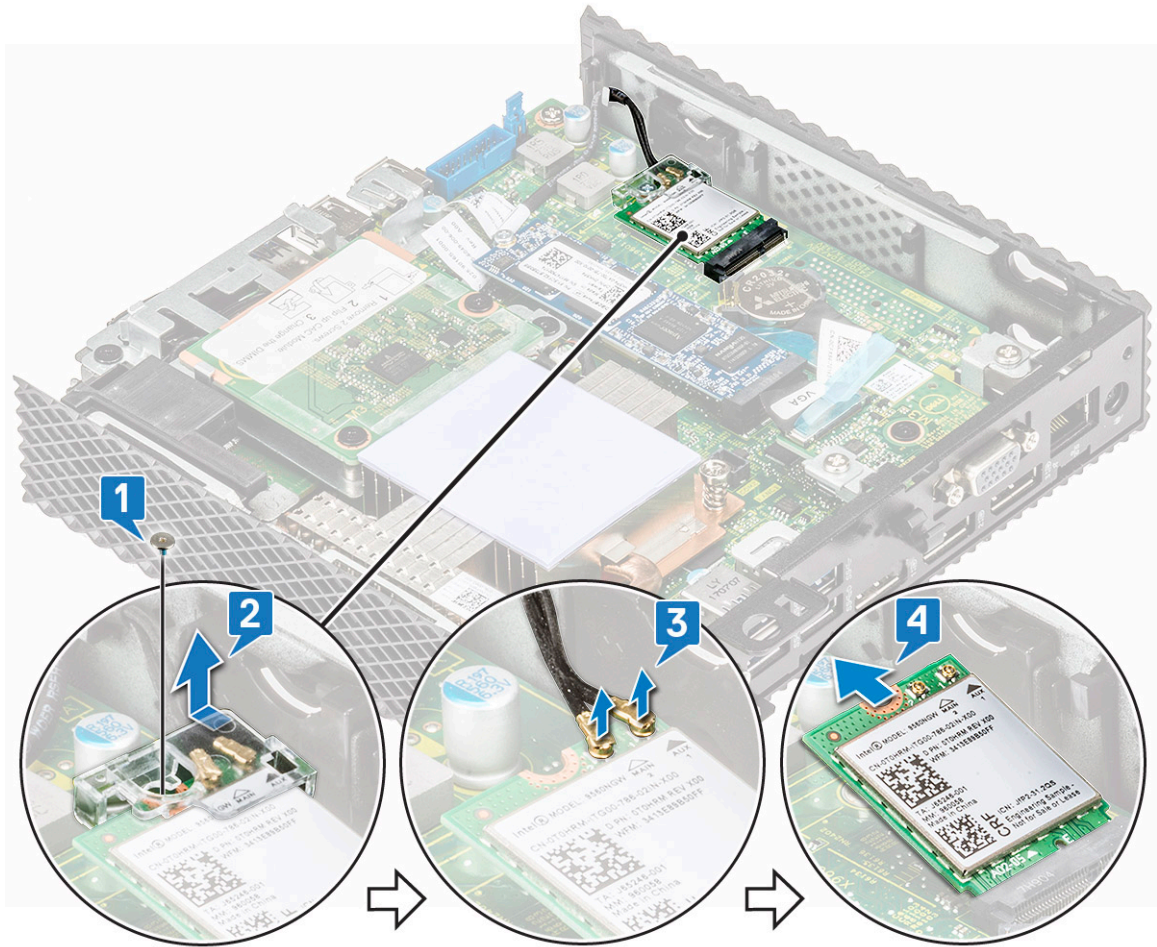
איור 20. הסר את כרטיס האלחוט
