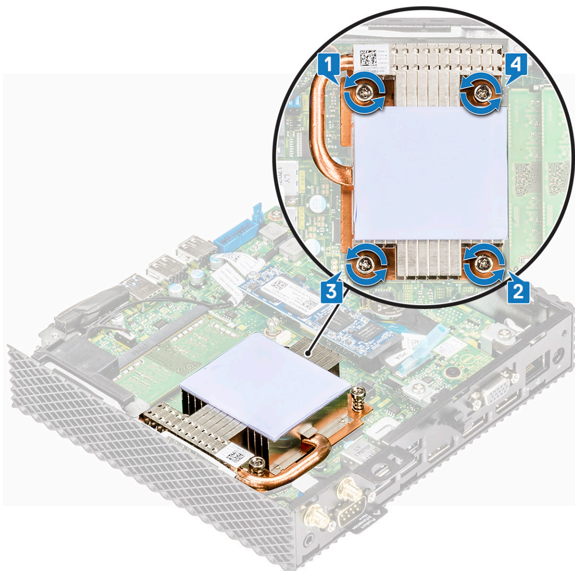
איור 28. הסר את ארבעת הברגים 3. הרם את גוף הקירור והרחק אותו מהלקוח הרזה.
