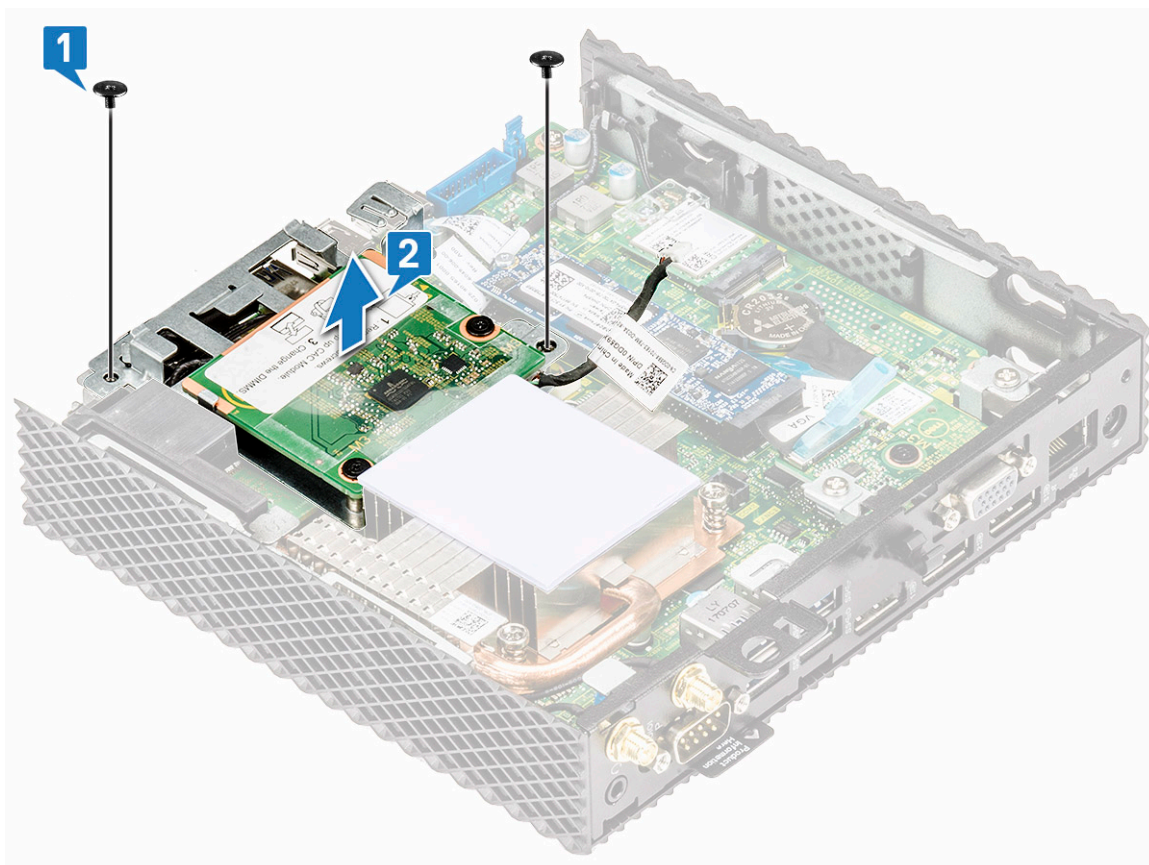
איור 24. הסר את תושבת קורא כרטיסי CAC
