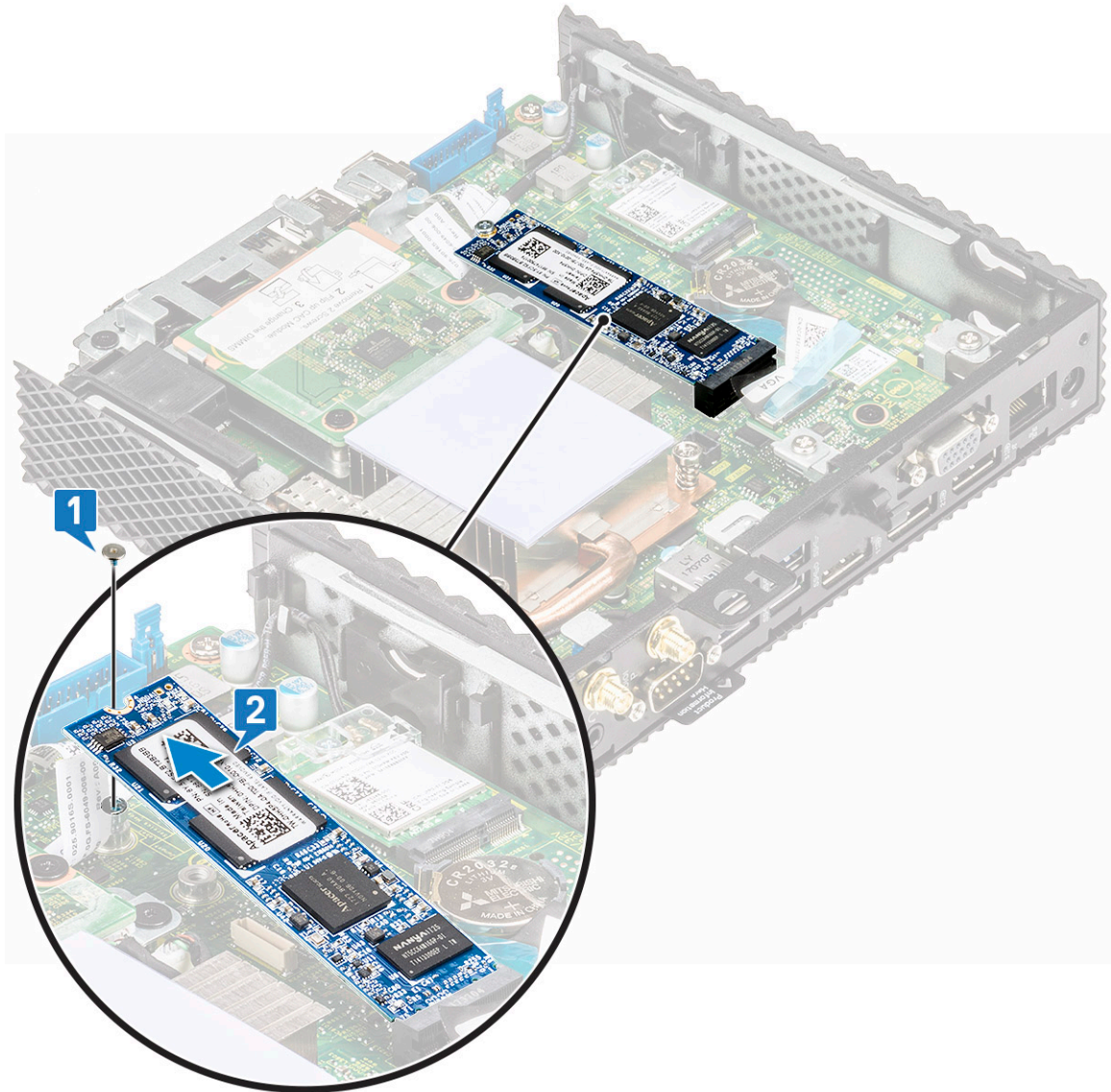
איור 18. הסר את ה-SSD
