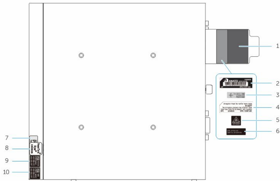
Kuva 4. Wyse 5070 Thin Client -merkinnät
