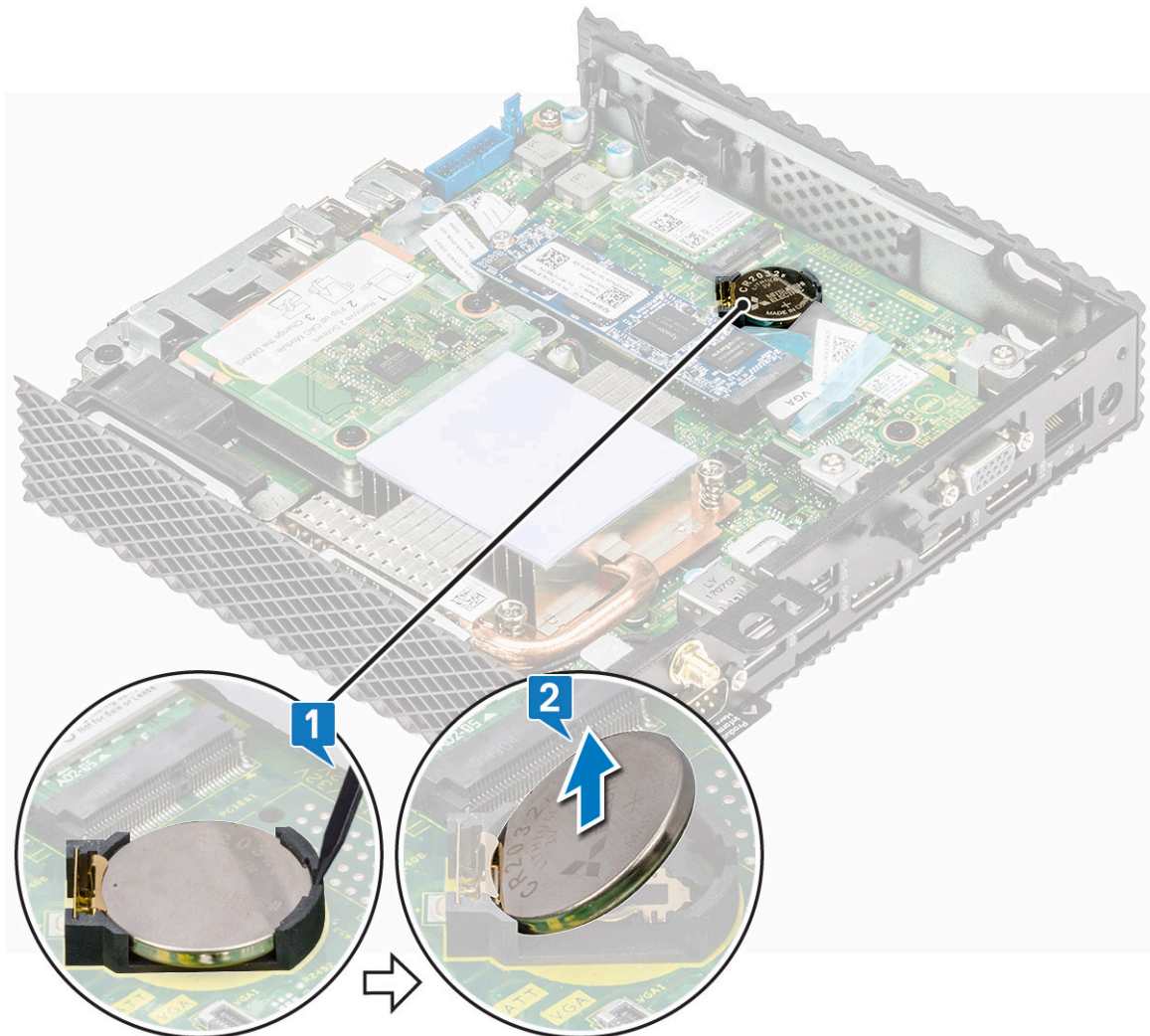
Kuva 19. Irrota nappiparisto
