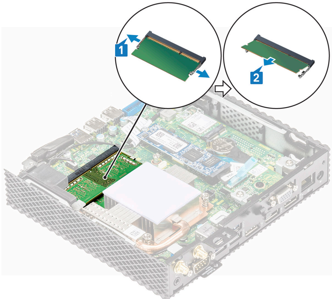
Kuva 33. Irrota muistikortit
