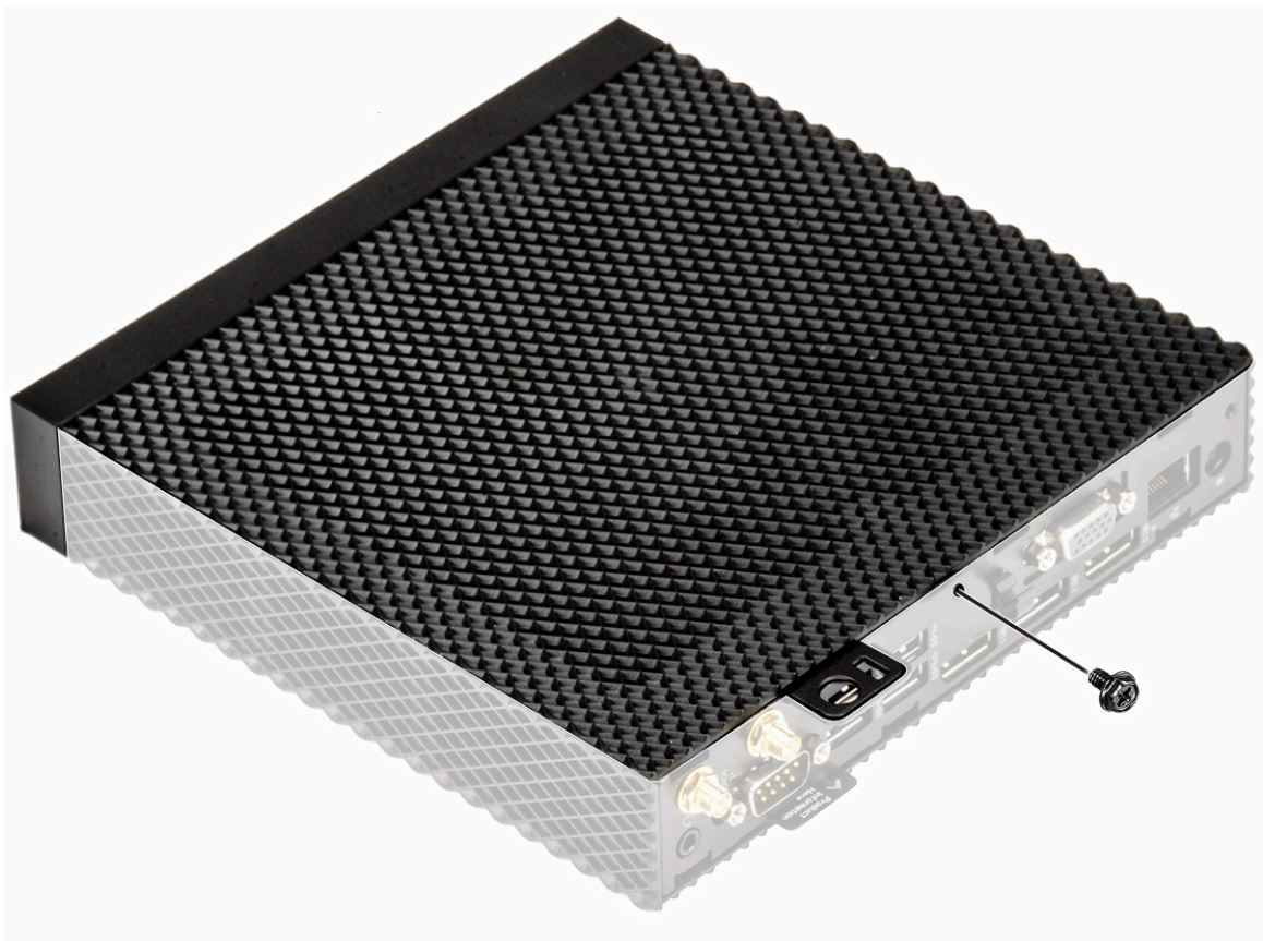
Kuva 12. Löysää lukkoruuvia
