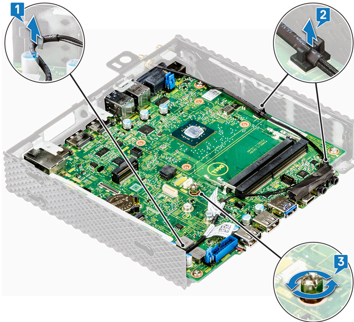
Kuva 36. Irrota kaapeli ja ruuvi
