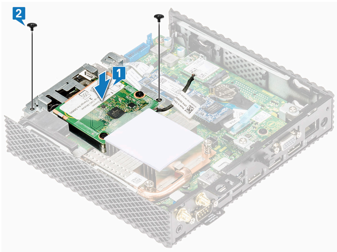
Figur 26. Juster skruehullerne, og isæt skruen
