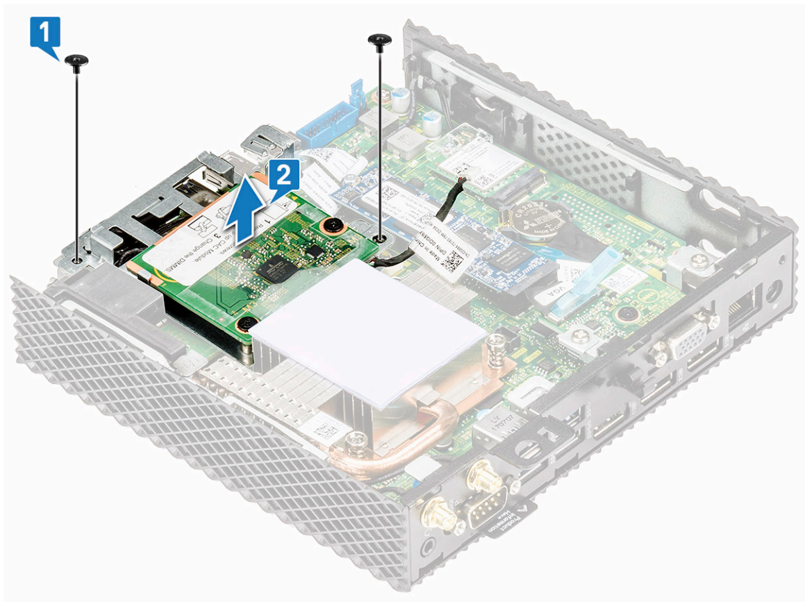
Figur 24. Fjern CAC-læserens beslag
