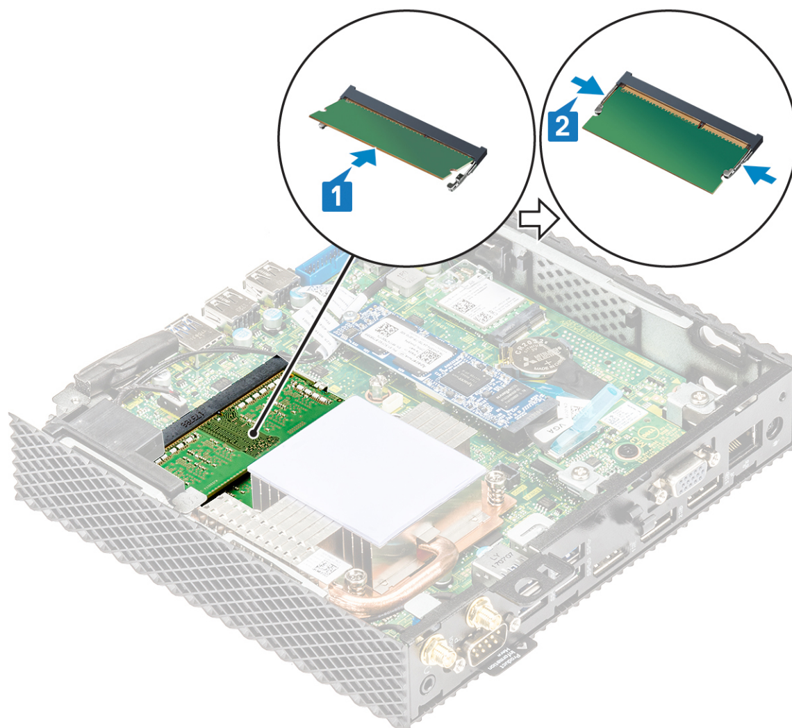
Figur 35. Installation af hukommelsesmodul
