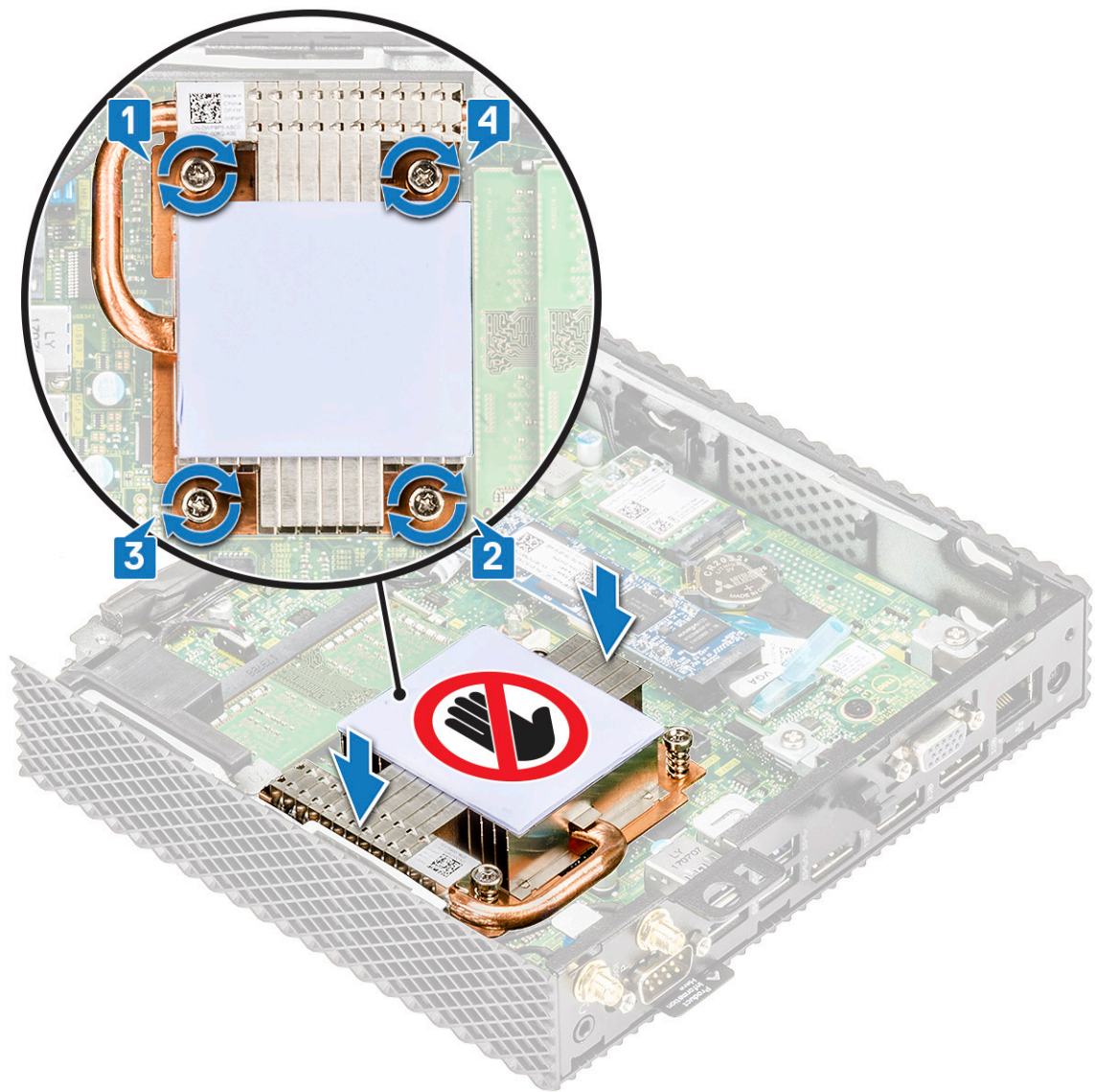
Figur 30. Installation af kølelegemet
