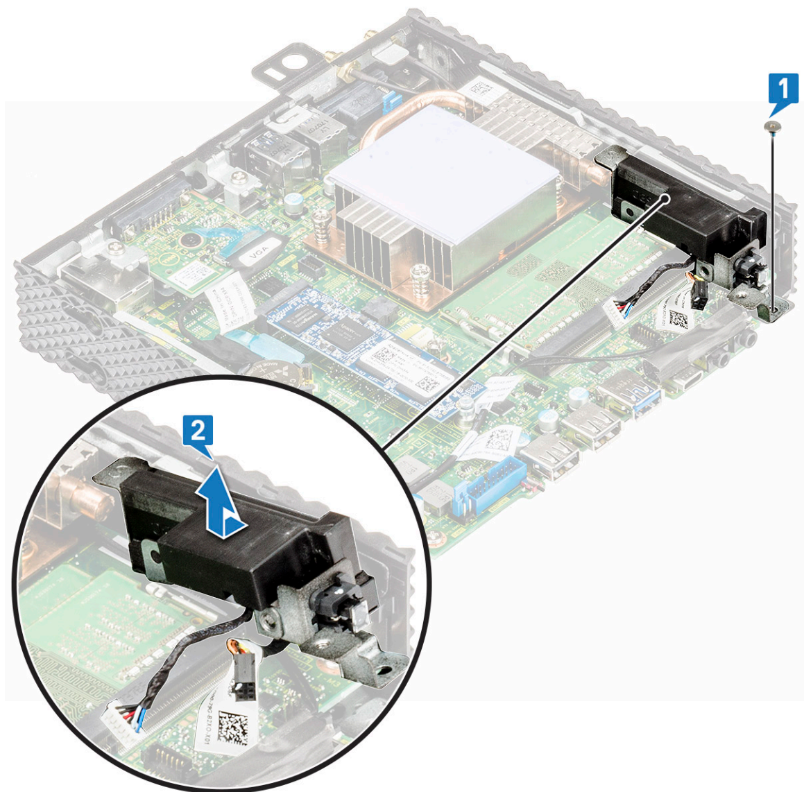
Figur 32. Fjern højttaleren og tænd/sluk-knappen
