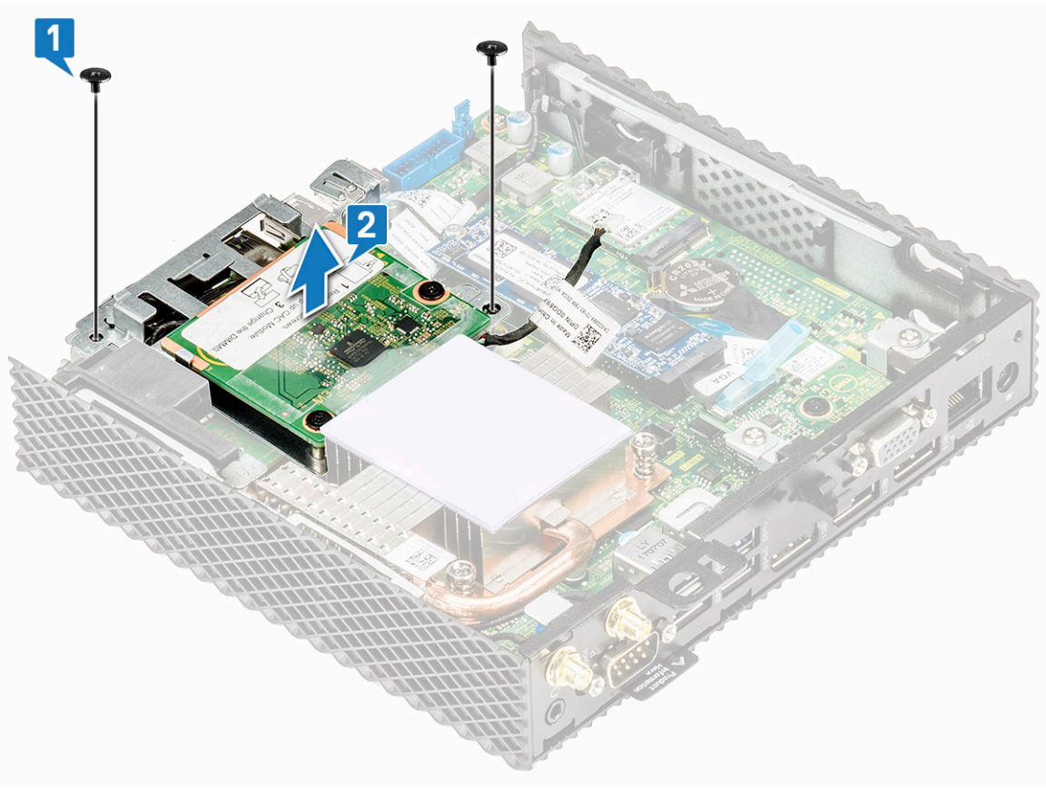
شكل 24. إزالة حامل قارئ بطاقة الوصول المشترك
