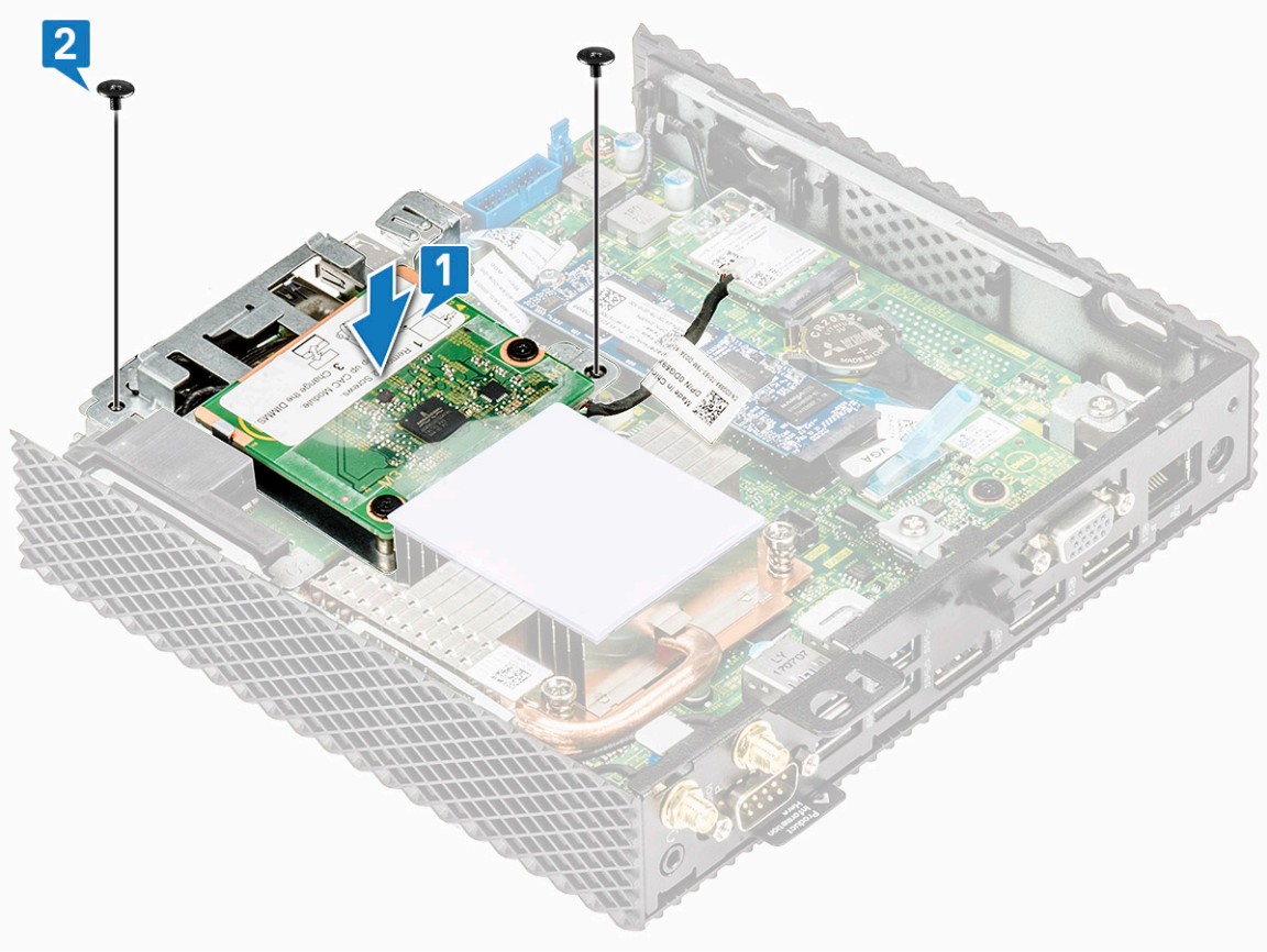
شكل 26. محاذاة فتحات المسامير وإعادة وضع المسامير 3. قم بتوصيل كابل قارئ بطاقة الوصول المشترك بلوحة النظام.
