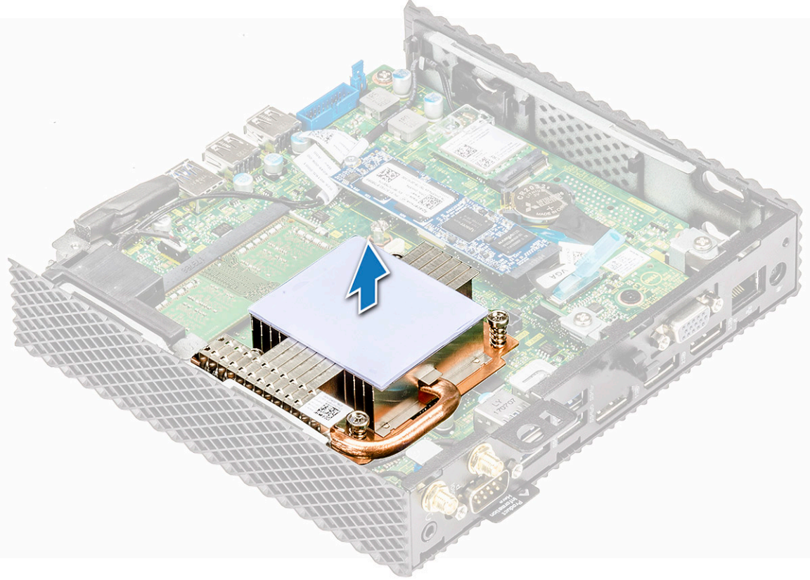
شكل 29. تركيب المشنت الحراري
