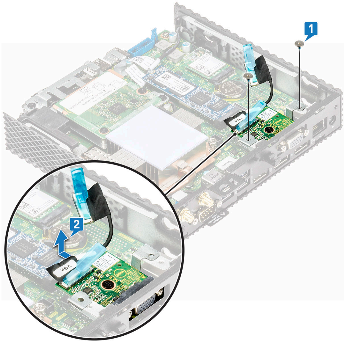
شكل 22. إزالة فتحة التوسعة
