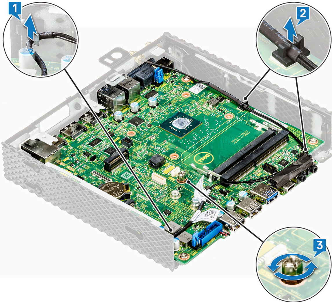
شكل 36. إزالة الكبل والمسامير اللولبية
