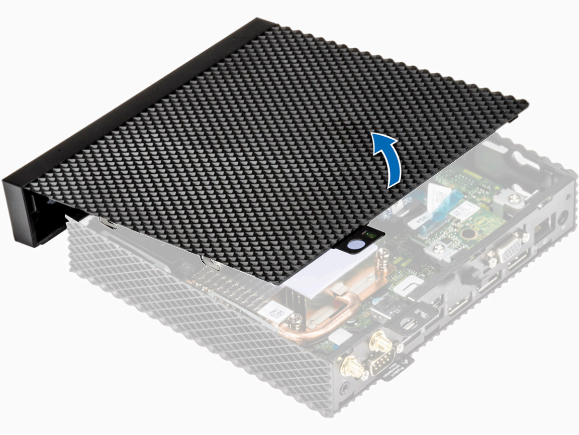
شكل 14. رفع الغطاء
