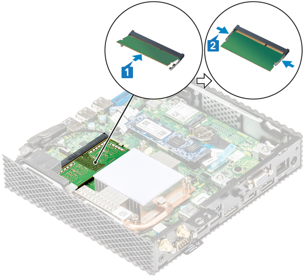
شكل 35. تركيب وحدة الذاكرة
