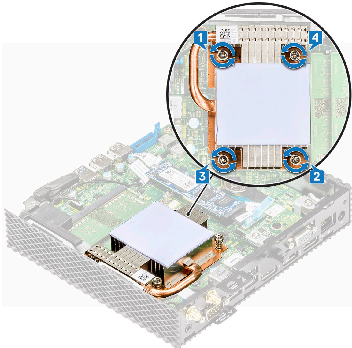
شكل 28. إزالة المسامير الأربعة 3. ارفع المشتت الحراري بعيداً عن جهاز الكمبيوتر التابع.
