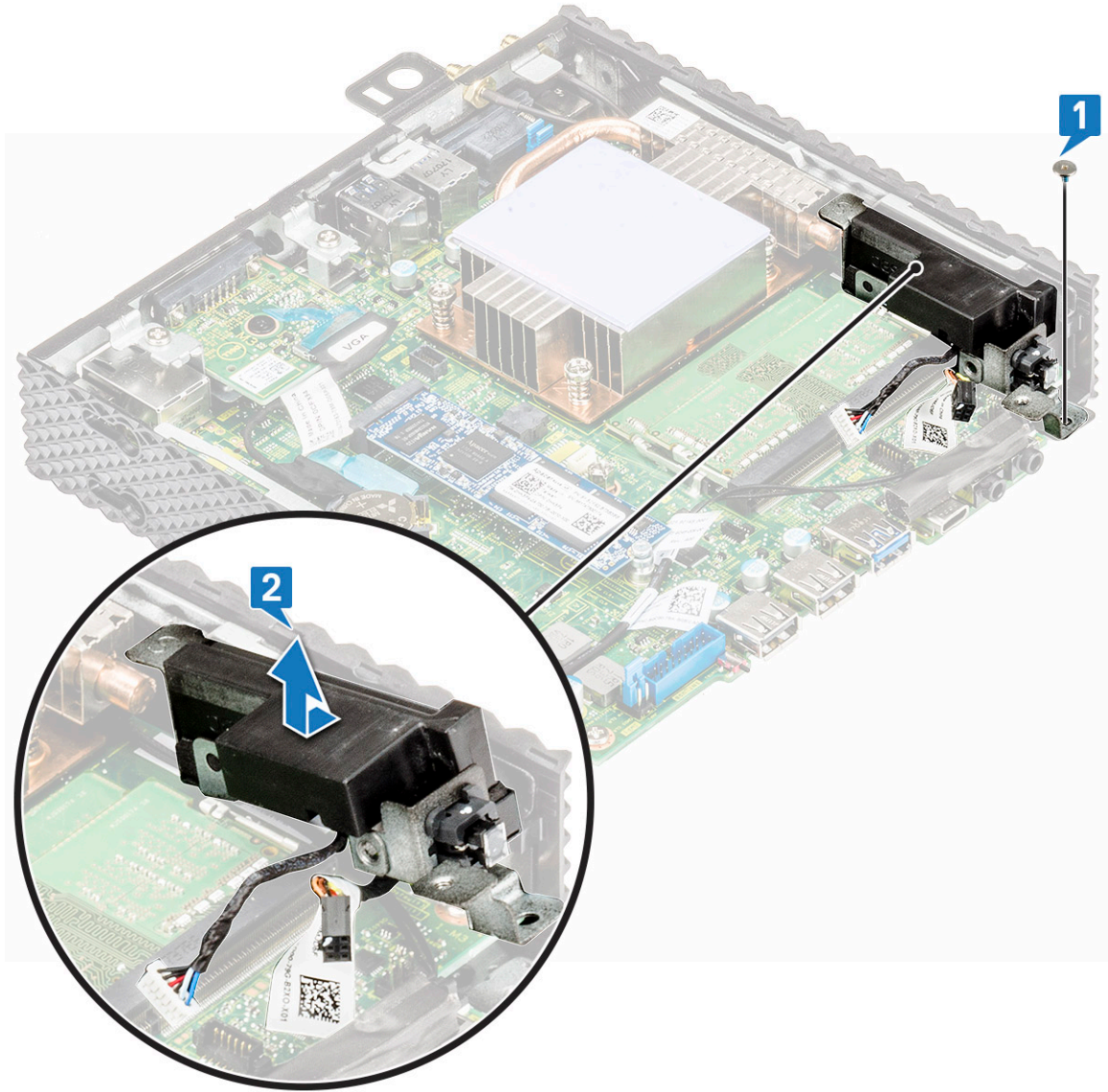
شكل 32. إزالة مكبر الصوت/زر التشغيل
