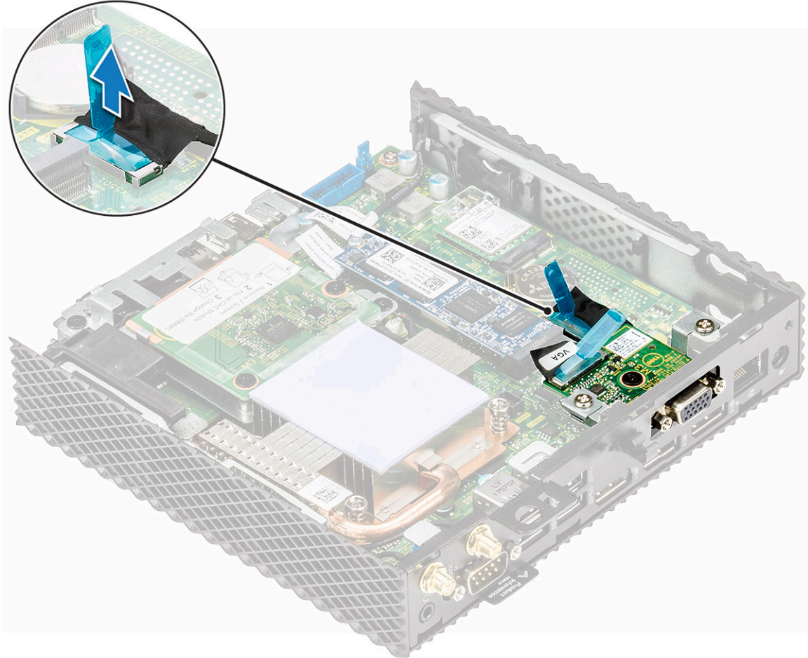
شكل 21. فصل كبل تسلسلي/RJ45/SFP/VGA
