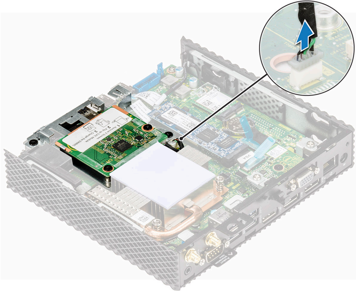
شكل 23. فصل الكبل
