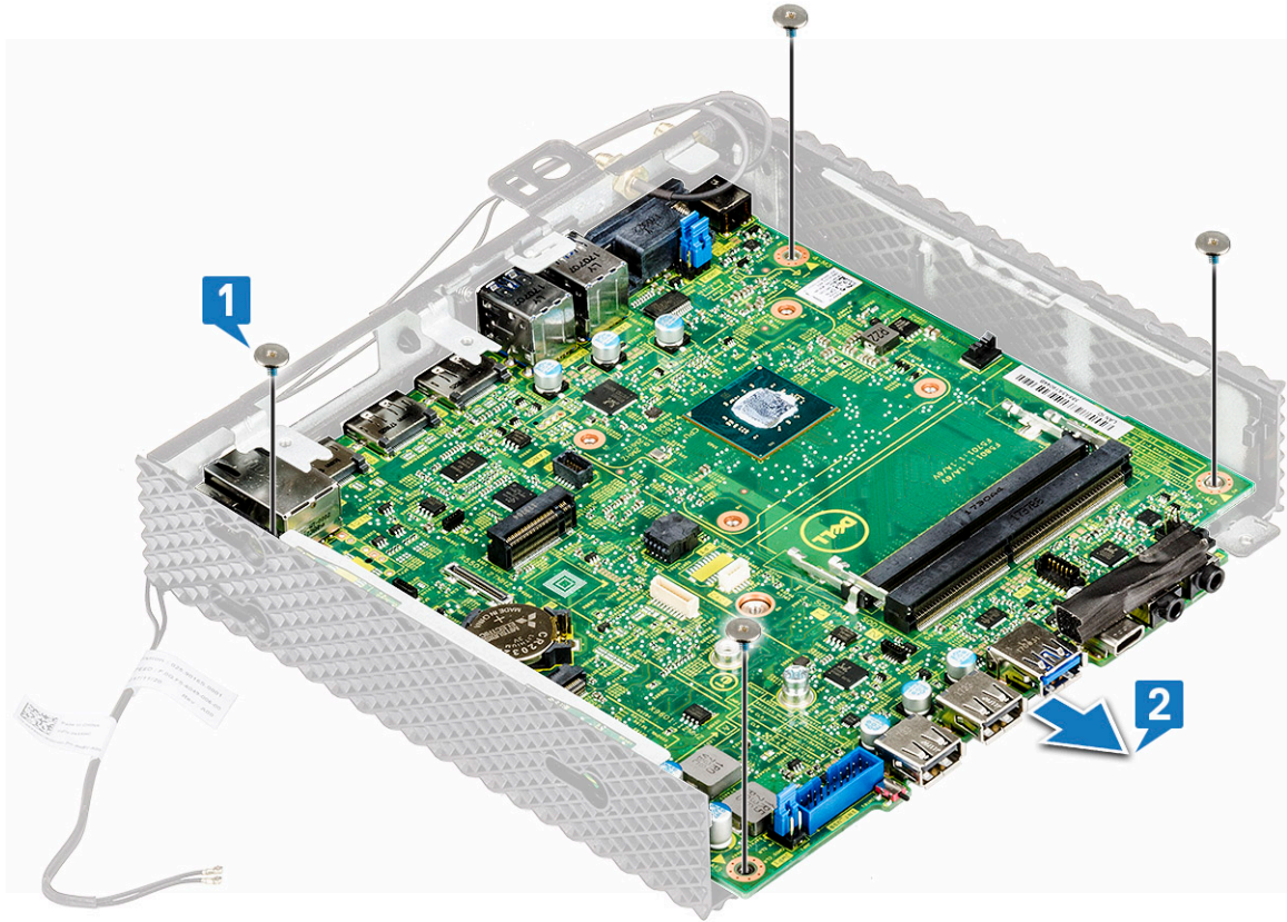
شكل 37. إزالة المسامير الأربعة
