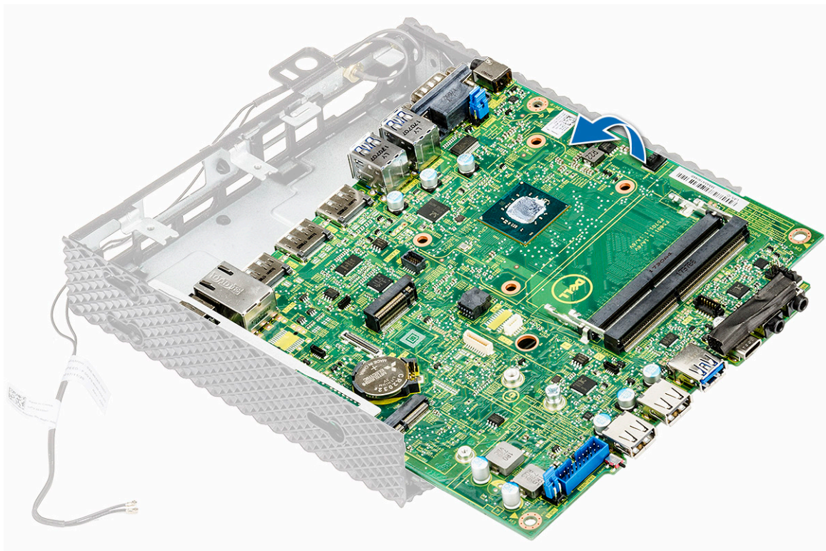
شكل 38. قم بإزالة لوحة النظام
