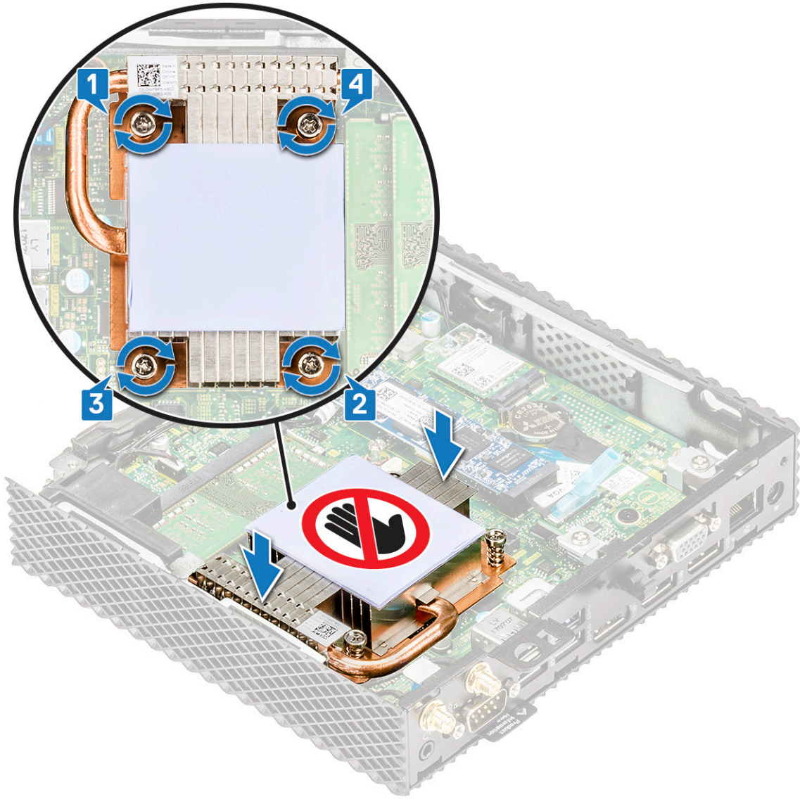
شكل 30. تركيب المشتت الحرارة
