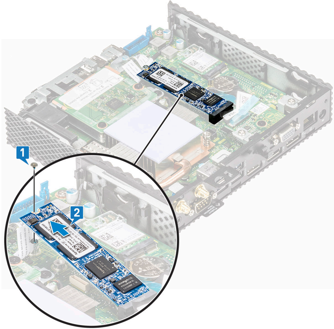
شكل 18. إزالة SSD
