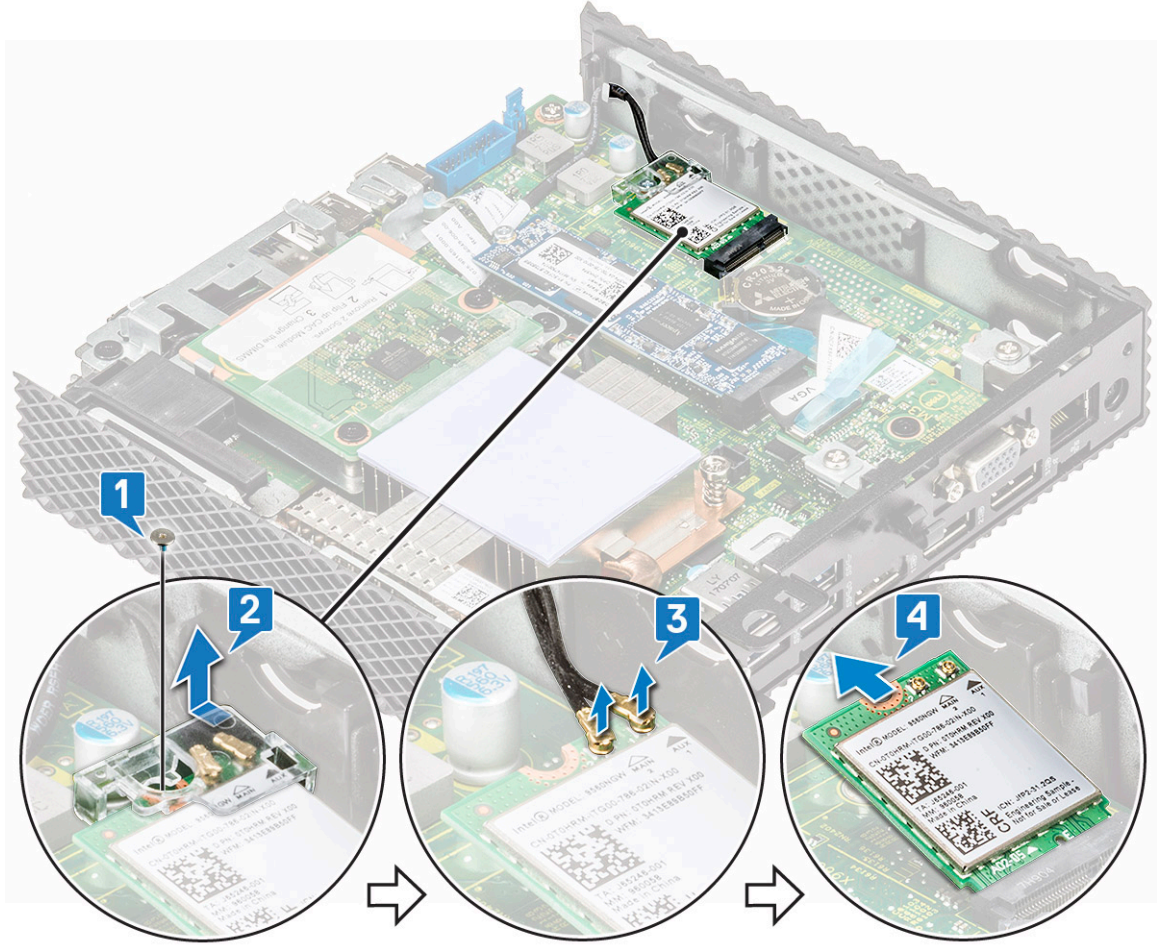
شكل 20. إزالة البطاقة اللاسلكية
