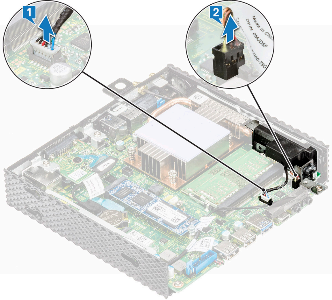
شكل 31. فصل الكبلين
