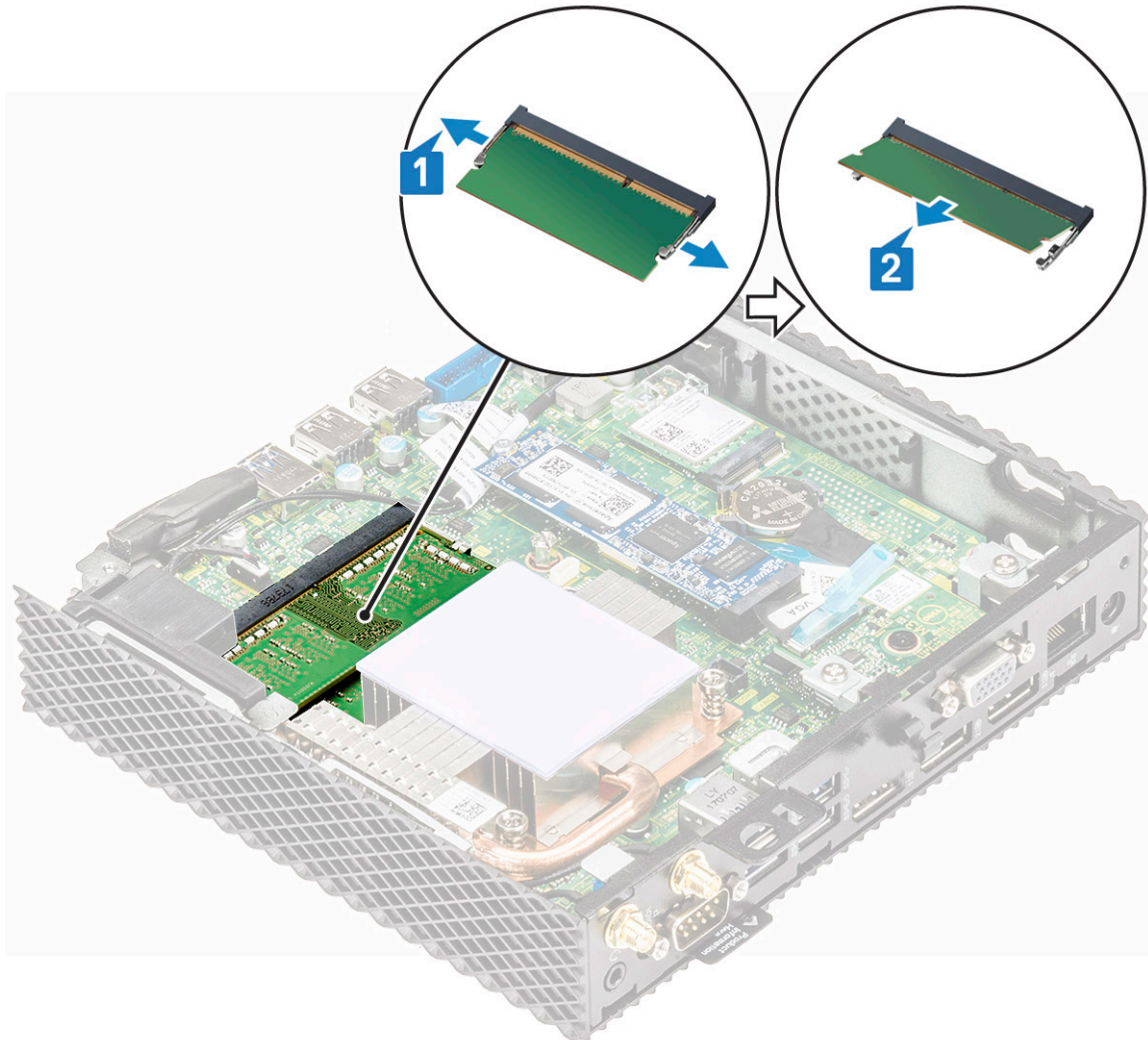
شكل 33. إزالة بطاقات الذاكرة
