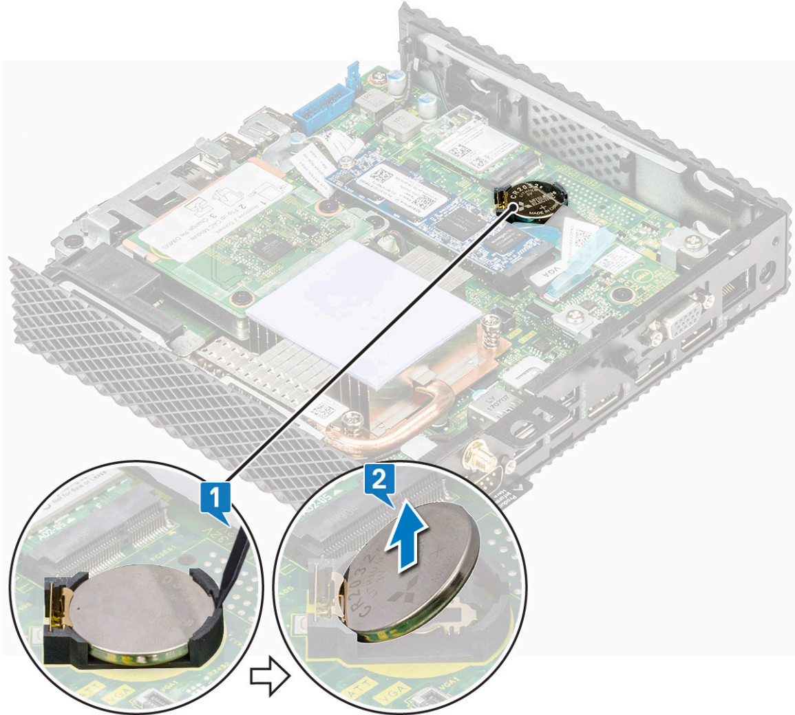
شكل 19. إزالة البطارية الخلية المصغرة
