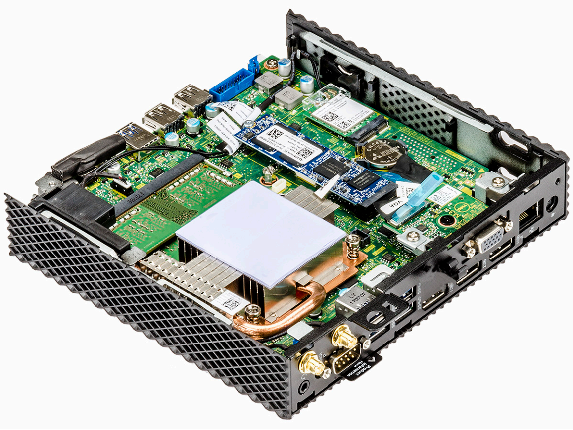
شكل 25. بعد إزالة حامل قارئ بطاقة الوصول المشترك
