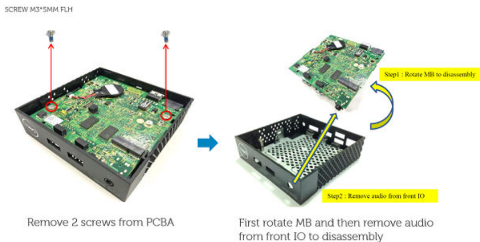
Figure 36. Retrait de la carte PCBA
