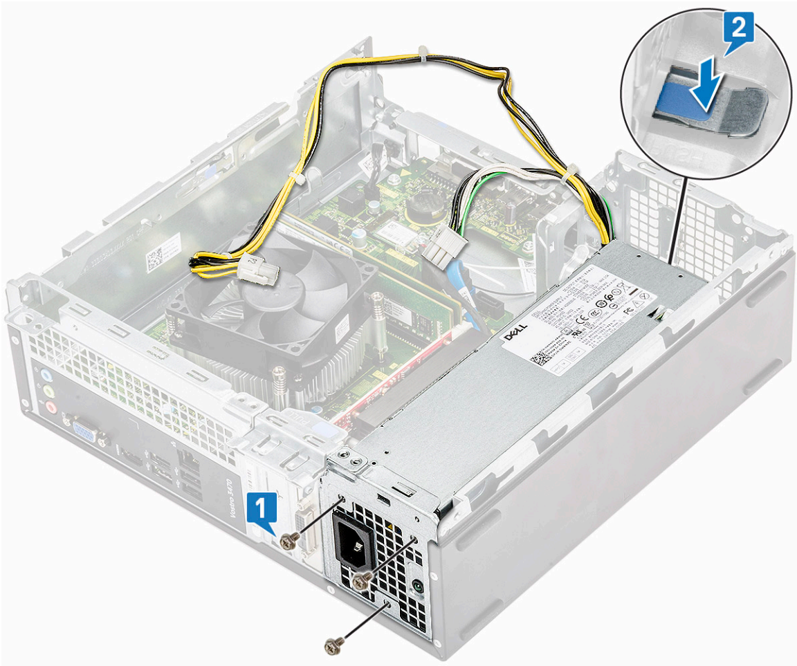
c) PSU를 밀어 컴퓨터에서 들어 올립니다.
