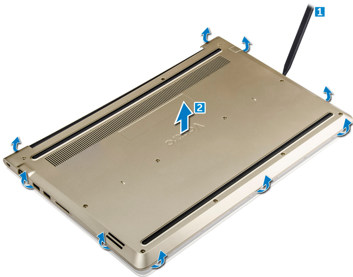
图 6: 撬动边缘以卸下后盖。
