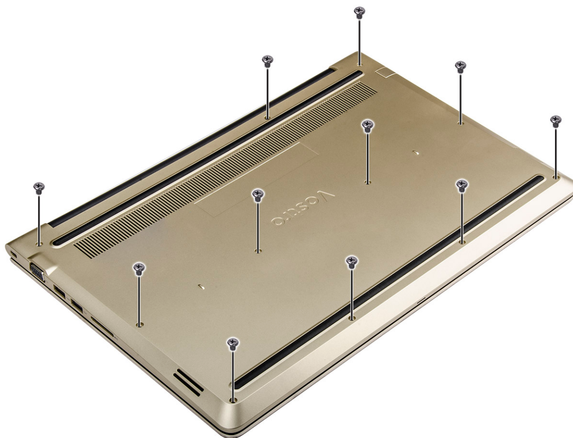
图 5: 拧下螺钉
