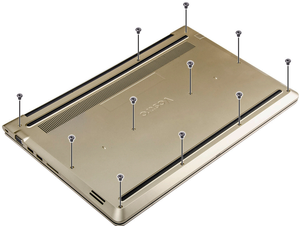
Figura 5. Rimozione delle viti
