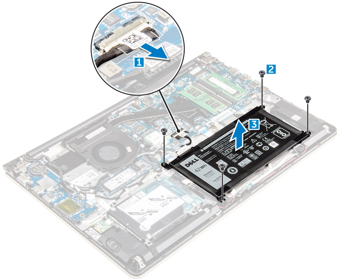
Abbildung 7. Entfernen des Akkus
