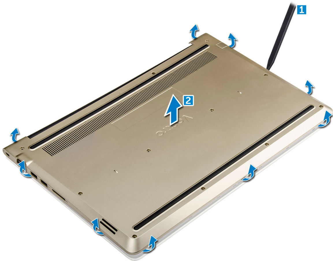
Abbildung 6. Hebeln an der Kante zum Entfernen der hinteren Abdeckung
