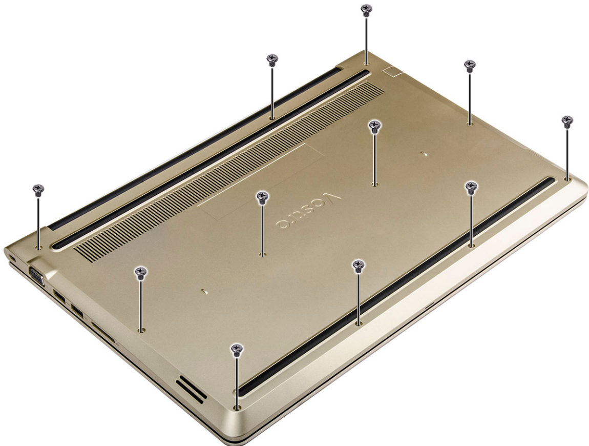
Abbildung 5. Entfernen der Schrauben
