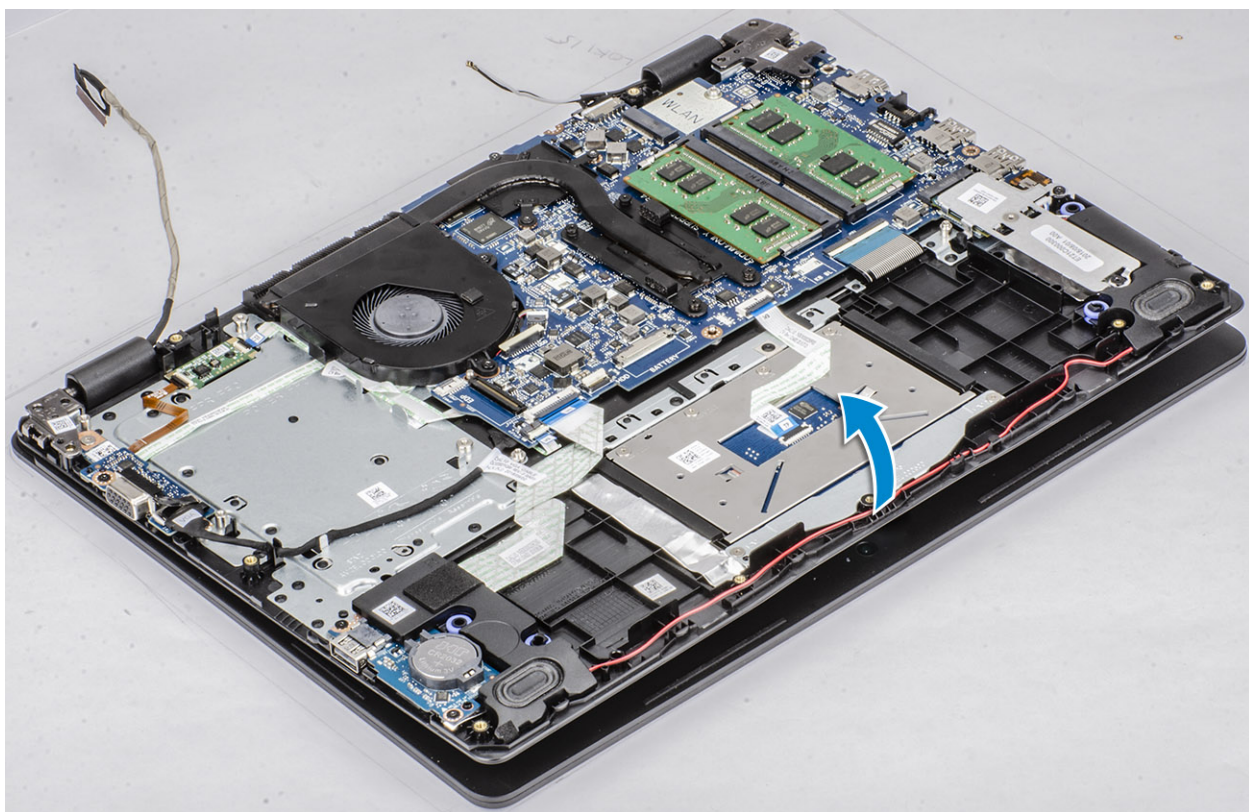
6 從顯示器組件拉出並卸下手掌墊和鍵盤組件。
