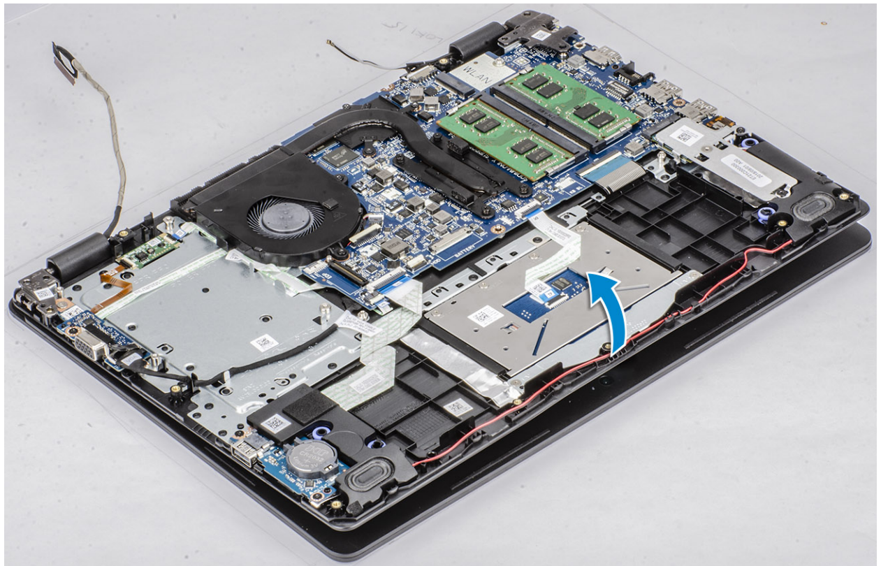
6 החלק והסר את מכלול משענת כף היד והמקלדת ממכלול הצג.
