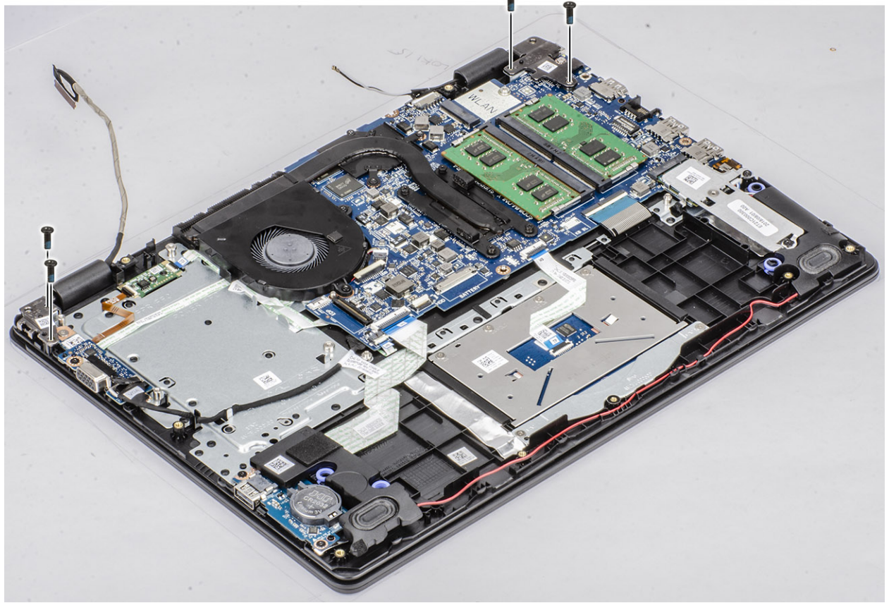
5 הרם בזווית את מכלול משענת כף היד והמקלדת.
