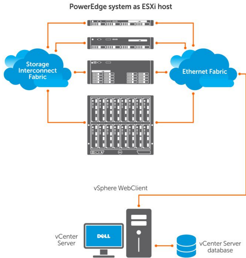
Abbildung 1. vSphere-Komponenten
