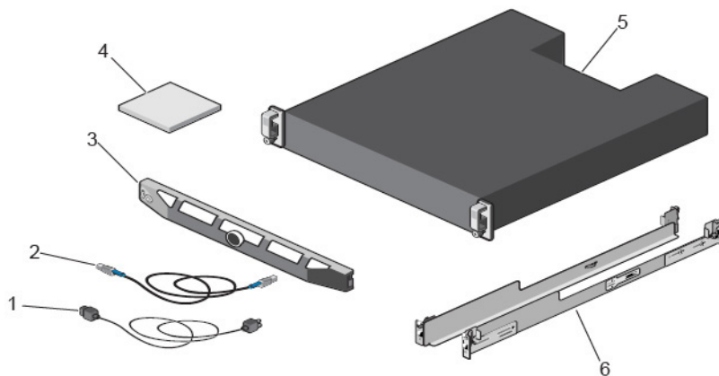
Abbildung 1. Komponenten des SCv300/SCv320-Erweiterungsgehäuse
