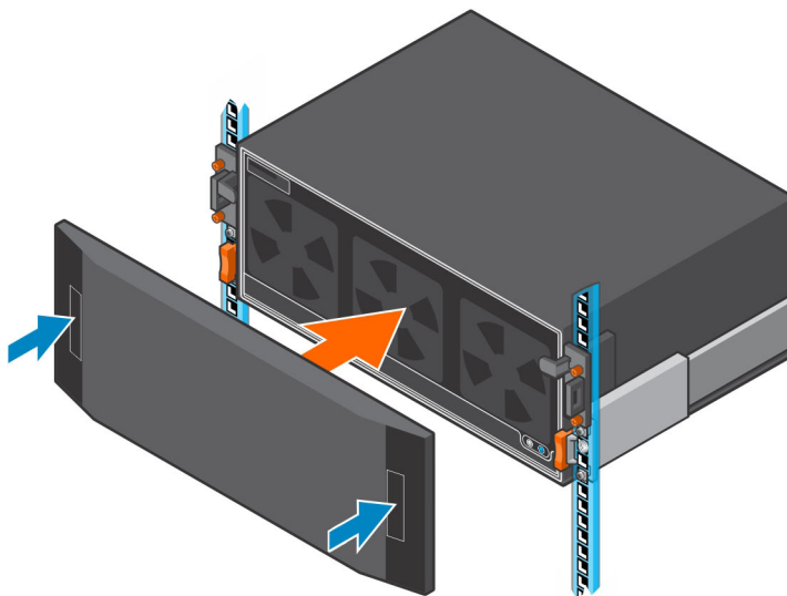
Slika 9. Instalirajte masku
