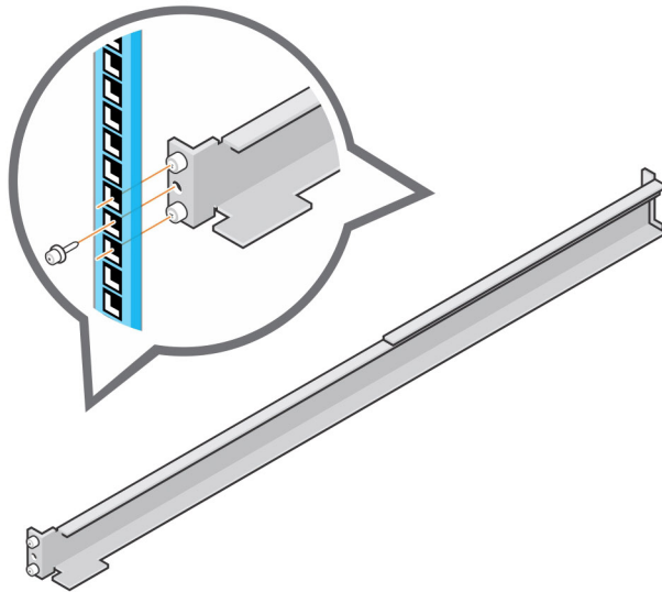
Figura 3. Como prender os trilhos no rack
