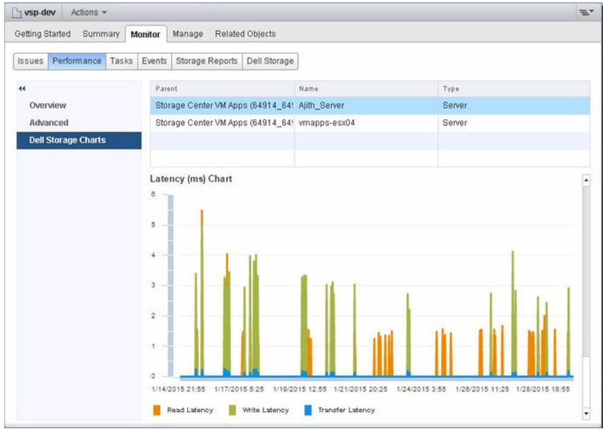
图 25: Storage Center 的延迟图表示例
