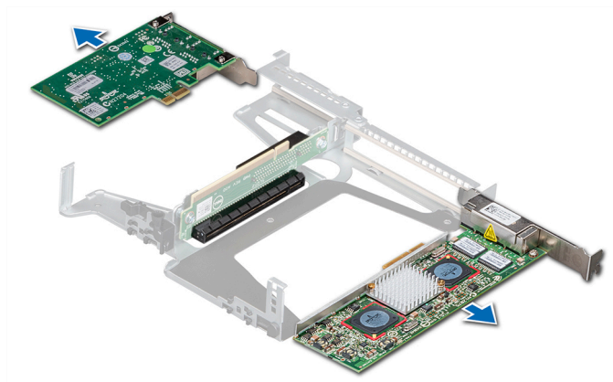
그림 40. 확장 카드 라이저에서 확장 카드 제거
