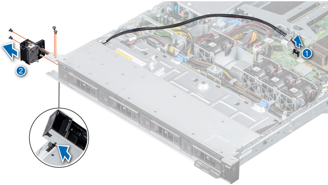
그림 66. 왼쪽 제어판 분리
