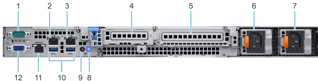
그림 2. 시스템의 후면 모습
