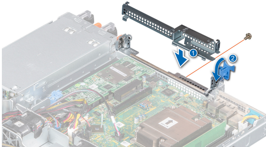
그림 38. 확장 카드 라이저 필러 설치
