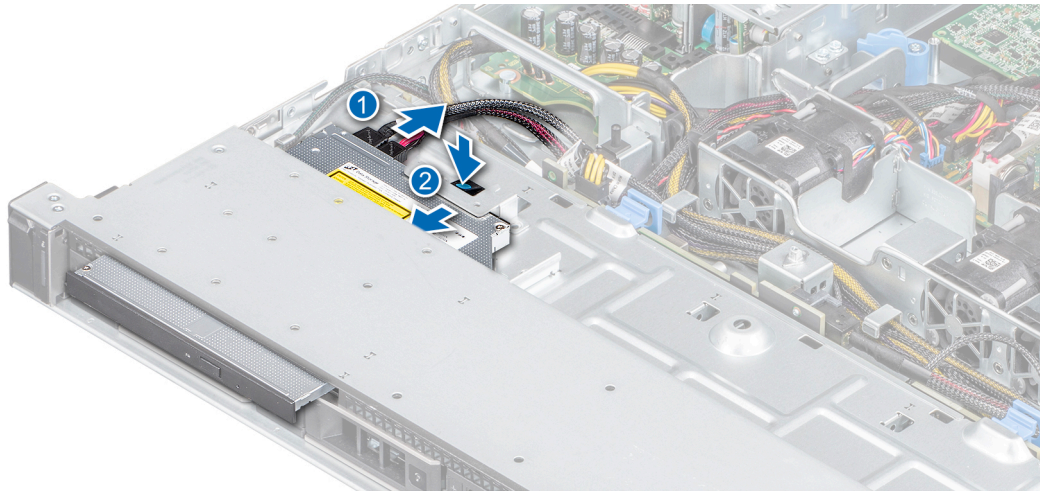
그림 47. 광학 드라이브 분리
