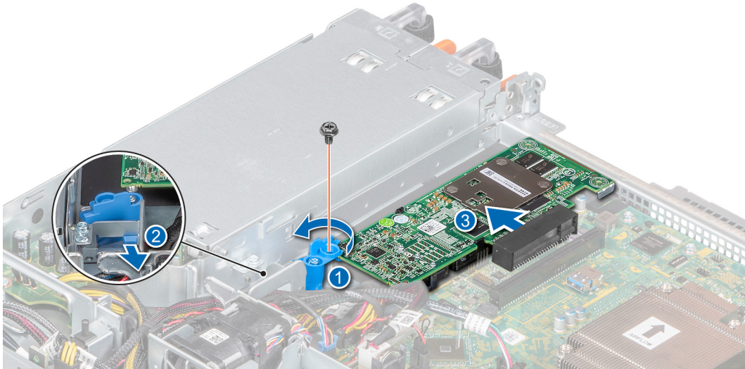
그림 43. PERC 카드 분리
