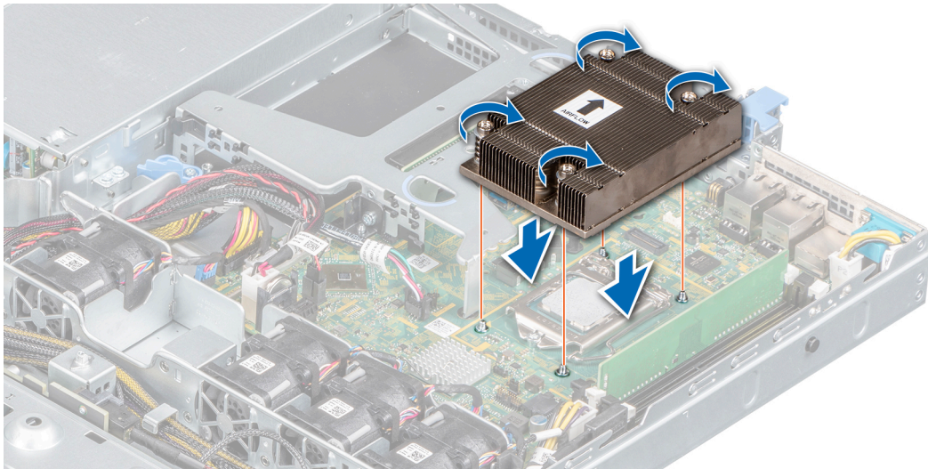
그림 53. 방열판 설치
