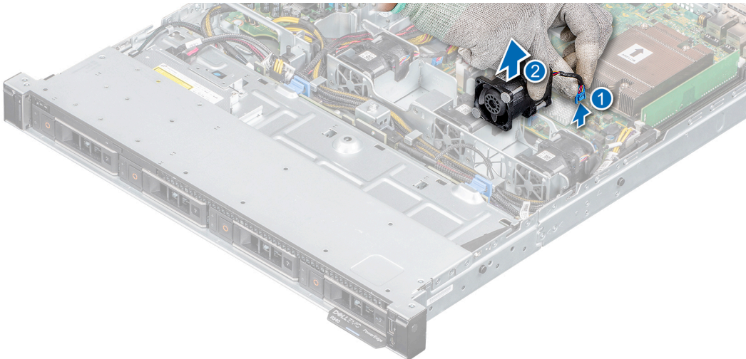
그림 28. 냉각 팬 분리
