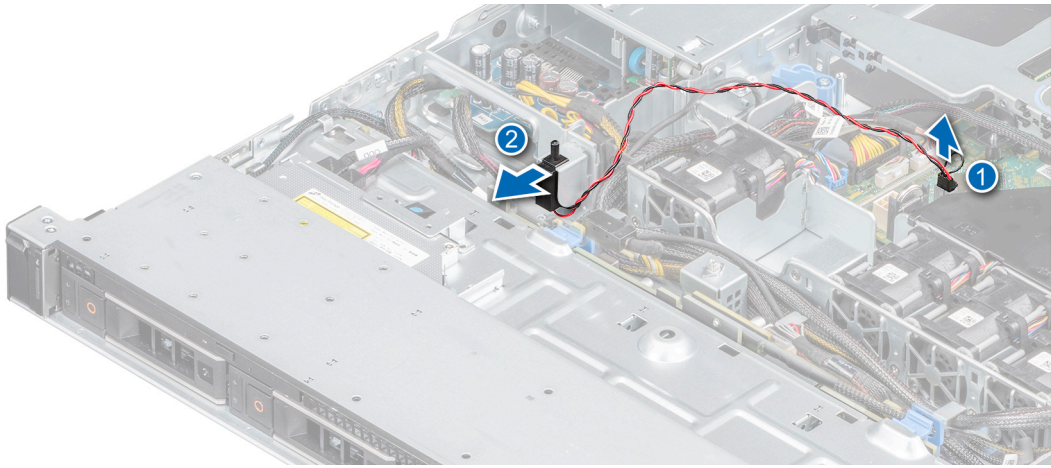
그림 30. 침입 스위치 제거
