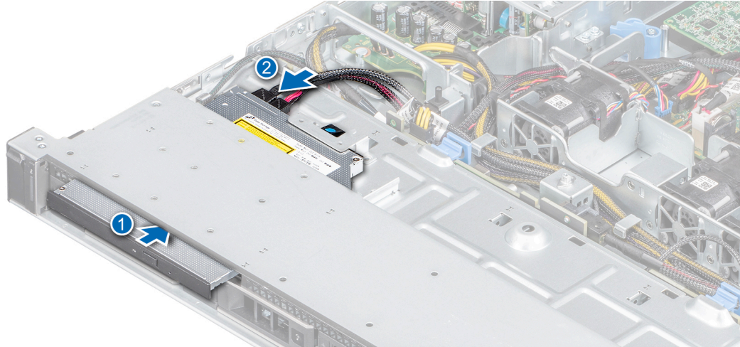
그림 48. 광학 드라이브 설치
