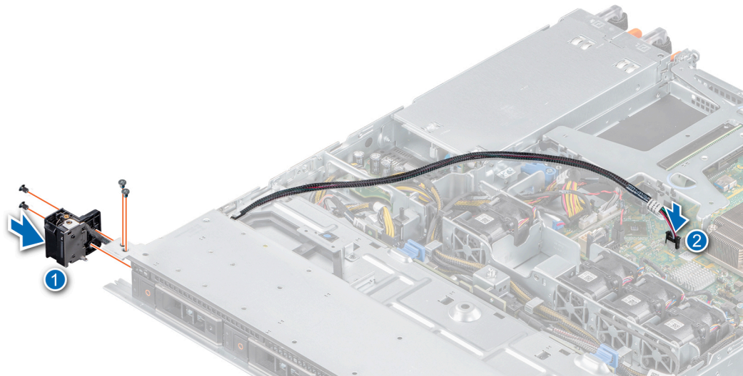
그림 67. 왼쪽 제어판 설치
