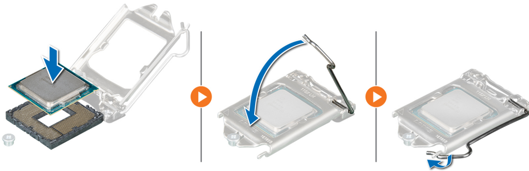
그림 51. 프로세서 장착
