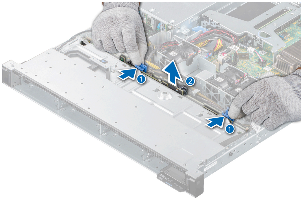
그림 54. 드라이브 백플레인 제거
