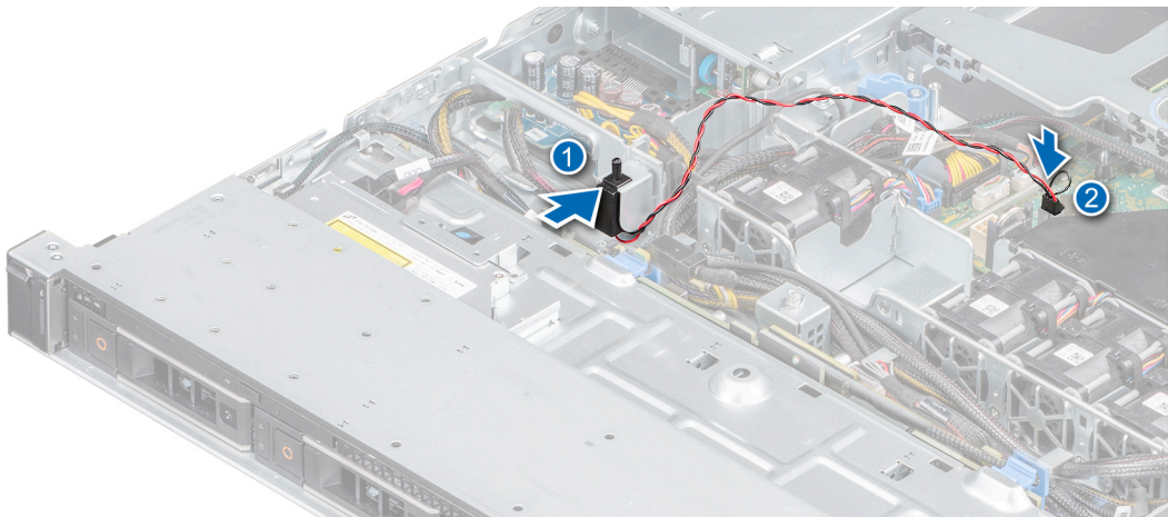
그림 31. 침입 스위치 설치
