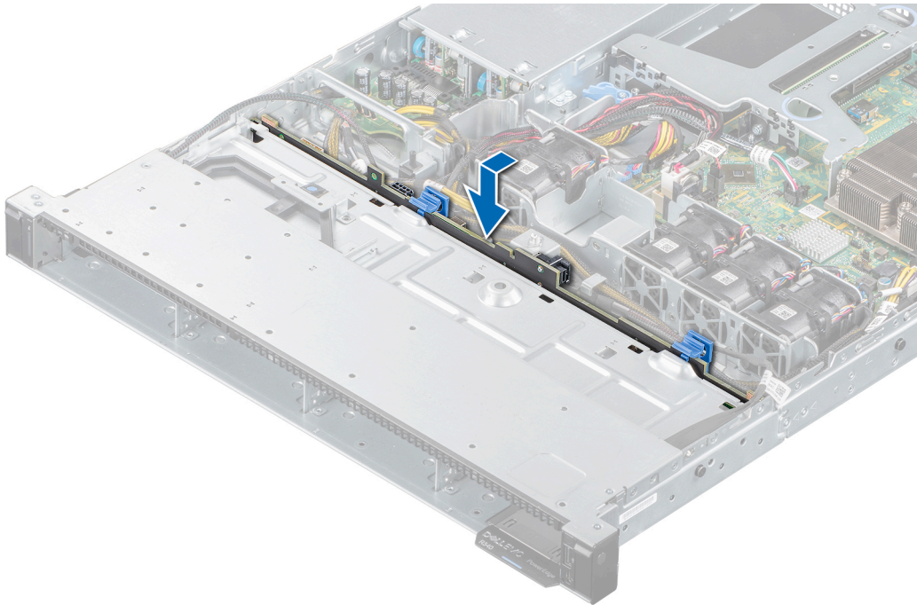
그림 55 . 드라이브 백플레인 설치
