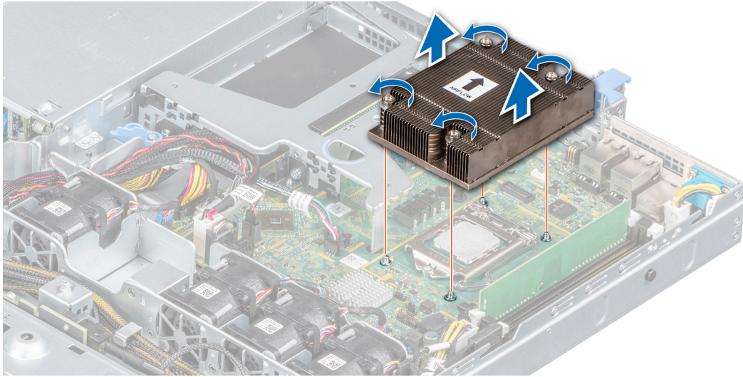
그림 49. 방열판 분리
