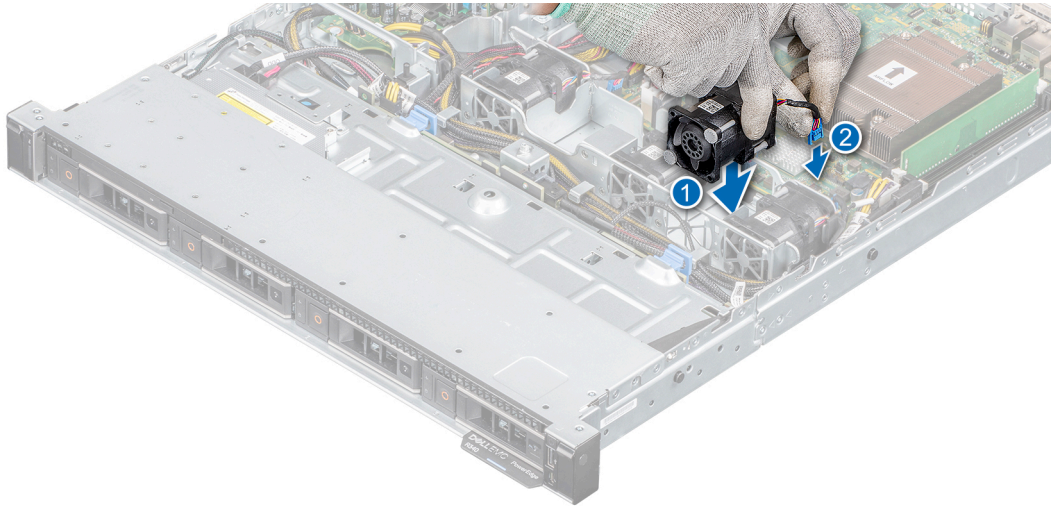
그림 29. 냉각 팬 설치
