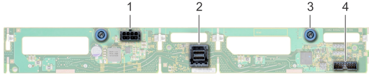
그림 79 . 8.89cm(3.5인치) 백플레인의 후면 모습(후면 드라이브 케이징)
