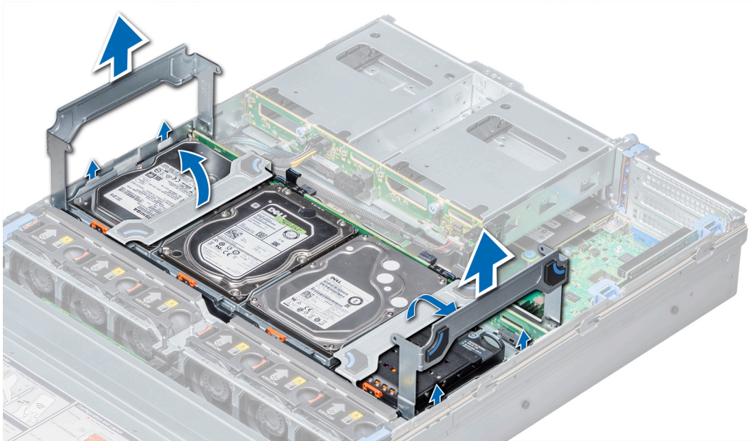
그림 24. 중간 드라이브 트레이 제거
