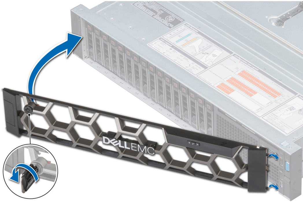
그림 11. LCD 패널을 포함하는 전면 베젤 설치
