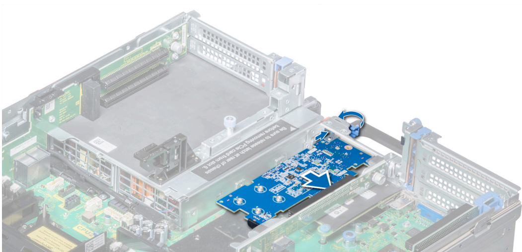
그림 61. 확장 카드 라이저 2B에 확장 카드 설치
