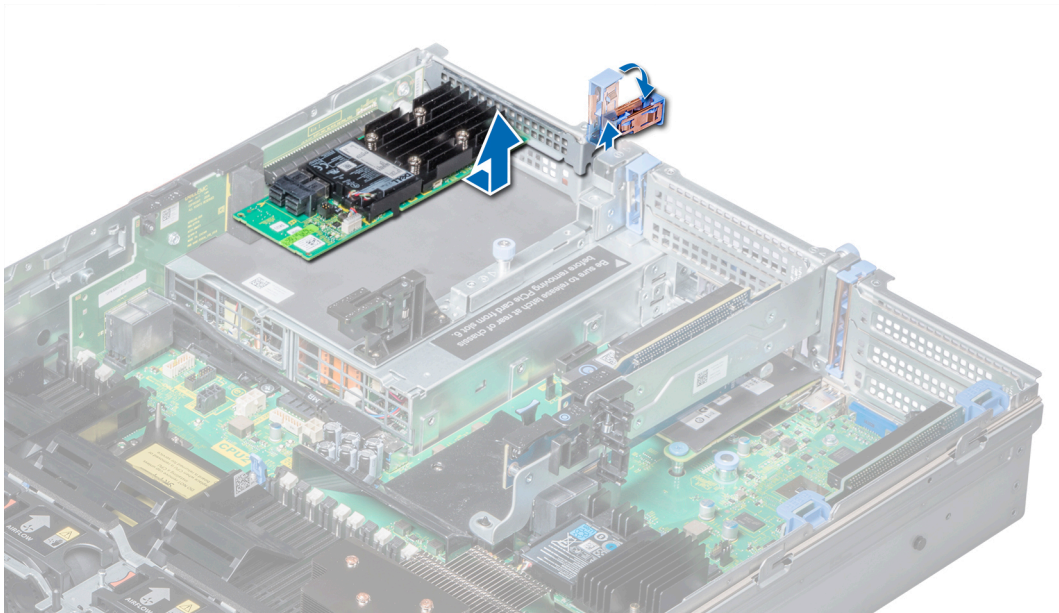
그림 59 . 확장 카드 라이저 3에서 확장 카드 제거
