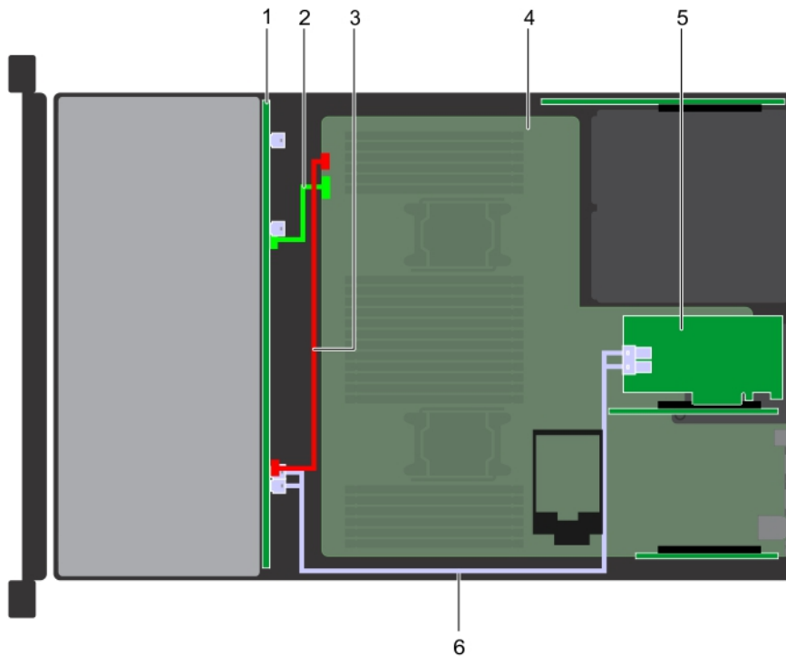
그림 87 . 12개의 8.89cm(3.5인치) 백플레인(어댑터 PERC 포함)
