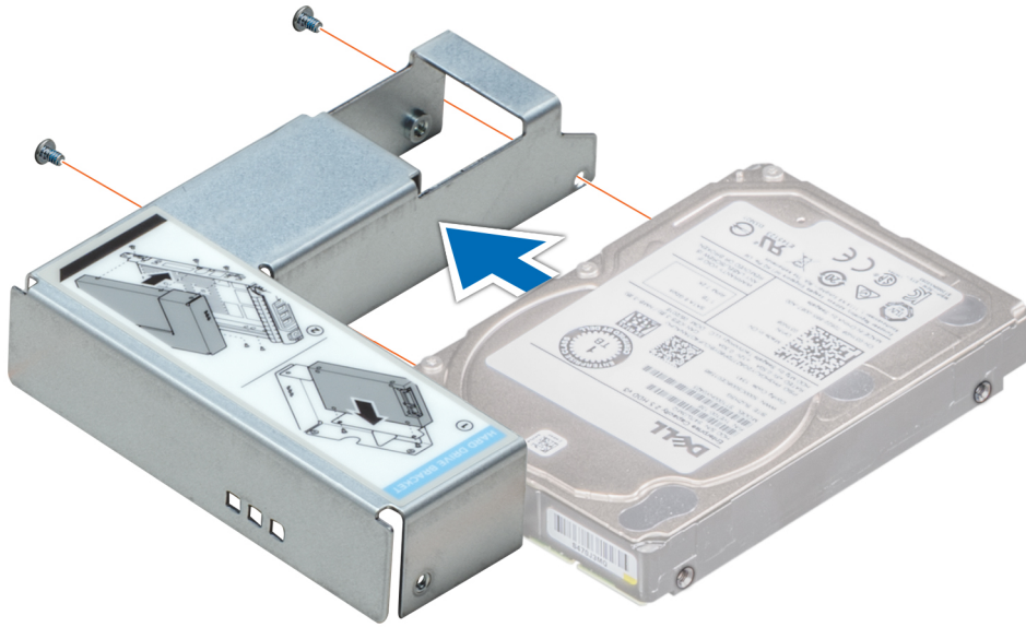
그림 37. 3.5" 드라이브 어댑터에 2.5" 드라이브 설치
