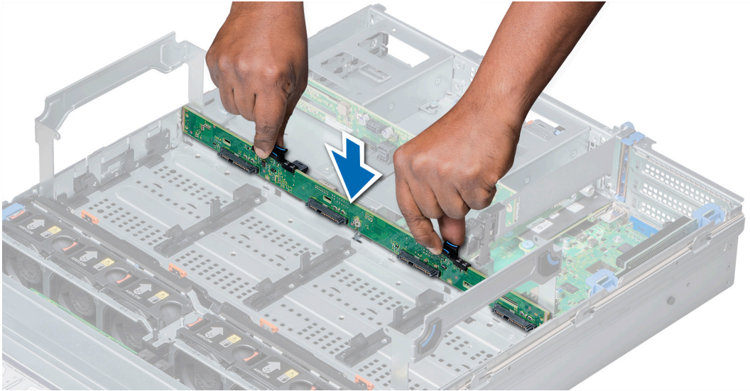
그림 83. 중간 드라이브 백플레인 설치
