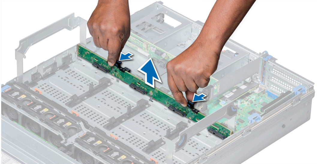
그림 82 . 중간 드라이브 백플레인 제거
