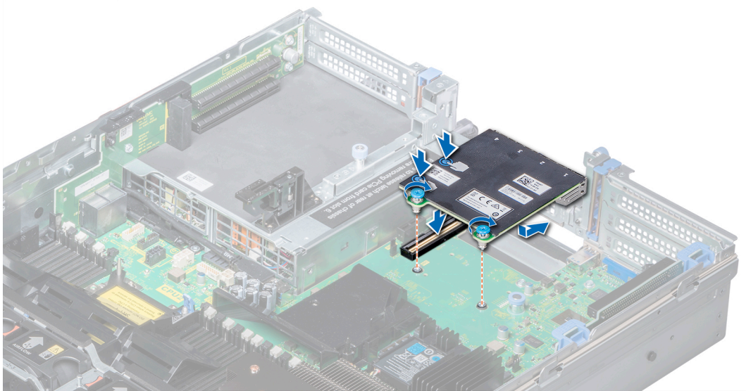
그림 71. 네트워크 도터 카드 설치
