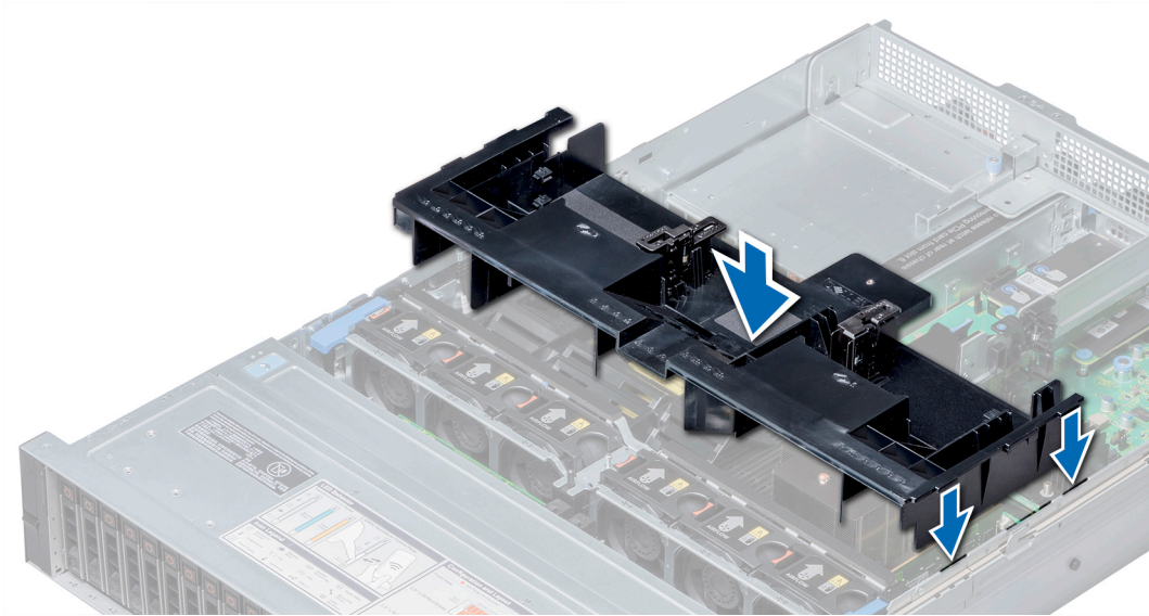
그림 17. 공기 덮개 장착
