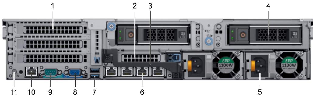
그림 5. 2개의 3.5" 드라이브 시스템의 후면
