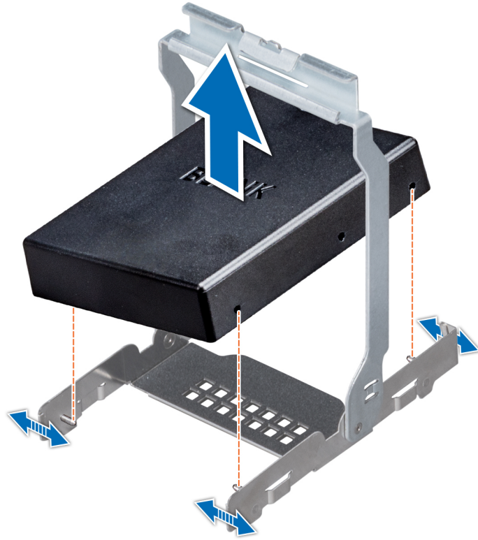
그림 26. 중간 드라이브 캐리어에서 드라이브 보호물 제거
