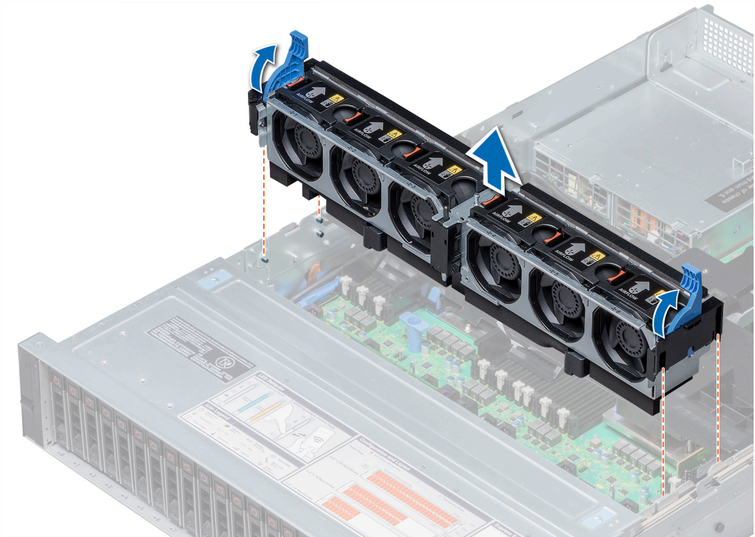
그림 18. 냉각 팬 조립품 분리
