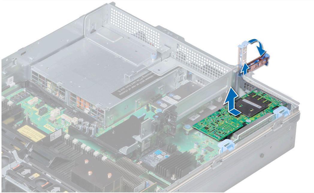
그림 56. 확장 카드 라이저 1에서 확장 카드 제거
