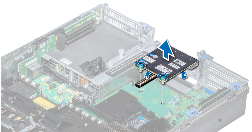
그림 70. 네트워크 도터 카드 분리
