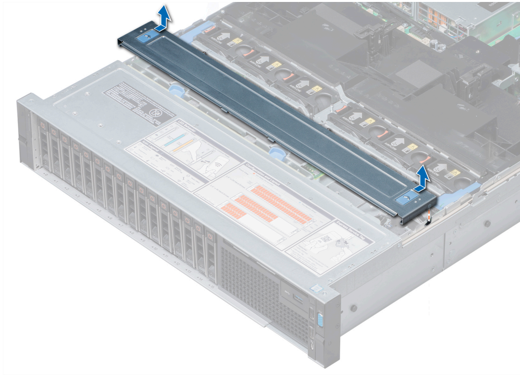
그림 14 . 백플레인 커버 제거
