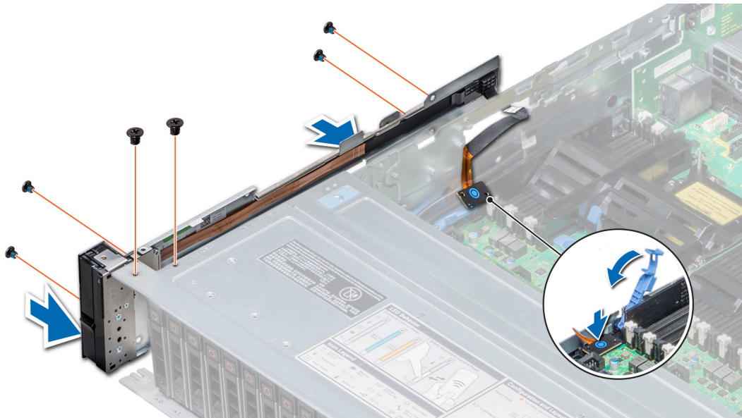
그림 100 . 왼쪽 컨트롤 패널 설치
