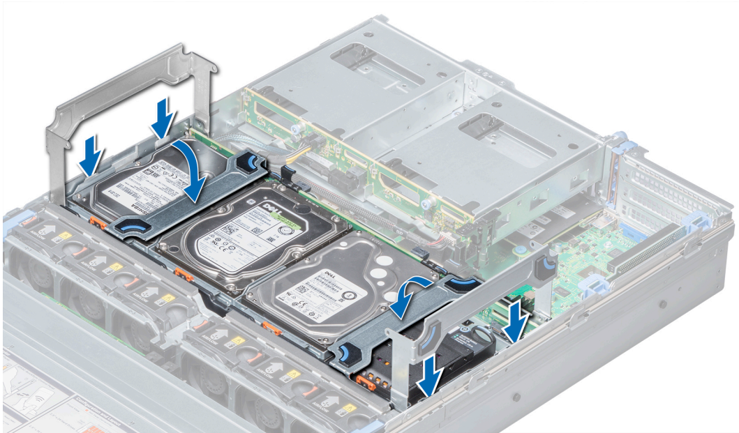
그림 25 . 중간 드라이브 트레이 설치
