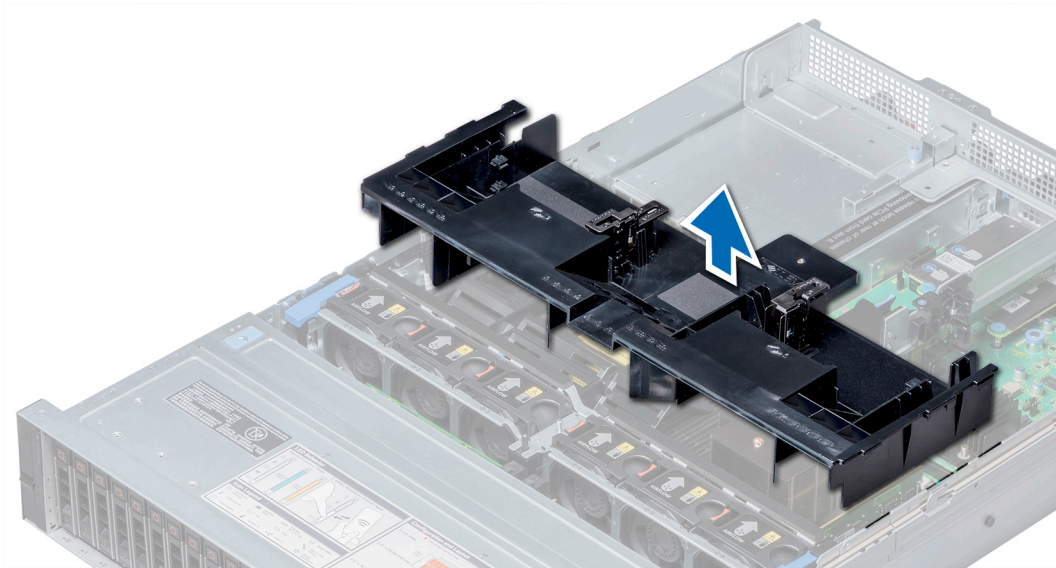
그림 16. 공기 덮개 분리
