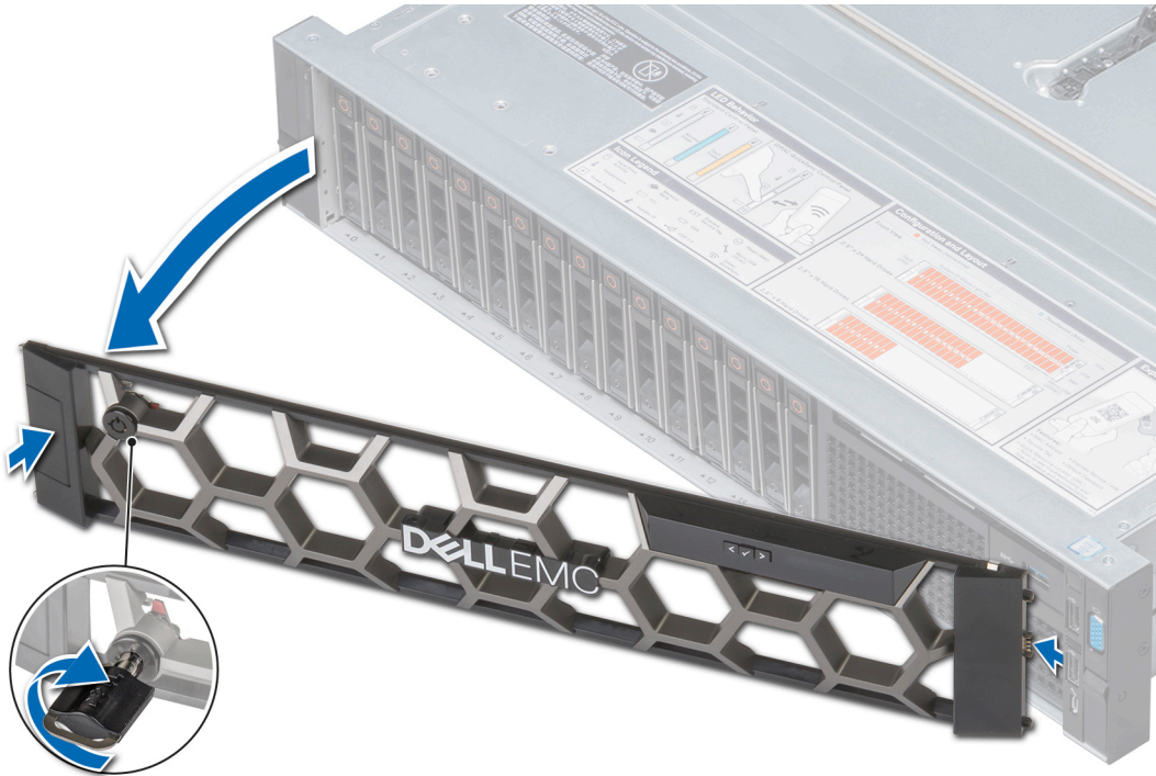
그림 10 . LCD 패널을 포함하는 전면 베젤 제거
