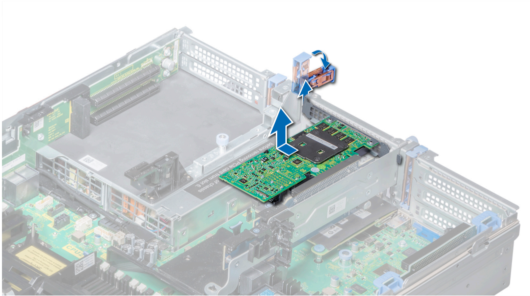
그림 58 . 확장 카드 라이저 2에서 확장 카드 제거
