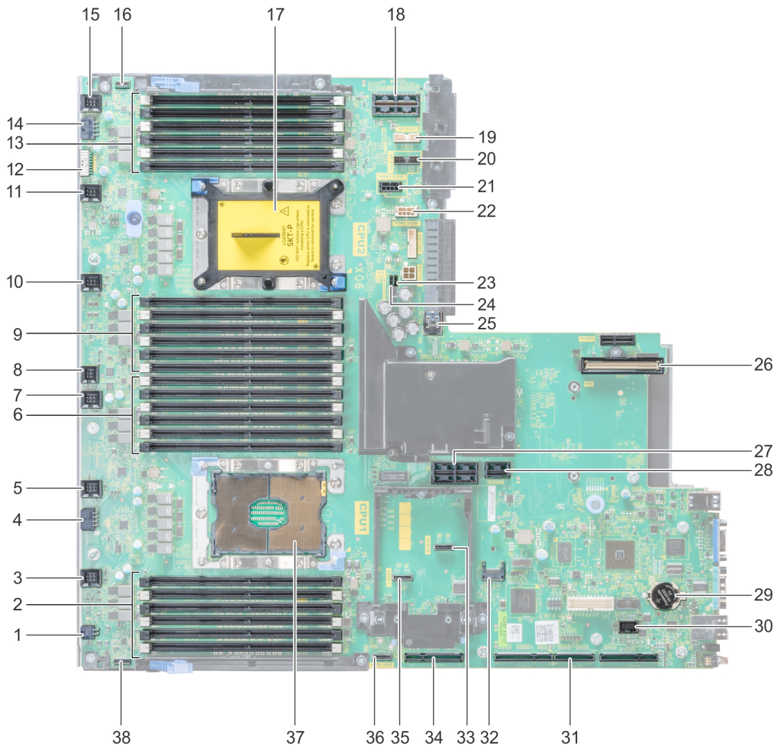
그림 108 . 시스템 보드 점퍼 및 커넥터
