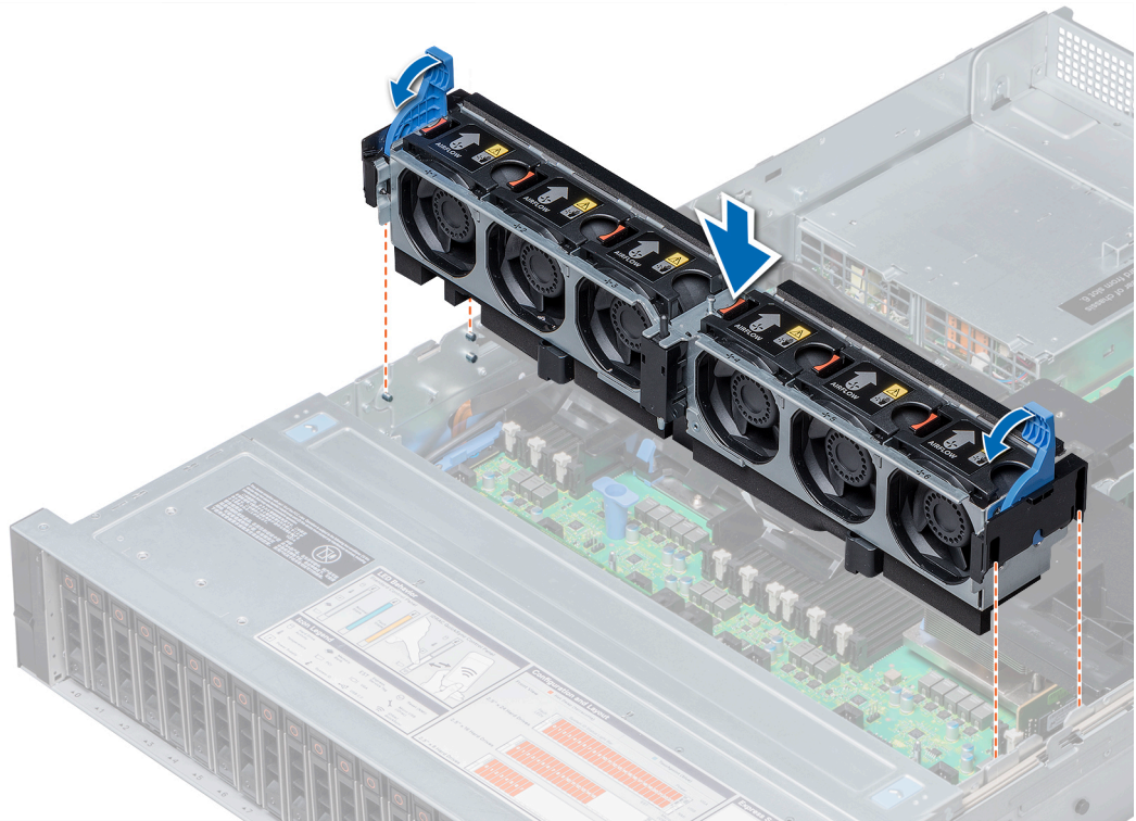
그림 19. 냉각 팬 조립품 설치
