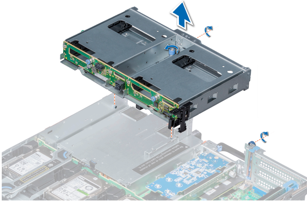
그림 42. 2개의 8.89cm(3.5인치) 후면 드라이브 케이스 제거
