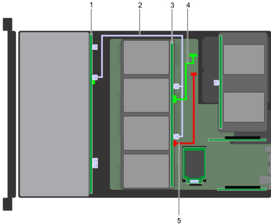
그림 89 . 케이블 라우팅 - 12개의 8.89cm(3.5인치) 백플레인을 포함하는 4개의 8.89cm(3.5인치) 중간 백플레인
