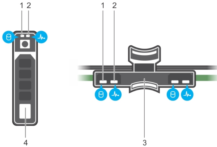
그림 103. 드라이브 및 중간 드라이브 트레이 백플레인의 드라이브 표시등
