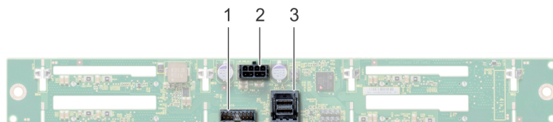
그림 78 . 6.35cm(2.5인치) 백플레인의 후면 모습(후면 드라이브 케이스)
