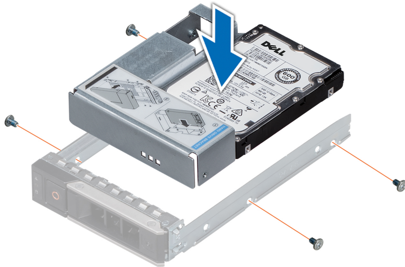
그림 39 . 8.89cm(3.5인치) 드라이브 캐리어에 8.89cm(3.5인치) 어댑터 설치
