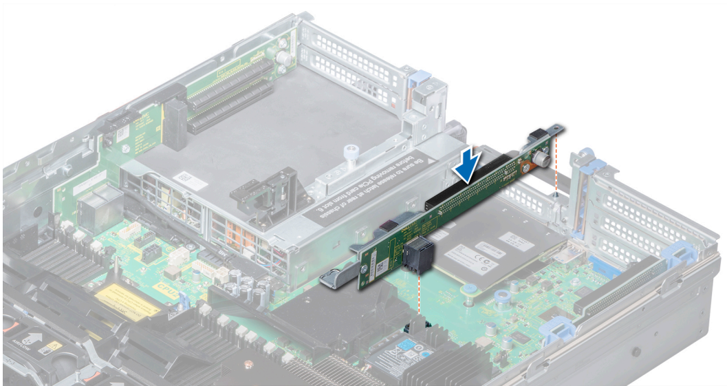
그림 69. 확장 카드 라이저 2 설치
