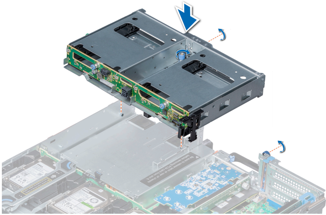
그림 43. 2개의 8.89cm(3.5인치) 후면 드라이브 케이지 설치
