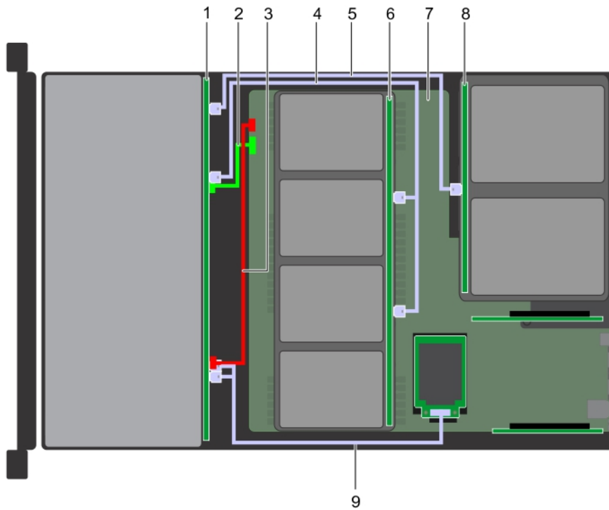
그림 88 . 케이블 라우팅 - 4개의 8.89cm(3.5인치) 중간 드라이브 트레이 및 2개의 8.89cm(3.5인치) 후면 드라이브 케이지를 포함하는 12개의 3.5인치 백플레인
