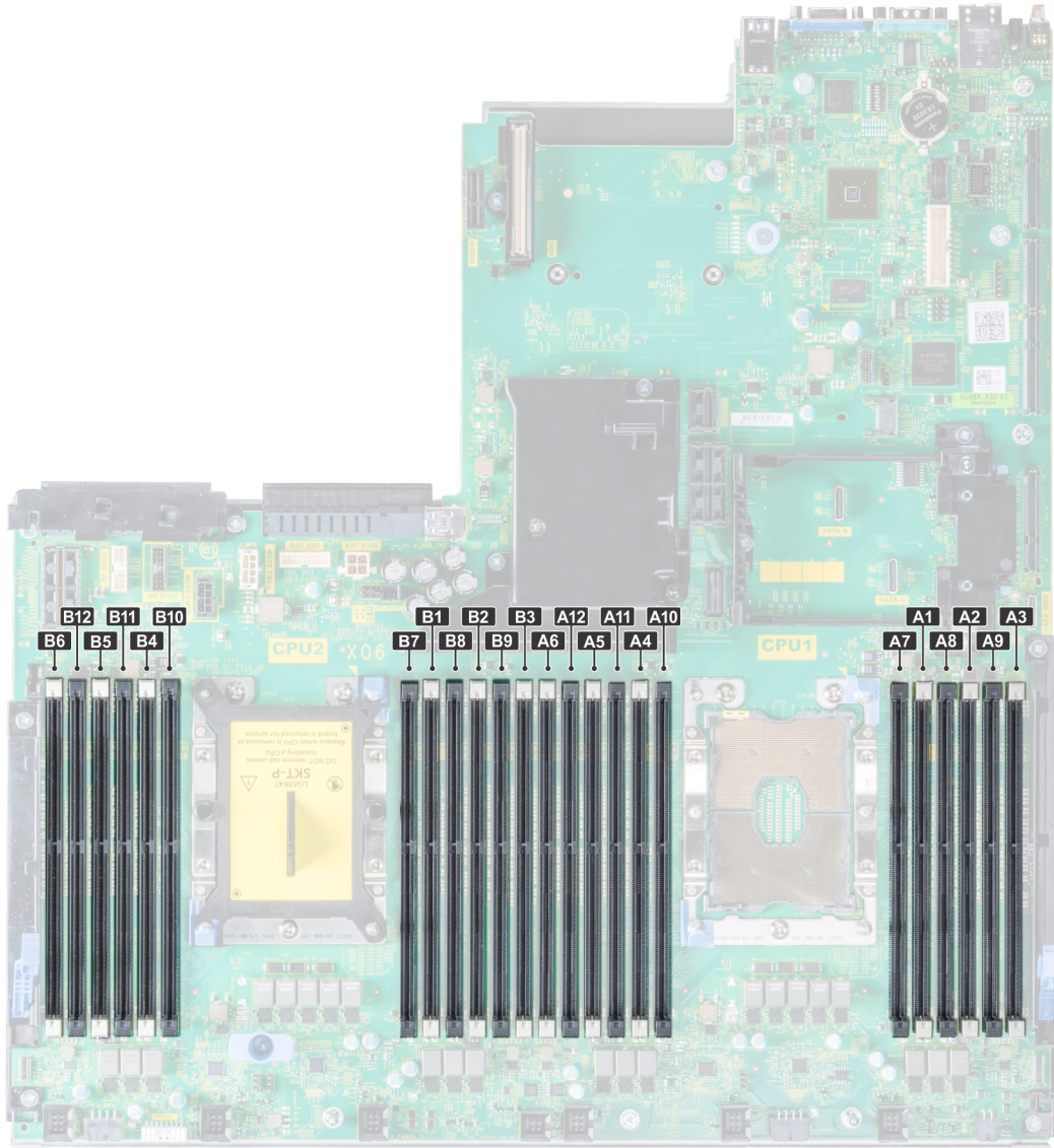
그림 44 . 시스템 메모리 모습
