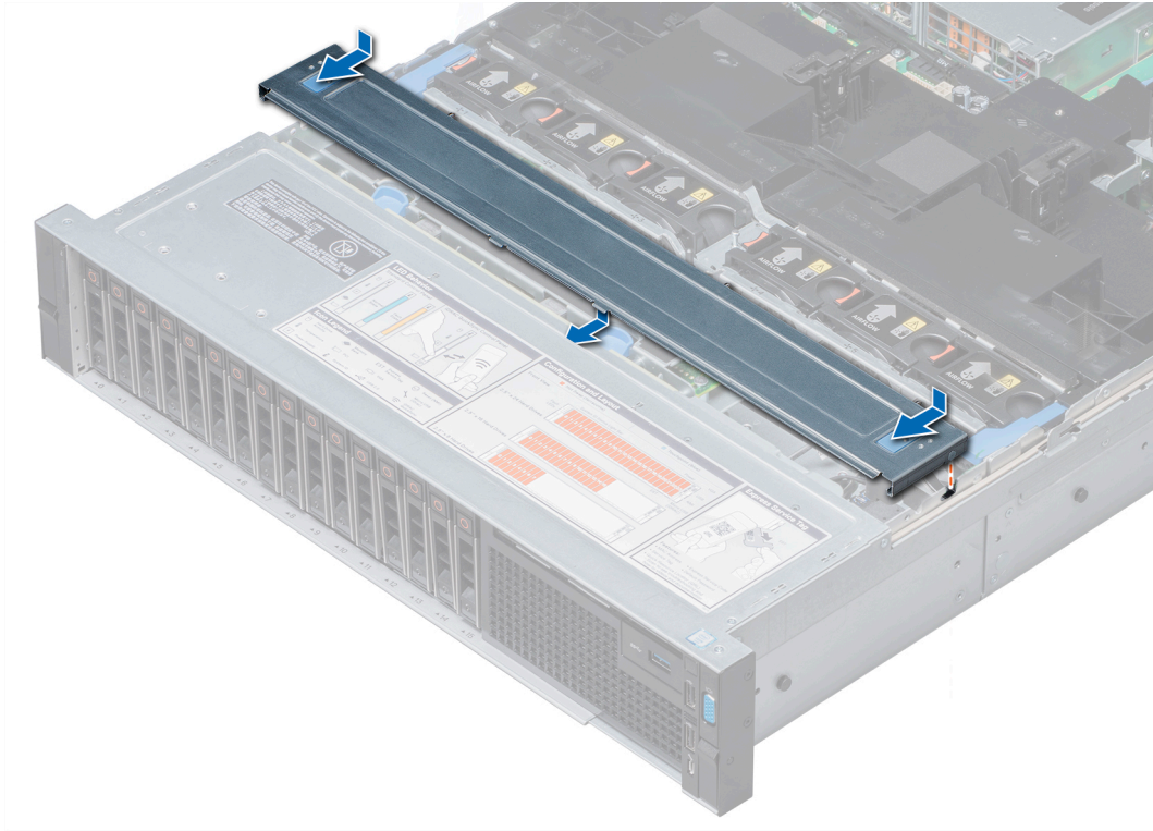
그림 15. 백플레인 커버 설치
