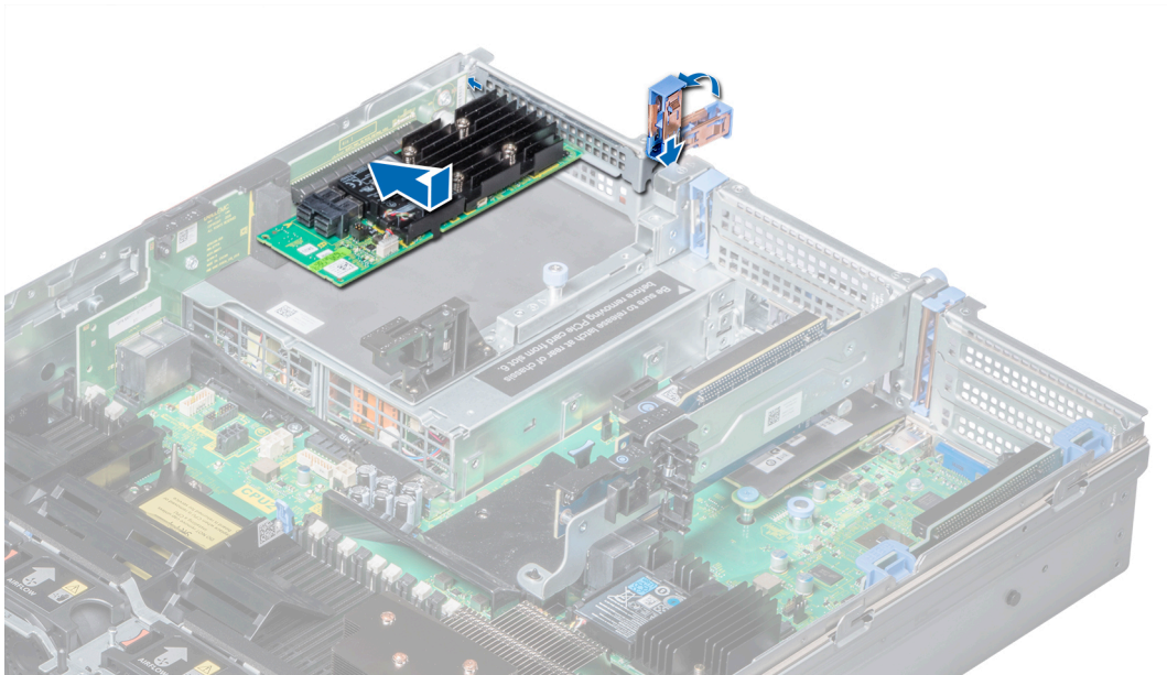
그림 63. 확장 카드 라이저 3에 확장 카드 설치
