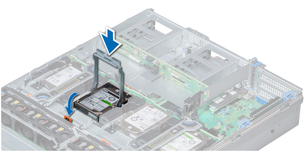
그림 29 . 중간 드라이브 트레이에 드라이브 캐리어 설치
