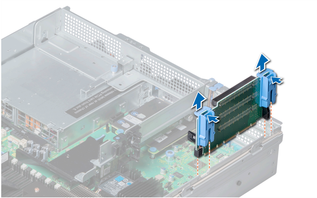
그림 66. 확장 카드 라이저 1 분리
