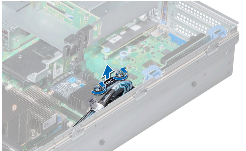
그림 72. 내장형 스토리지 컨트롤러 케이블 제거
