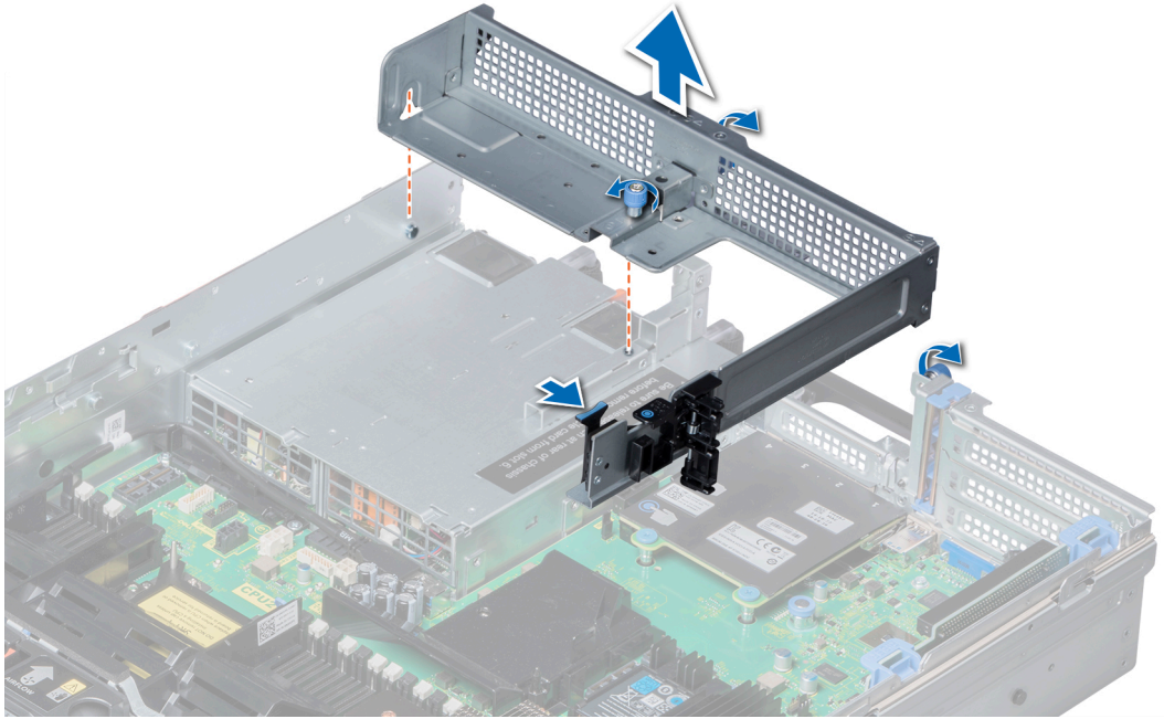
그림 64 . 라이저 2 보호물 제거
