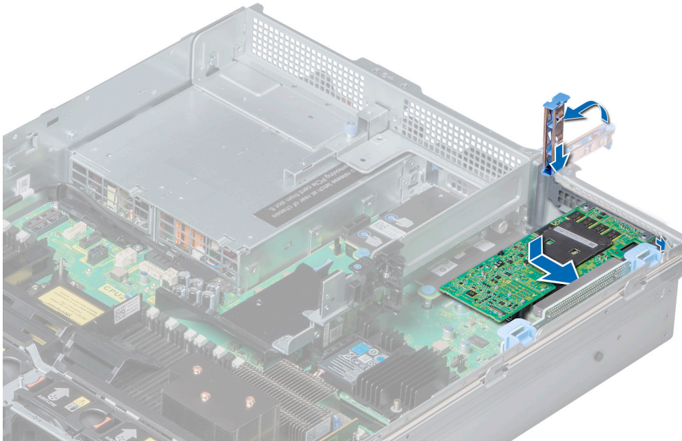
그림 60. 확장 카드 라이저 1에 확장 카드 설치
