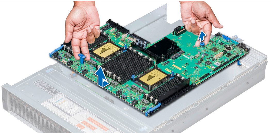
그림 96. 시스템 보드 분리
