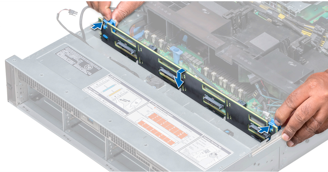
그림 81. 후면판 설치
