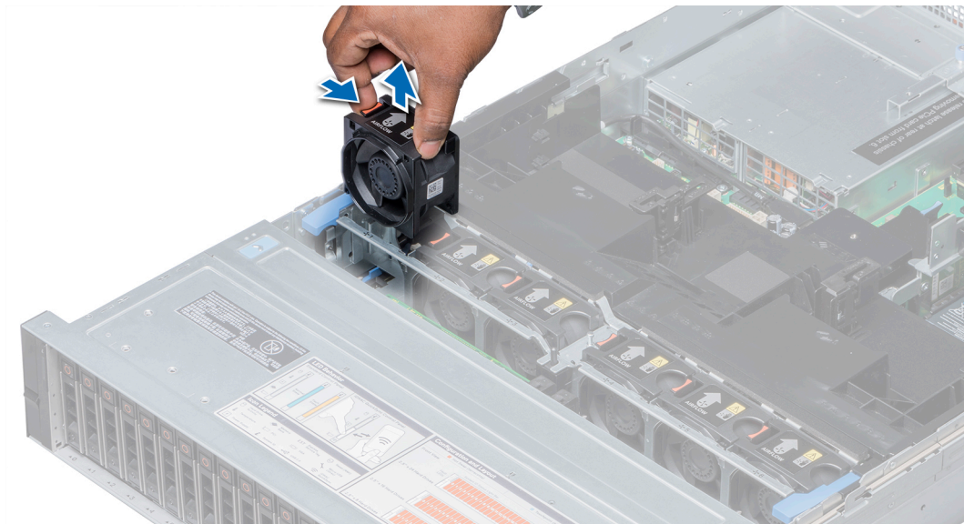
그림 20. 냉각 팬 분리
