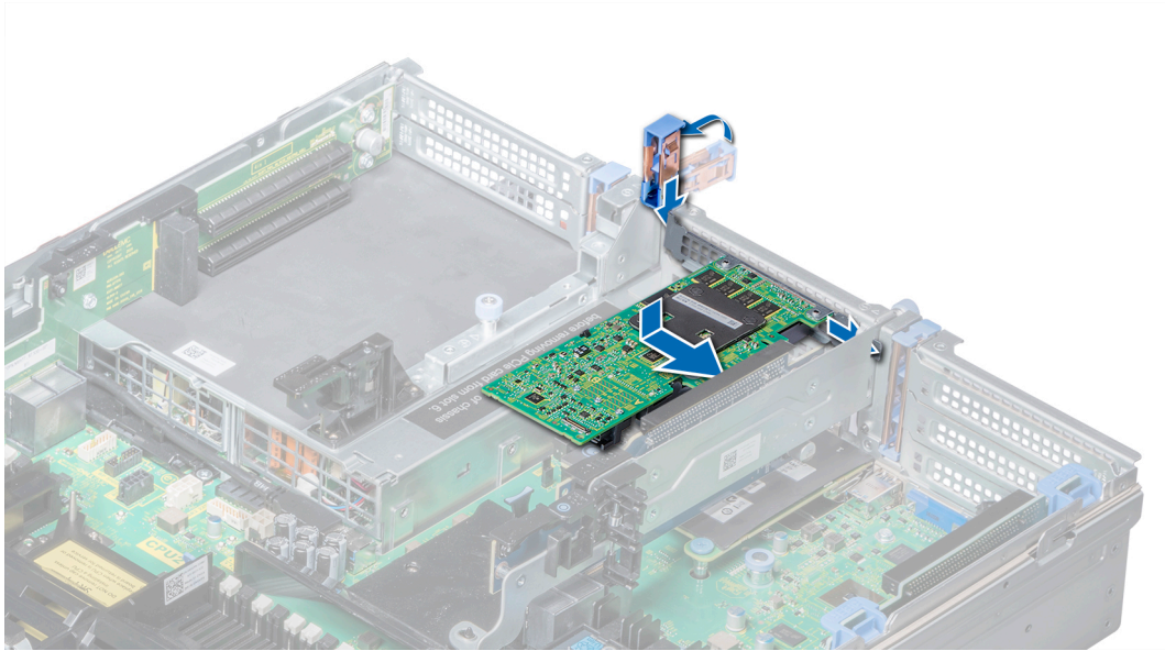
그림 62. 확장 카드 라이저 2에 확장 카드 설치
