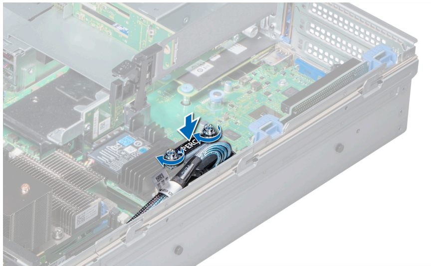
그림 75. 내장형 스토리지 컨트롤러 카드 케이블 설치
