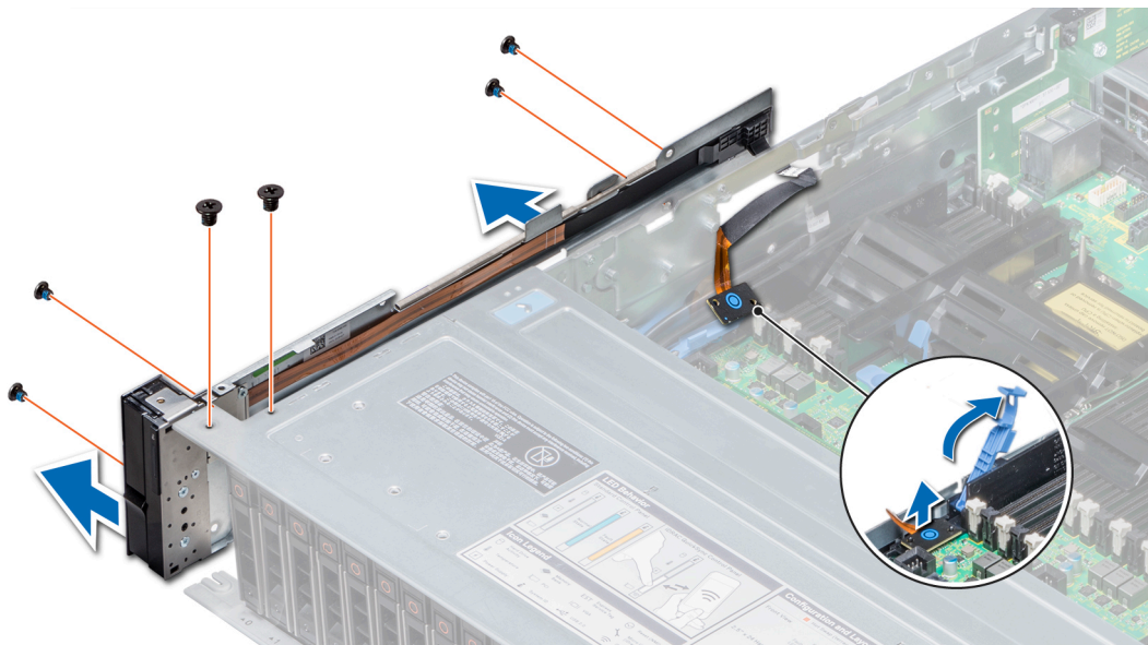
그림 99. 왼쪽 제어판 분리
