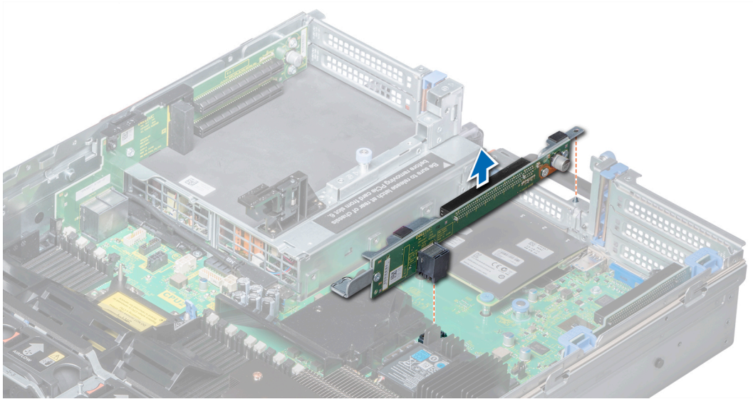
그림 68. 확장 카드 라이저 2 제거
