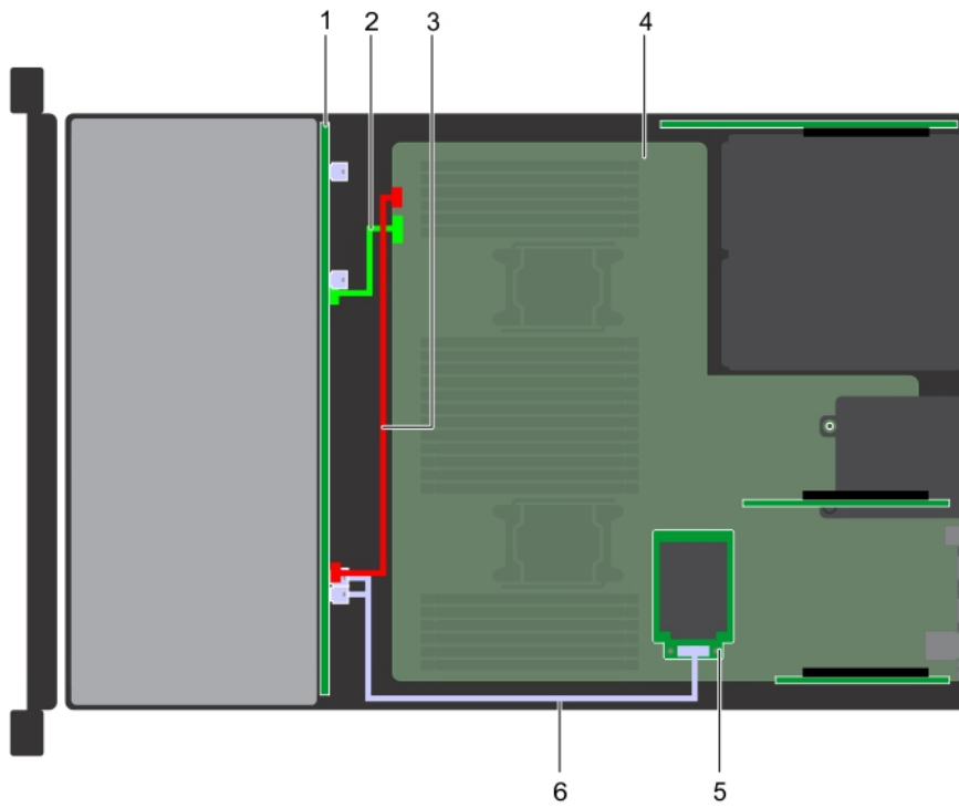
그림 86 . 케이블 라우팅 - 12개의 8.89cm(3.5인치) 백플레인(미니 PERC 포함)
