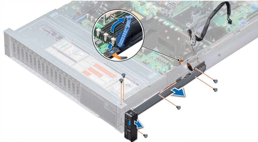
그림 101. 오른쪽 컨트롤 패널 제거
