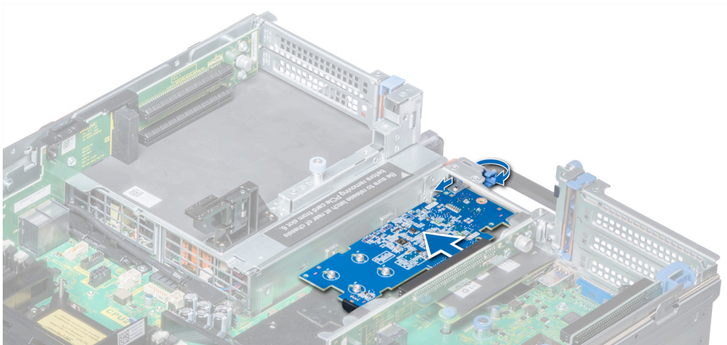
그림 57. 확장 카드 라이저 2B에서 확장 카드 제거
