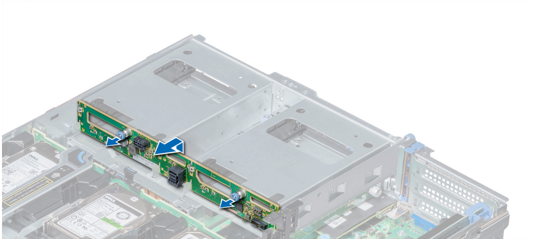
그림 84 . 8.89cm(3.5인치) 후면 드라이브 백플레인 제거
