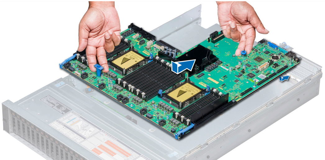
그림 97. 시스템 보드 설치
