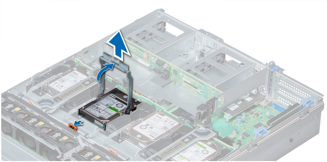
그림 28. 중간 드라이브 트레이에서 드라이브 캐리어 제거
