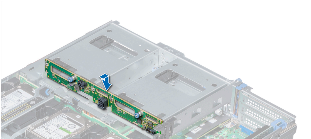
그림 85 . 8.89cm(3.5인치) 후면 드라이브 백플레인 설치
