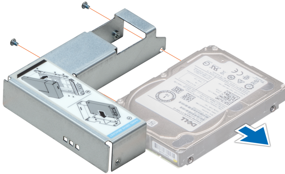
그림 36 . 3.5" 드라이브 어댑터에서 2.5" 드라이버 제거
