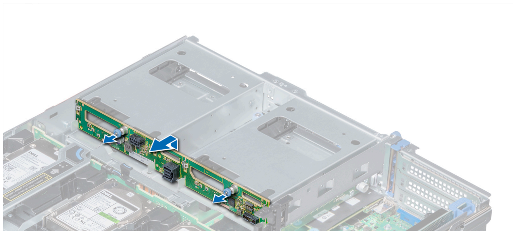
図 84. 3.5 インチ背面ドライブ バックプレーンの取り外し
