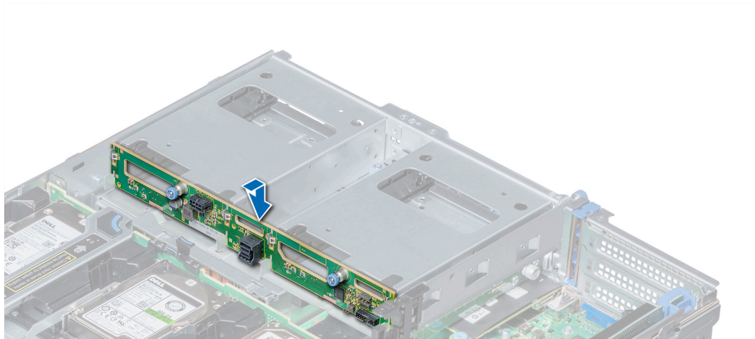
図 85. 3.5 インチ背面ドライブ バックプレーンの取り付け
