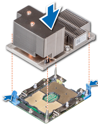
図 53. プロセッサとヒートシンクモジュールの取り付け
