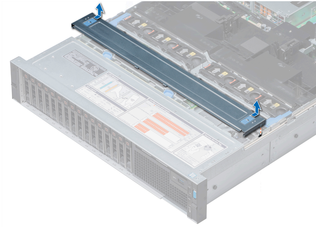
図 14. バックプレーン カバーの取り外し
