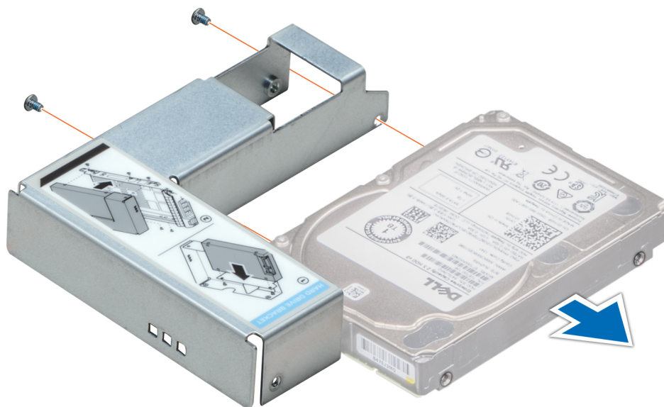
図 36. 3.5 インチ ドライブ アダプターからの 2.5 インチ ドライブの取り外し
