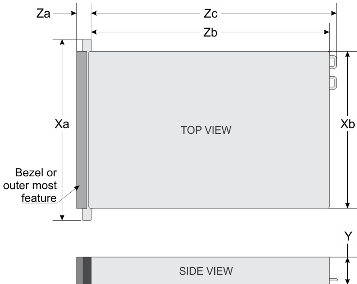
図 9. システムの寸法
