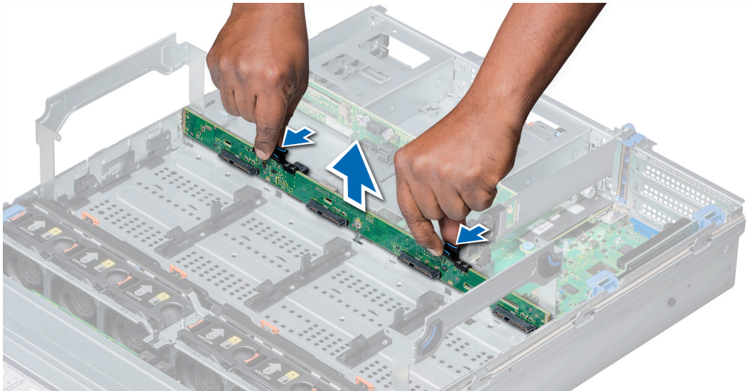
図 82. 中間ドライブ バックプレーンの取り外し
