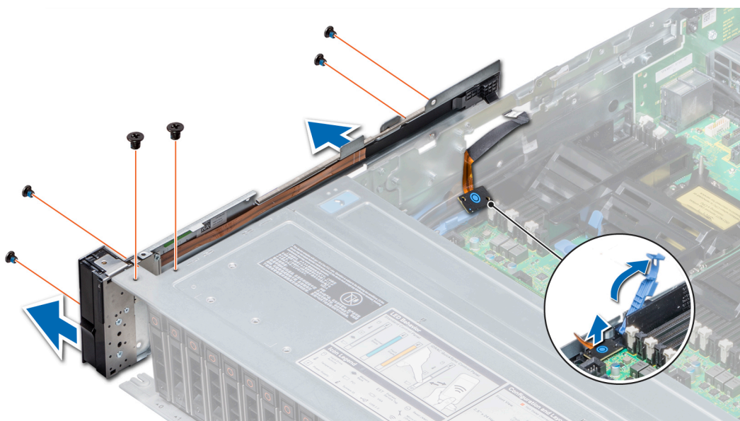
図 99. 左のコントロールパネルの取り外し
