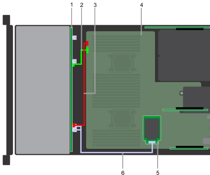
図 86. ケーブル配線 - Mini-PERC 搭載の 12 x 3.5 インチ バックプレーン
