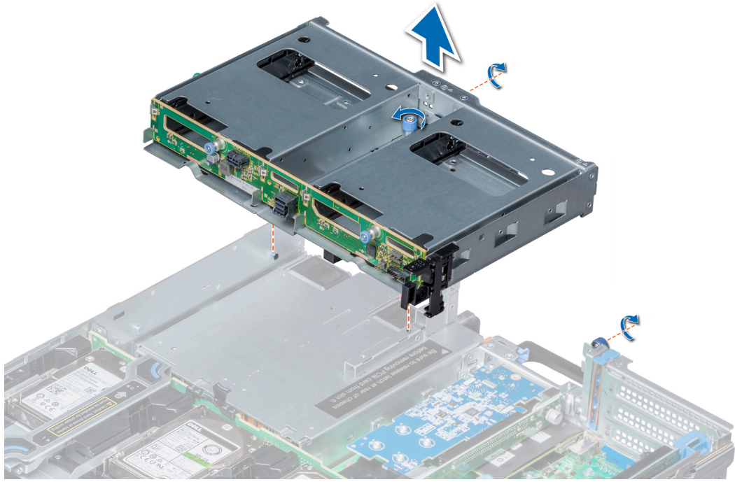
図 42. 2 x 3.5 インチ ドライブ背面ケージの取り外し
