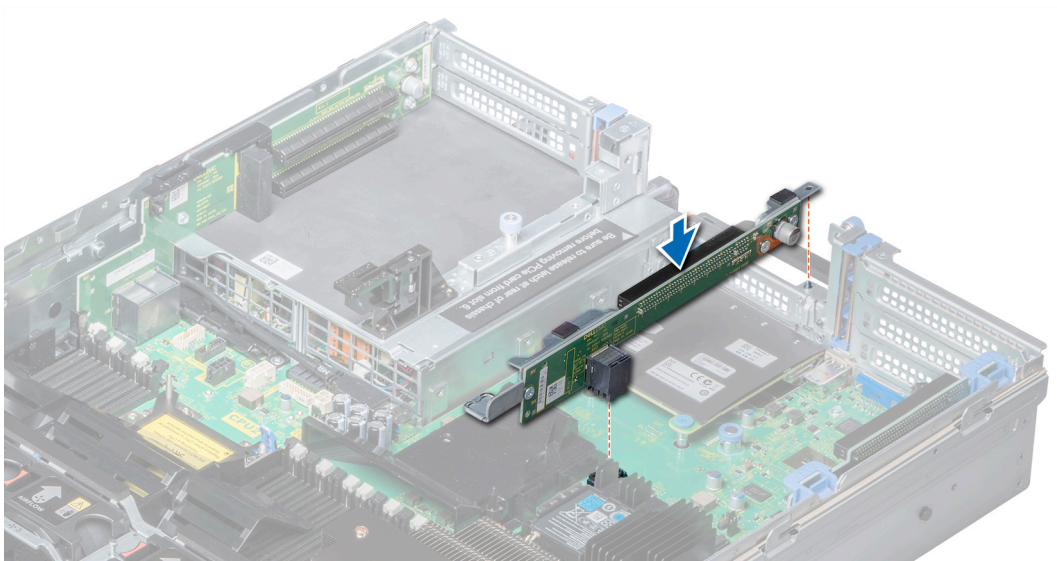
図 69. 拡張カードライザー 2 の取り付け
