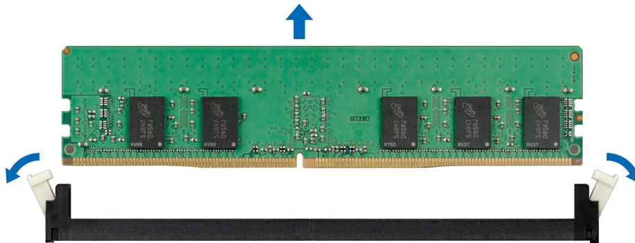
図 45. メモリモジュールの取り外し
