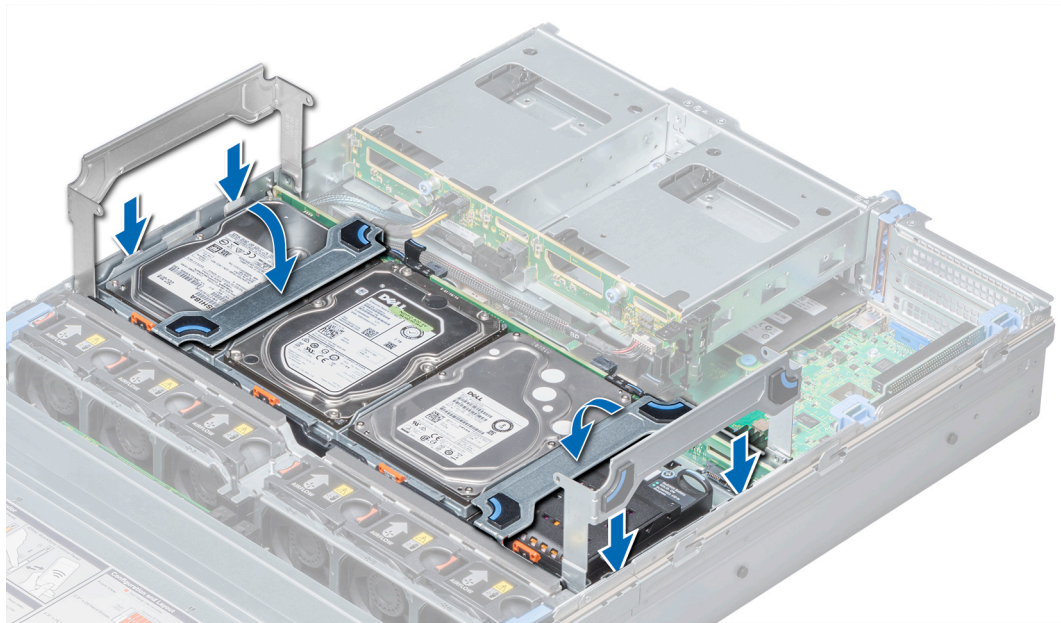
図 25. 中間ドライブトレイの取り付け
