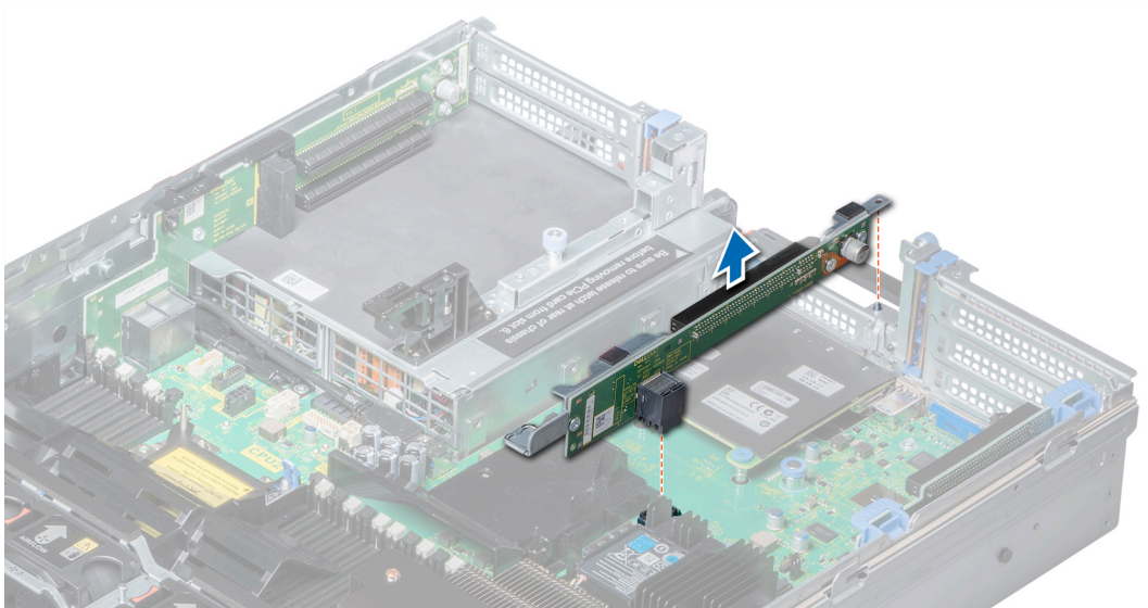
図 68. 拡張カードライザー 2 の取り外し
