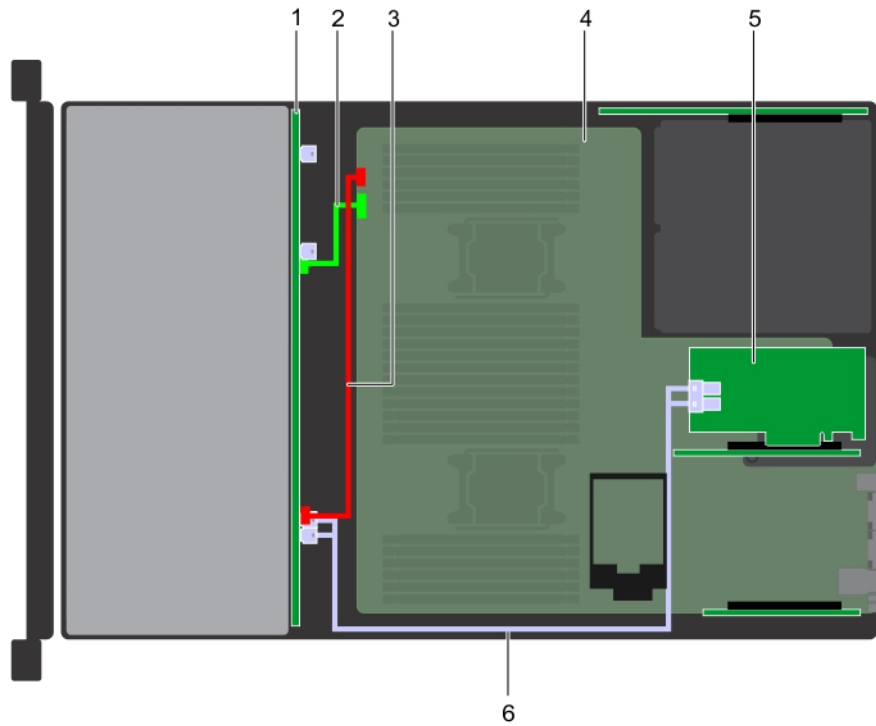
図 87. アダプタ PERC 搭載の 12×3.5 インチ バックプレーン
