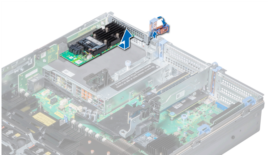
図 59. 拡張カード ライザー 3 からの拡張カードの取り外し
