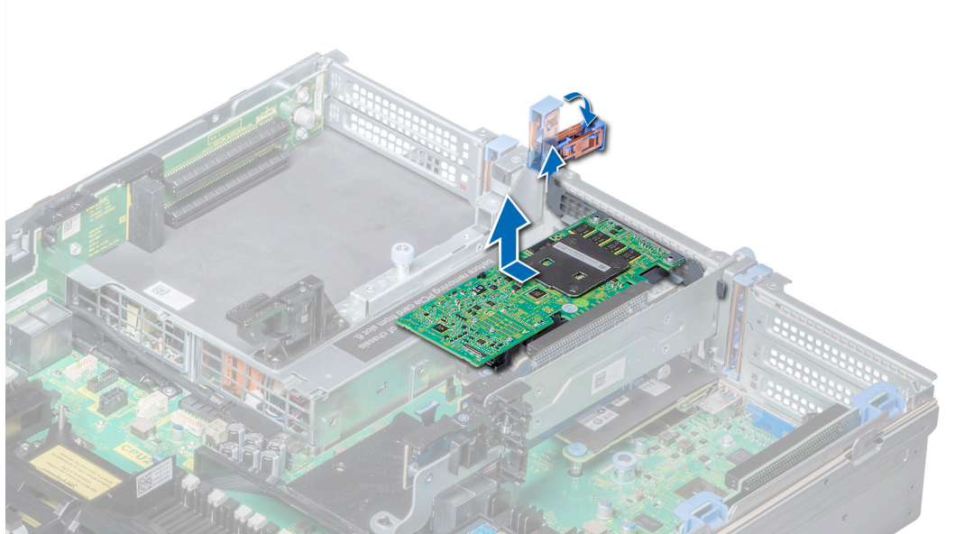
図 58. 拡張カード ライザー 2 からの拡張カードの取り外し
