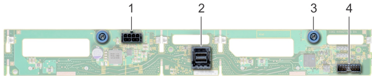
図 79. 3.5 インチ バックプレーンの背面図 (背面ドライブ ケージ)
