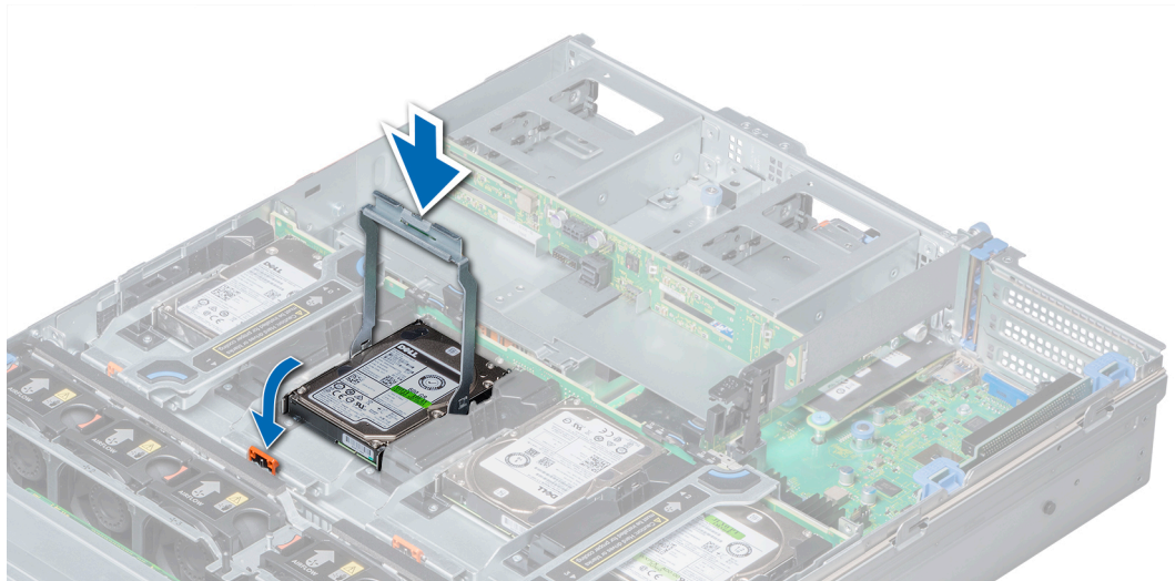
図 29. 中間ドライブトレイへのドライブキャリアの取り付け
