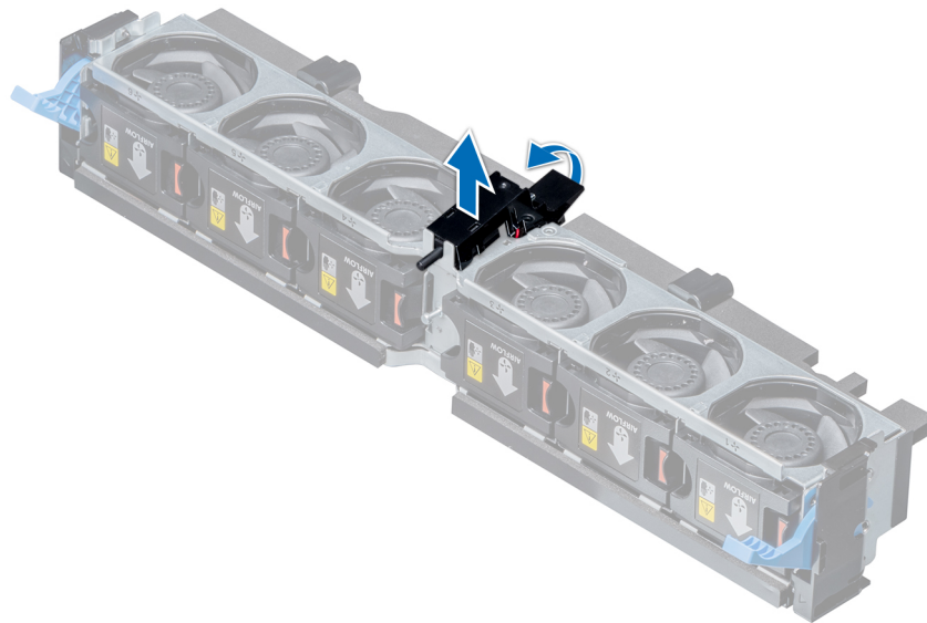
図 22. イントルージョンスイッチの取り外し
