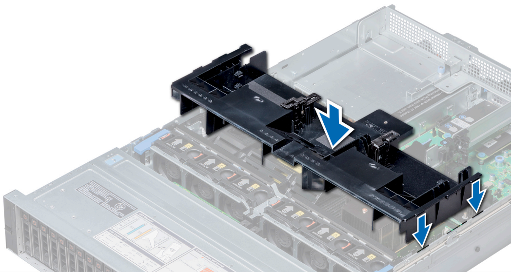
図 17. エアフロー カバーの取り付け
