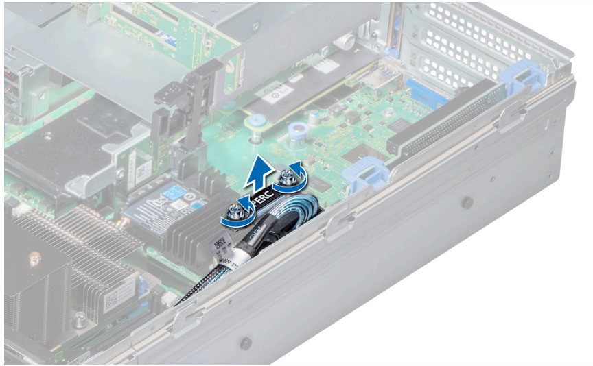
図 72. 内蔵ストレージ コントローラ ケーブルの取り外し
