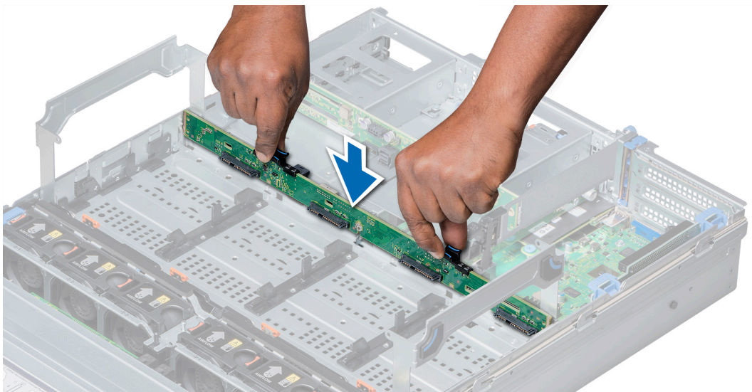
図 83. 中間ドライブ バックプレーンの取り付け
