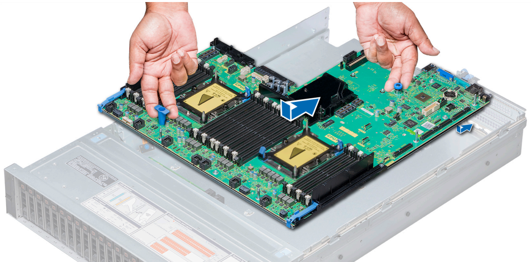
図 97. システム ボードの取り付け
