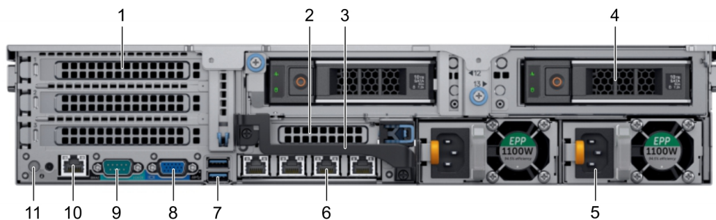
図 5. 2 x 3.5 インチ ドライブ システムの背面図
