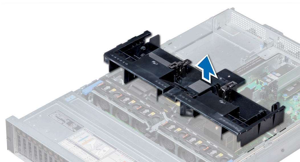
図 16. エアフローカバーの取り外し
