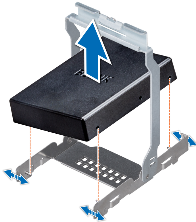
図 26. 中間ドライブ キャリアからのドライブ ダミーの取り外し
