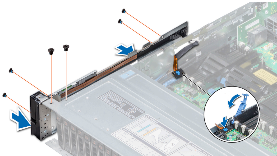
図 100. 左コントロールパネルの取り付け
