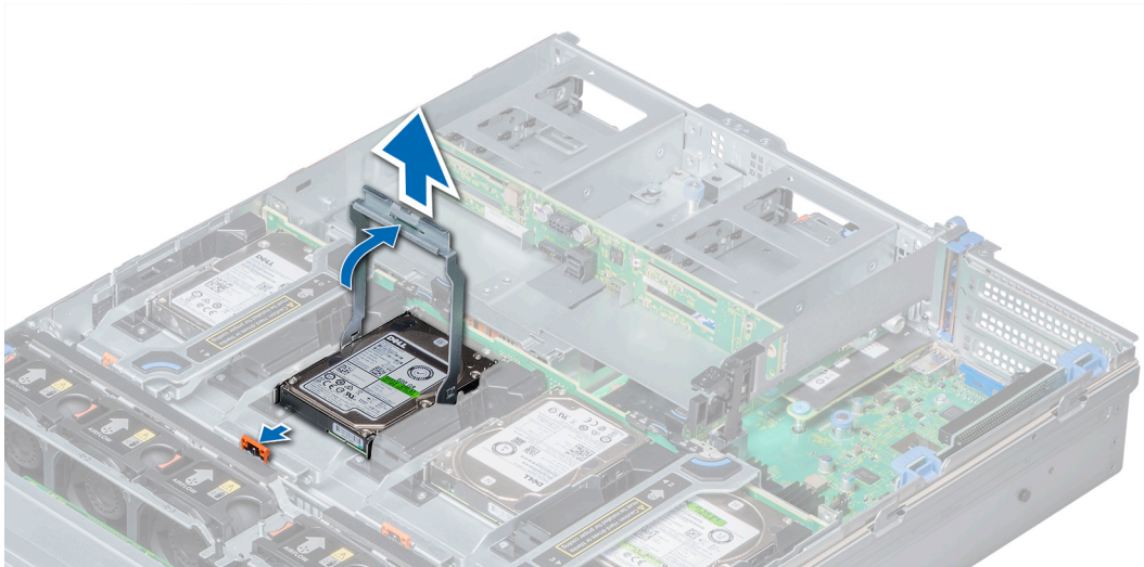
図 28. 中間ドライブ トレイからのドライブ キャリアの取り外し
