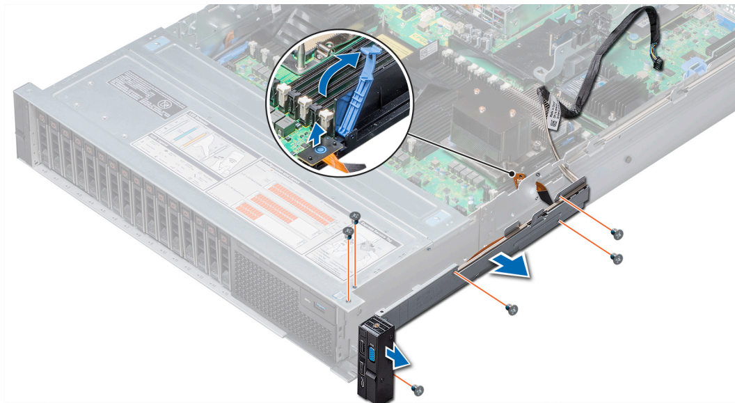
図 101. 右コントロールパネルの取り外し
