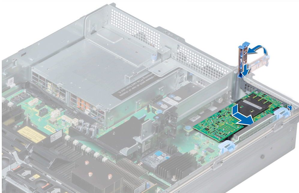
図 60. 拡張カード ライザー 1 への拡張カードの取り付け
