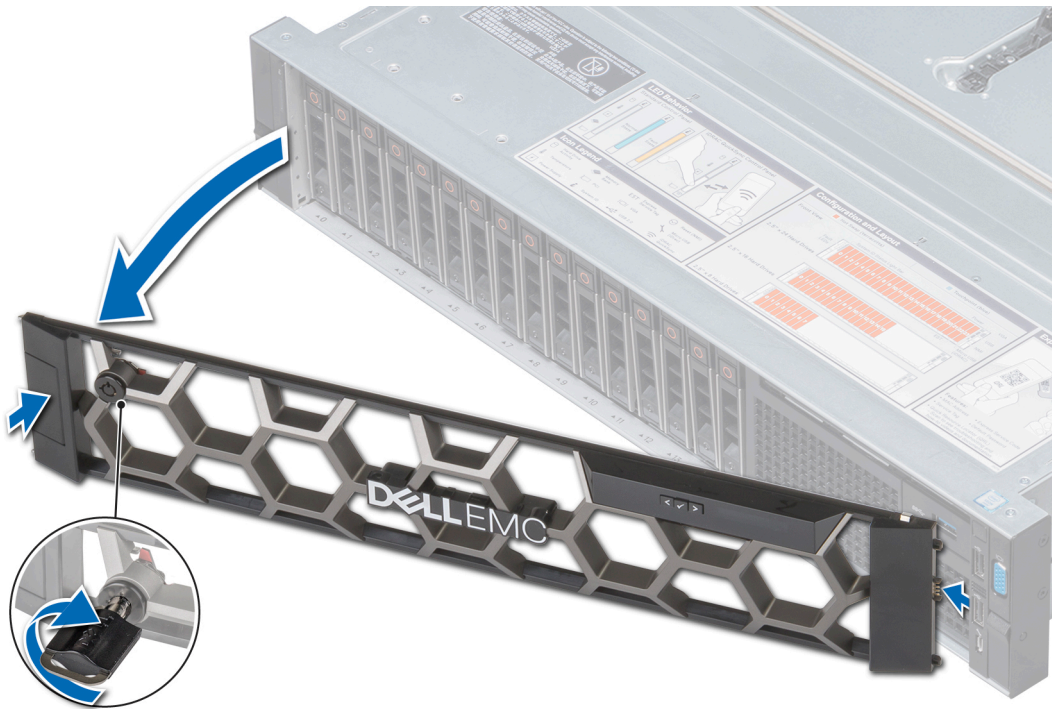
図 10. LCD パネルを搭載した前面ベゼルの取り外し
