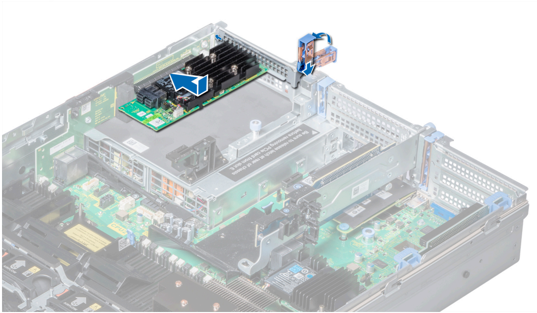
図 63. 拡張カード ライザー 3 への拡張カードの取り付け
