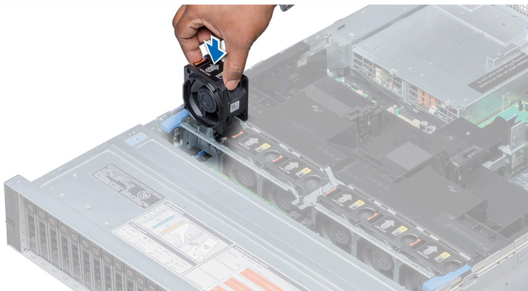
図 21. 冷却ファンの取り付け
