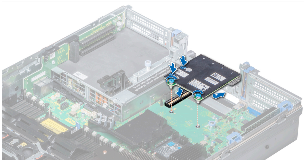
図 71. ネットワークドーターカードの取り付け
