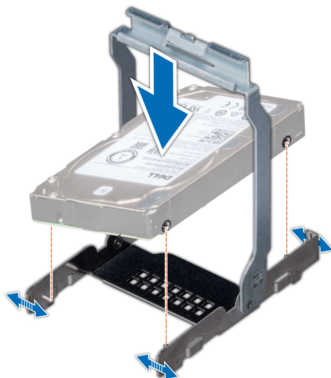
図 31. ドライブ キャリアへの 3.5 インチ ドライブの取り付け
