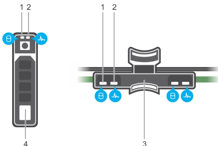
図 103. ドライブのドライブ インジケータおよび中間ドライブ トレイ バックプレーン
