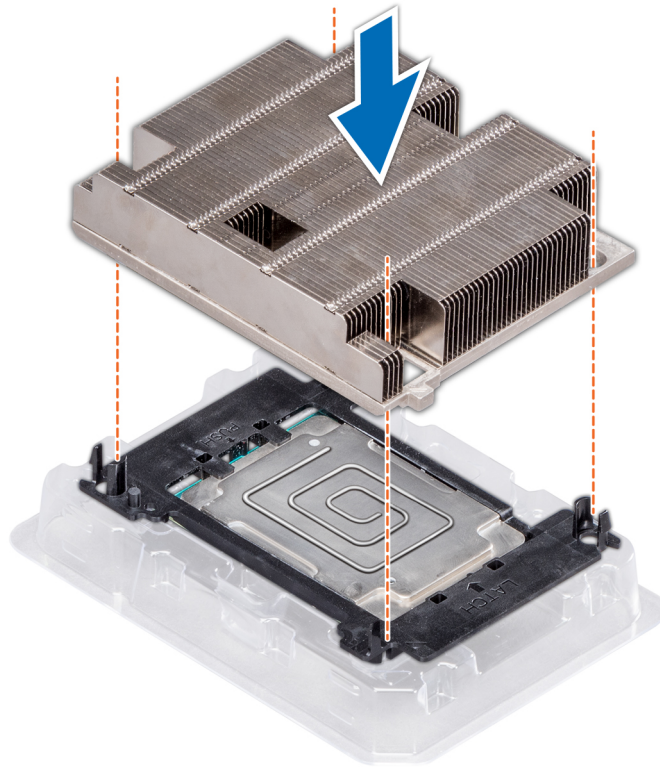
図 52. ヒートシンクをプロセッサに取り付けます。
