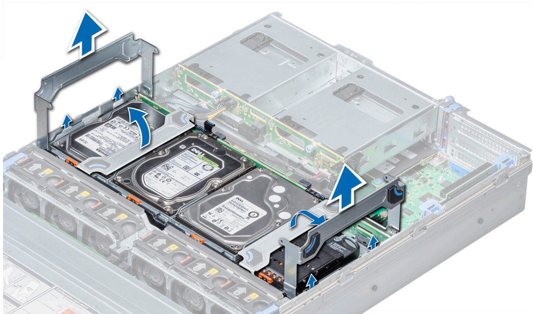
図 24. 中間ドライブトレイの取り外し
