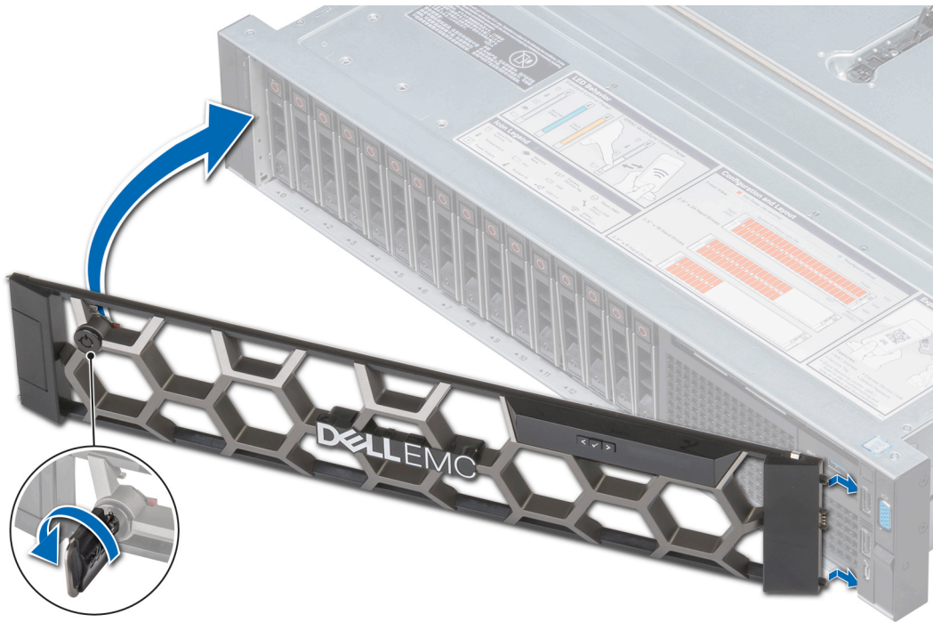
図 11. LCD パネルを搭載した前面ベゼルの取り付け
