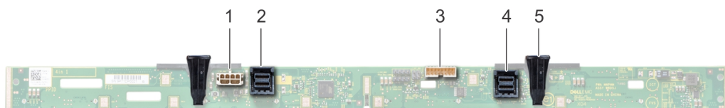
図 77. 3.5 インチ バックプレーンの背面図 (中間ドライブトレイ)
