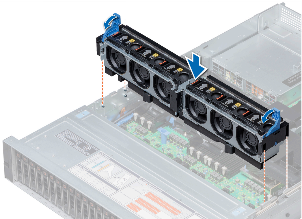
図 19. 冷却ファンアセンブリの取り付け
