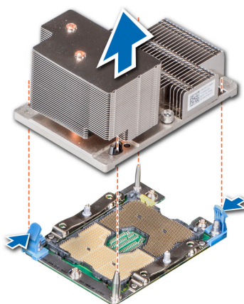
図 47. プロセッサとヒートシンクモジュールの取り外し
