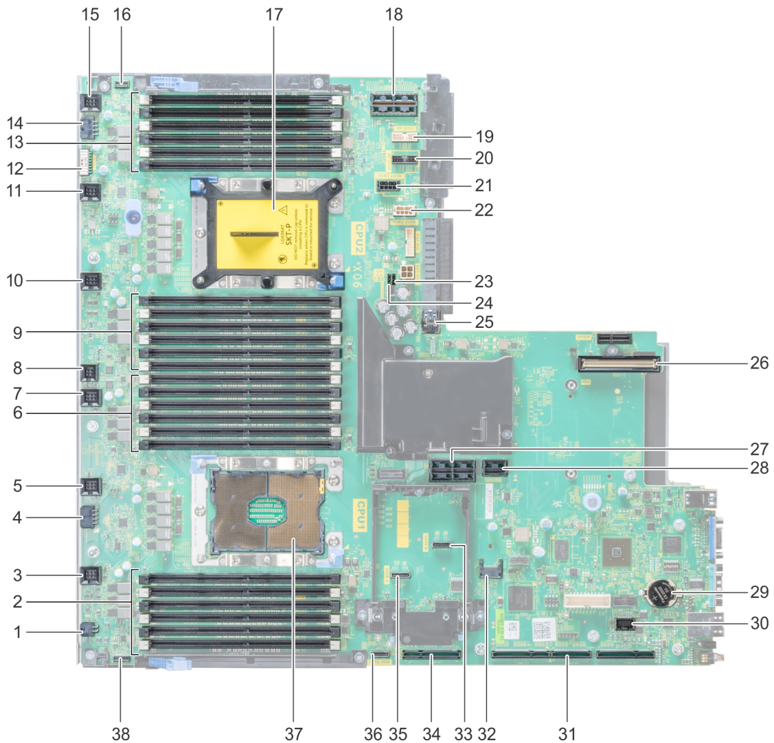
図 108. システム基板のジャンパとコネクタ
