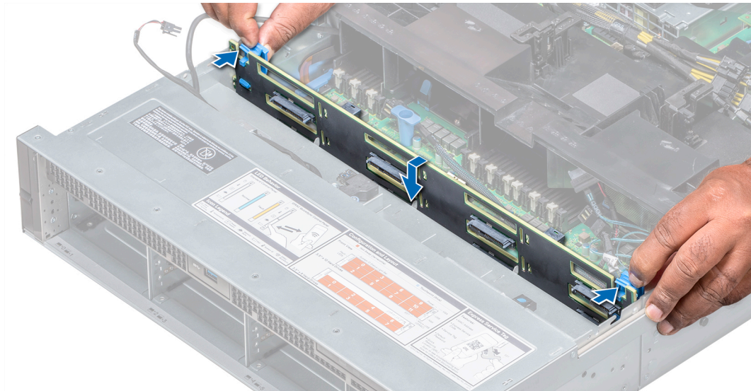
図 81. バックプレーンの取り付け
