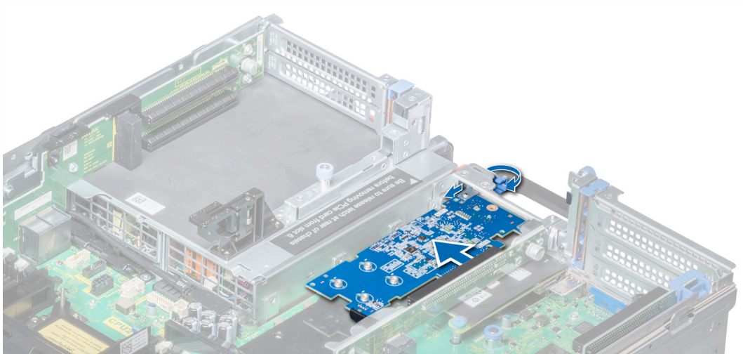
図 57. 拡張カード ライザー 2B からの拡張カードの取り外し
