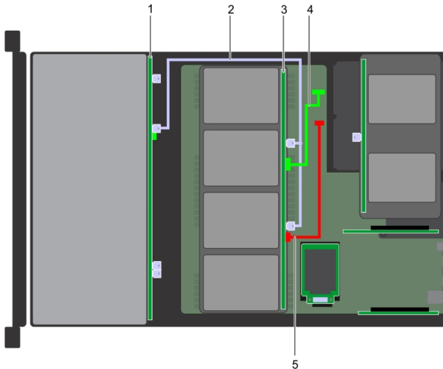
図 89. ケーブル配線 - 12 x 3.5 インチ バックプレーン搭載の 4 x 3.5 中間バックプレーン
