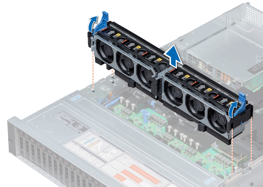
図 18. 冷却ファンアセンブリの取り外し
