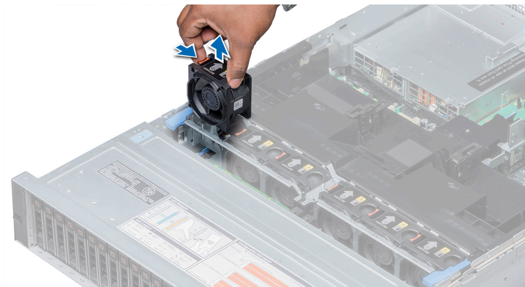
図 20. 冷却ファンの取り外し
