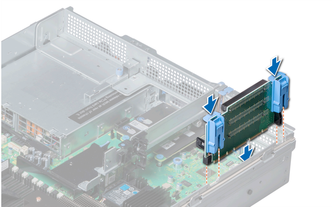
図 67. 拡張カードライザー 1 の取り付け
