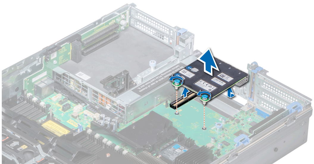
図 70. ネットワークドーターカードの取り外し
