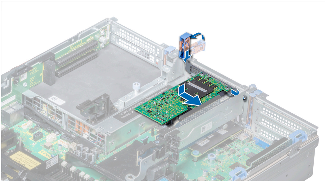
図 62. 拡張カード ライザー 2 への拡張カードの取り付け
