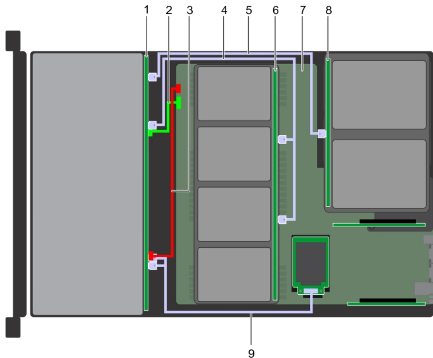
図 88. ケーブル配線 - 4×3.5 中間ドライブトレイおよび 2×3.5 背面ドライブケージ搭載の 12×3.5 インチ バックプレーン
