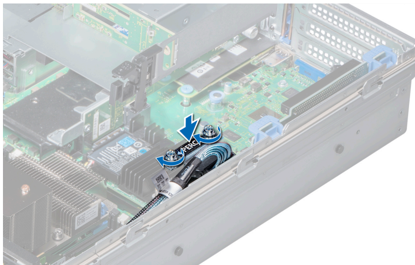
図 75. 内蔵ストレージコントローラカードケーブルの取り付け
