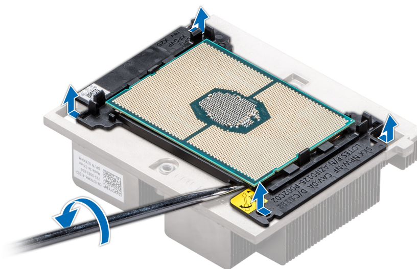
図 48. プロセッサブラケットを緩める
