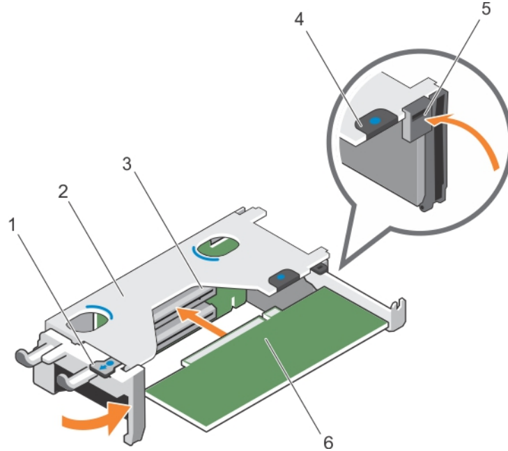
그림 25. 확장 카드 라이저 1에 확장 카드 설치
