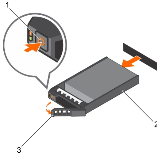
그림 15. 핫 스왑 가능한 하드 드라이브 또는 SSD 분리
