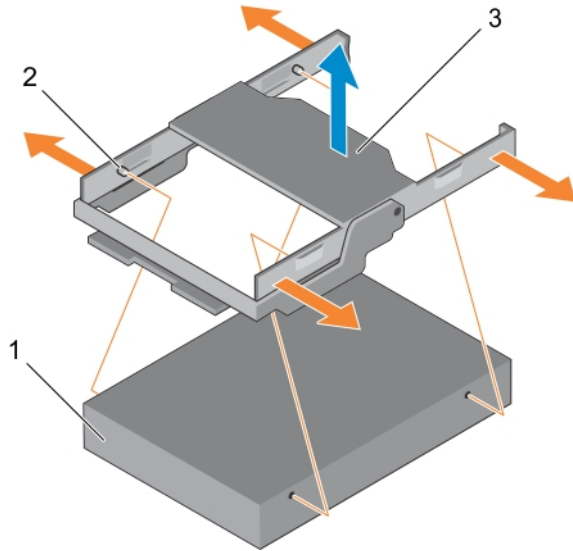
그림 18 . 하드 드라이브 설치 및 하드 드라이브 캐리어에서 분리
