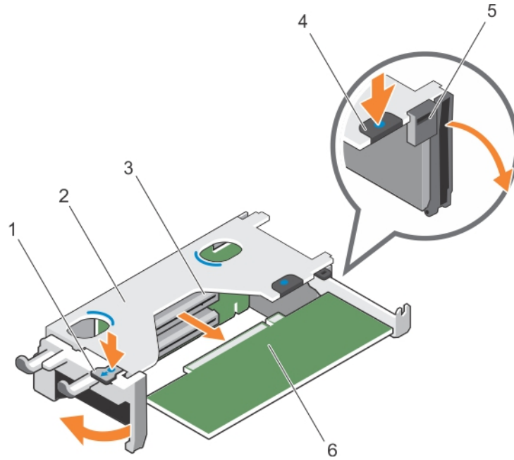
그림 24. 확장 카드 라이저 1에서 확장 카드 분리
