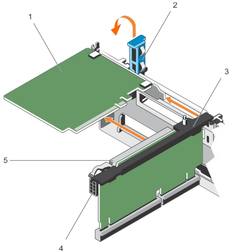
그림 22. 확장 카드 라이저 2 또는 3에서 확장 카드 분리
