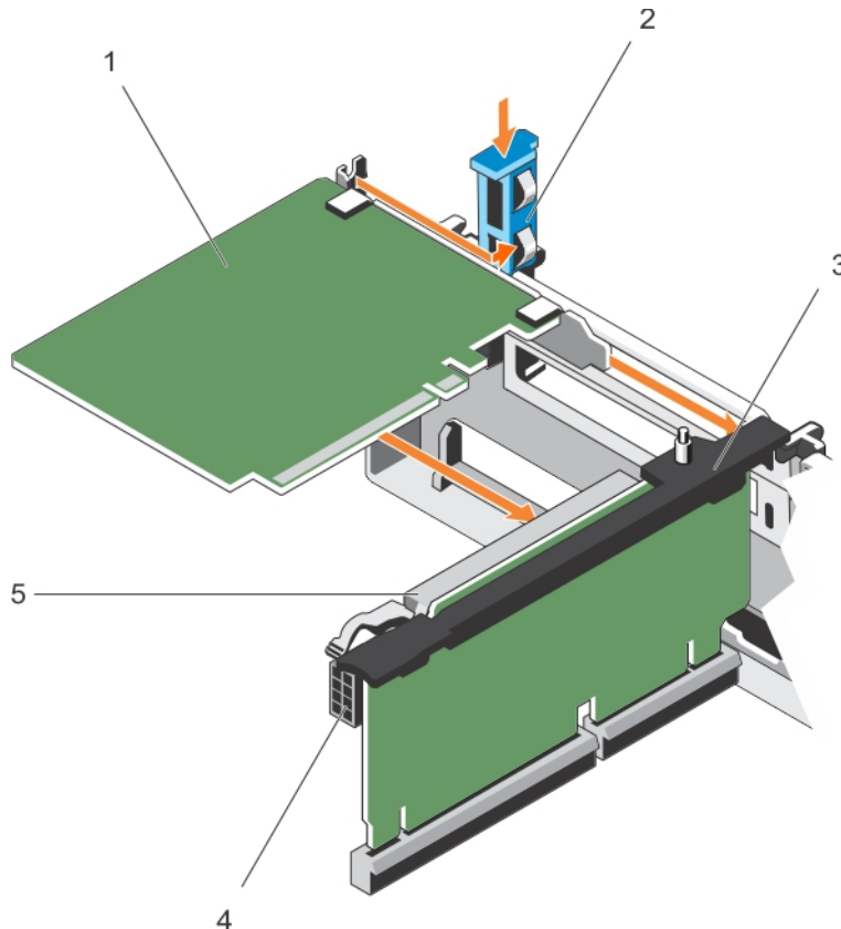
그림 23. 확장 카드 라이저 2 또는 3에 확장 카드 설치
