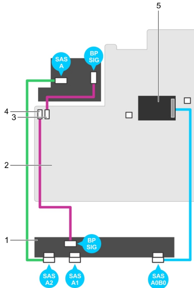
그림 54. 케이블 연결 다이어그램 - 3.5인치(x12) SAS/SATA 후면판 - NX3230 (선택사양 1)
