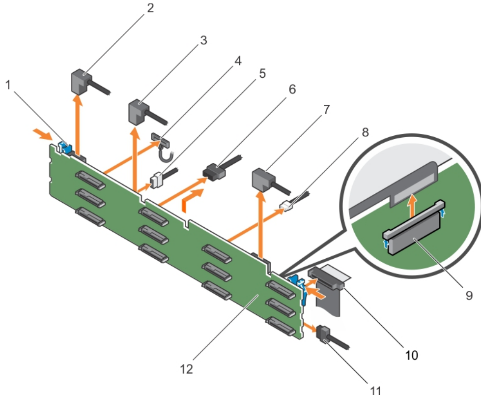
그림 53. 3.5인치(x12) SAS/SATA 후면판 분리 및 설치 - NX3230
