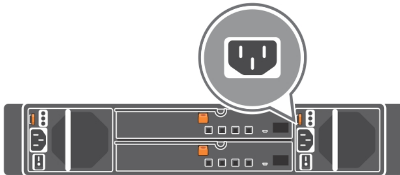
Ilustración 2. Conexión de los cables de alimentación
