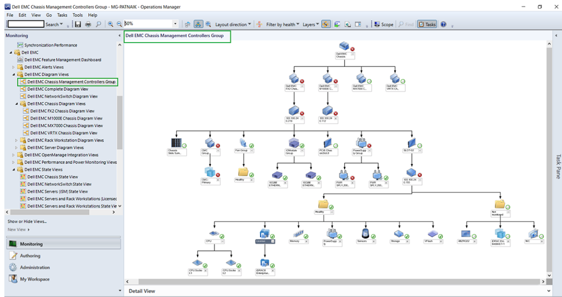
圖 7. Dell EMC 機箱管理控制器群組圖表檢視
