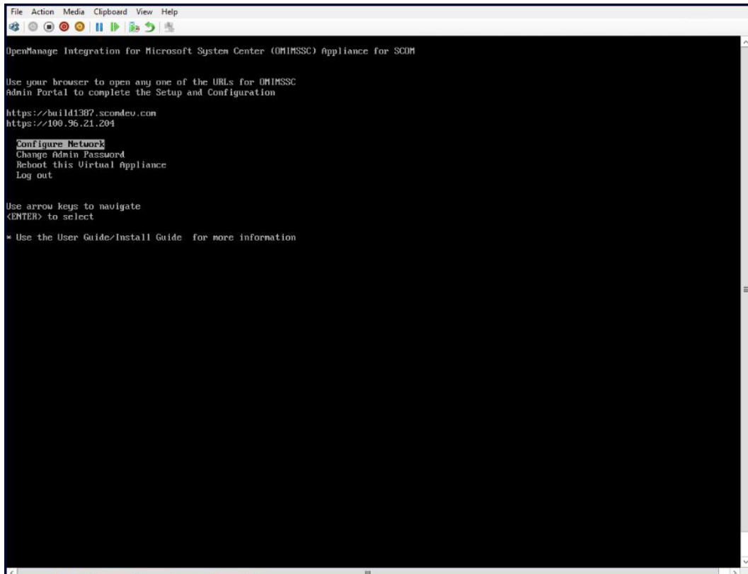
圖 3. OMIMSSC 命令行介面
