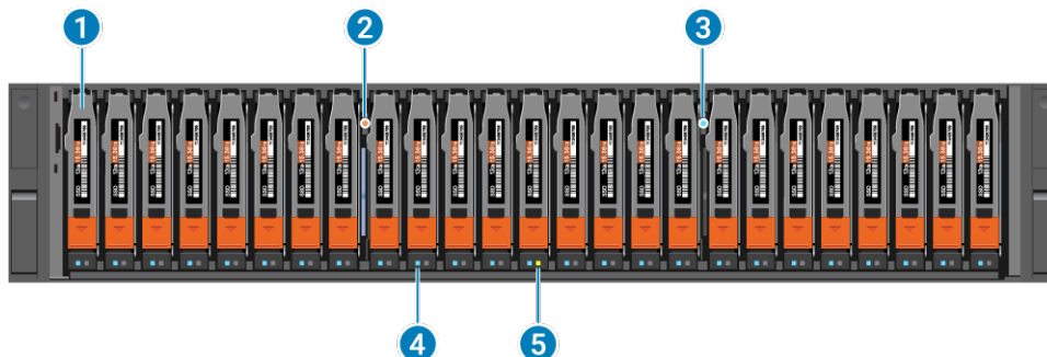
Figure 13. Vue avant du boîtier d'extension SAS
