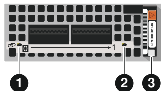
Figure 10. Voyants du module d'E/S à 2 ports sur le boîtier de base
