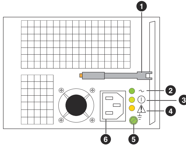
Figure 16. Module d'alimentation CA et de refroidissement du boîtier d'extension SAS
