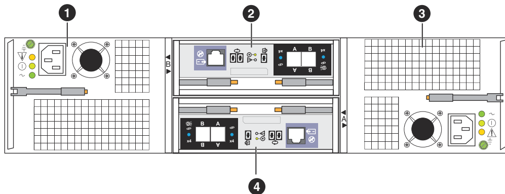
Figure 14. Emplacements des composants arrière du boîtier d'extension SAS
