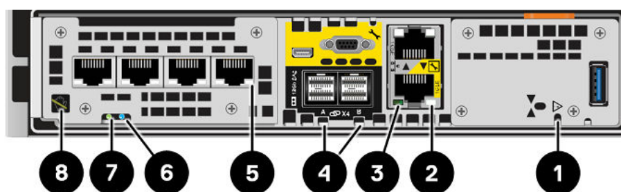
Figure 7. Voyants du module intégré
