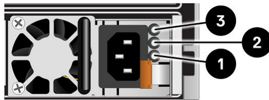
Figure 12. Voyants LED du bloc d'alimentation secteur du Boîtier de base
