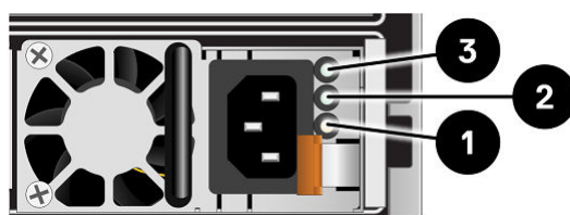
Figure 22. Voyants du bloc d'alimentation CA du boîtier d'extension NVMe
