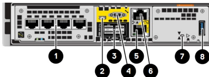
Figure 6. Vue arrière du module intégré v1 indiquant les emplacements des composants
