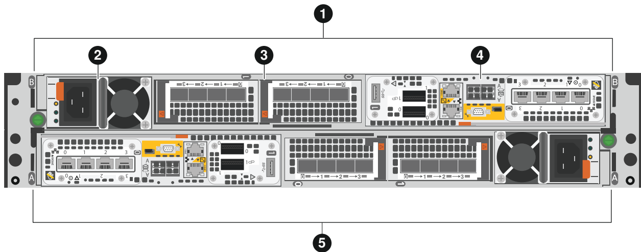
Figure 5. Vue arrière du boîtier de base indiquant les emplacements des composants matériels
