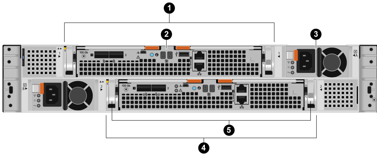
Figure 19. Emplacements des composants arrière du boîtier d'extension NVMe
