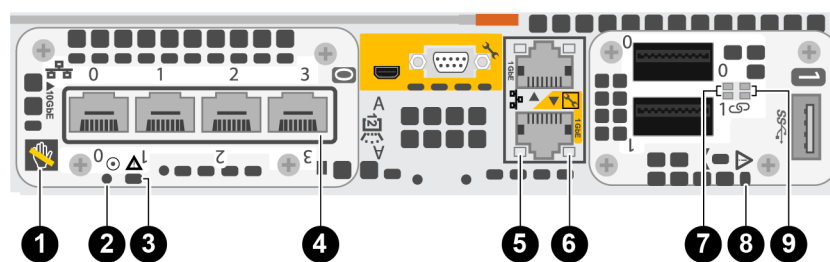
Figure 9. Voyants du module intégré
