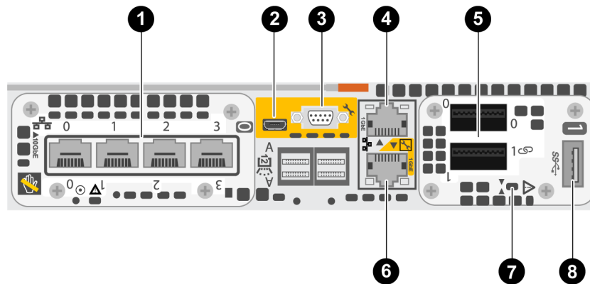
Figure 8. Vue arrière avec emplacements des composants
