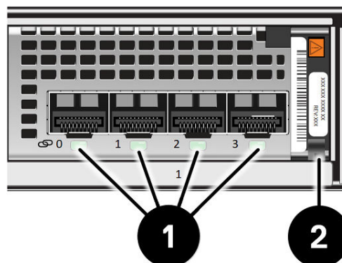
Figure 11. Voyants du module d'E/S à 4 ports sur le boîtier de base
