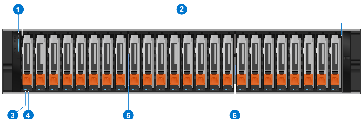
Figure 17. Vue avant du boîtier d'extension NVMe
