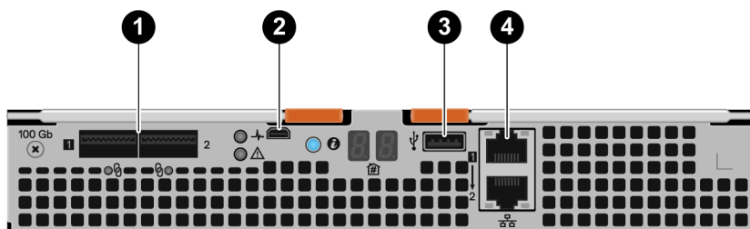
Figure 20. Vue arrière du module d'accès indiquant les emplacements des composants
