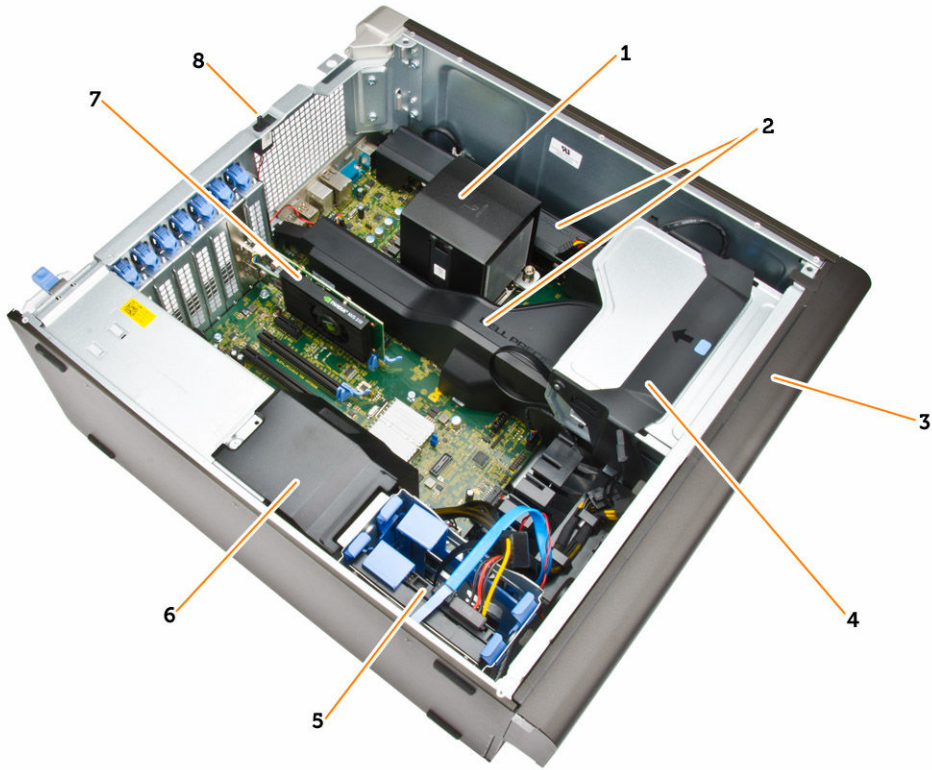
图 2: T5810 计算机内部视图
