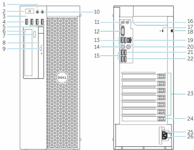
图 1: T5810 计算机的正面和背面视图
