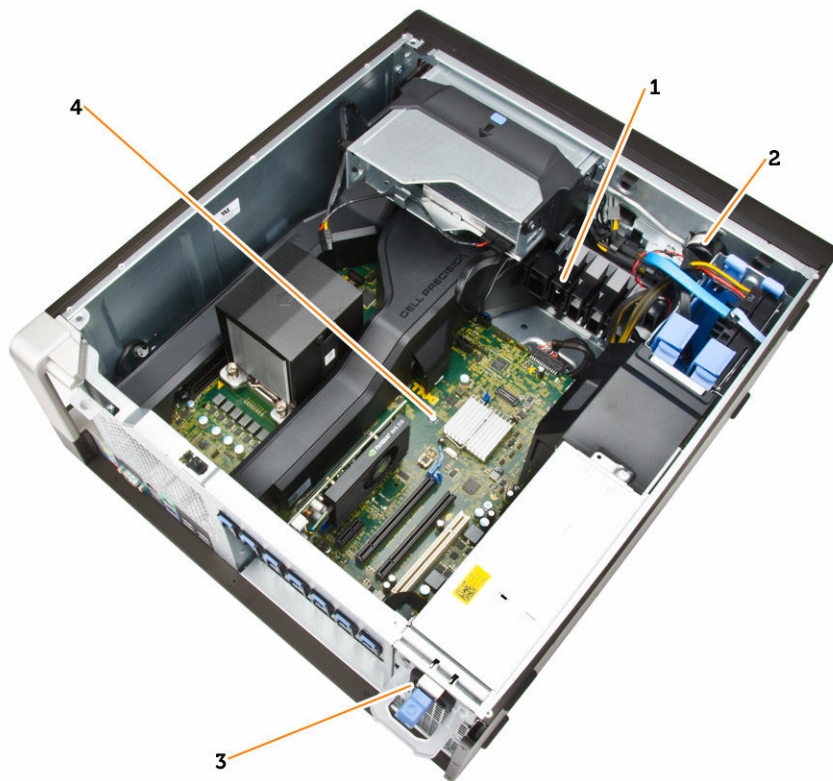
图 3: T5810 计算机内部视图
