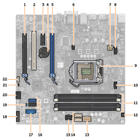
Ilustración 1. Componentes de la placa base
