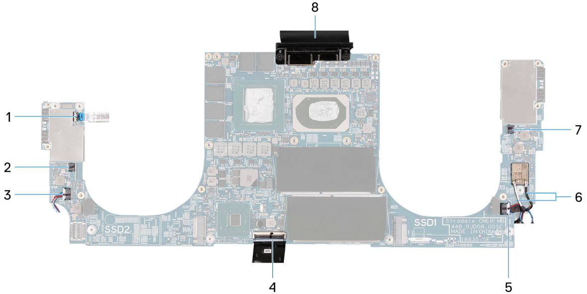
그림 2. 시스템 보드 커넥터
