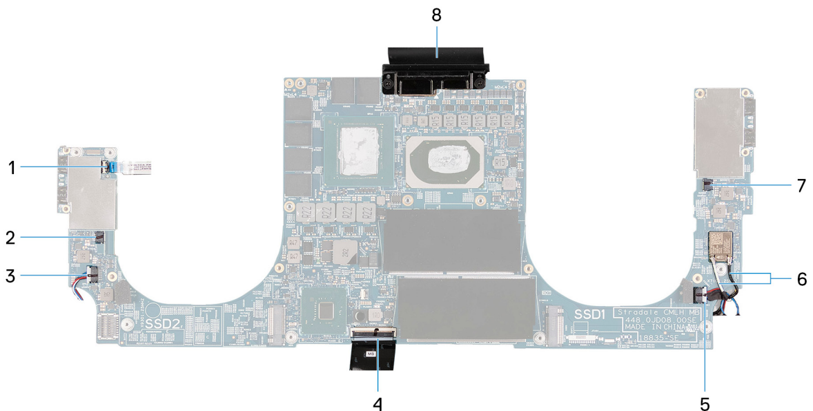
그림 1. 시스템 보드 커넥터
