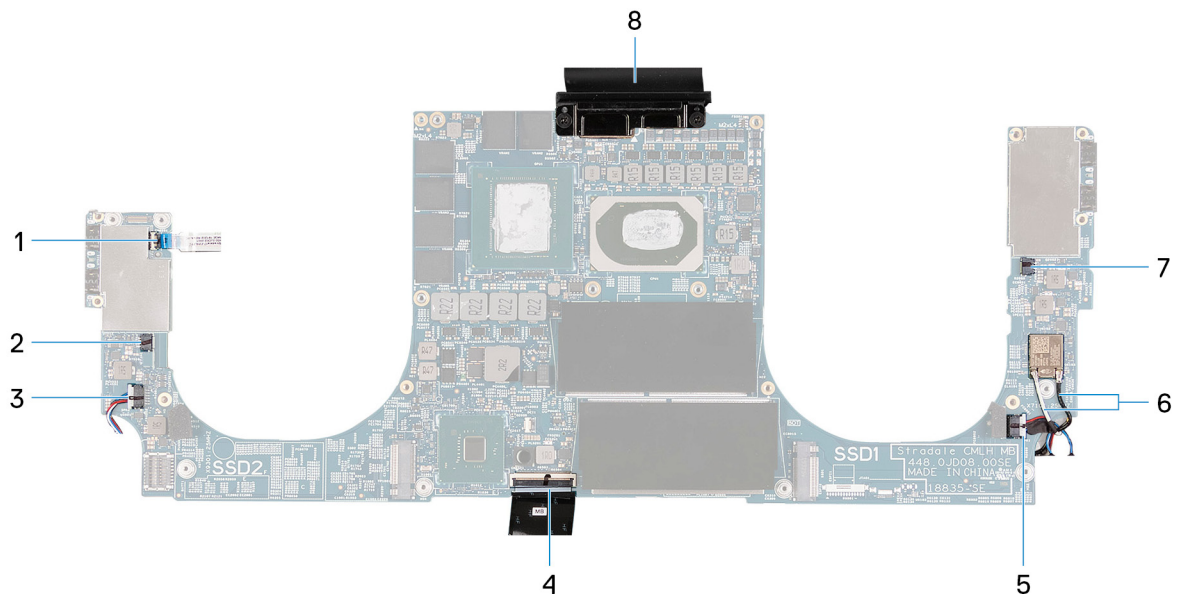
Ilustración 1. Conectores de la tarjeta madre
