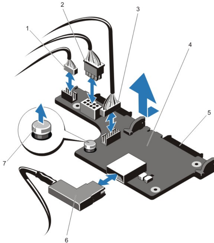
그림 46. 선택 사양 2.5 인치 (x2) 하드 드라이브 후면판 분리 및 설치(후면)
