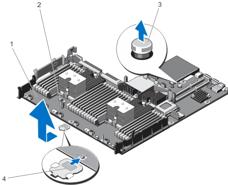
그림 50. 시스템 보드 분리 및 설치
