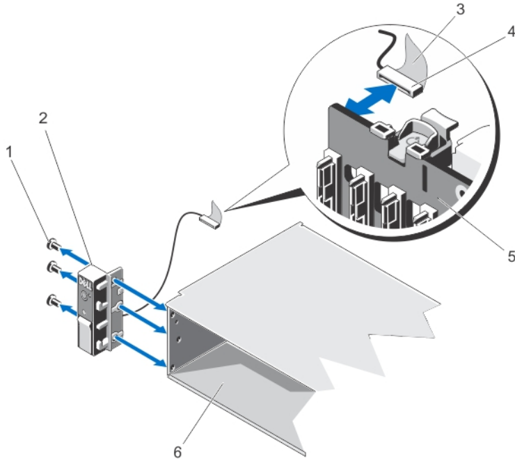
그림 48. 제어판 분리 및 설치
