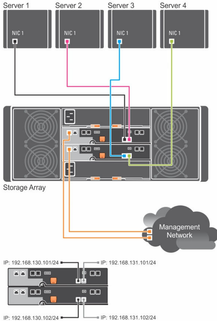
그림 1. 이중-RAID 컨트롤러 구성의 호스트 4개
