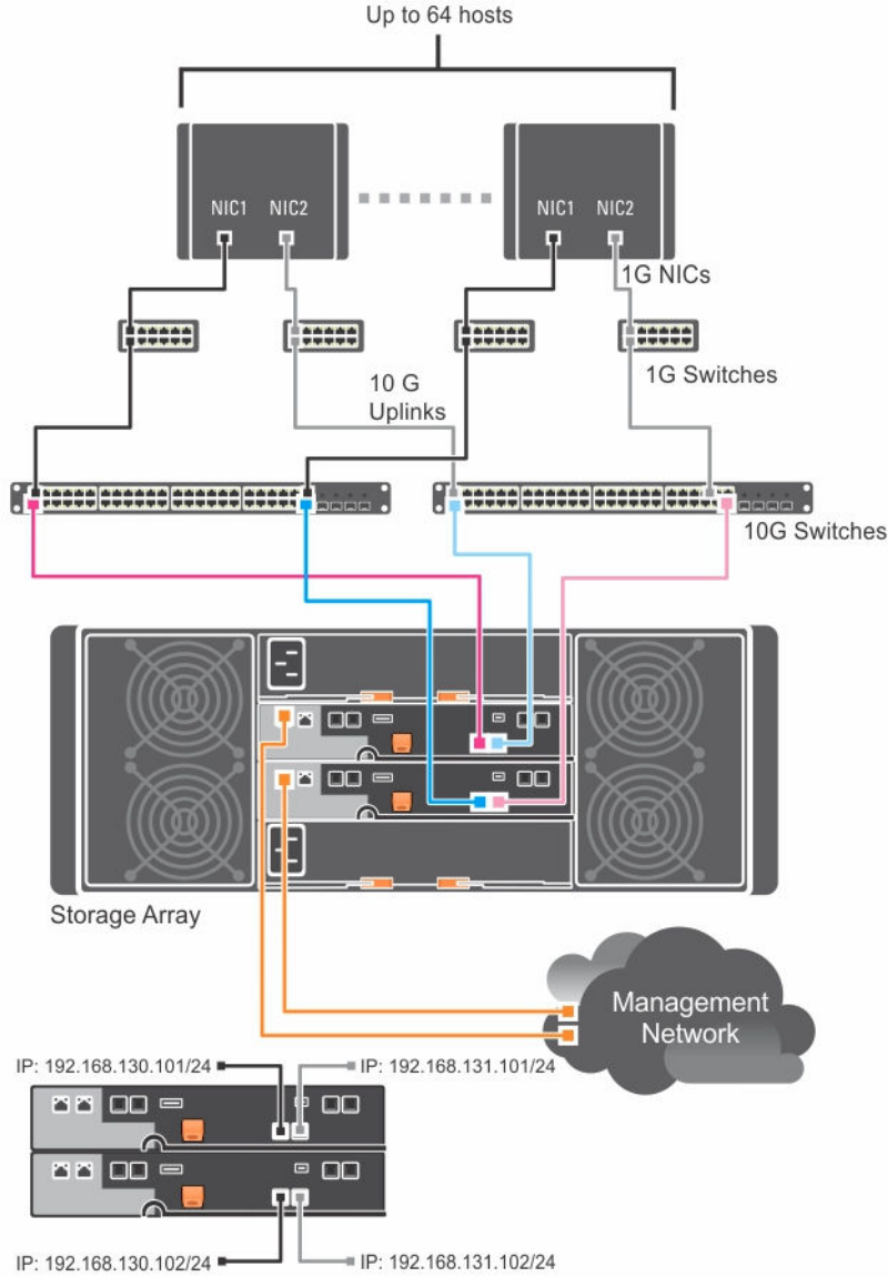
그림 4. 2개의 RAID 컨트롤러에 연결된 64개의 서버
