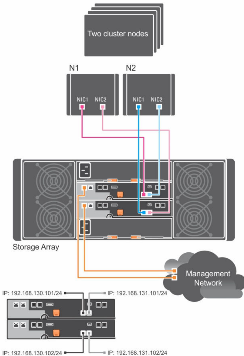
図 3. 2 台の RAID コントローラに接続された 2 台のクラスタノード
