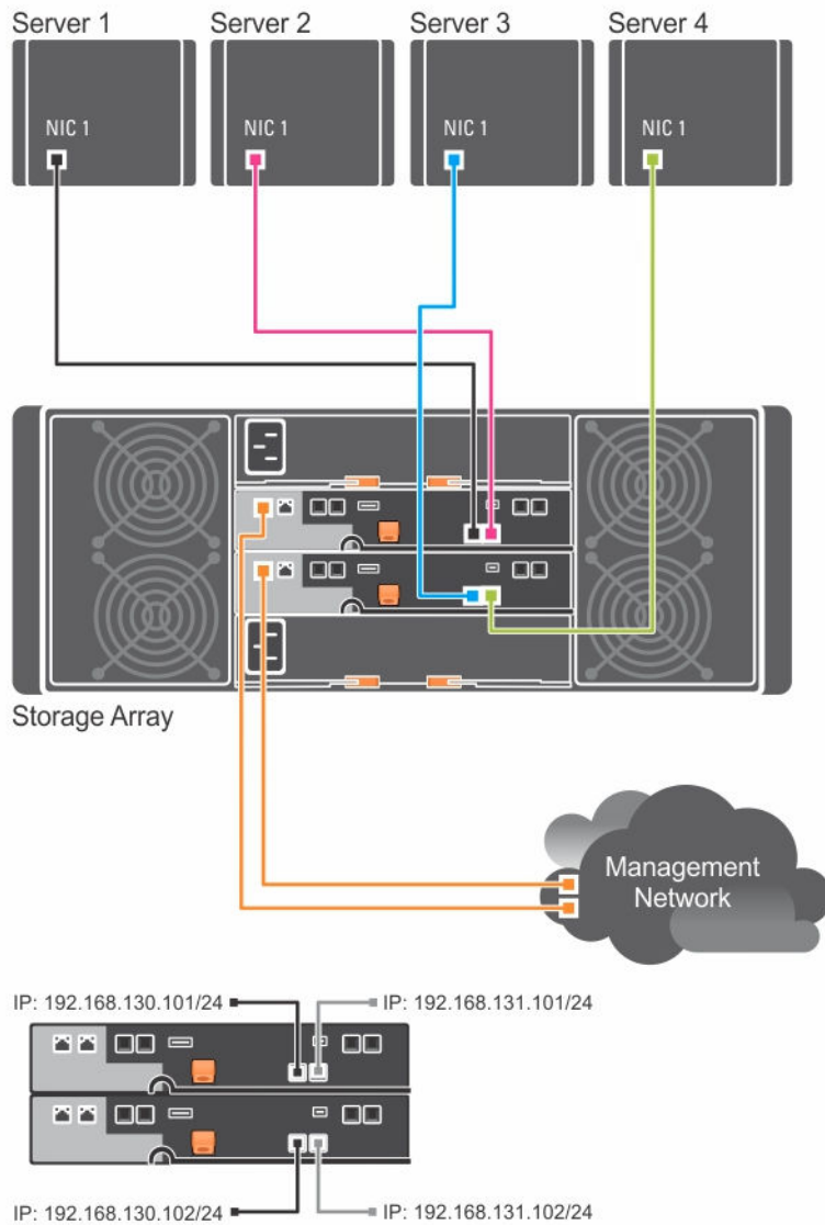
図 1. デュアル RAID コントローラ構成の 4 台のホスト
