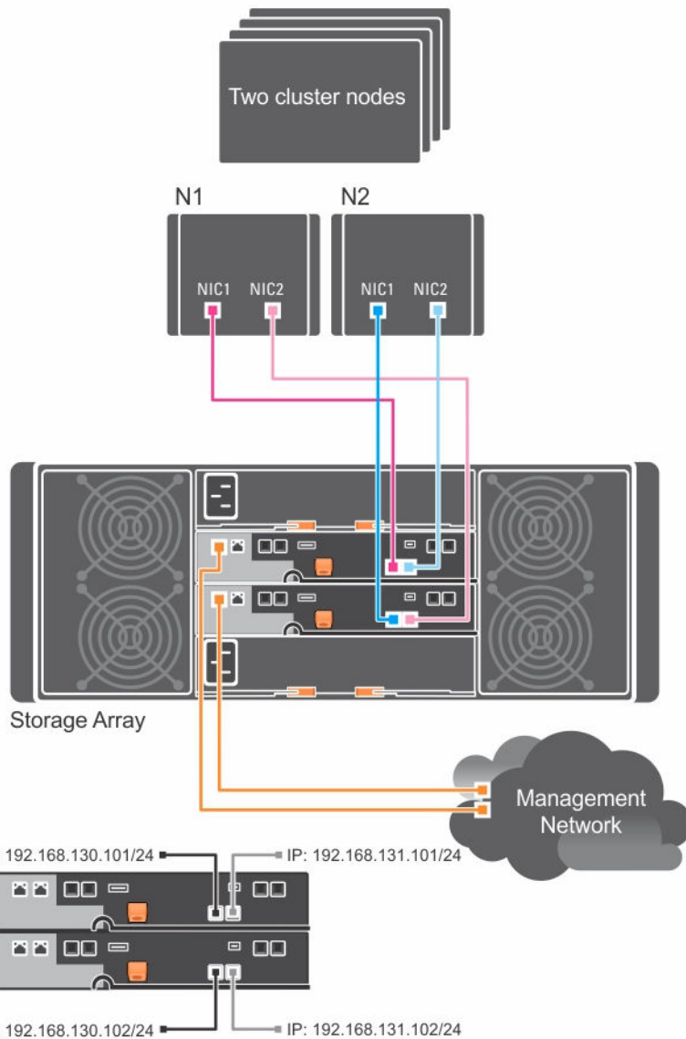
Ilustración 3. Dos nodos de clúster conectados a dos controladoras RAID
