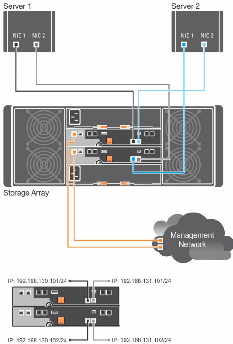
Ilustración 2. Dos hosts conectados a dos controladoras RAID
