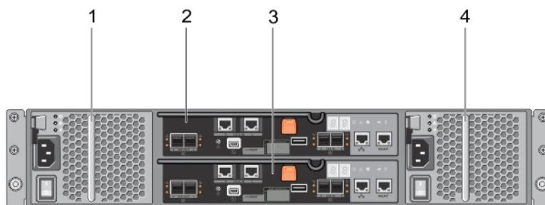
図 4. 背面パネルの機能およびインジケータ - Dell PowerVault MD3800i および MD3820i シリーズ
