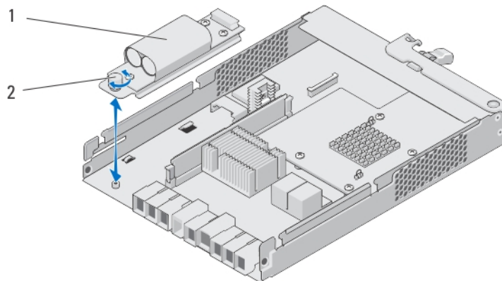
Abbildung 17. Entfernen und Installieren des RAID-Controller-Modul-Akkusicherungsmoduls
