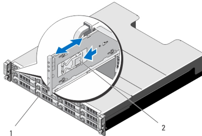
Abbildung 20. Entfernen und Installieren der Bedienfeldplatte – PowerVault MD3800i
