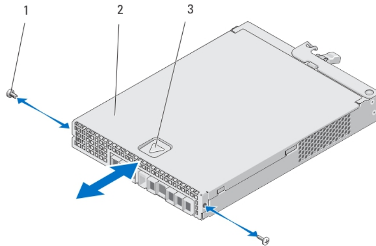
Abbildung 16. Öffnen und Schließen des RAID-Controller-Moduls
