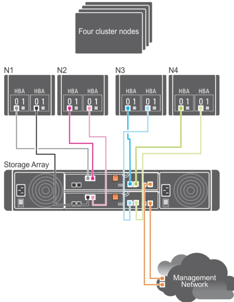
Abbildung 11. Vier Cluster-Knoten, die mit zwei RAID-Controllern verbunden sind
