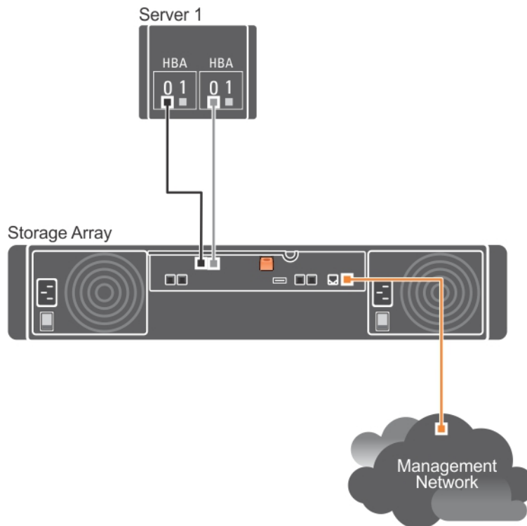
Abbildung 2. Ein Host, der mit einem einzigen RAID-Controller verbunden ist
