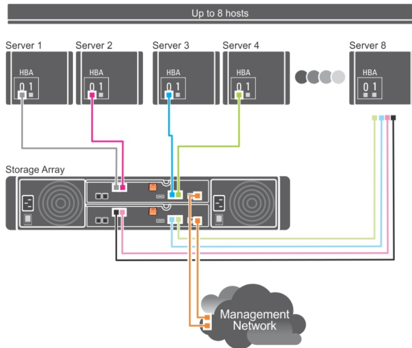
Abbildung 9. Acht Hosts, die mit zwei RAID-Controllern verbunden sind
