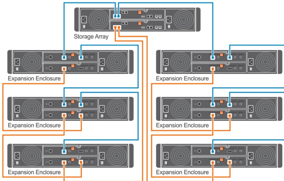
Abbildung 13. Dual-Erweiterung-Verkabelungsdiagramm
