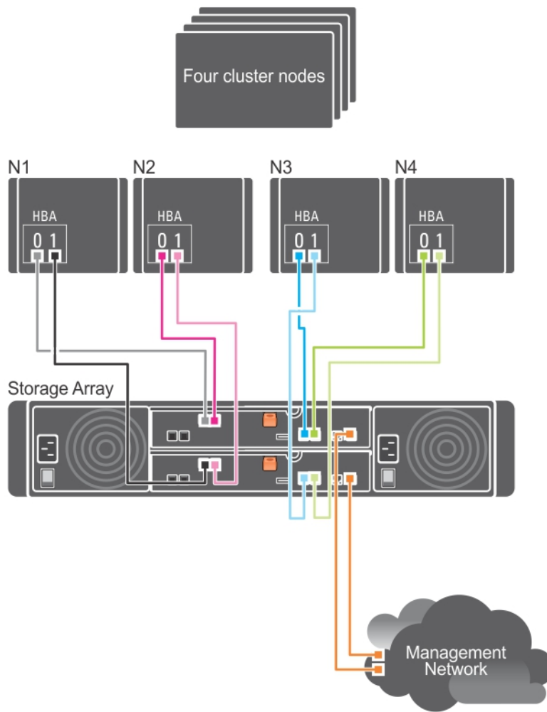
Abbildung 10. Vier Cluster-Knoten, die mit zwei RAID-Controllern verbunden sind
