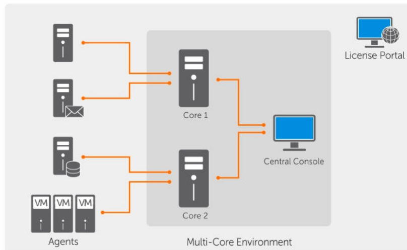
Figure 3. Architecture de déploiement avec plusieurs Cores
