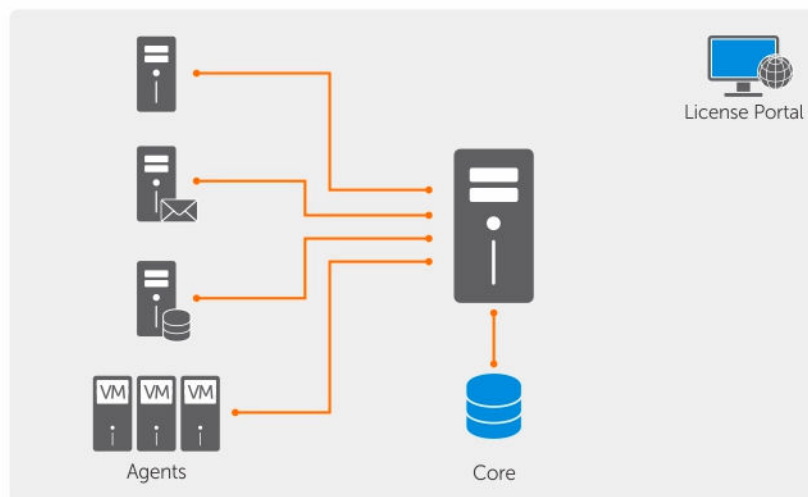
Figure 2. Architecture de déploiement de base
