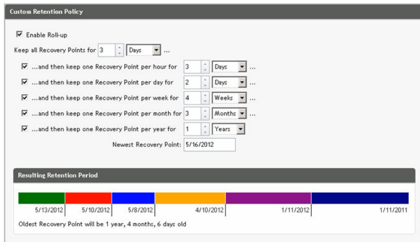
Figure 6. Stratégie de rétention personnalisée
