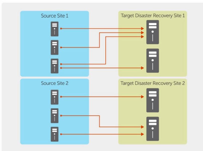
Figure 8. Diagramme de l'architecture de réplication multipoint
