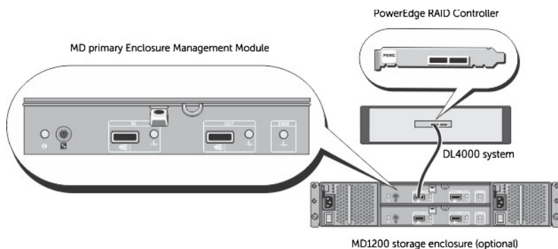
Figura 2. Conectar o cabo SAS do sistema DL4000 ao gabinete de armazenamento PowerVault MD1200
