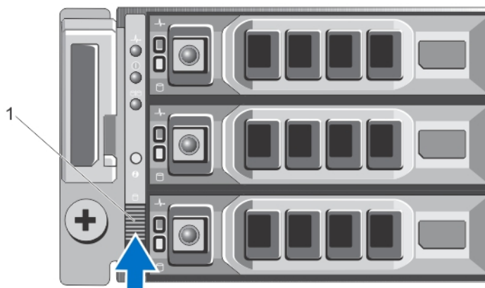
Figura 1. Configurar o comutador de configuração do gabinete de armazenamento PowerVault MD1200
