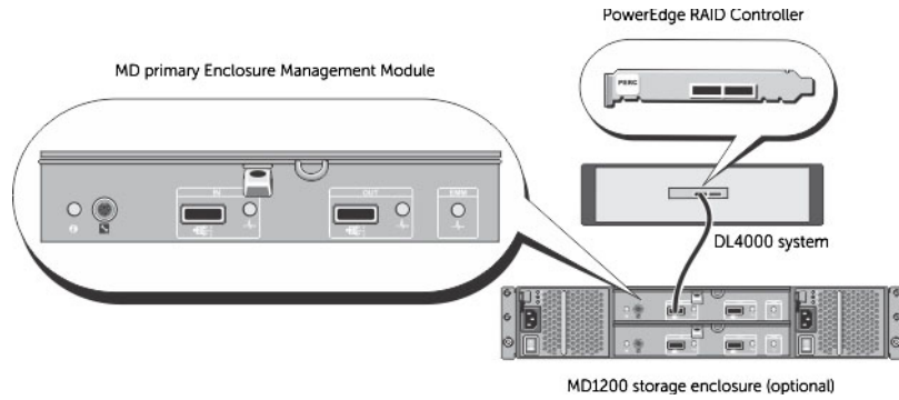
그림 2 . PowerVault MD1200 스토리지 인클로저에 DL4000의 SAS 케이블을 연결
