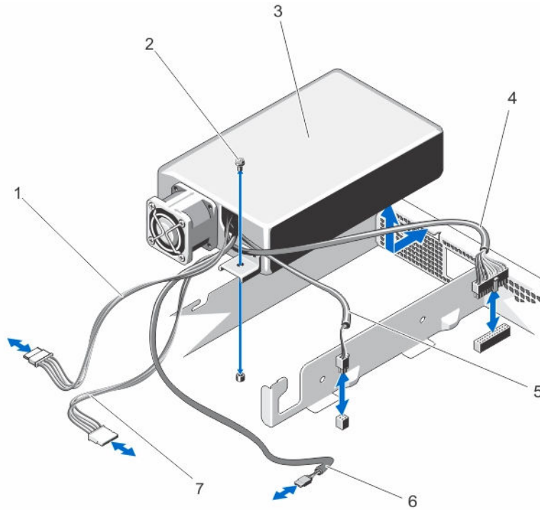
图 22: 卸下和安装电源设备
