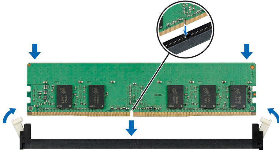
图 54: 在系统板或 PEM 上安装内存模块
