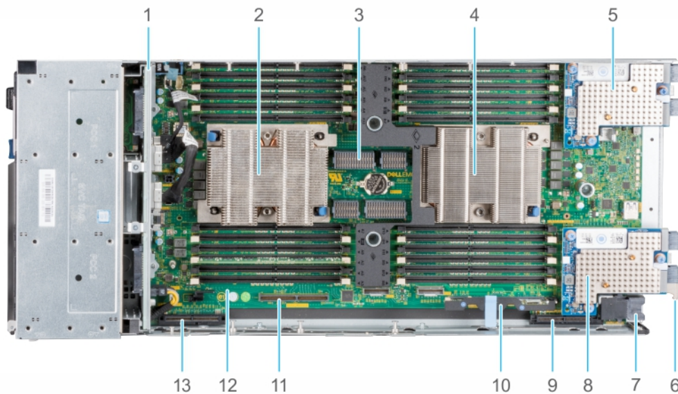
图 3: 带系统板的底座内部组件
