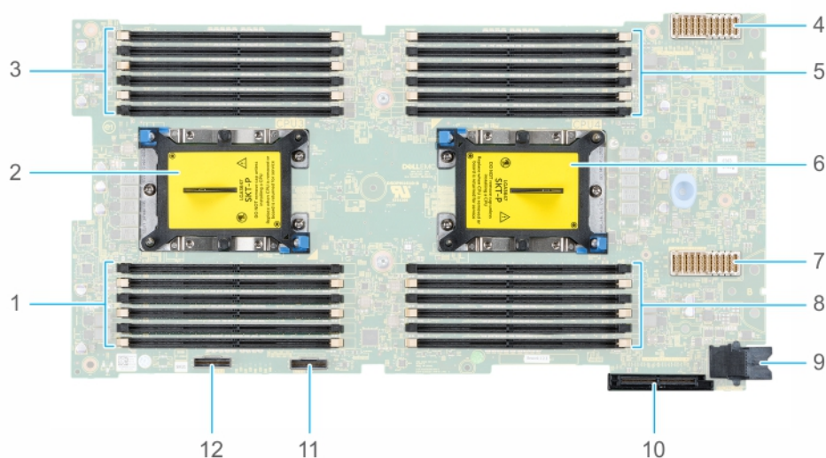
Figure 92. Connecteurs et cavaliers de la carte PEM
