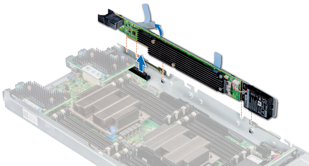
Figure 64. Retrait de la carte PERC Jumbo
