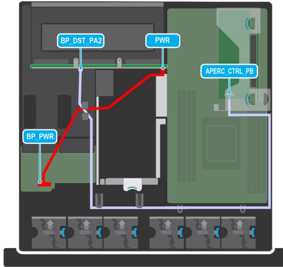
Ilustración 94. Cable NVMe PERC PB con un backplane de 6 x 2,5 pulgadas
