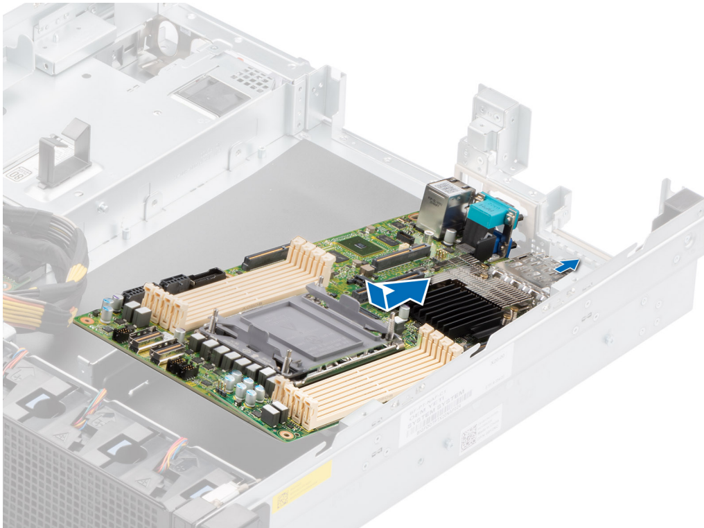
Ilustración 140. Instalación de la tarjeta madre
