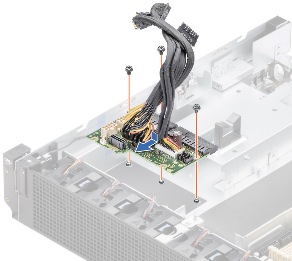
Ilustración 136. Instalación de la placa mediadora de alimentación
