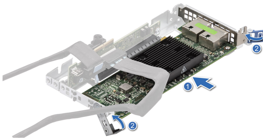
Ilustración 57. Instalación de una tarjeta de expansión de altura completa en la tarjeta elevadora 1A
