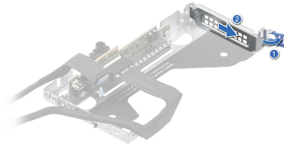
Ilustración 54. Extracción del soporte de relleno de la tarjeta elevadora 1A
