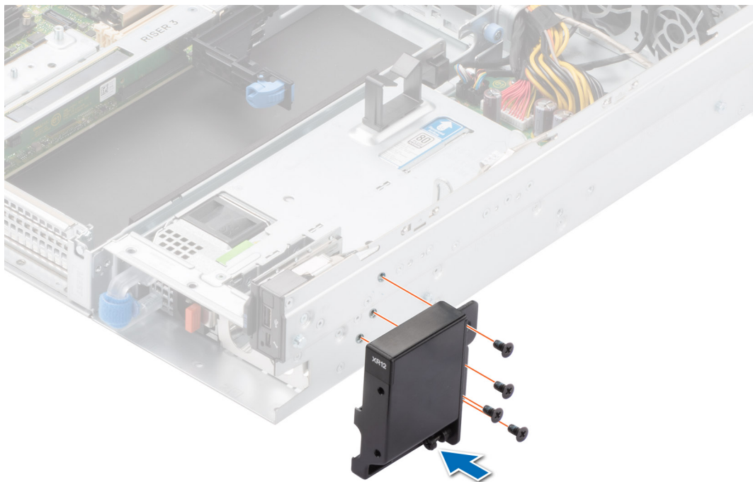
Ilustración 157. Instalación del panel de control del botón de encendido para la configuración de acceso frontal
