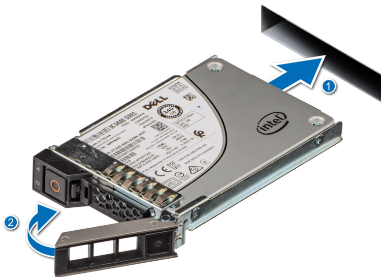
Ilustración 87. Instalación de un portaunidades
