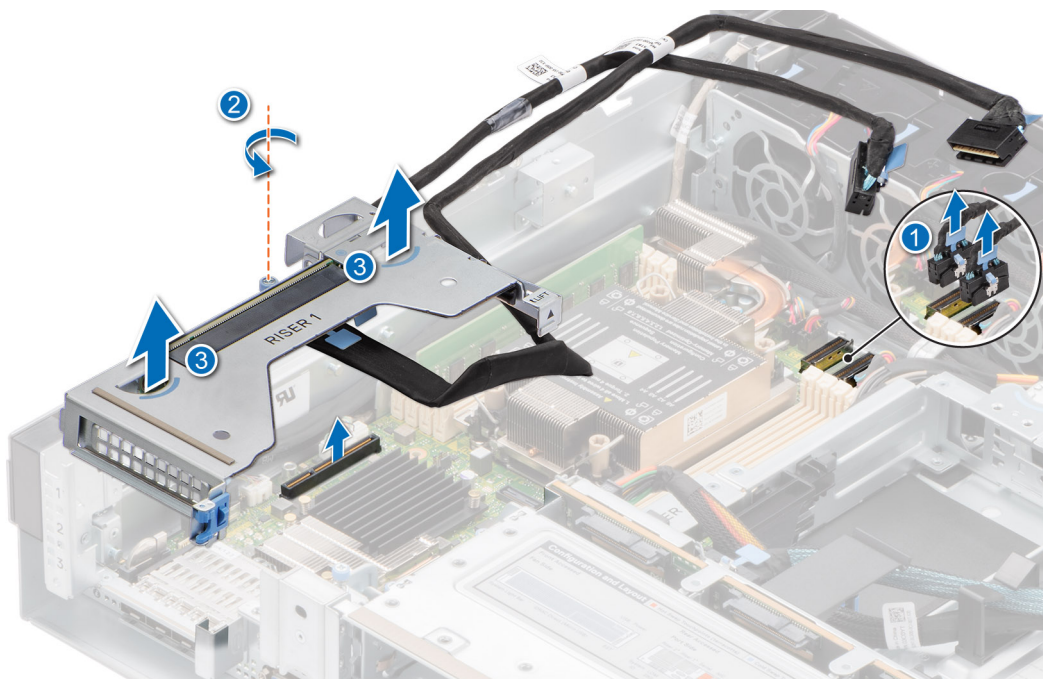
Ilustración 40. Extracción de la tarjeta elevadora para tarjetas de expansión 1A
