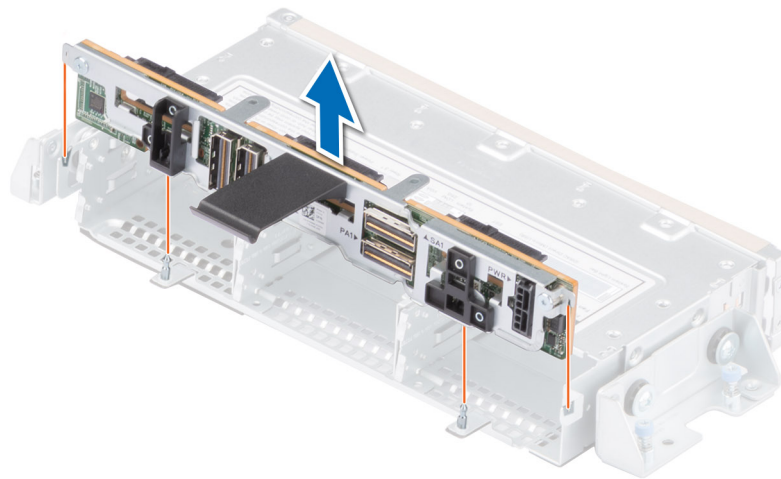
Ilustración 91. Extracción del backplane de la unidad
