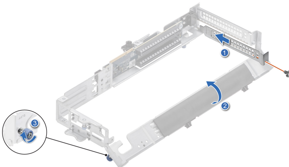
Ilustración 77. Instalación del soporte de relleno en la tarjeta elevadora 3B
