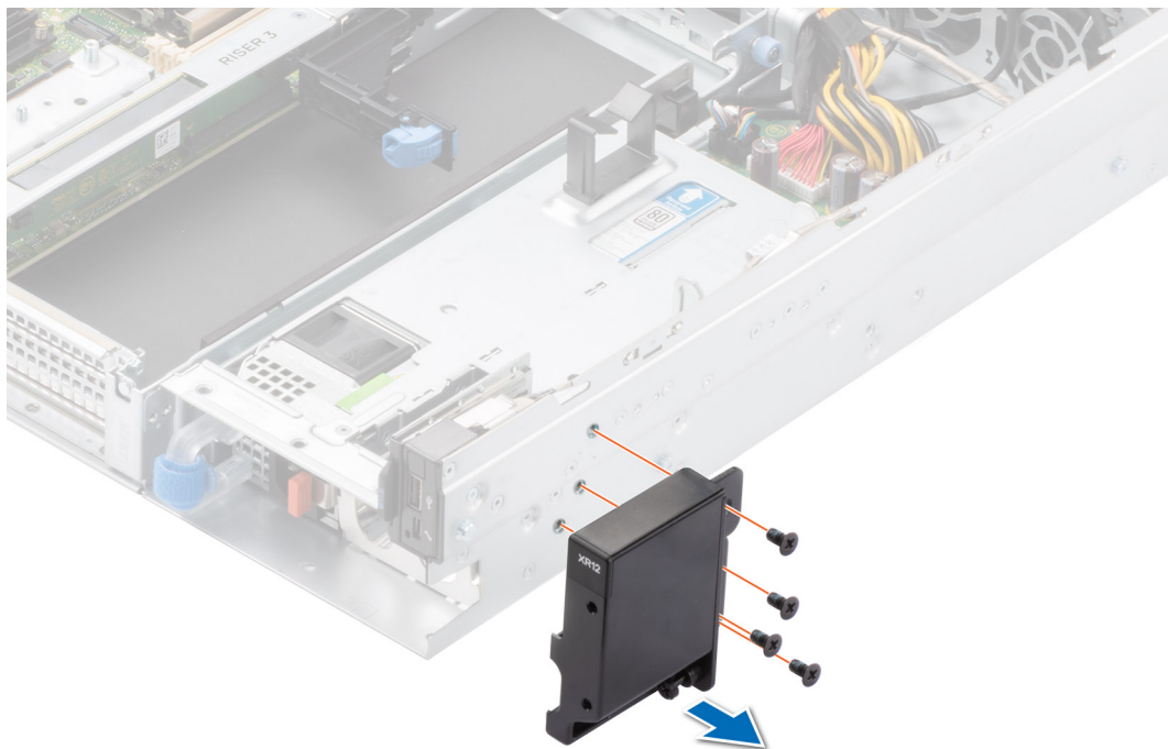
Ilustración 152. Extracción del panel de control del botón de encendido para la configuración de acceso posterior
