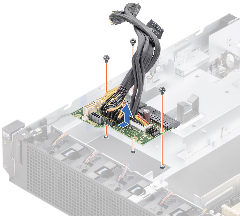
Ilustración 135. Extracción de la placa mediadora de alimentación
