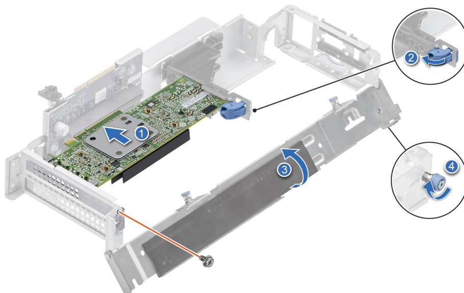
Ilustración 72. Instalación de una tarjeta de expansión de longitud media y bajo perfil en la tarjeta elevadora 2B
