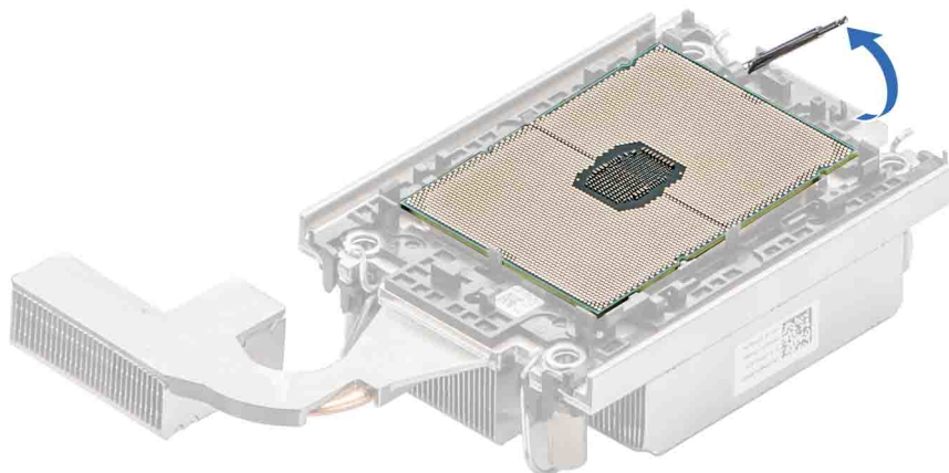
Ilustración 115. Levante la palanca de liberación del TIM
