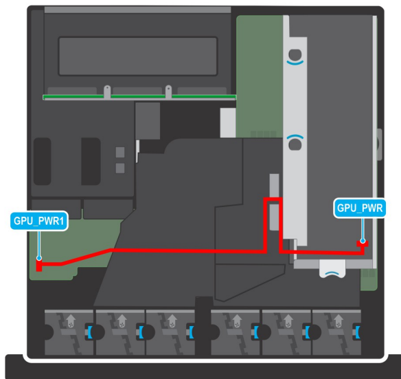
Ilustración 101. PIB a la tarjeta elevadora 2 con GPU de ancho doble y longitud completa
