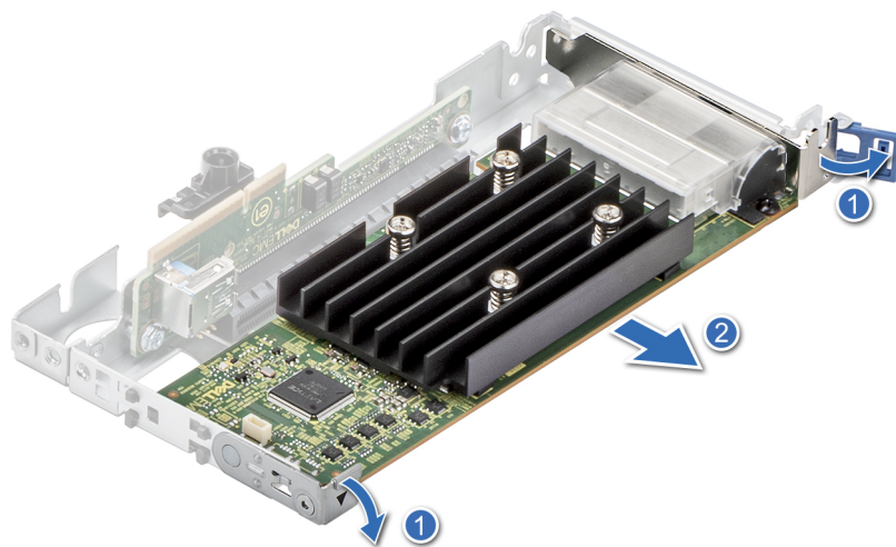
Ilustración 51. Extracción de una tarjeta de expansión de altura completa de la tarjeta elevadora 1B
