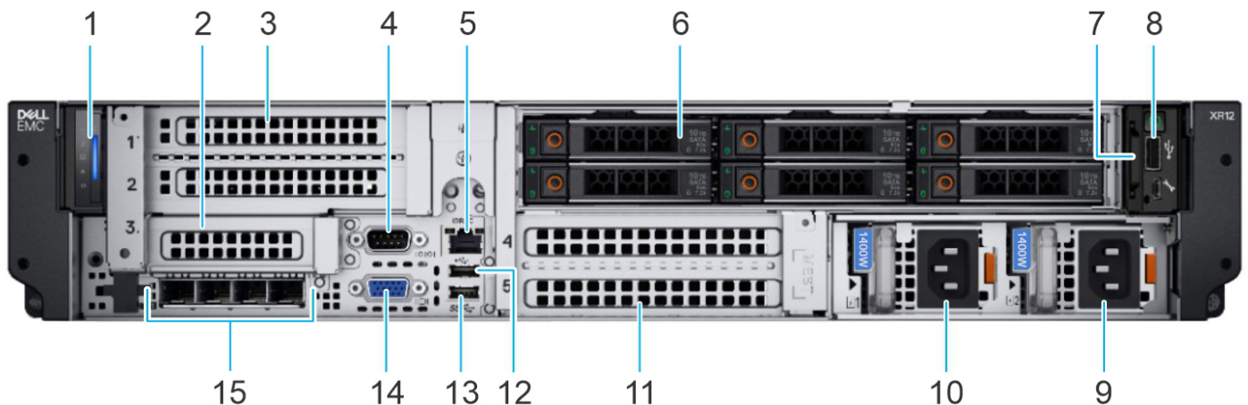
Ilustración 2. Vista frontal de la configuración de 6 unidades de 2,5 pulgadas de acceso frontal
