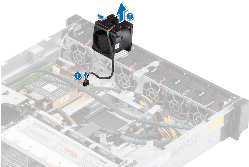
Ilustración 106. Extracción de un ventilador
