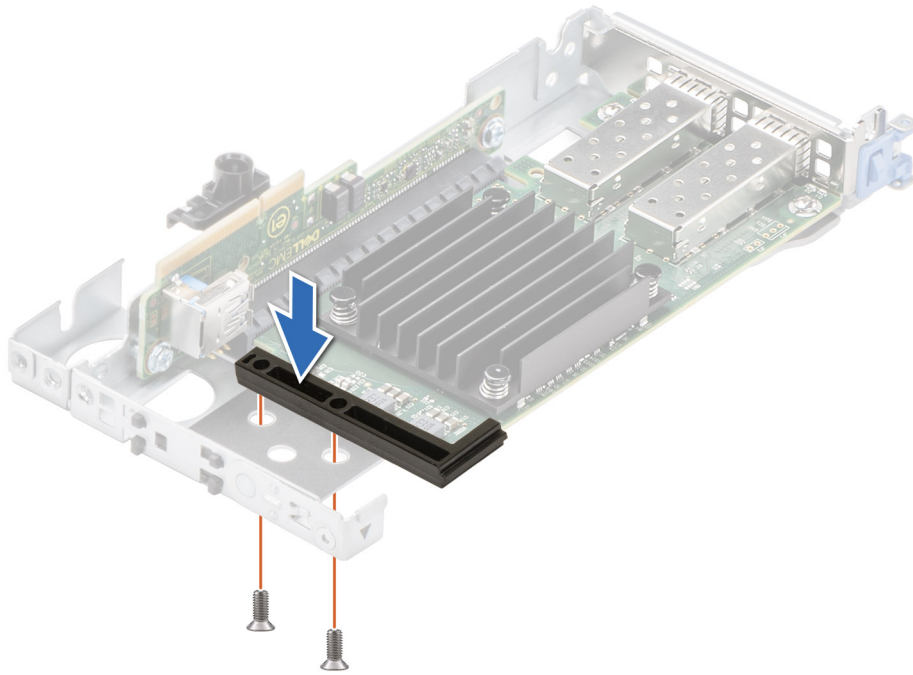
Ilustración 160. Instalación del soporte para tarjetas de expansión en la tarjeta elevadora 1 para tarjetas de expansión de longitud media
