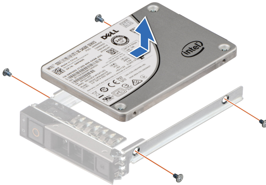
Ilustración 88. Extracción de una unidad del portaunidades
