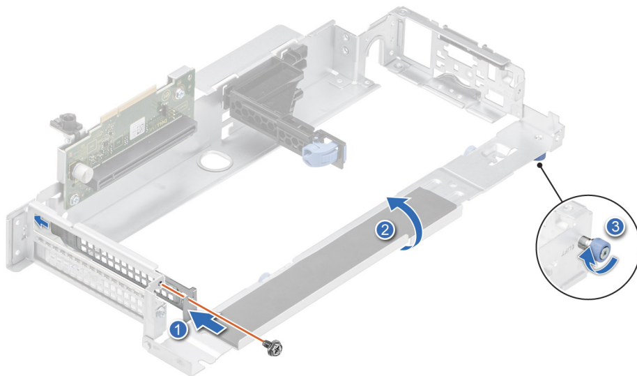
Ilustración 64. Instalación del soporte de relleno en la tarjeta elevadora 2A
