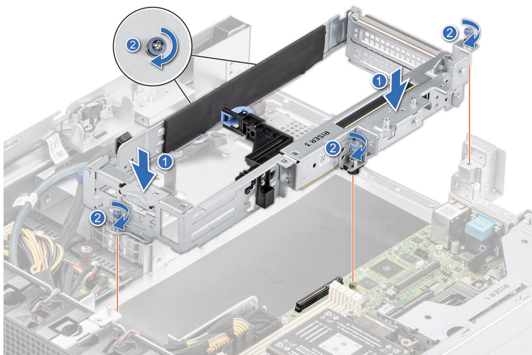
Ilustración 47. Instalación de la tarjeta elevadora para tarjetas de expansión 3
