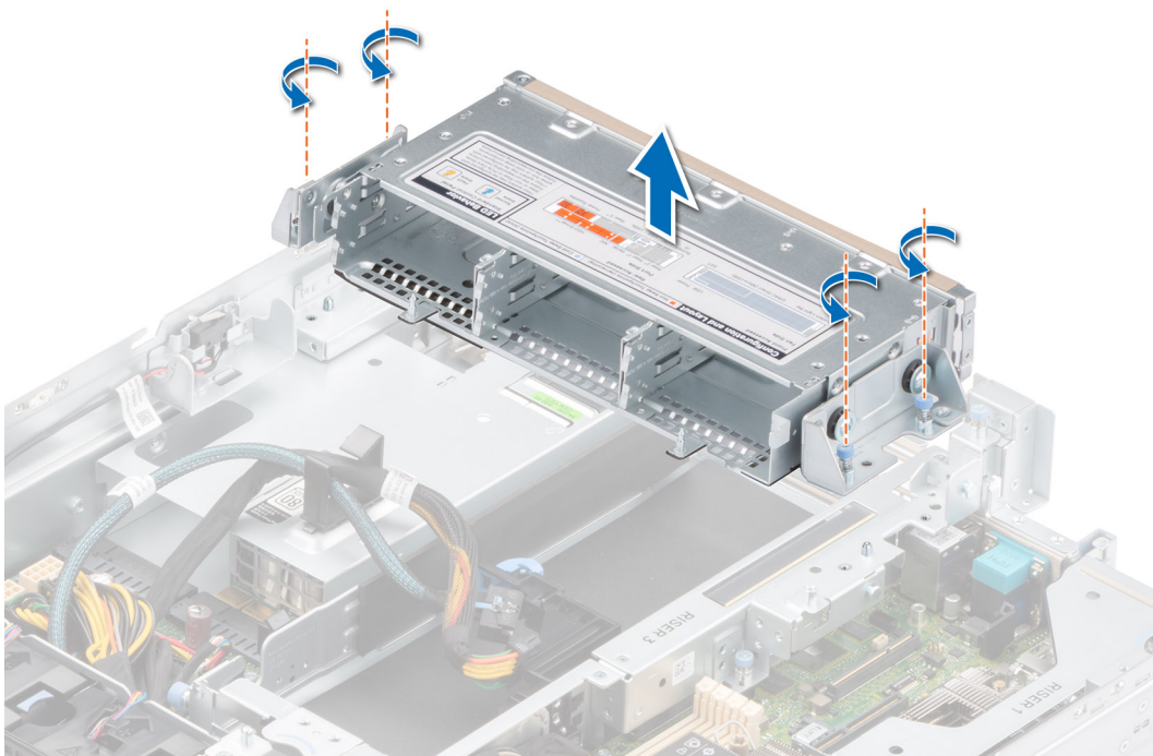
Ilustración 104. Extracción de la caja de la unidad
