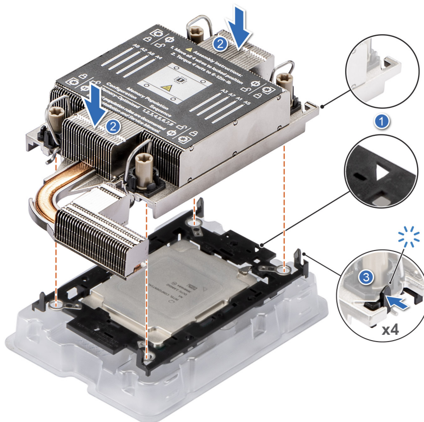
Ilustración 122. Instalación del disipador de calor en el procesador.
