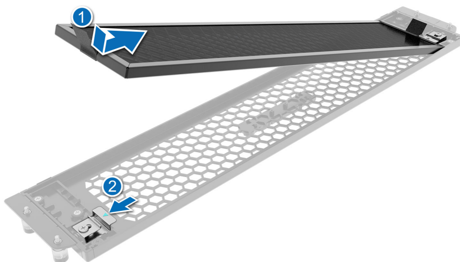
Ilustración 25. Instalación del filtro del bisel para la configuración de acceso posterior
