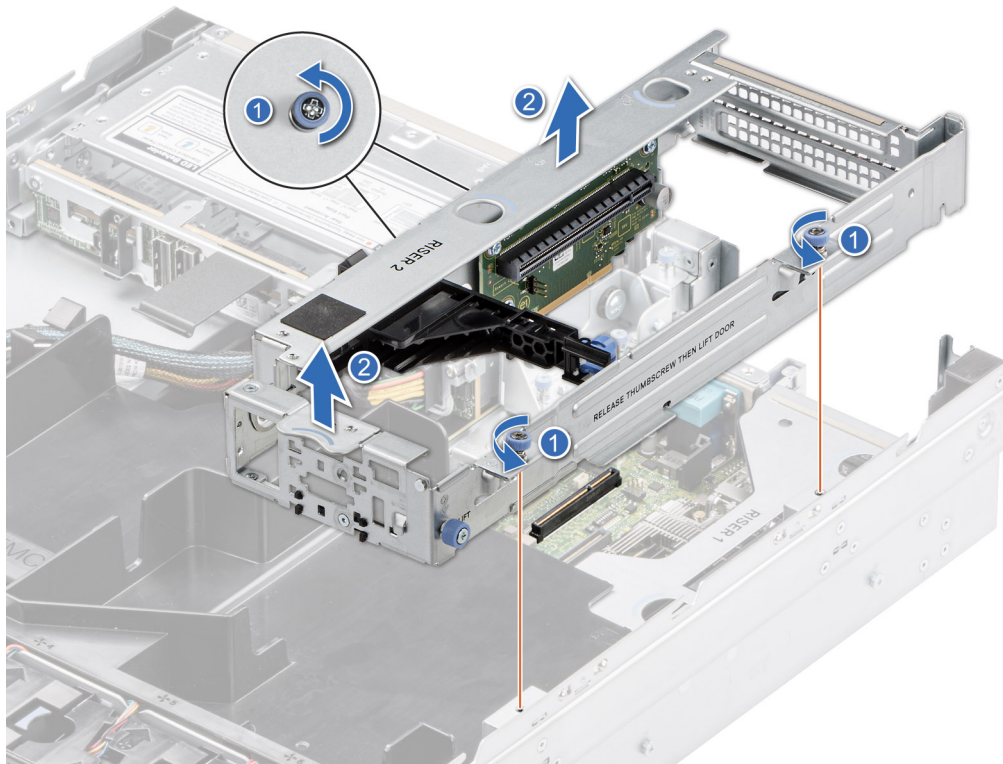
Ilustración 44. Extracción de la tarjeta elevadora para tarjetas de expansión 2
