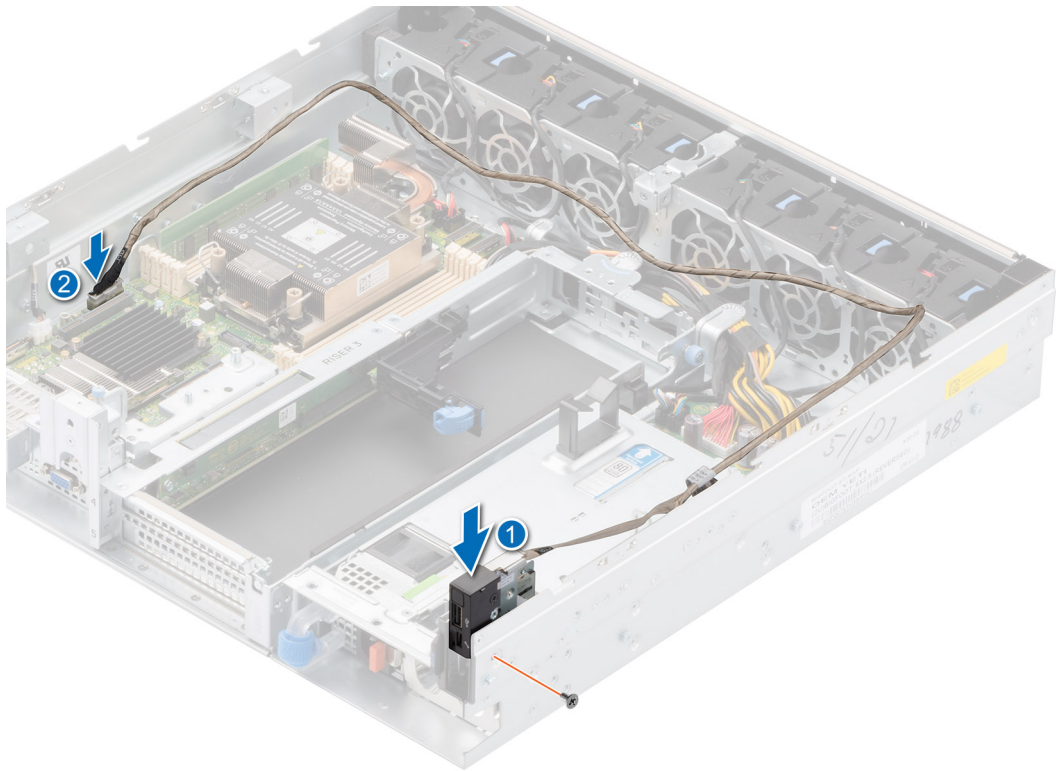
Ilustración 157. Instalación del panel de control del botón de encendido para la configuración de acceso frontal
