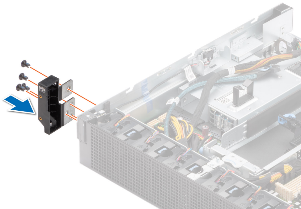
Ilustración 148. Instalación de la lengüeta izquierda para la configuración de acceso posterior
