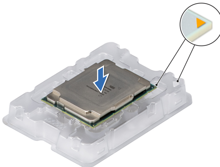
Ilustración 116. Alineación de las marcas de la pata 1 del procesador con la bandeja
