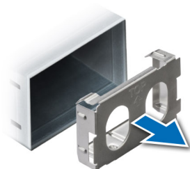
Ilustración 131. Extracción de una fuente de alimentación de relleno
