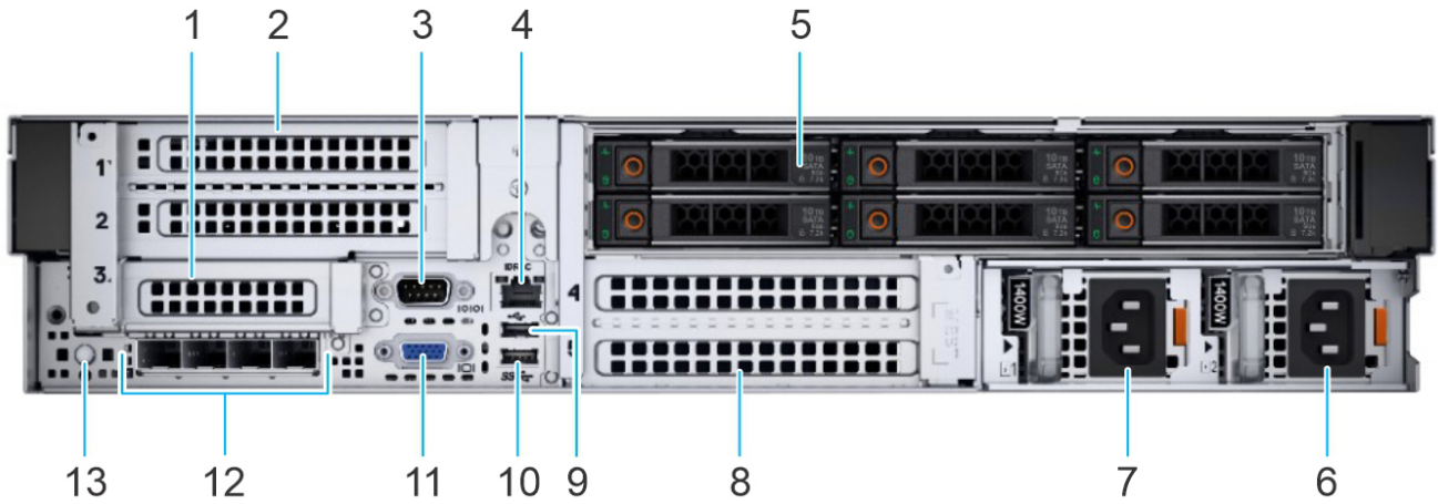
Ilustración 3. Vista posterior de la configuración de 6 unidades 2,5 pulgadas de acceso posterior
