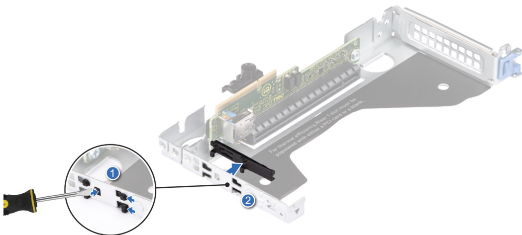
Ilustración 161. Extracción del soporte para tarjetas de expansión de la tarjeta elevadora 1
