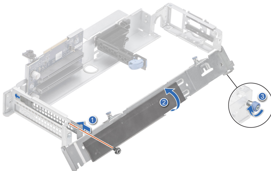
Ilustración 65. Instalación del soporte de relleno en la tarjeta elevadora 2B
