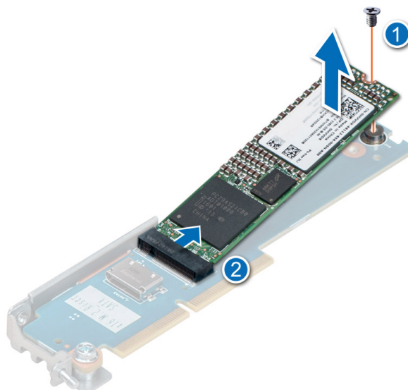
Ilustración 129. Extracción del módulo de SSD M.2
