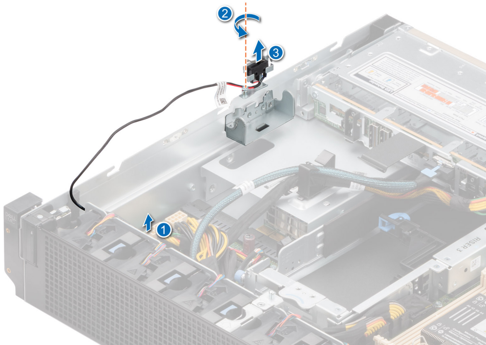
Ilustración 108. Extracción del módulo del interruptor de intrusiones
