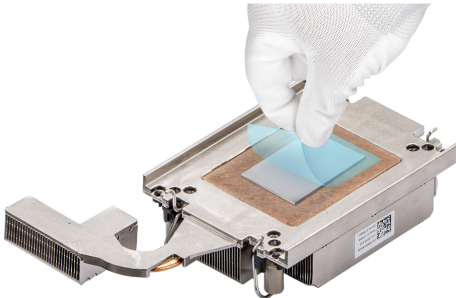
Ilustración 121. Extraiga la película de protección del material de interfaz térmica (TIM)
