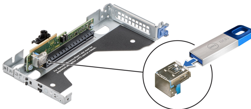
Ilustración 126. Instalación de la llave de memoria USB interna
