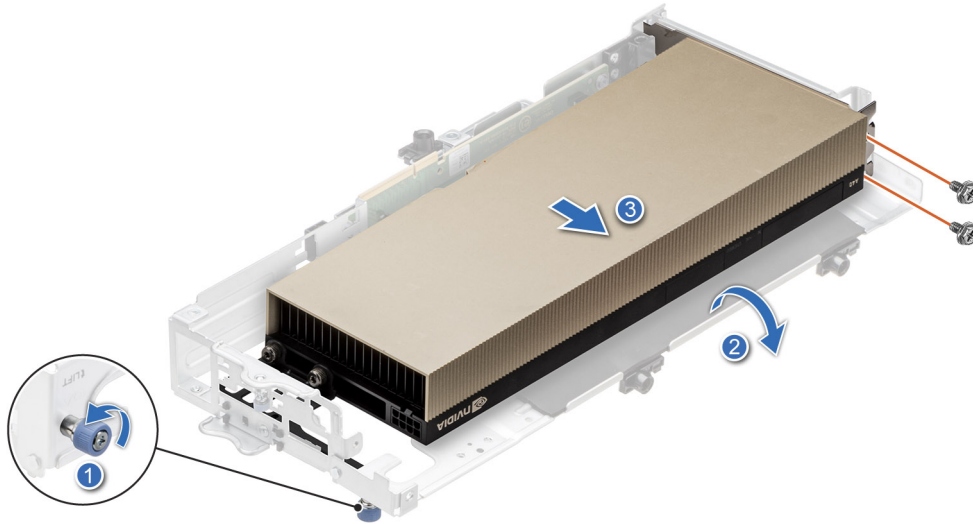
Ilustración 73. Extracción de una tarjeta GPU de longitud completa y ancho doble de la tarjeta elevadora 3A
