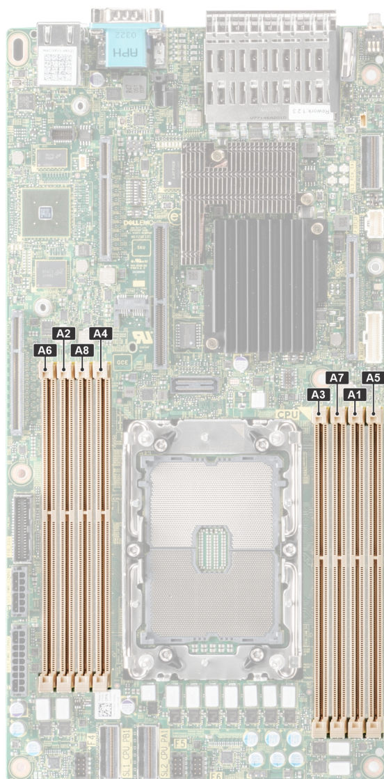
Ilustración 110. Zócalos de memoria en la tarjeta madre del sistema
