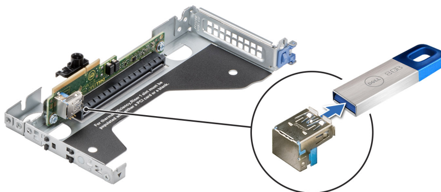
Ilustración 125. Extracción de la llave de memoria USB interna
