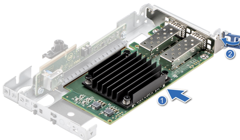
Ilustración 58. Instalación de una tarjeta de expansión de longitud media en la tarjeta elevadora 1B
