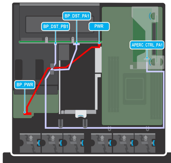
Ilustración 93. Cable NVMe PERC PA con un backplane de 6 x 2,5 pulgadas
