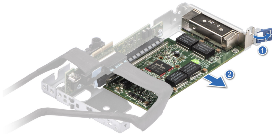
Ilustración 48. Extracción de una tarjeta de expansión de longitud media de la tarjeta elevadora 1A
