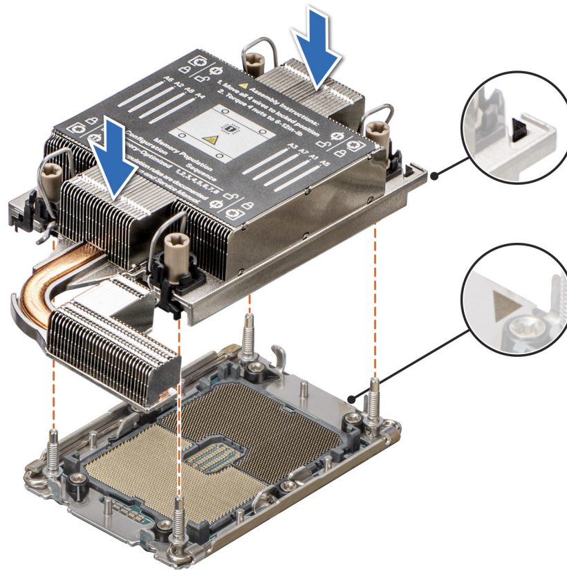
Ilustración 123. Instalación del módulo del procesador y del disipador de calor (PHM).
