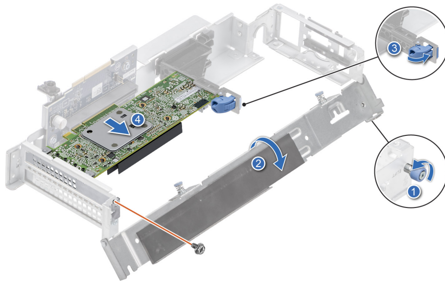
Ilustración 63. Extracción de una tarjeta de expansión de longitud media y bajo perfil de la tarjeta elevadora 2B
