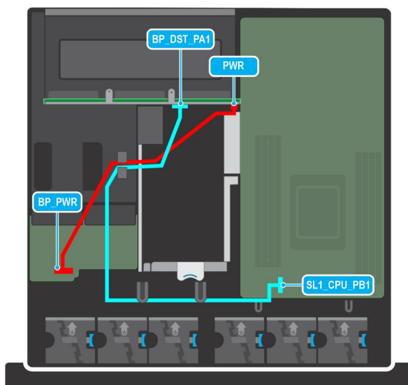
Ilustración 97. Conector del cable NVMe con un backplane de 6 x 2,5 pulgadas
