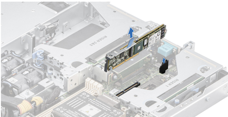
Ilustración 127. Extracción de la tarjeta de Boot Optimized Storage Subsystem M.2 de la tarjeta madre
