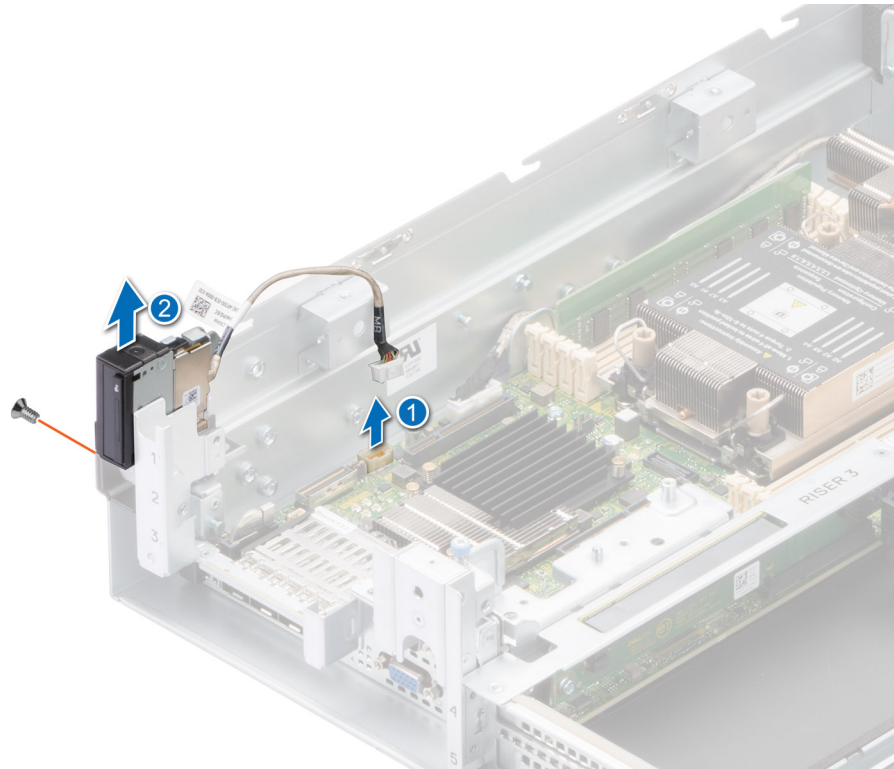
Ilustración 146. Extracción del panel de control del LED de estado para la configuración de acceso frontal
