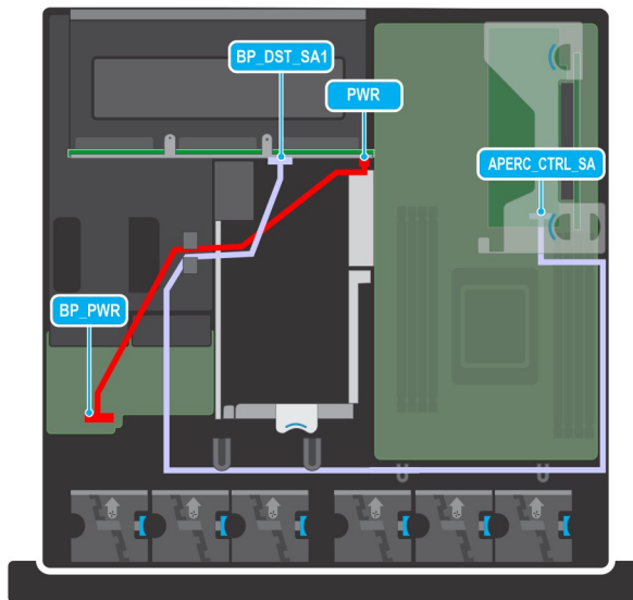
Ilustración 95. Cable de SAS SA PERC con un backplane de 6 x 2,5 pulgadas
