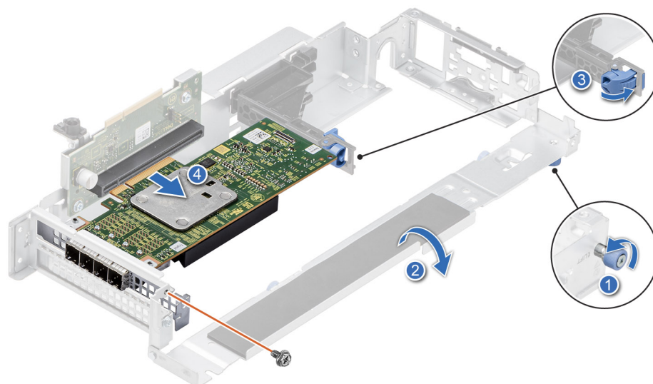
Ilustración 62. Extracción de una tarjeta de expansión de longitud media y bajo perfil de la tarjeta elevadora 2A
