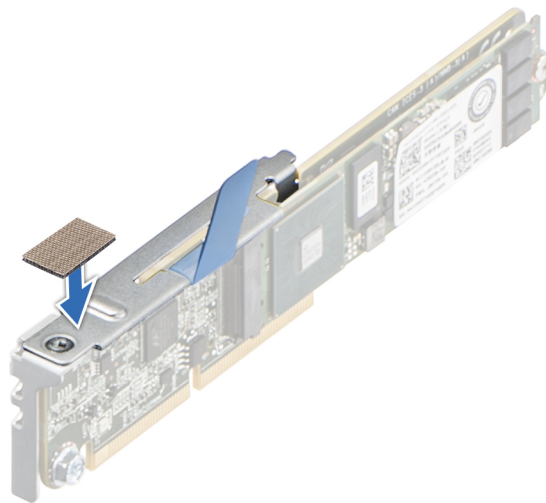
Ilustración 163. Pegado de la espuma en la tarjeta BOSS M.2
