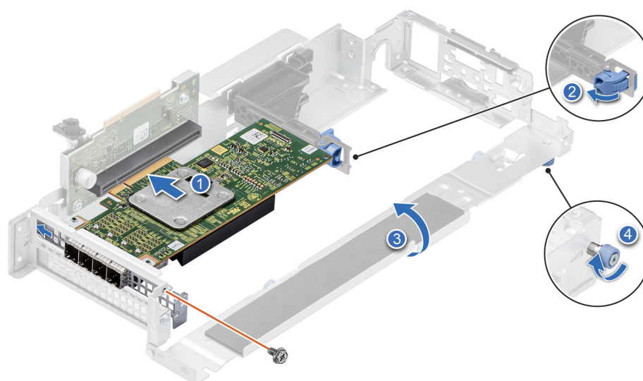
Ilustración 71. Instalación de una tarjeta de expansión de longitud media y bajo perfil en la tarjeta elevadora 2A
