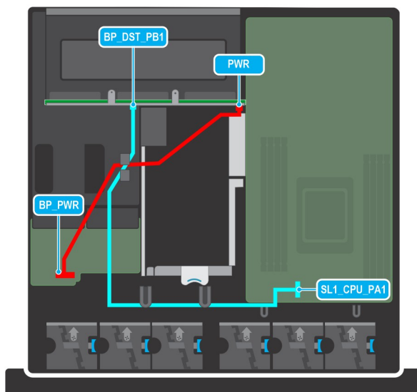
Ilustración 98. Conector del cable NVMe con un backplane de 6 x 2,5 pulgadas
