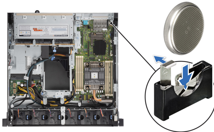
Ilustración 138. Instalación de la batería del sistema
