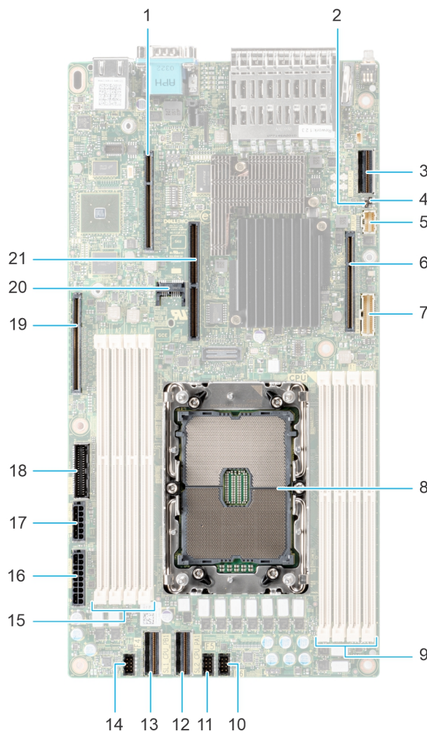
Ilustración 167. Puentes y conectores de la tarjeta madre
