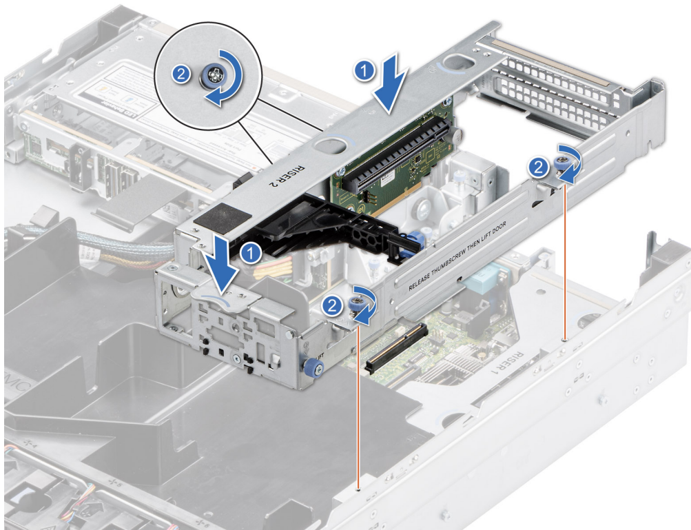
Ilustración 45. Instalación de la tarjeta elevadora para tarjetas de expansión 2
