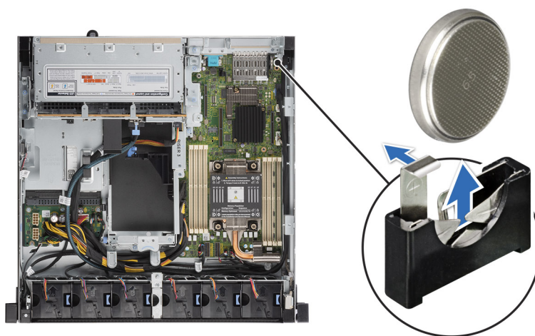
Ilustración 137. Extracción de la batería del sistema
