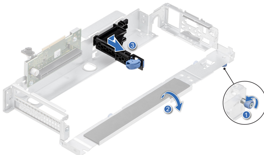
Ilustración 159. Extracción de la guía de la tarjeta plástica de la tarjeta elevadora
