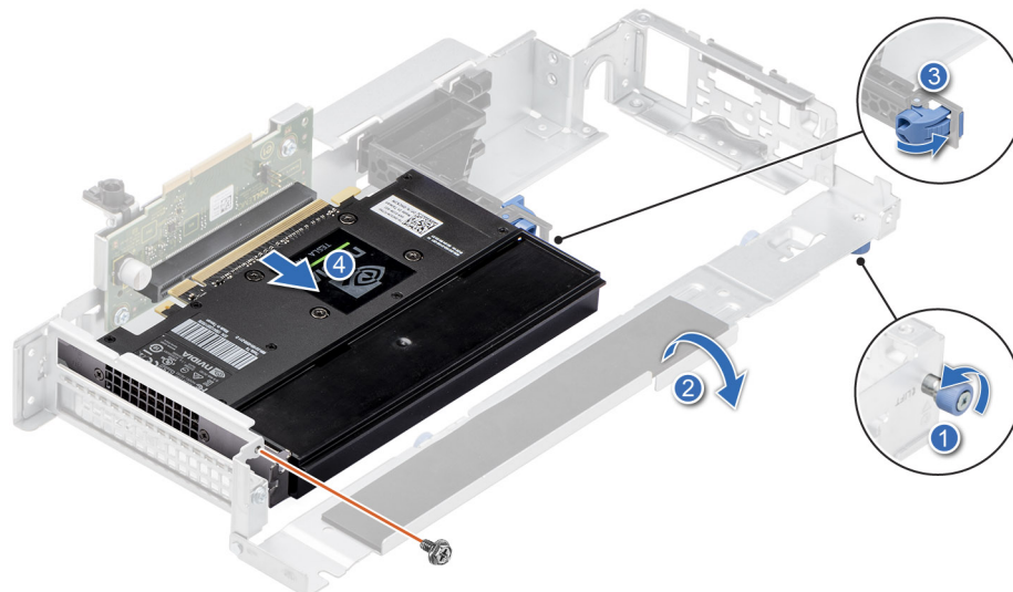
Ilustración 60. Extracción de una tarjeta GPU de expansión de altura completa y longitud media de la tarjeta elevadora 2A
