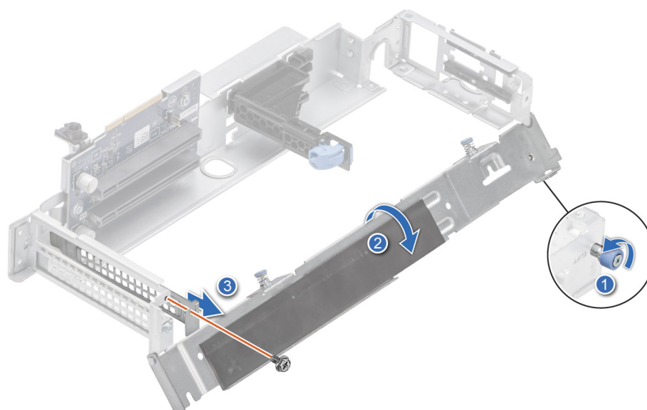
Ilustración 67. Extracción del soporte de relleno de la tarjeta elevadora 2B
