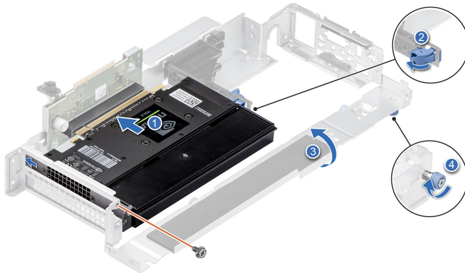
Ilustración 68. Instalación de una tarjeta GPU de altura completa y longitud media en la tarjeta elevadora 2A
