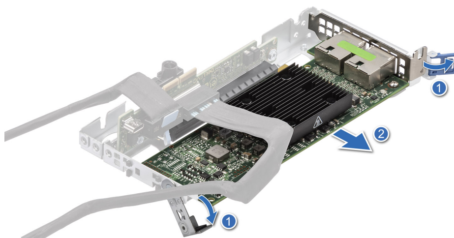
Ilustración 49. Extracción de una tarjeta de expansión de altura completa de la tarjeta elevadora 1A
