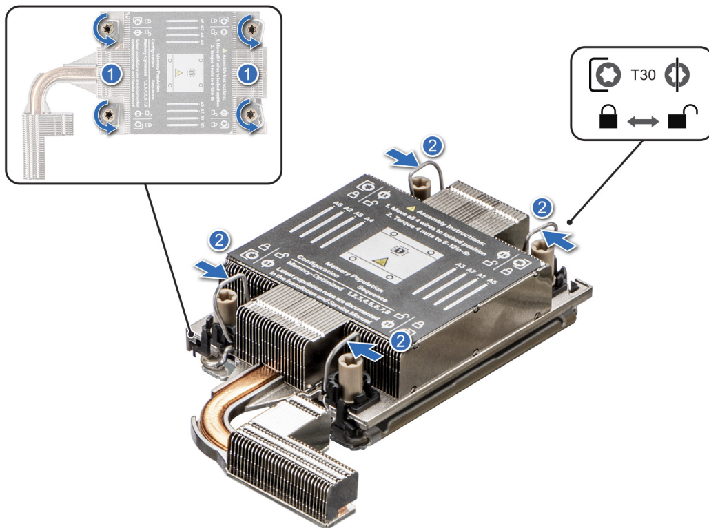
Ilustración 113. Aflojar las tuercas y establecer los cables de inclinación en la posición de desbloqueo
