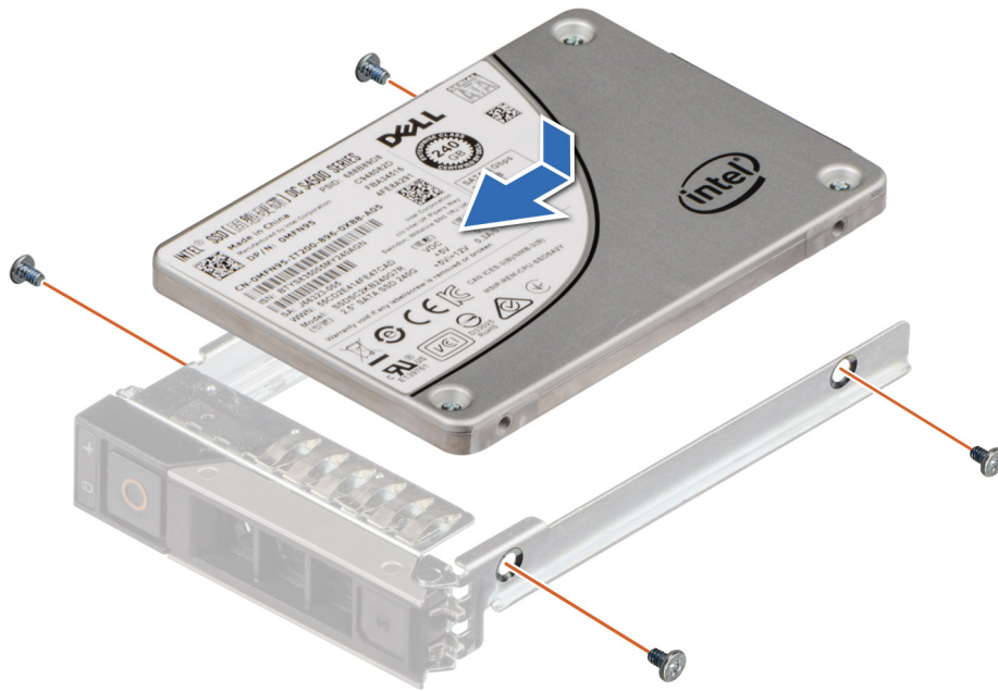
Ilustración 89. Instalación de una unidad en el portaunidades
