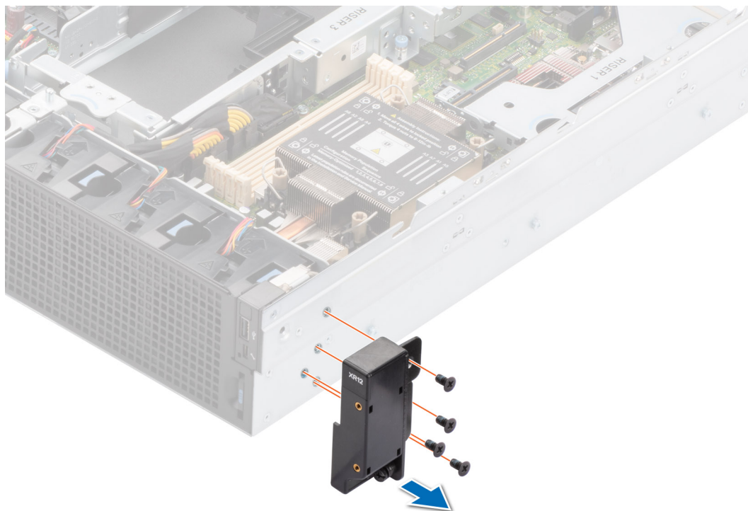
Ilustración 151. Extracción de la lengüeta derecha para la configuración de acceso posterior
