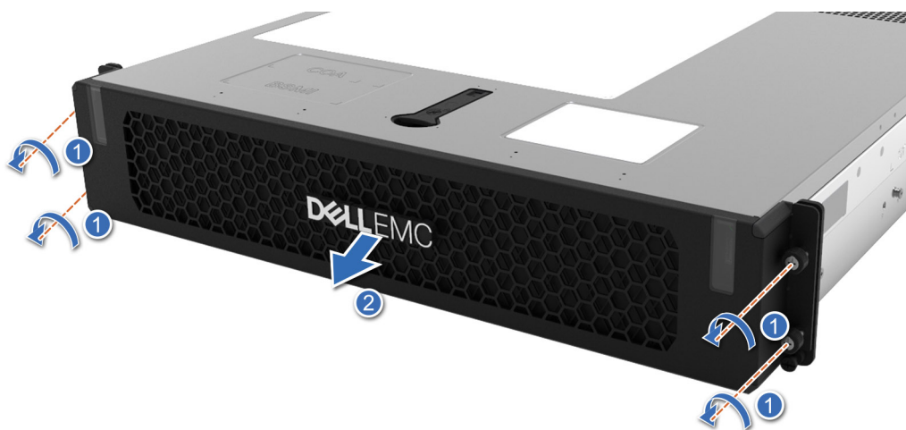
Ilustración 19. Extracción del bisel frontal para la configuración de acceso posterior
