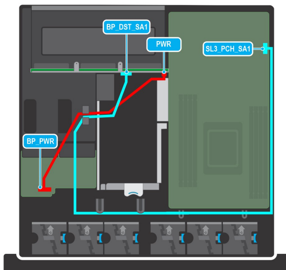
Ilustración 96. Conector del cable de SATA con un backplane de 6 x 2,5 pulgadas
