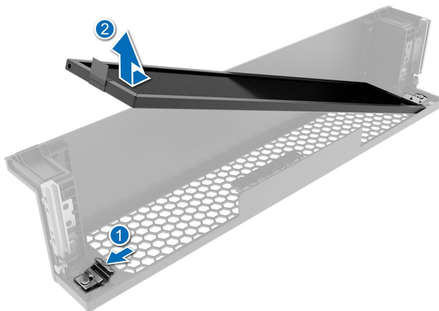
Ilustración 24. Extracción del filtro del bisel para la configuración de acceso frontal
