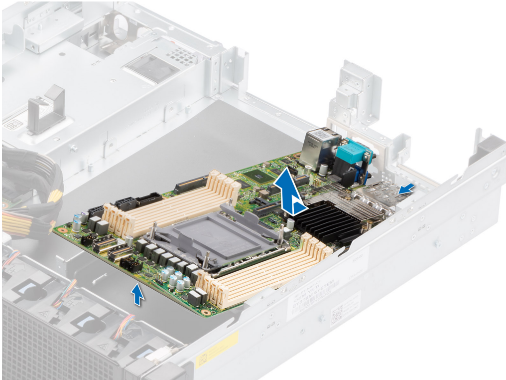
Ilustración 139. Extracción de la tarjeta madre
