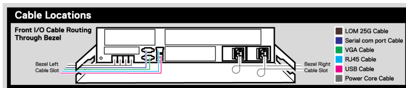
Ilustración 18. Cableado de SIL en el bisel frontal opcional
