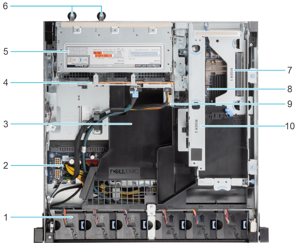
Ilustración 7. Interior del sistema: Configuración de acceso posterior
