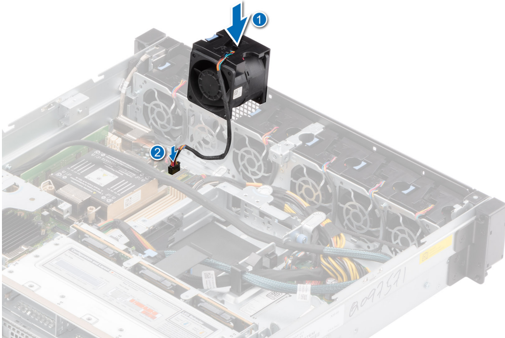
Ilustración 107. Instalación de un ventilador
