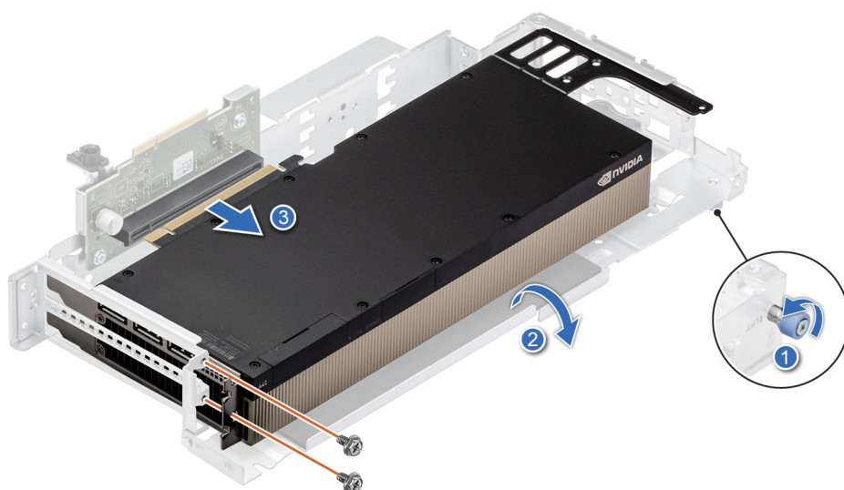
Ilustración 61. Extracción de una tarjeta GPU de longitud completa y ancho doble de la tarjeta elevadora 2A
