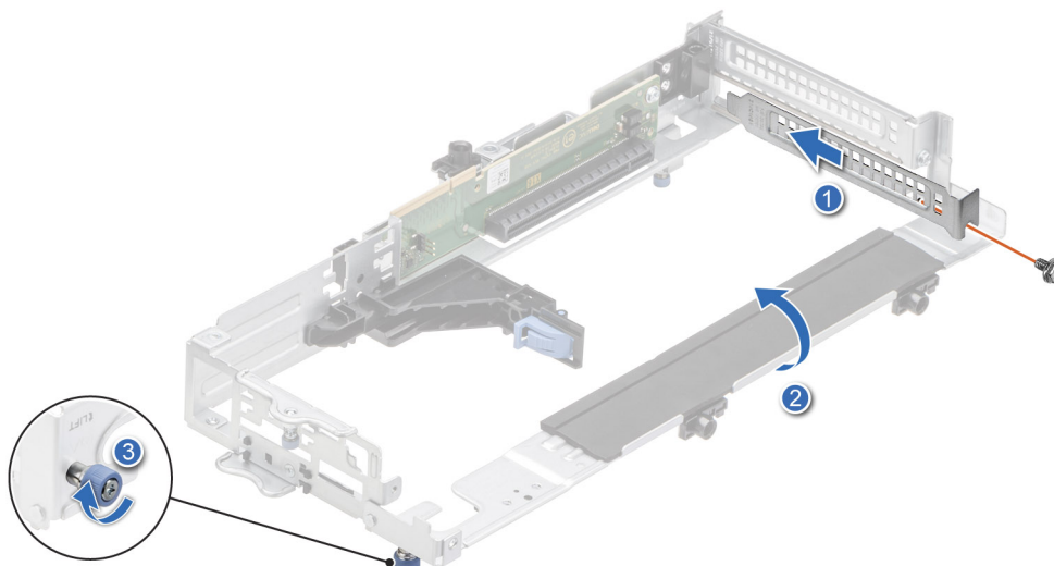
Ilustración 76. Instalación del soporte de relleno en la tarjeta elevadora 3A
