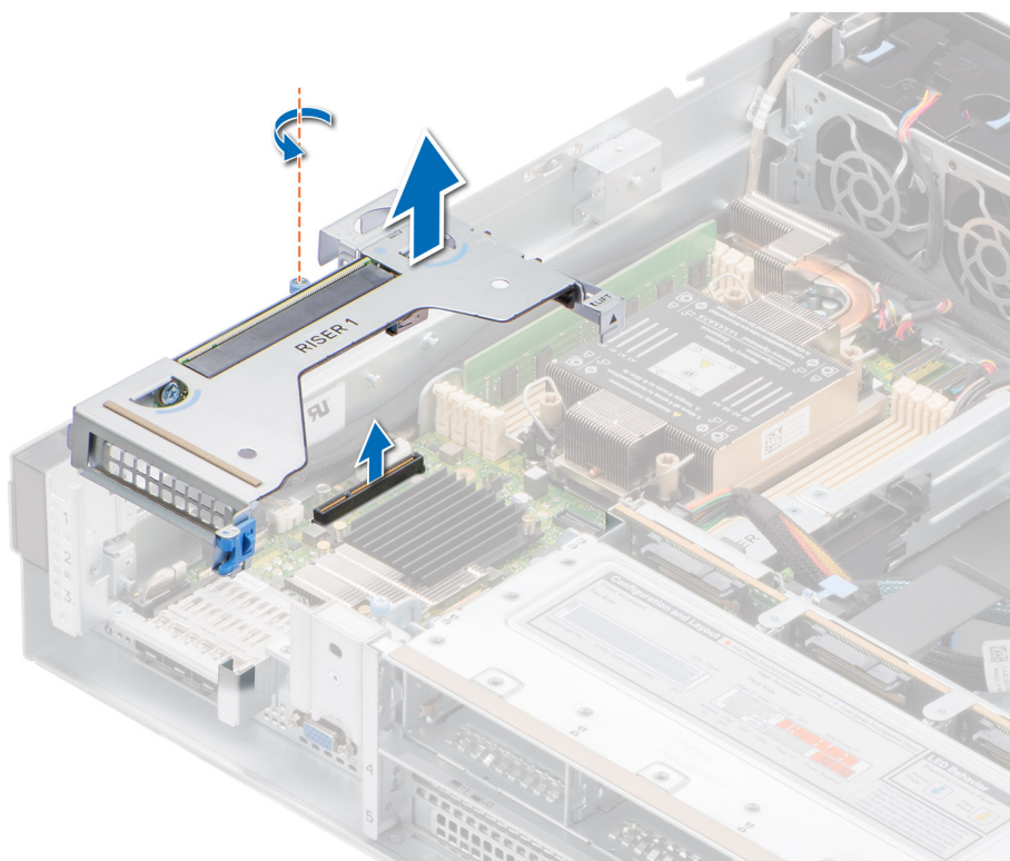
Ilustración 41. Extracción de la tarjeta elevadora para tarjetas de expansión 1B
