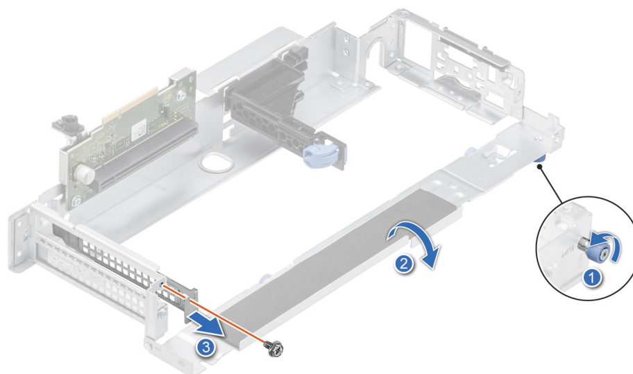
Ilustración 66. Extracción del soporte de relleno de la tarjeta elevadora 2A
