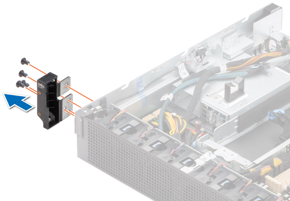
Ilustración 143. Extracción de la lengüeta izquierda para la configuración de acceso posterior
