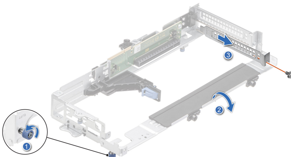
Ilustración 78. Extracción del soporte de relleno de la tarjeta elevadora 3A
