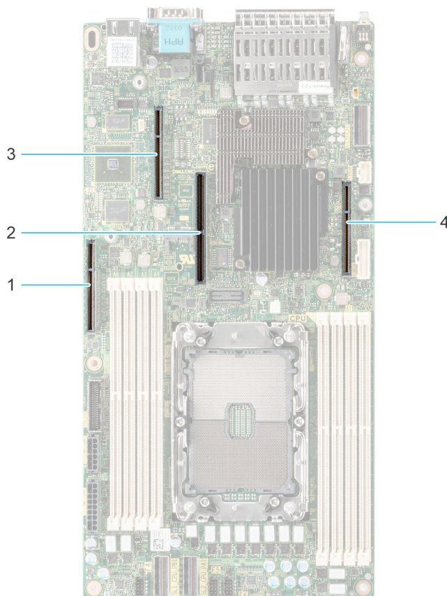
Ilustración 33. Conectores de la ranura de tarjeta de expansión
