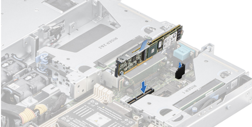
Ilustración 128. Instalación de la tarjeta de Boot Optimized Storage Subsystem M.2 en la tarjeta madre
