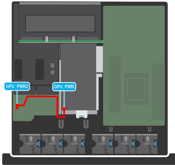
Ilustración 102. PIB a la tarjeta elevadora 3 con GPU de ancho doble y longitud completa
