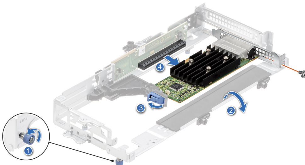
Ilustración 74. Extracción de una tarjeta de expansión de longitud media y bajo perfil de la tarjeta elevadora 3A
