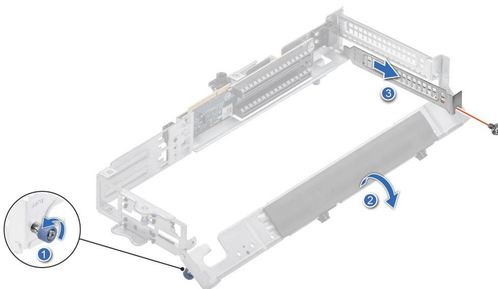
Ilustración 79. Extracción del soporte de relleno de la tarjeta elevadora 3B
