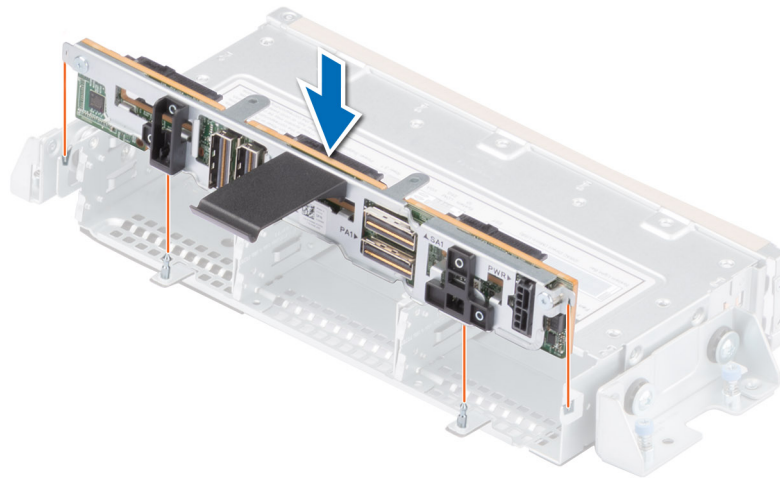
Ilustración 92. Instalación del backplane de la unidad
