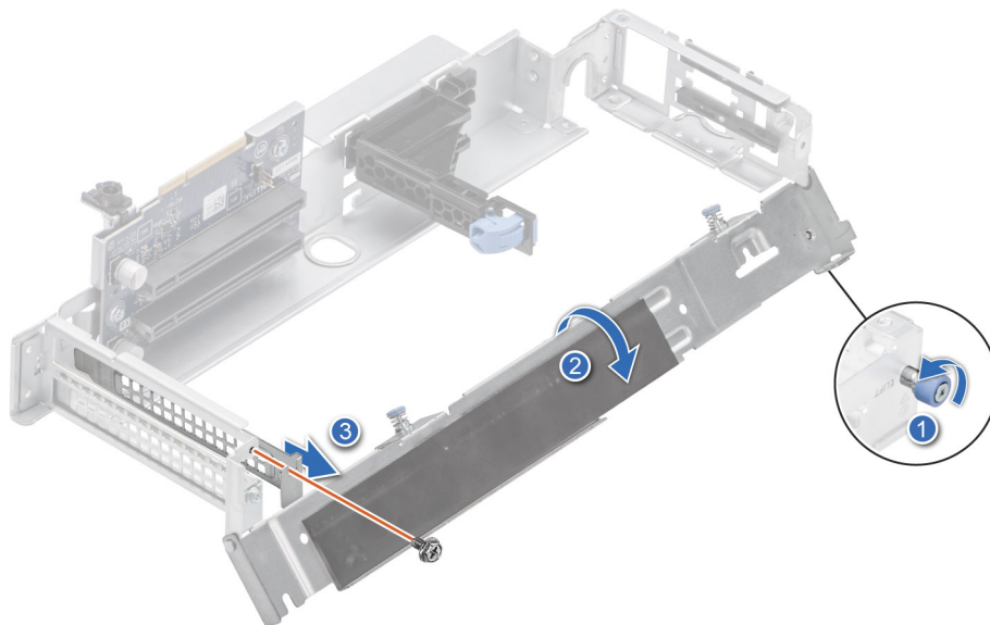
Abbildung 67. Entfernen eines Abdeckblechs aus Riser 2B
