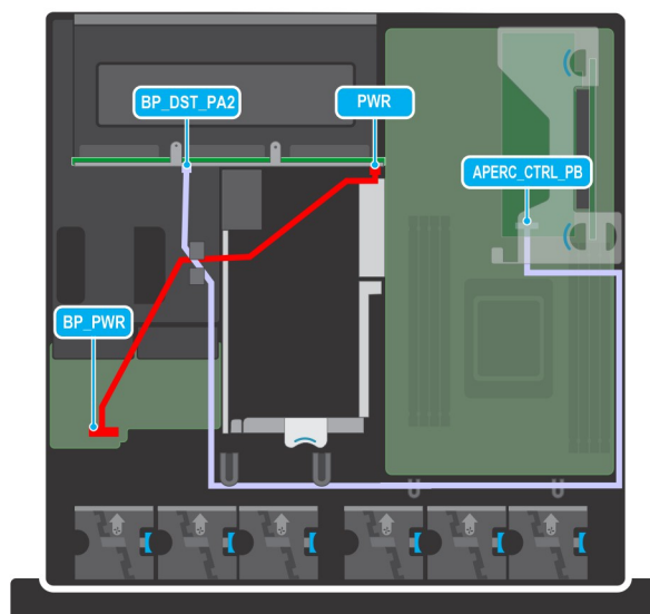
Abbildung 94. PERC PB NVMe-Kabel mit 6 x 2,5-Zoll-Rückwandplatine
