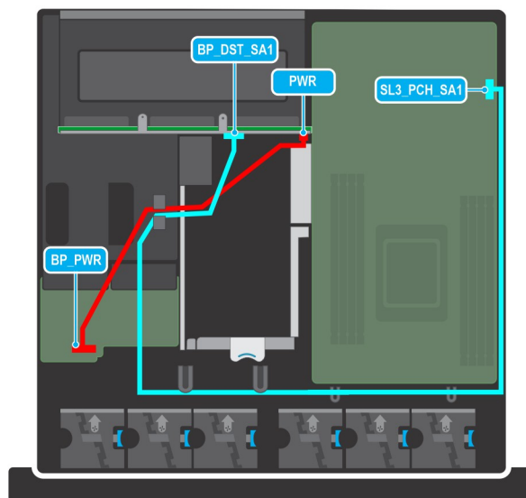
Abbildung 96. SATA-Kabelanschluss mit 6 x 2,5-Zoll-Rückwandplatine
