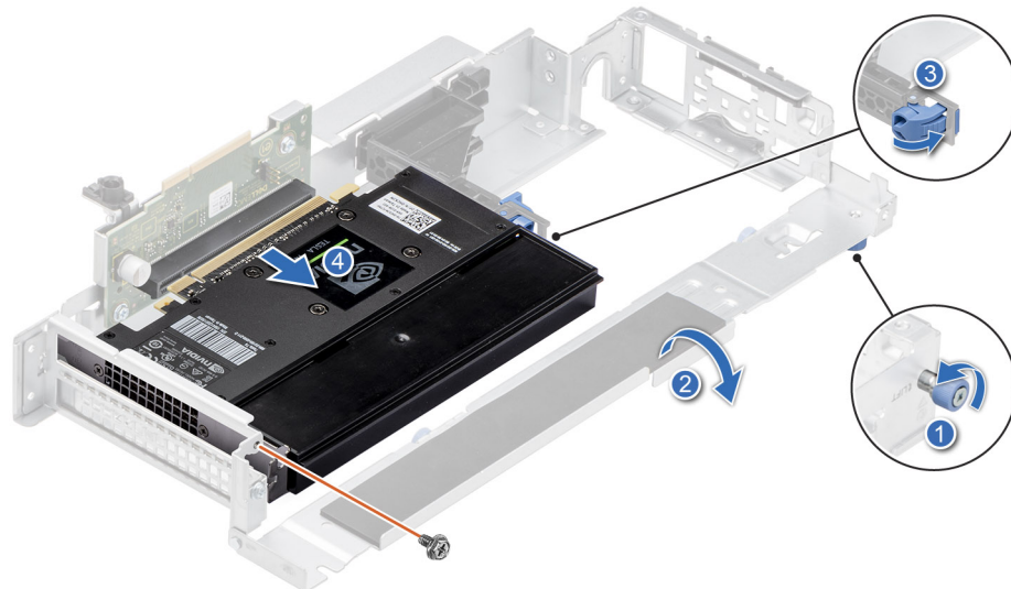
Abbildung 60. Entfernen einer GPU-Erweiterungskarte mit halber Länge und voller Höhe aus Riser 2A
