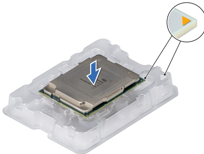
Abbildung 116. Ausrichten von Pin-1-Markierungen des Prozessors mit dem Schacht
