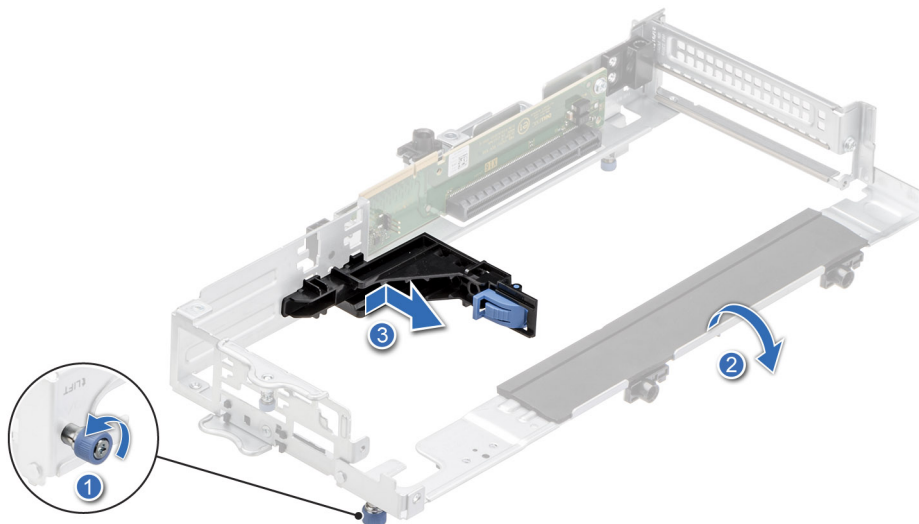
Abbildung 80. Entfernen der Kunststoffkartenführung von Riser 3
