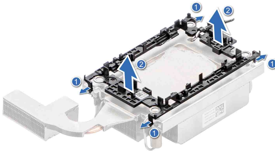
Abbildung 117. Entfernen des Prozessorträgers
