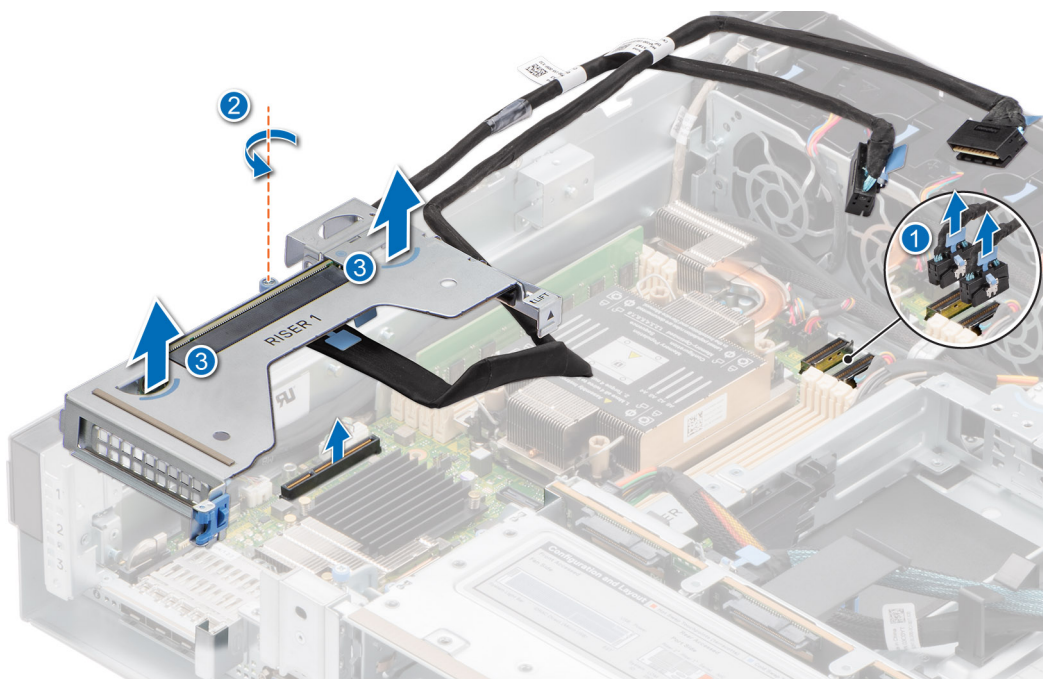
Abbildung 40. Entfernen des Erweiterungskarten-Risers 1A
