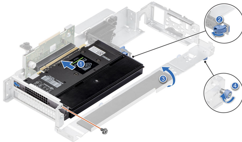
Abbildung 68. Installieren einer GPU-Karte mit halber Länge und voller Höhe in Riser 2A
