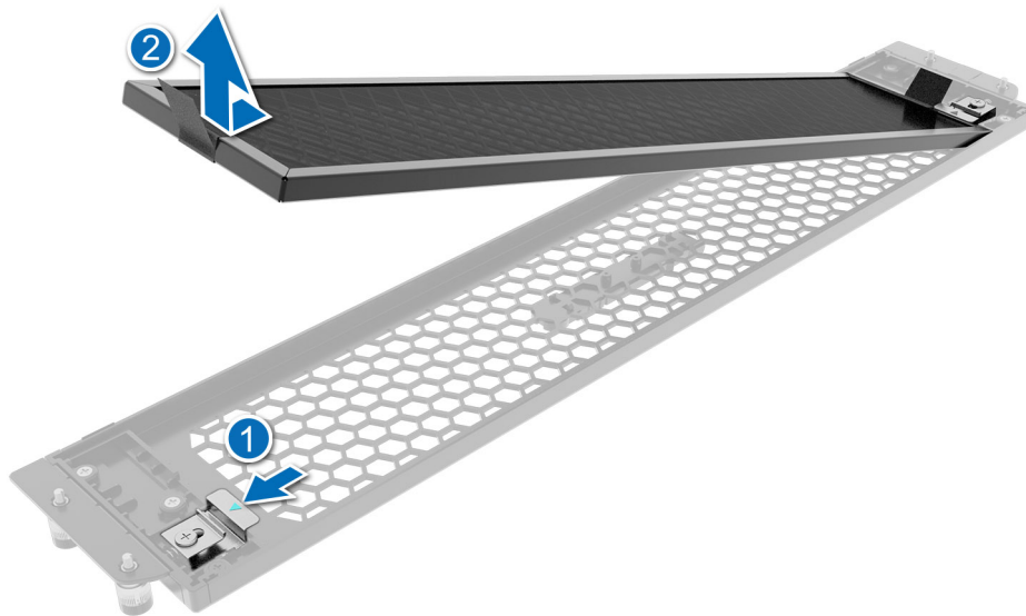
Abbildung 23. Entfernen des Blendenfilters für die rückseitig zugängliche Konfiguration
