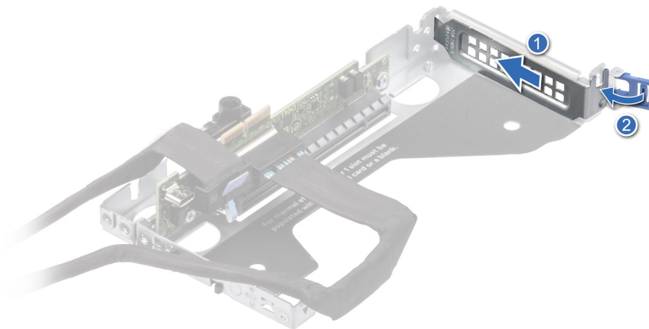
Abbildung 52. Einsetzen eines Abdeckblechs in Riser 1A
