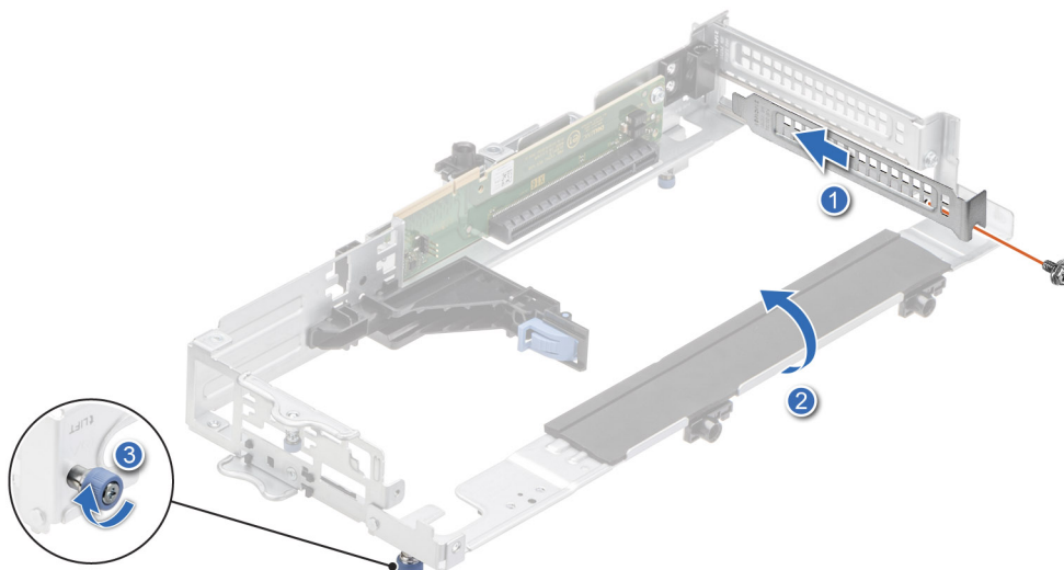
Abbildung 76. Einsetzen eines Abdeckblechs in Riser 3A
