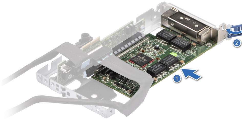
Abbildung 56. Einsetzen einer Erweiterungskarte mit halber Länge in Riser 1A
