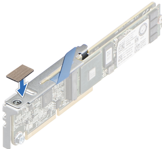
Abbildung 163. Kleben des Schaumstoffs auf die M.2-BOSS-Karte
