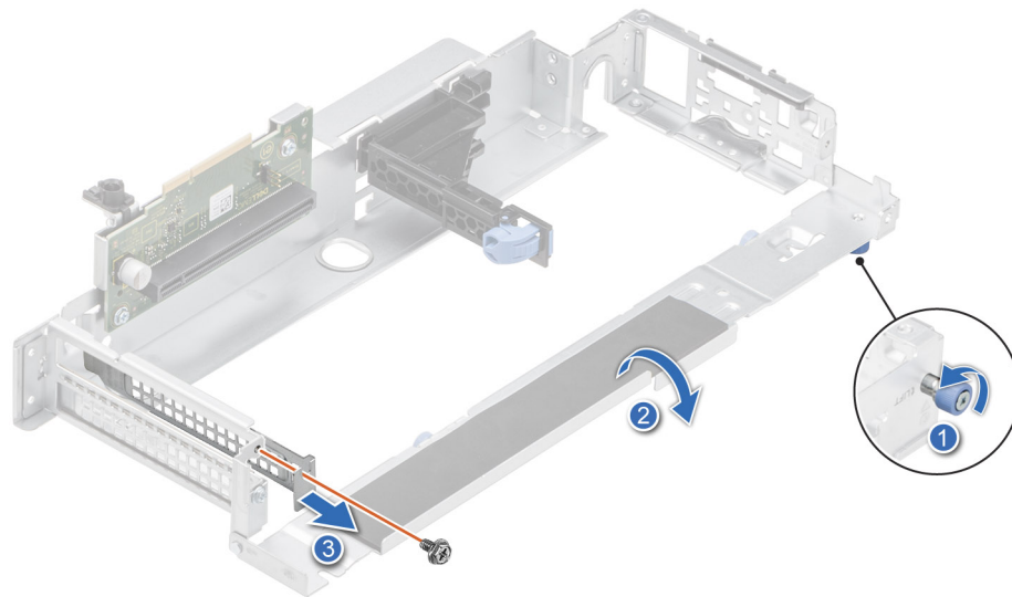
Abbildung 66. Entfernen eines Abdeckblechs aus Riser 2A
