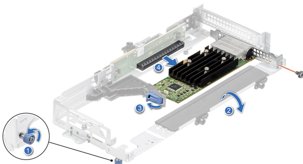
Abbildung 74. Entfernen einer Erweiterungskarte mit halber Länge und flachem Profil aus Riser 3A
