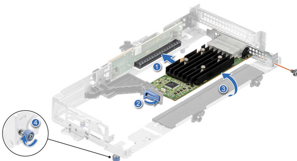
Abbildung 82. Installieren einer Erweiterungskarte mit halber Länge und flachem Profil in Riser 3A
