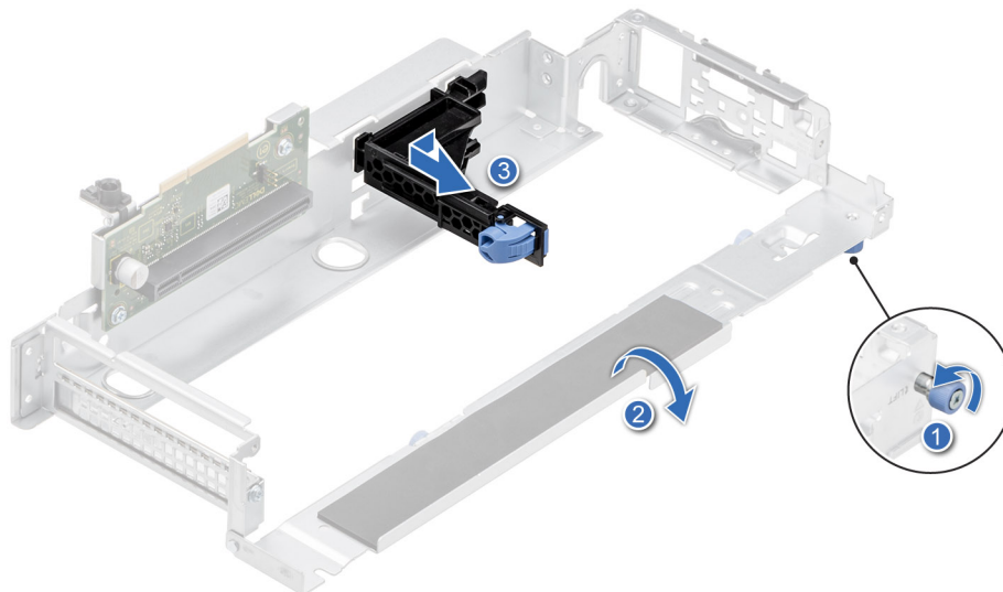
Abbildung 69. Entfernen der Kunststoffkartenführung vom Riser
