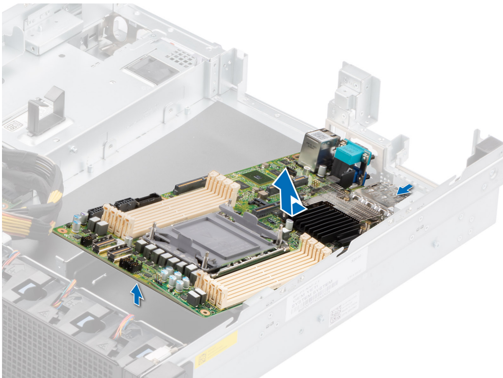
Abbildung 139. Entfernen der Hauptplatine
