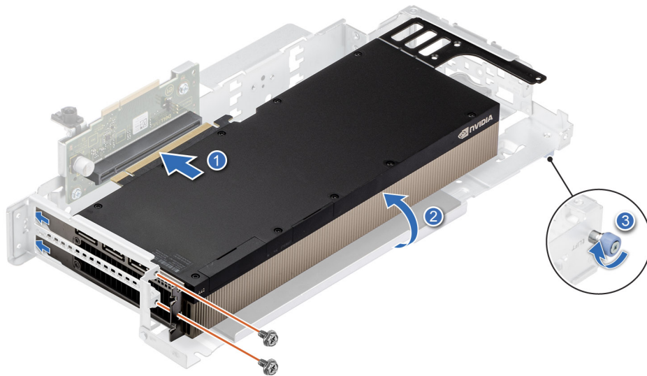
Abbildung 70. Installieren einer GPU-Karte mit doppelter Breite und voller Länge in Riser 2A
