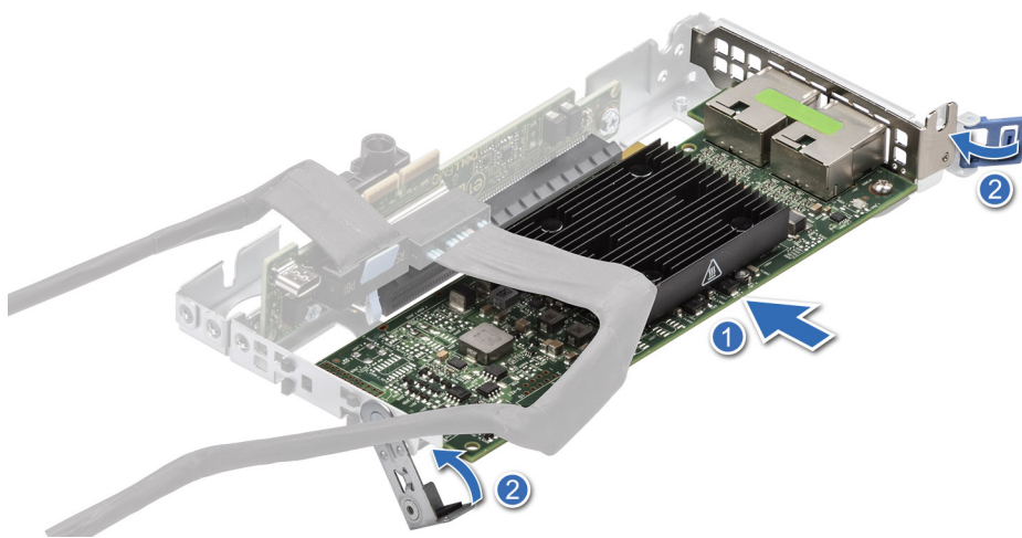
Abbildung 57. Einsetzen einer Erweiterungskarte mit voller Höhe in Riser 1A
