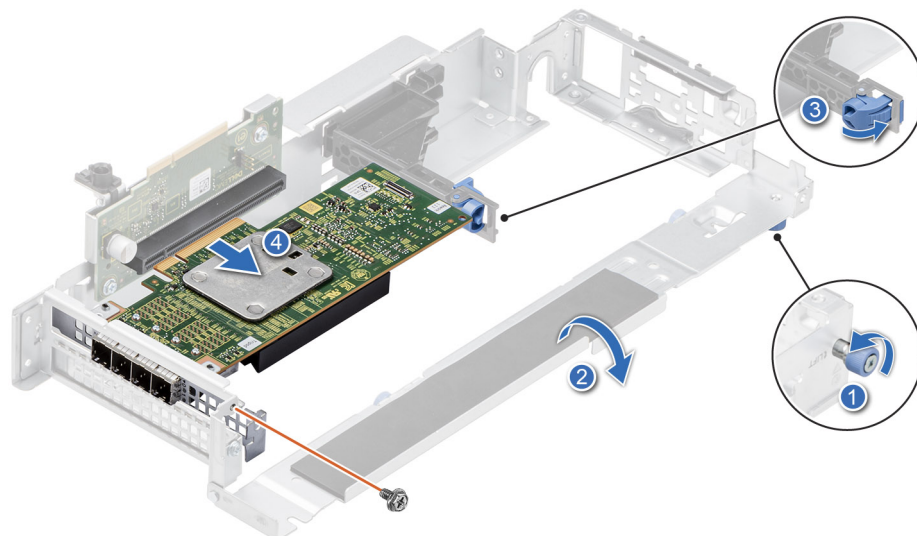
Abbildung 62. Entfernen einer Erweiterungskarte mit halber Länge und flachem Profil aus Riser 2A
