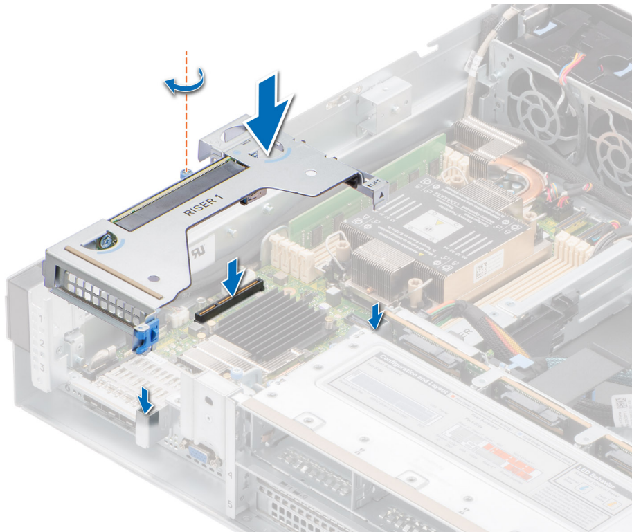
Abbildung 43. Installieren des Erweiterungskarten-Risers 1B
