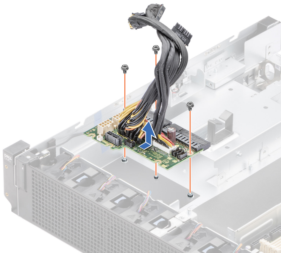
Abbildung 135. Stromzwischenplatine entfernen
