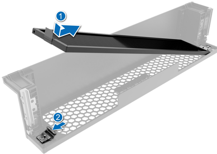
Abbildung 26. Installieren des Blendenfilters für die vorn zugängliche Konfiguration
