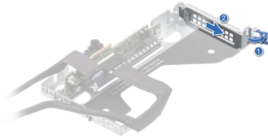
Abbildung 54. Entfernen eines Abdeckblechs aus Riser 1A
