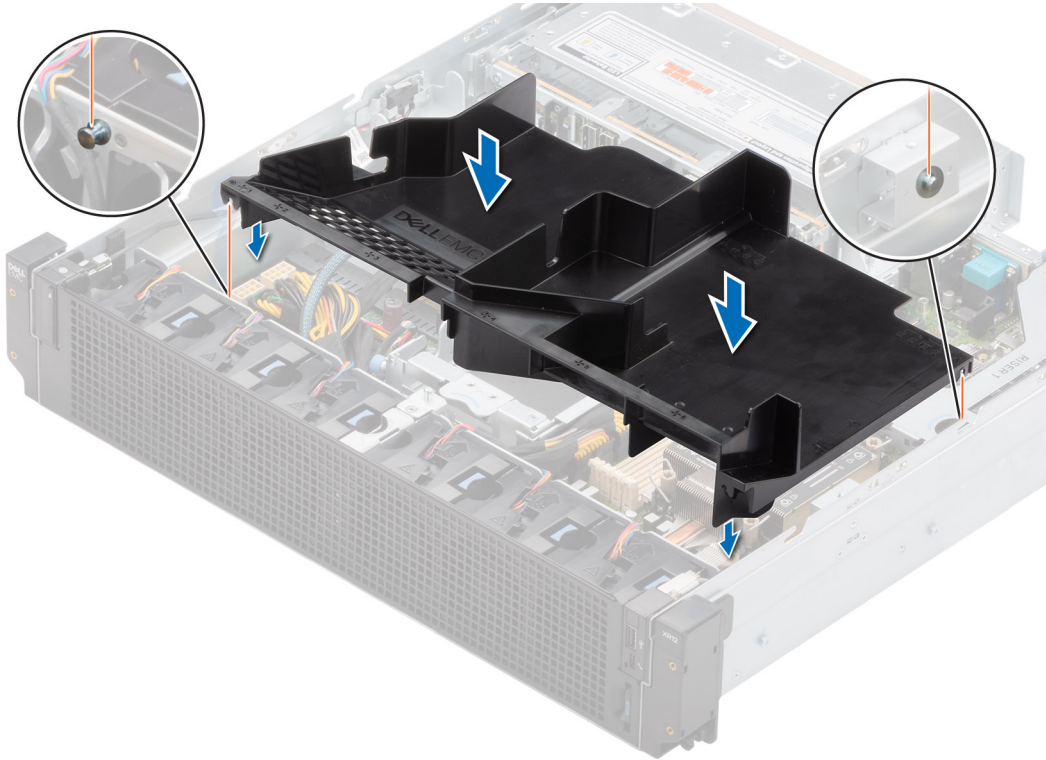
Abbildung 32. Luftstromverkleidung einbauen
