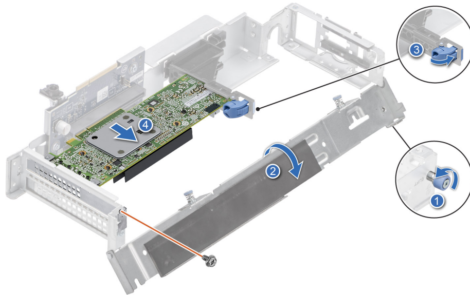
Abbildung 63. Entfernen einer Erweiterungskarte mit halber Länge und flachem Profil aus Riser 2B
