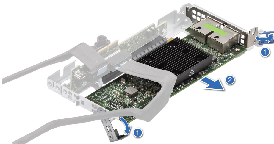
Abbildung 49. Entfernen einer Erweiterungskarte mit voller Höhe aus Riser 1A
