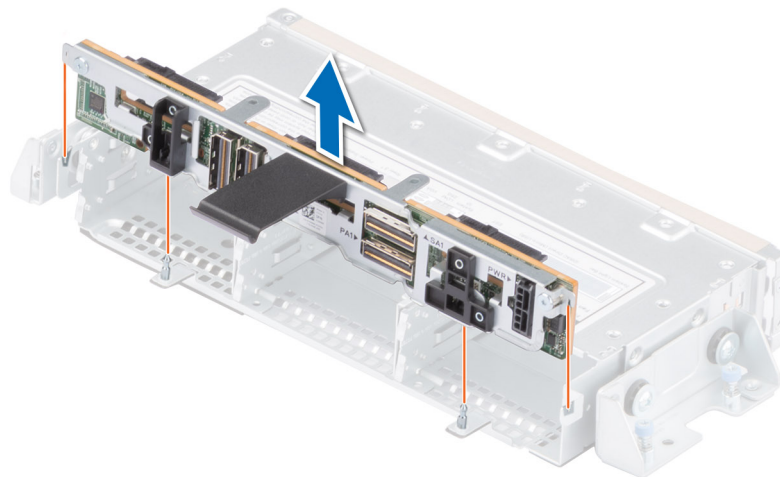
Abbildung 91. Laufwerkrückwandplatine entfernen
