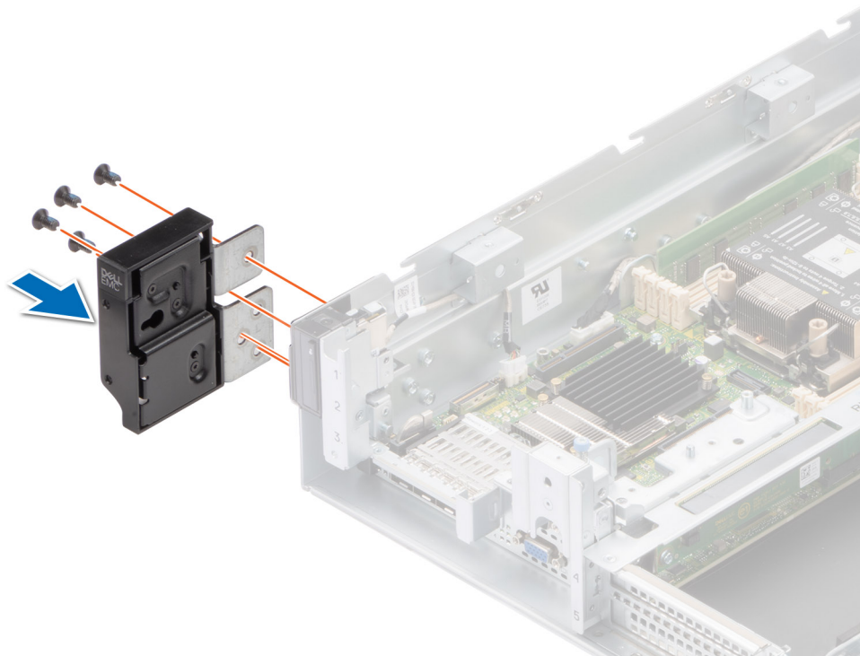
Abbildung 150. Installieren des linken Winkels für die vorn zugängliche Konfiguration
