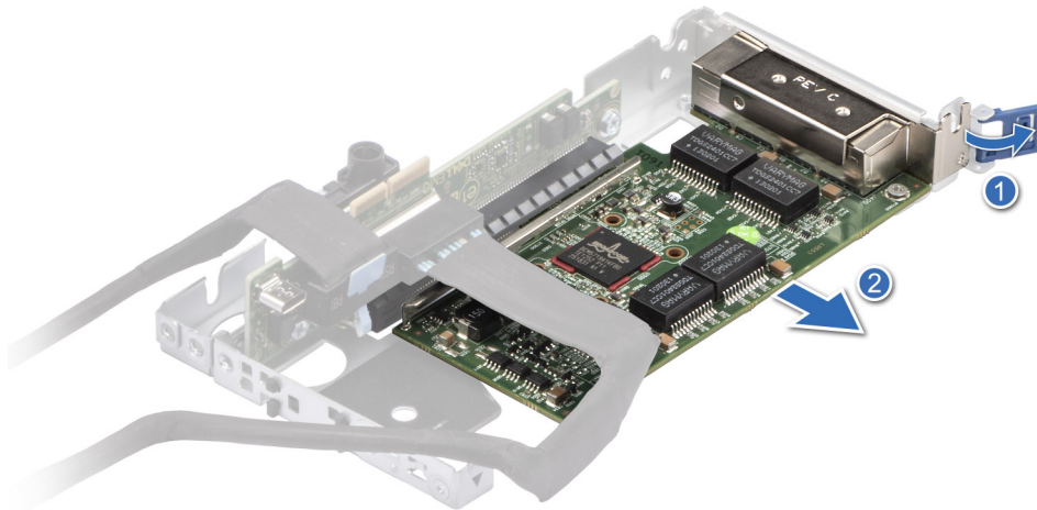
Abbildung 48. Entfernen einer Erweiterungskarte mit halber Länge aus Riser 1A
