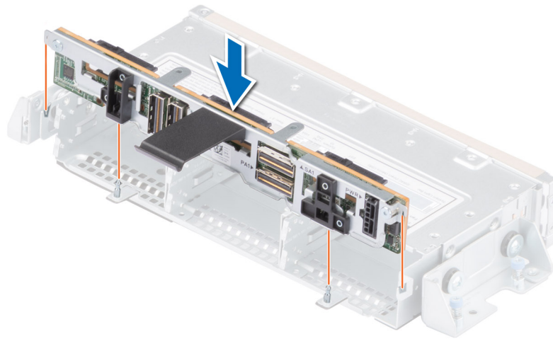
Abbildung 92. Laufwerkrückwandplatine installieren
