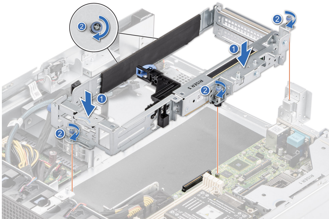
Abbildung 47. Installieren des Erweiterungskarten-Risers 3
