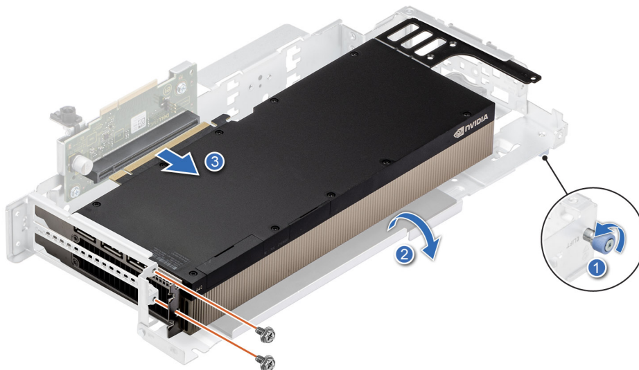
Abbildung 61. Entfernen einer GPU-Karte mit doppelter Breite und voller Länge aus Riser 2A
