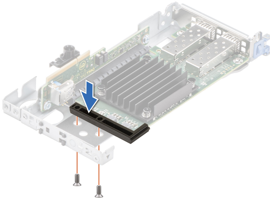
Abbildung 160. Installieren des Erweiterungskartenhalters auf Riser 1 für Erweiterungskarten halber Länge
