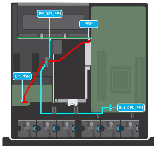
Abbildung 98. NVMe-Kabelanschluss mit 6 x 2,5-Zoll-Rückwandplatine
