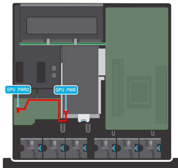
Abbildung 102. PIB zu Riser 3 mit GPU mit doppelter Breite und voller Baulänge
