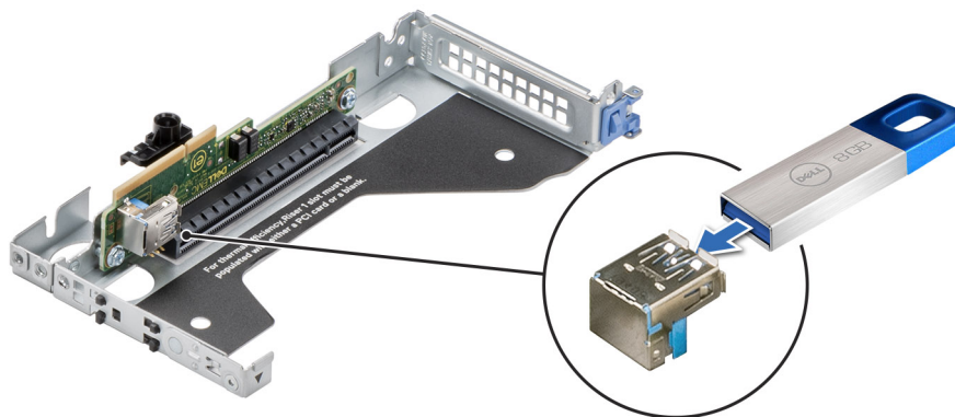
Abbildung 126. Installieren des internen USB-Speichersticks
