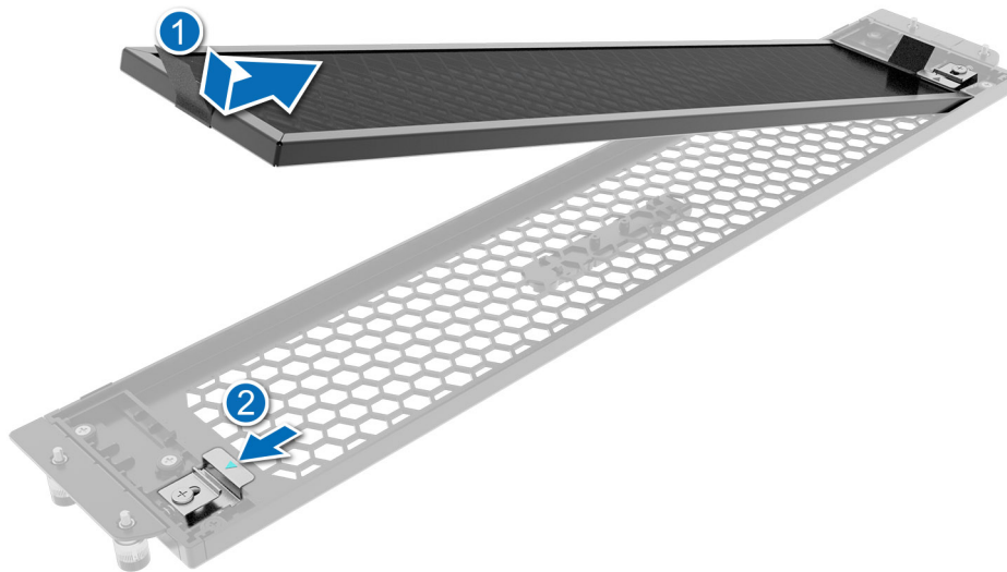
Abbildung 25. Installieren des Blendenfilters für die rückseitig zugängliche Konfiguration
