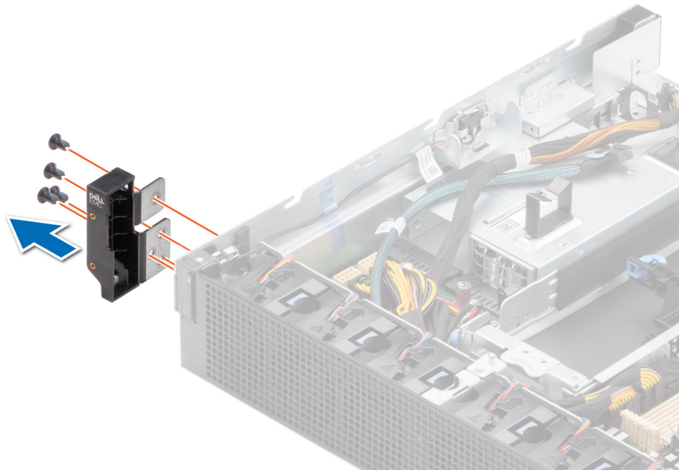
Abbildung 143. Entfernen des linken Winkels für die rückseitig zugängliche Konfiguration
