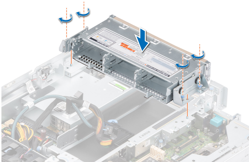
Abbildung 105. Einbauen des Laufwerksgehäuses
