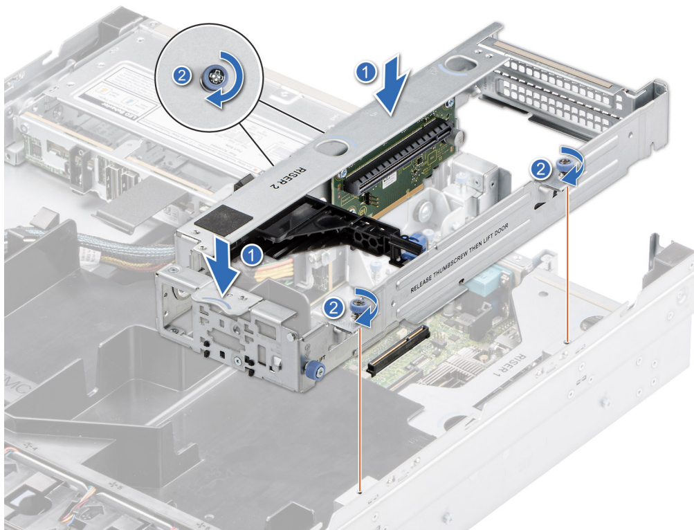
Abbildung 45. Installieren des Erweiterungskarten-Risers 2
