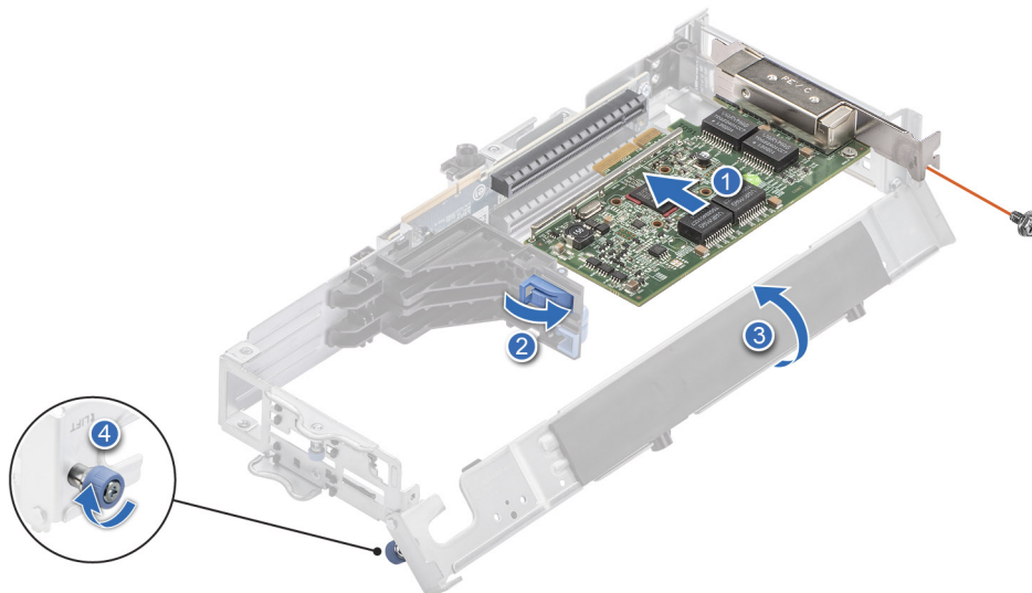
Abbildung 83. Installieren einer Erweiterungskarte mit halber Länge und flachem Profil in Riser 3B
