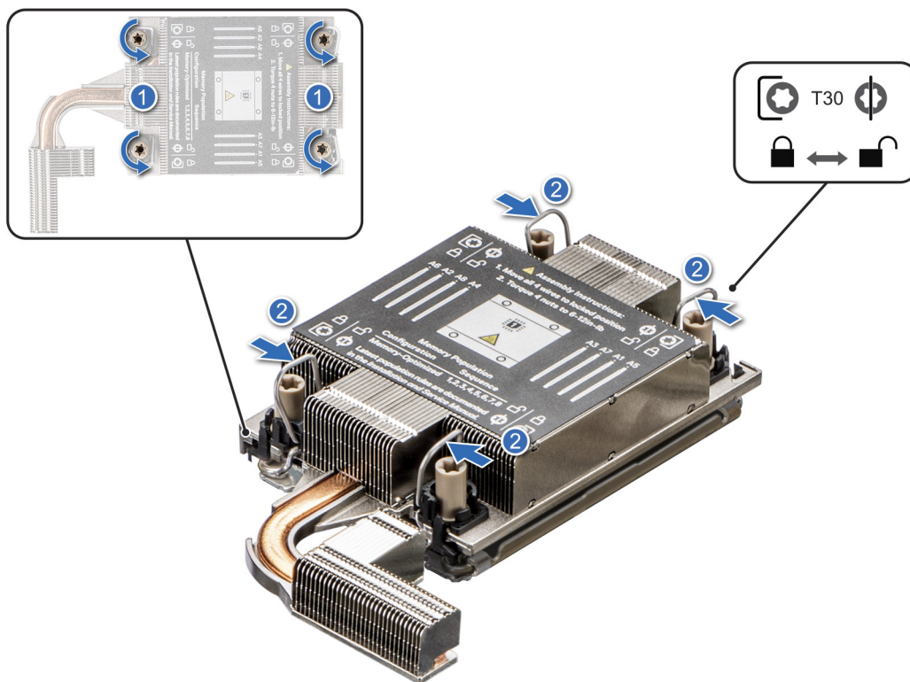
Abbildung 113. Lösen der Muttern und Einstellen der Kippdrähte in die entriegelte Position
