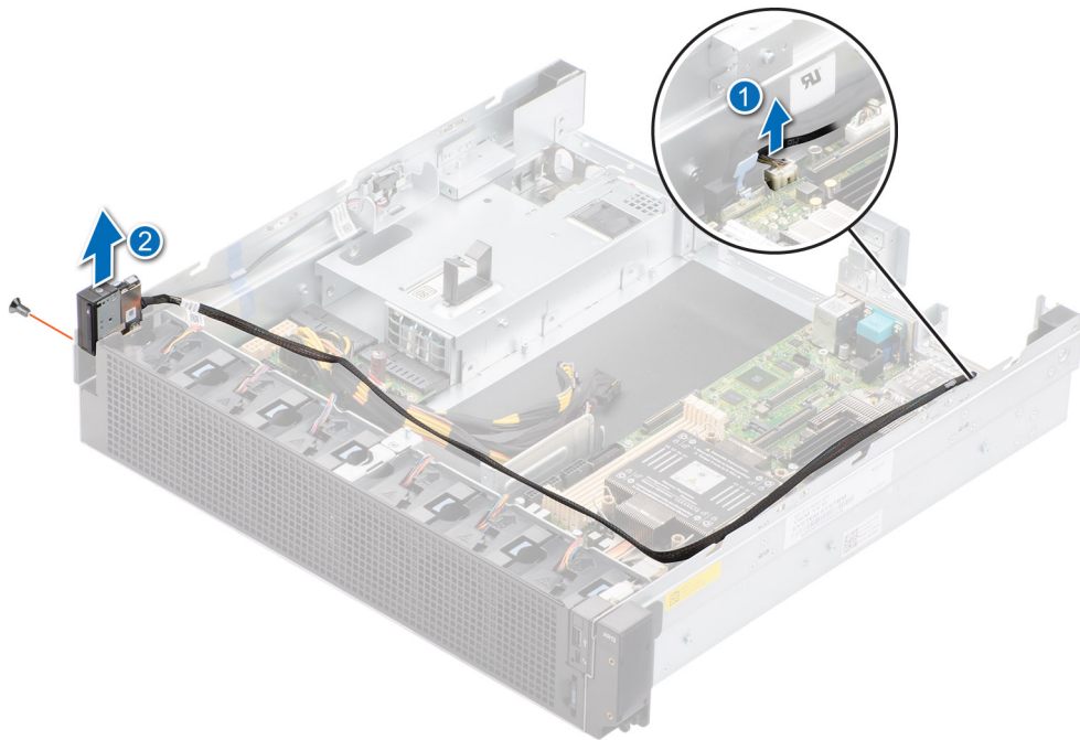
Abbildung 144. Entfernen des Status-LED-Bedienfelds für die rückseitig zugängliche Konfiguration
