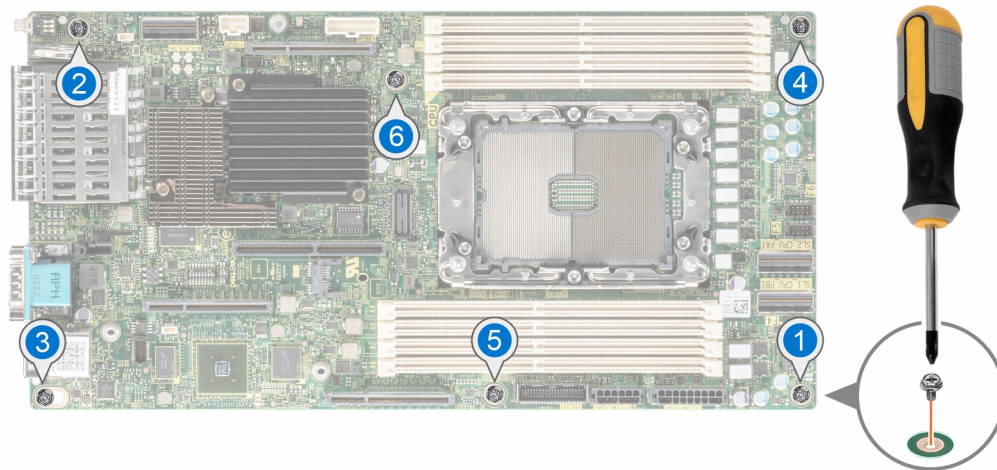
Abbildung 141. Anziehen der Schrauben der Systemplatine nacheinander
