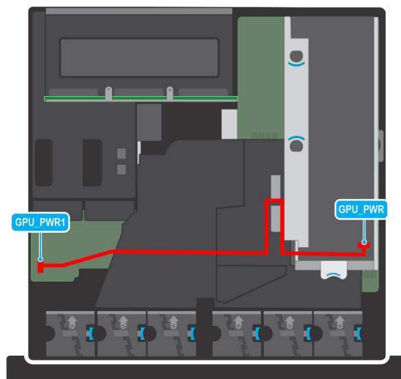
Abbildung 100. PIB zu Riser 2 mit GPU mit einfacher Breite und voller Baulänge
