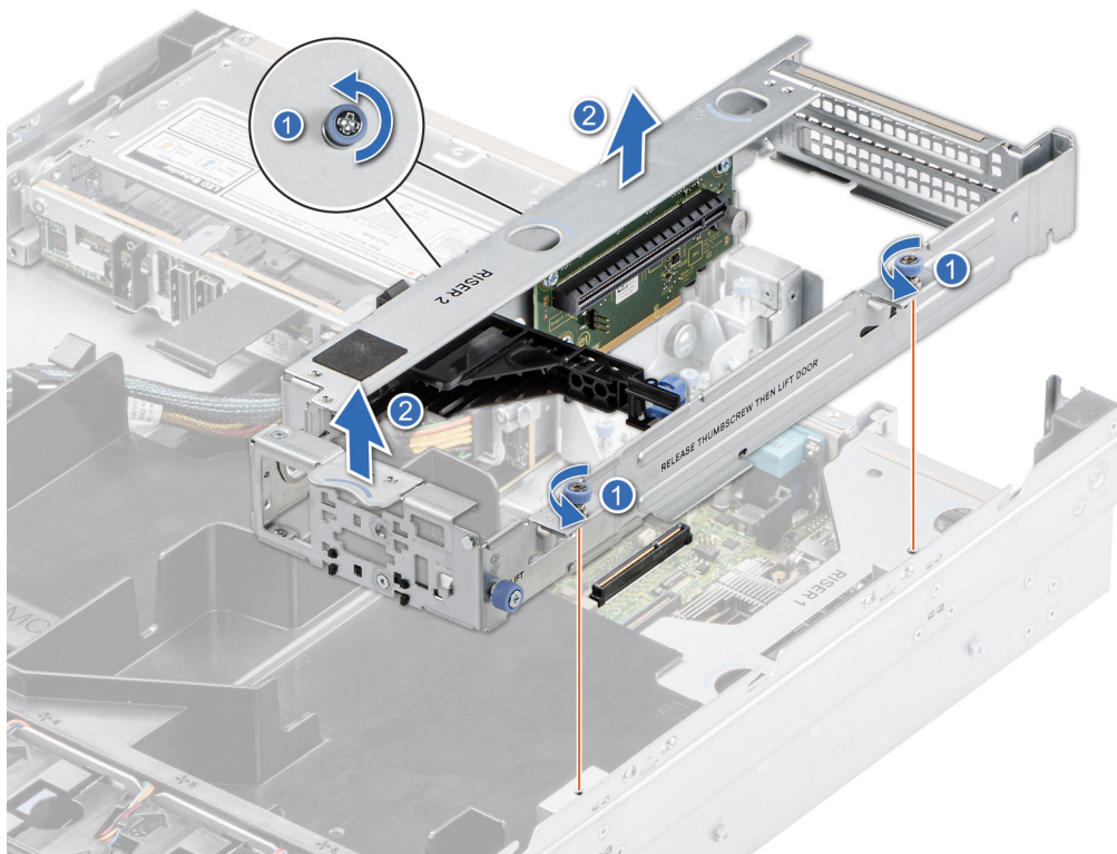
Abbildung 44. Entfernen des Erweiterungskarten-Risers 2
