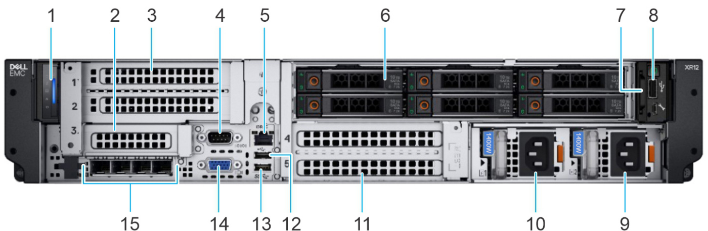
Abbildung 2. Vorderansicht der vorn zugänglichen 6 x 2,5-Zoll-Laufwerkskonfiguration
