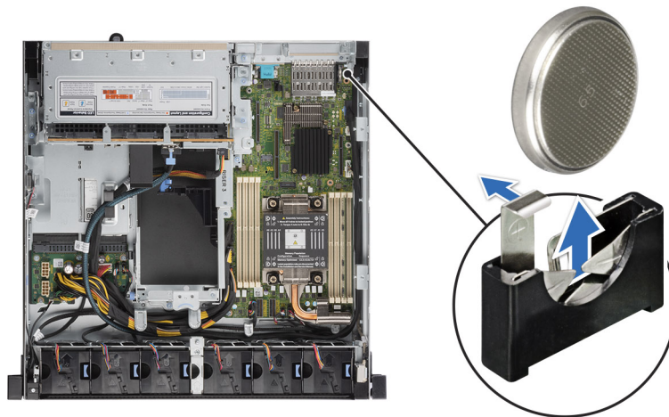
Abbildung 137. Entfernen der Systembatterie
