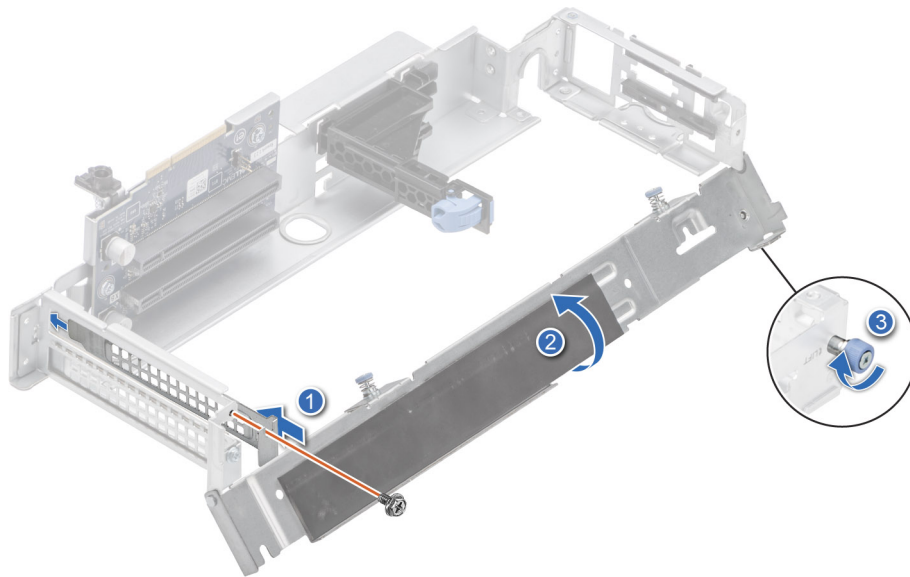
Abbildung 65. Einsetzen des Abdeckblechs in Riser 2B
