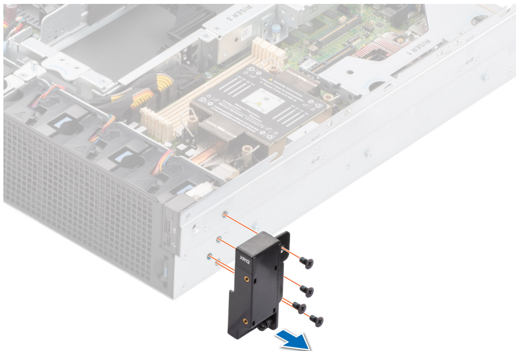
Abbildung 151. Entfernen des rechten Winkels für die rückseitig zugängliche Konfiguration
