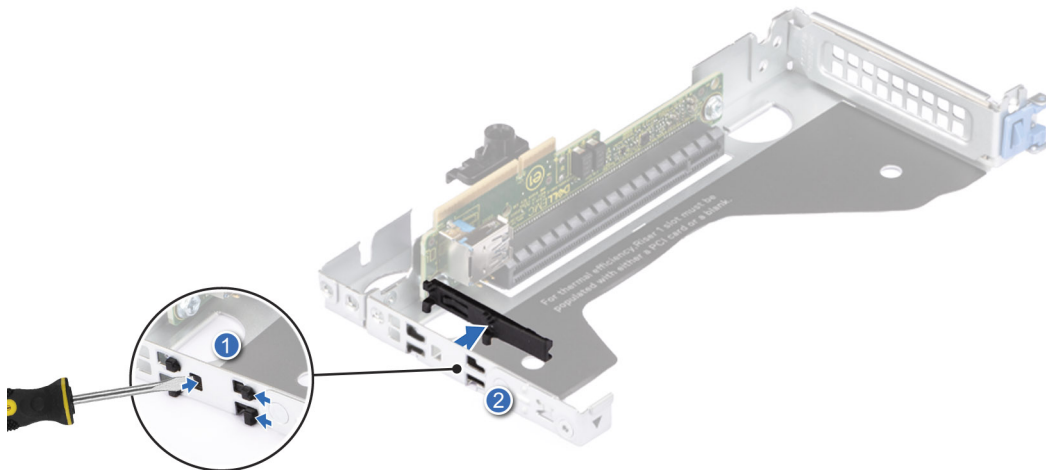
Abbildung 161. Entfernen des Erweiterungskartenhalters aus dem Riser 1
