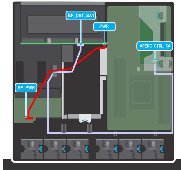
Abbildung 95. PERC SA SAS-Kabel mit 6 x 2,5-Zoll-Rückwandplatine
