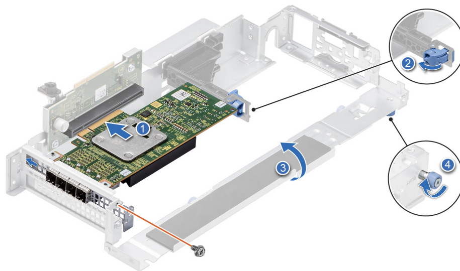
Abbildung 71. Installieren einer Erweiterungskarte mit halber Länge und flachem Profil in Riser 2A
