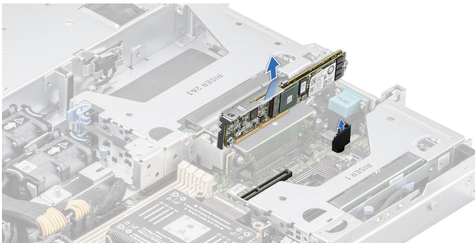
Abbildung 127. Entfernen der M.2-BOSS-Karte von der Systemplatine
