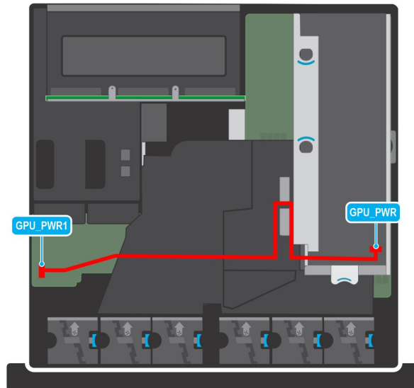
Abbildung 101. PIB zu Riser 2 mit GPU mit doppelter Breite und voller Baulänge
