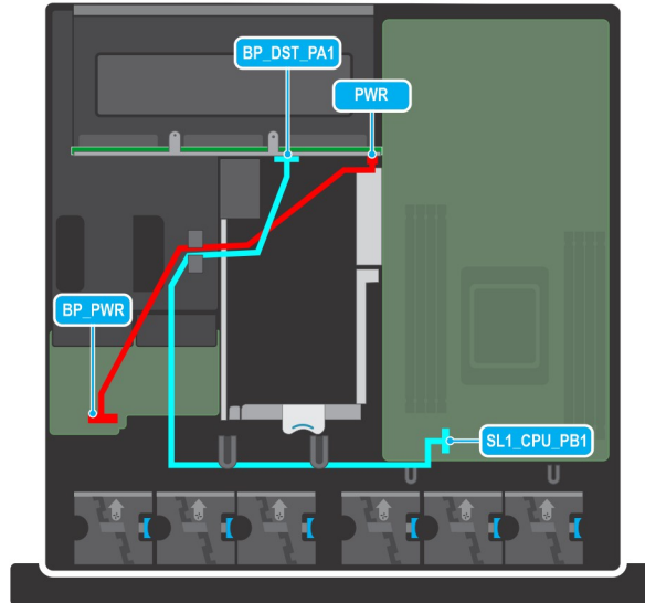
Abbildung 97. NVMe-Kabelanschluss mit 6 x 2,5-Zoll-Rückwandplatine
