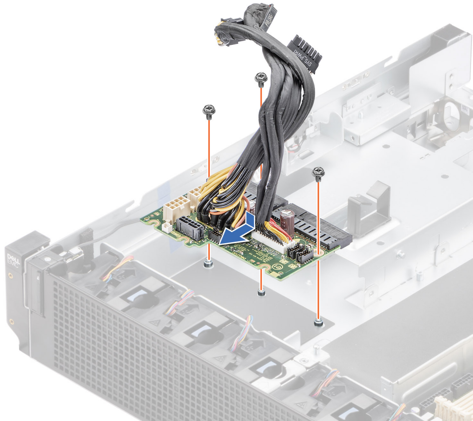
Abbildung 136. Installieren der Stromzwischenplatine
