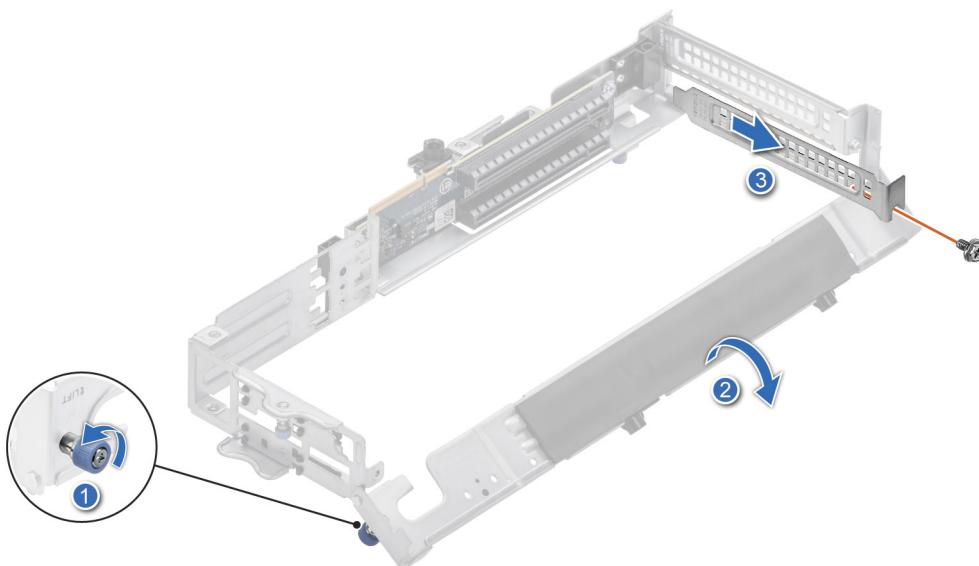
Abbildung 79. Entfernen eines Abdeckblechs aus Riser 3B
