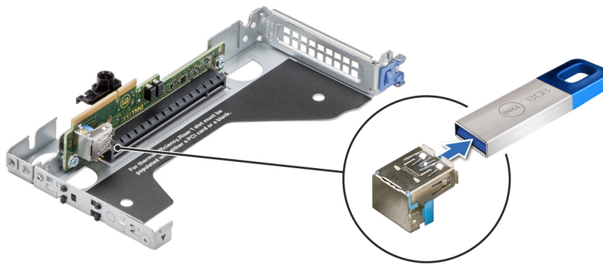
Abbildung 125. Entfernen des internen USB-Speichersticks
