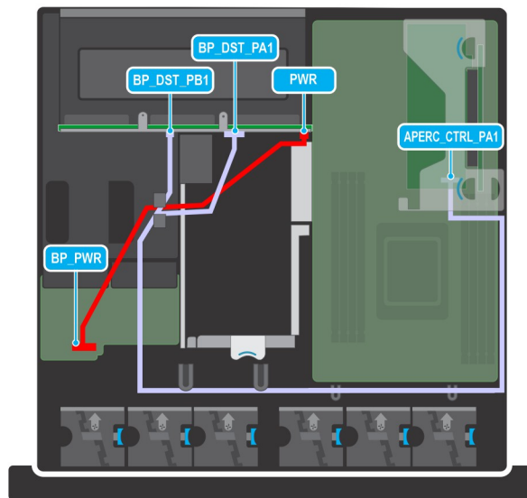
Abbildung 93. PERC PA NVMe-Kabel mit 6 x 2,5-Zoll-Rückwandplatine
