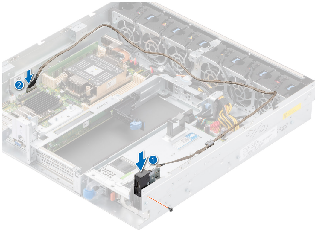
Abbildung 157. Installieren des Netzschalter-Bedienfelds für die vorn zugängliche Konfiguration
