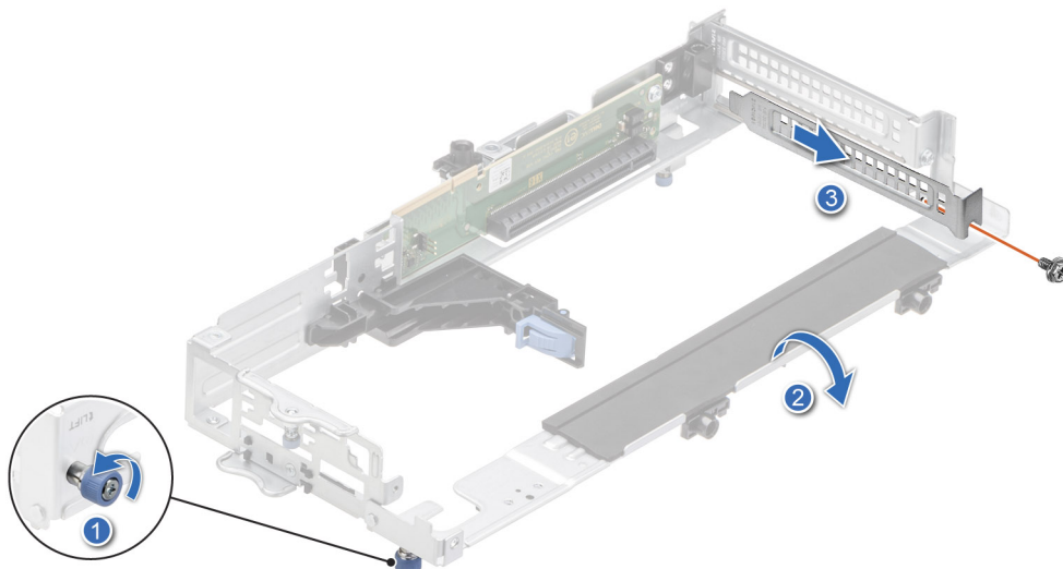
Abbildung 78. Entfernen eines Abdeckblechs aus Riser 3A
