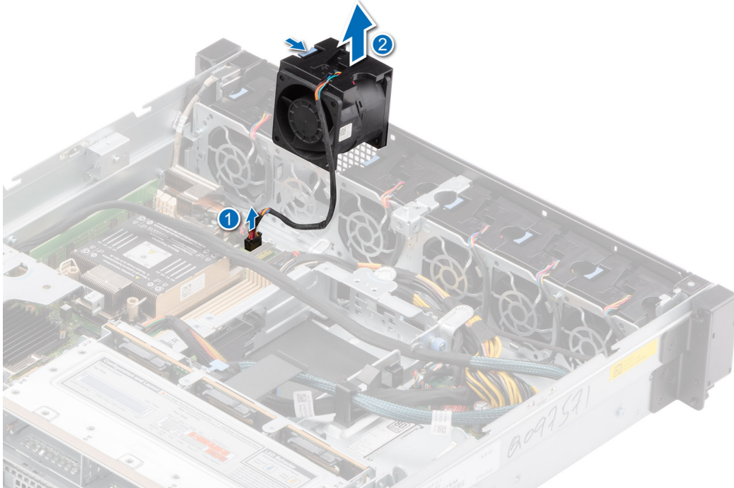
Abbildung 106. Entfernen eines Kühlungslüfters
