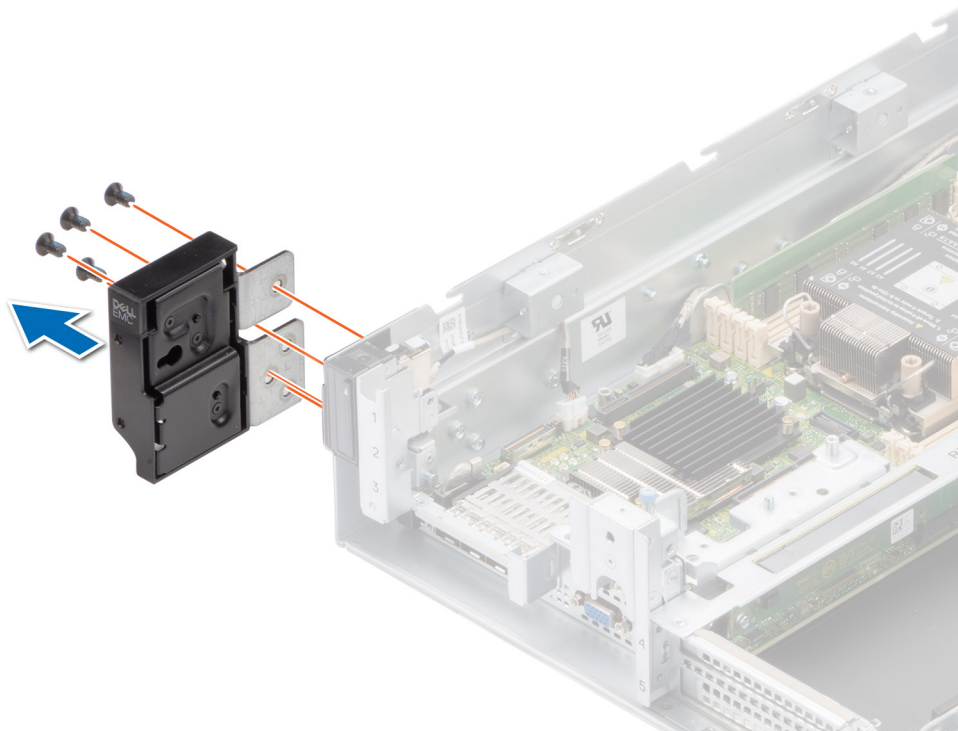
Abbildung 145. Entfernen des linken Winkels für die vorn zugängliche Konfiguration
