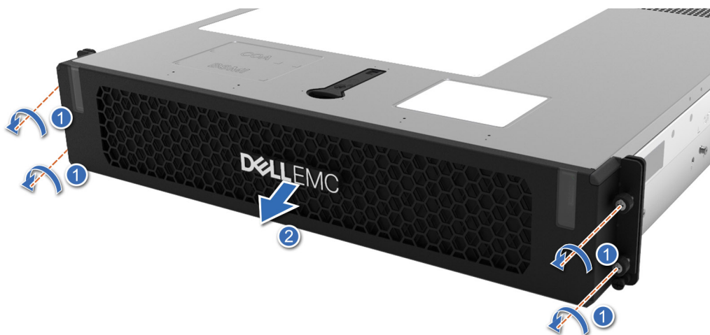
Abbildung 19. Entfernen der Frontblende für die rückseitig zugängliche Konfiguration
