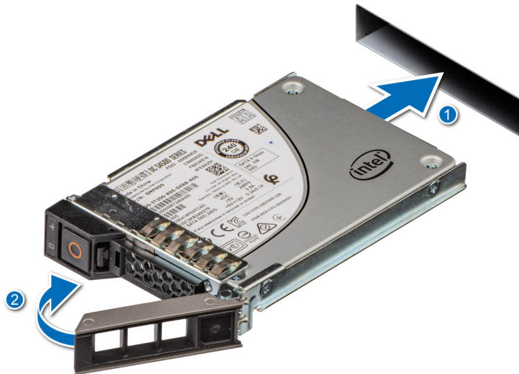
Abbildung 87. Installieren eines Laufwerksträgers
