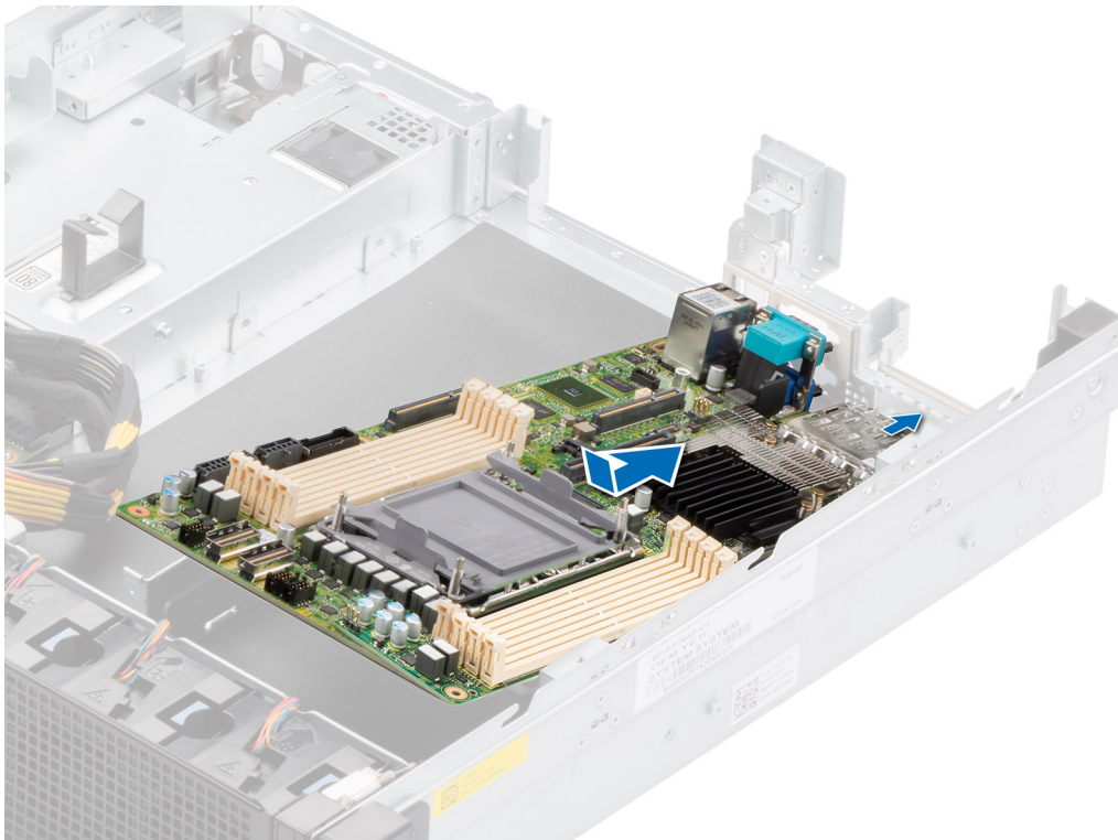
Abbildung 140. Installieren der Hauptplatine
