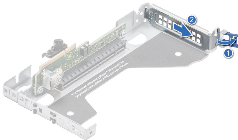
Abbildung 55. Entfernen eines Abdeckblechs aus Riser 1B
