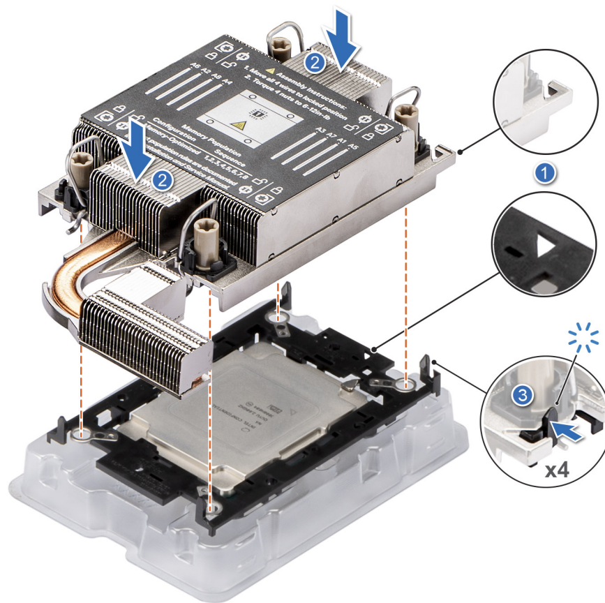
Abbildung 122. Setzen des Kühlkörpers auf den Prozessor ein
