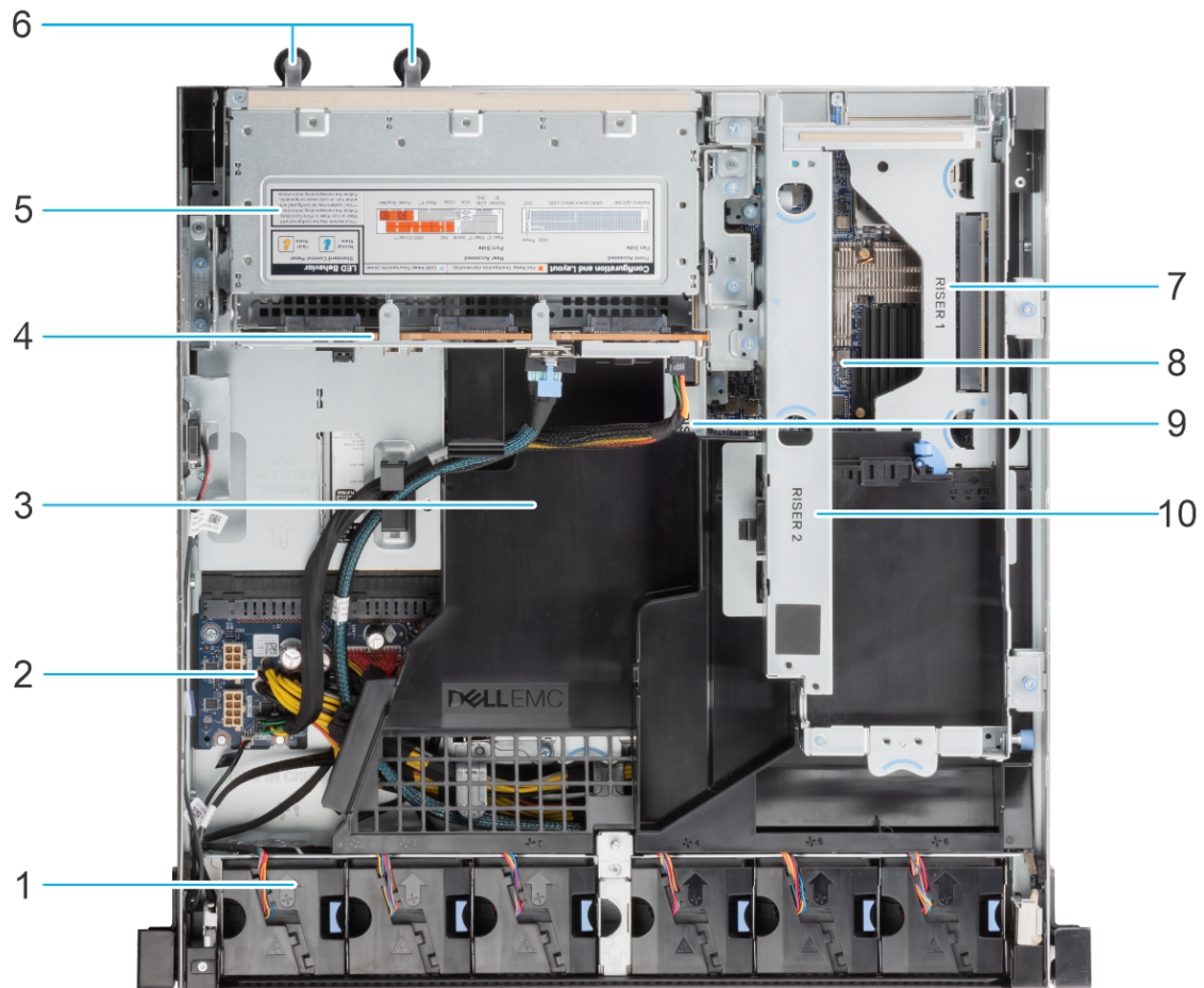
Abbildung 7. Das Systeminnere – Rückseitig zugängliche Konfiguration
