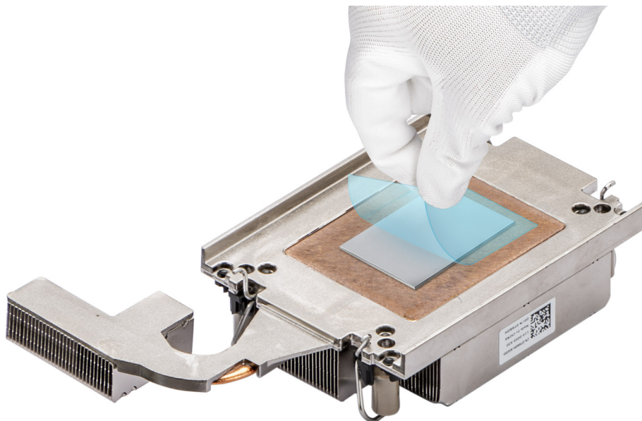
Abbildung 121. Entfernen Sie die Schutzfolie der Wärmeleitfolie (TIM)
