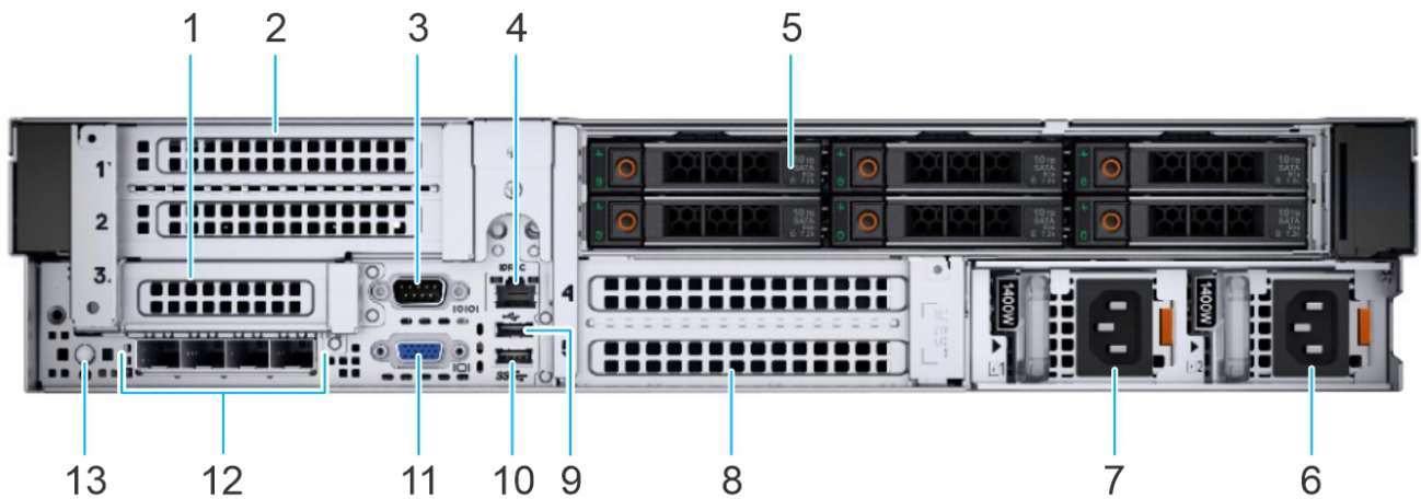
Abbildung 3. Rückansicht der rückseitig zugänglichen 6 x 2,5-Zoll-Laufwerkskonfiguration
