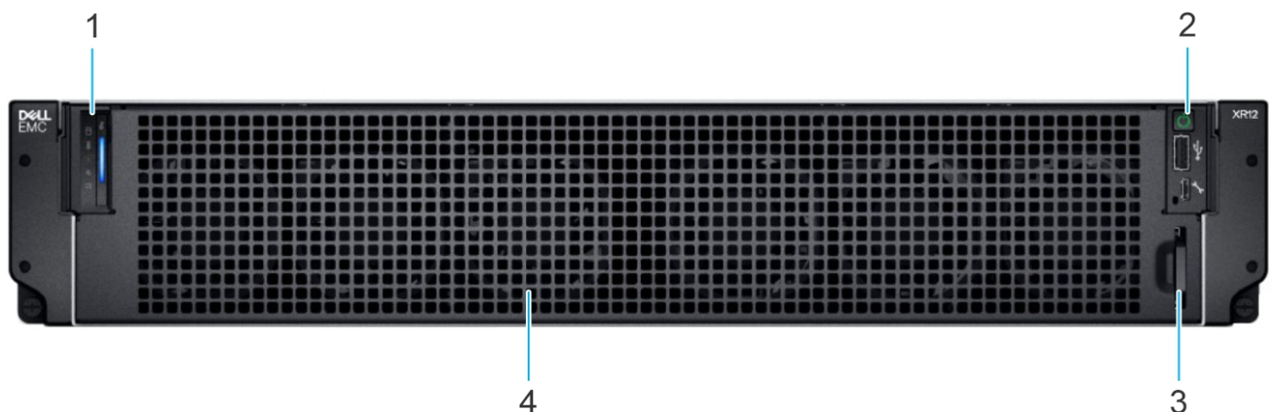
Abbildung 1. Vorderansicht der rückseitig zugänglichen 6 x 2,5-Zoll-Laufwerkskonfiguration
