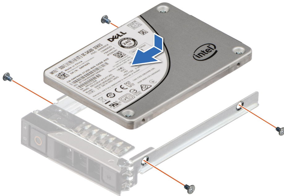
Abbildung 89. Einsetzen eines Laufwerks in den Laufwerksträger
