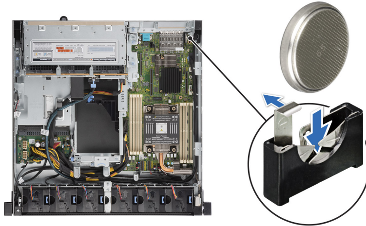
Abbildung 138. Installieren der Systembatterie
