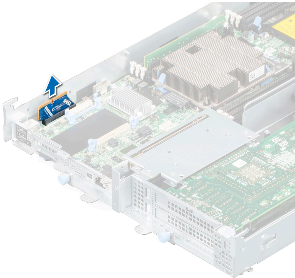
Figure 38. Retrait de la carte de montage mini PERC
