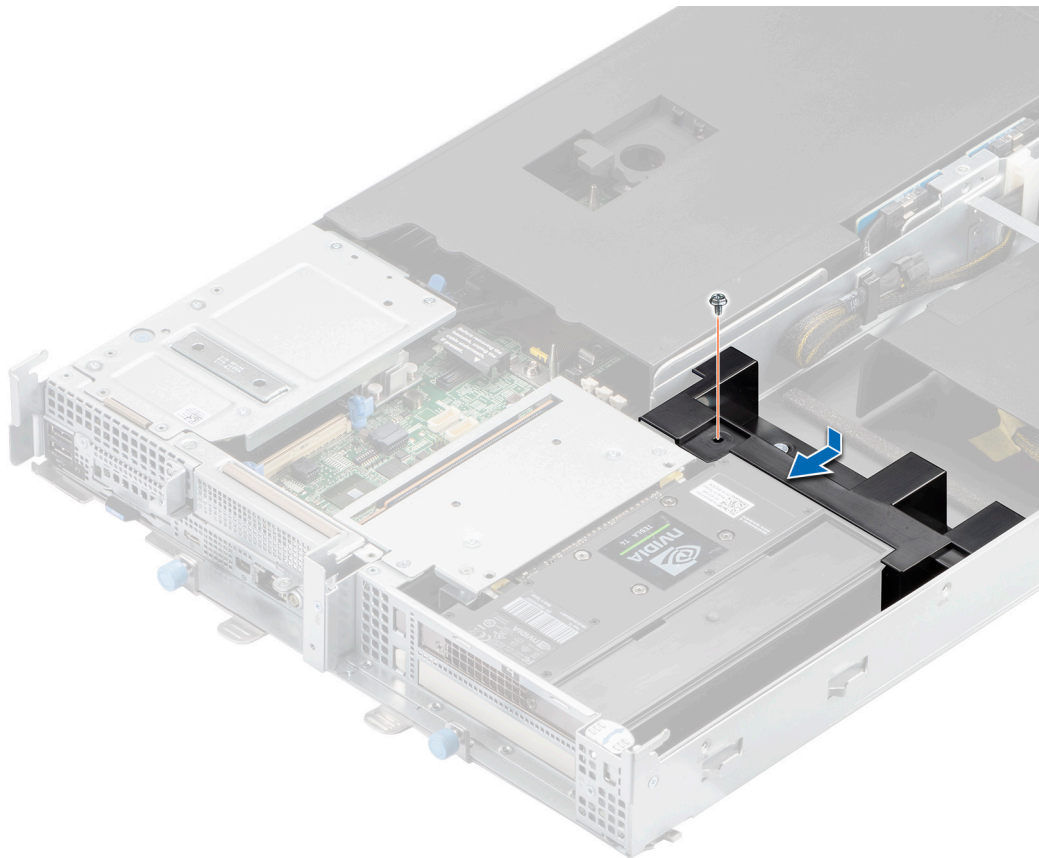
Figure 78. Installation du déflecteur d'air
