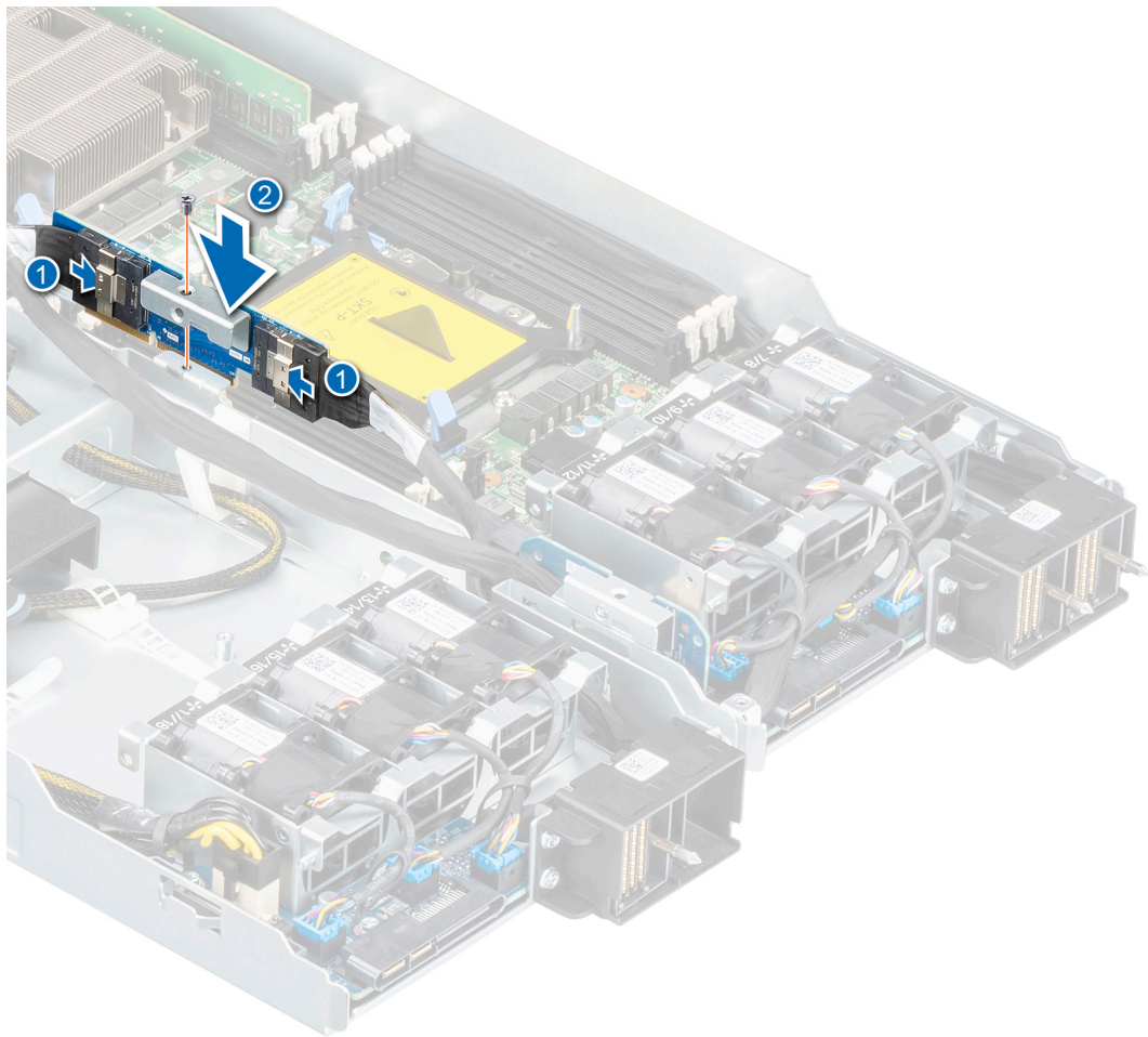
Figure 31. Installation de la carte de montage M.2
