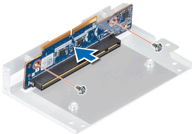
Figure 84. Installation de la carte de montage hauteur standard
