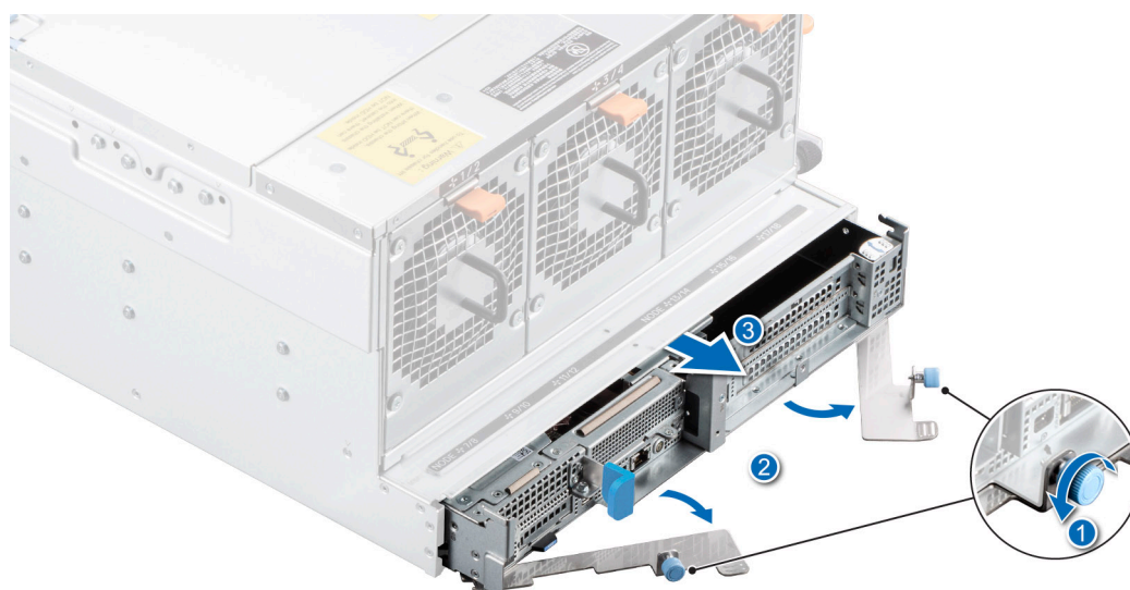
Figure 16. Retrait du traineau
