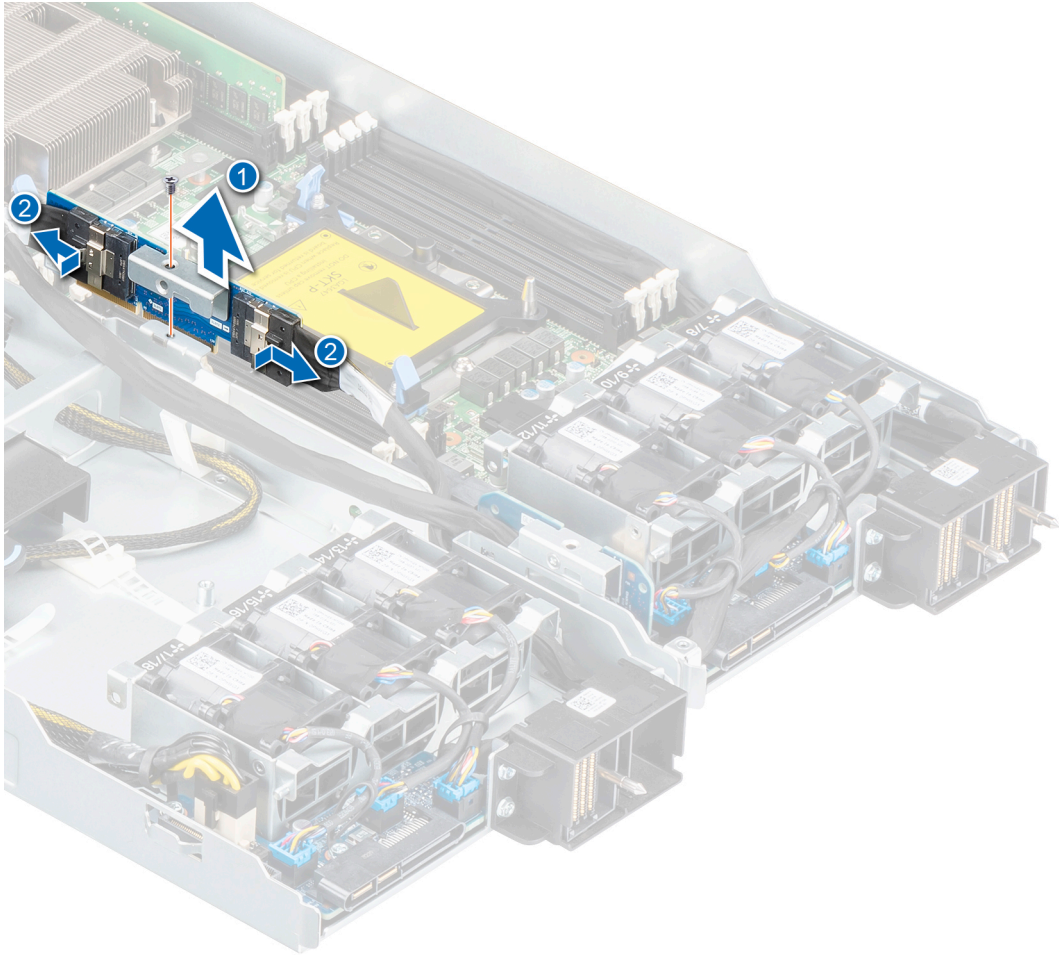
Figure 28. Retrait de la carte de montage M.2
