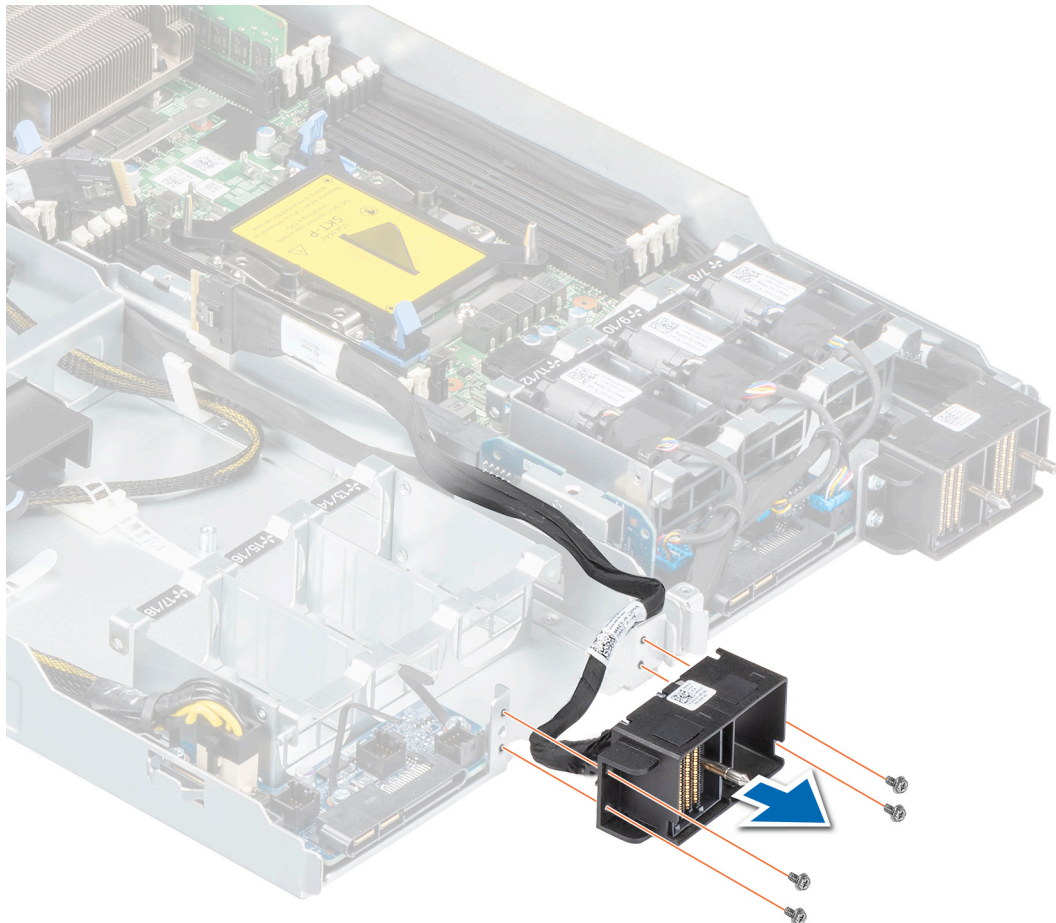
Figure 50. Retrait du kit de câbles pour traîneau (2)
