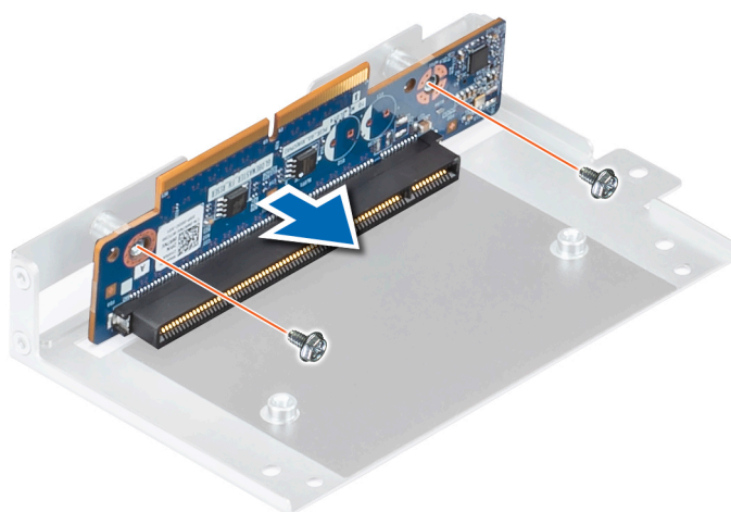
Figure 83. Retrait de la carte de montage hauteur standard
