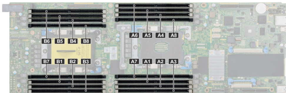
Figure 106. Emplacement des sockets de mémoire
