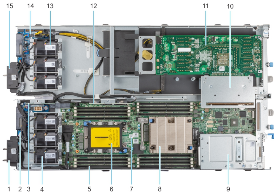
Figure 3. Traîneau PowerEdge XE7440 (pleine largeur, hauteur standard)
