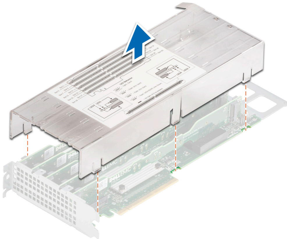
Figure 60. Retrait du conduit d'air FE1
