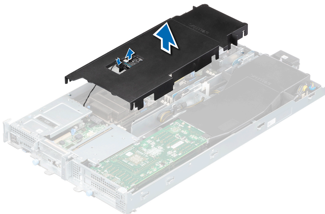
Figure 18. Retrait du carénage d'aération
