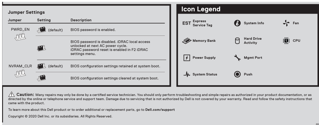
Figure 12. Réglages des cavaliers
