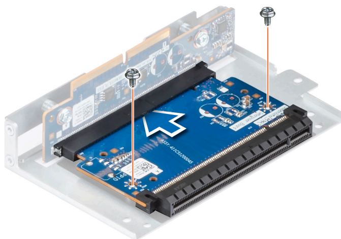
Figure 81. Installation de la carte intercalaire hauteur standard, pleine longueur
