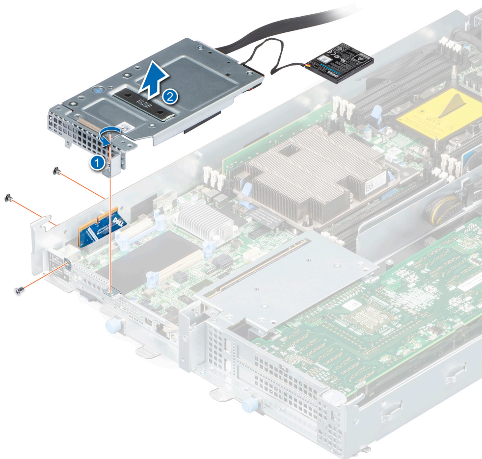
Figure 32. Retrait du module de carte mini PERC
