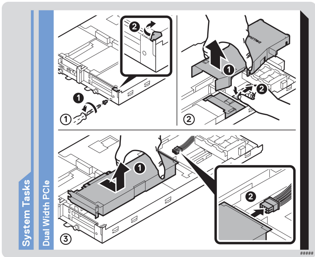
Figure 10. Tâches système sur la configuration pleine largeur, hauteur standard
