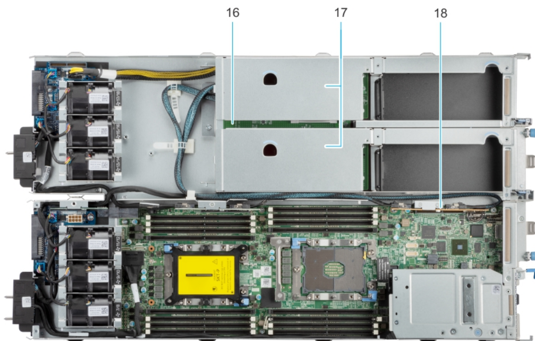
Figure 4. Traîneau PowerEdge XE7440 (pleine largeur, demi-hauteur)
