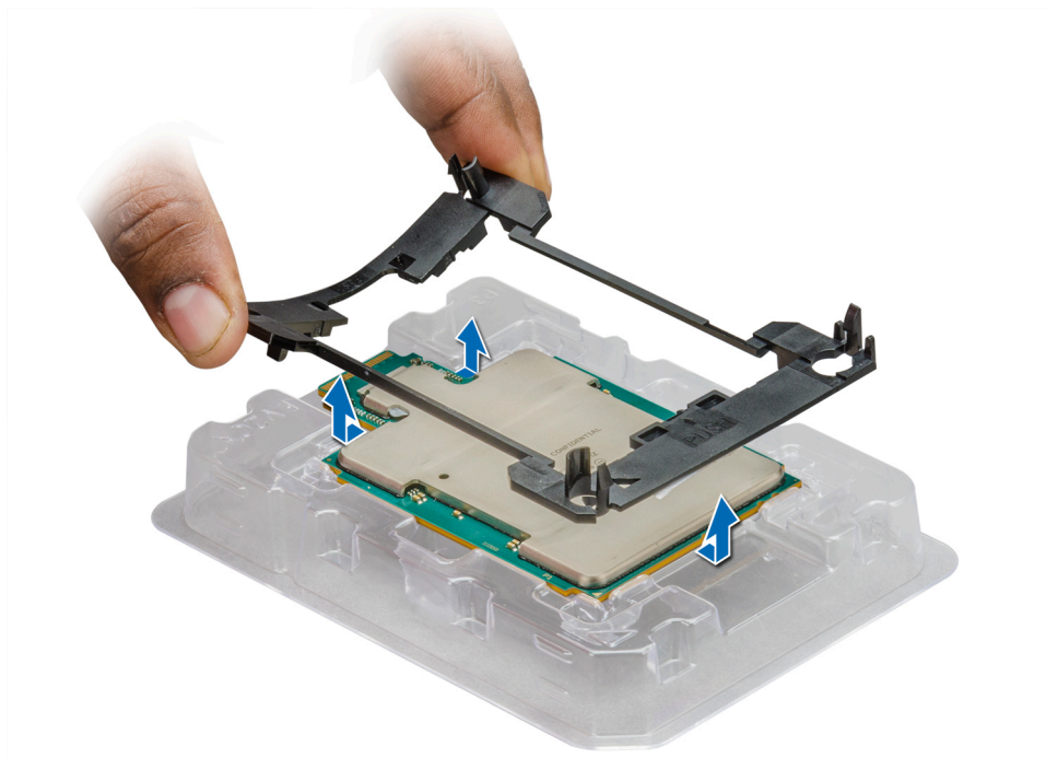
Figure 102. Retrait du support de processeur
