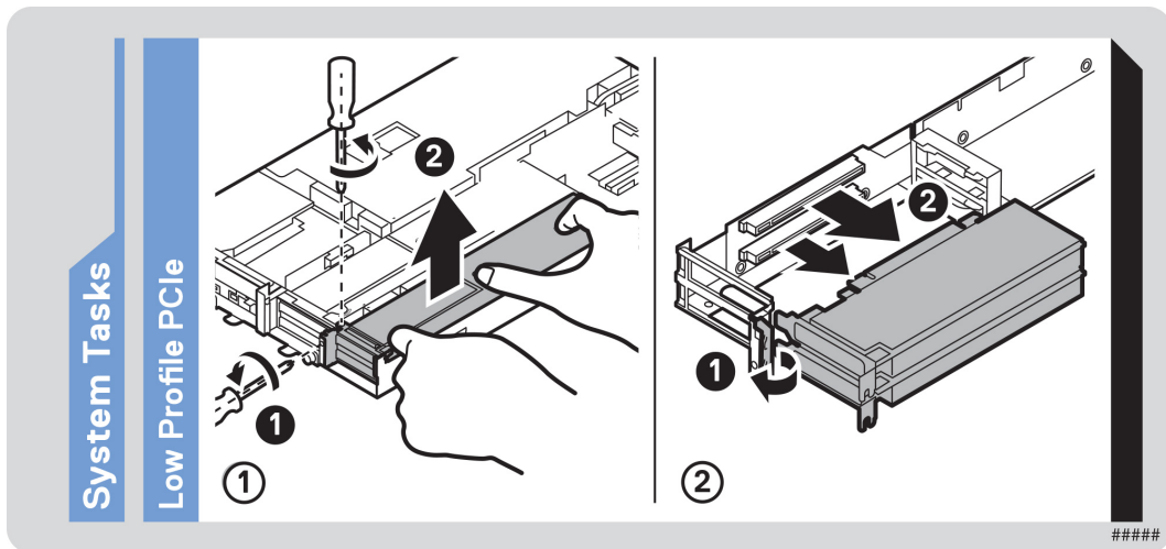
Figure 11. Tâches système sur la configuration pleine largeur, demi-hauteur
