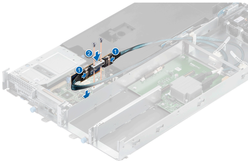
Figure 94. Installation de la carte de montage principale pour câble
