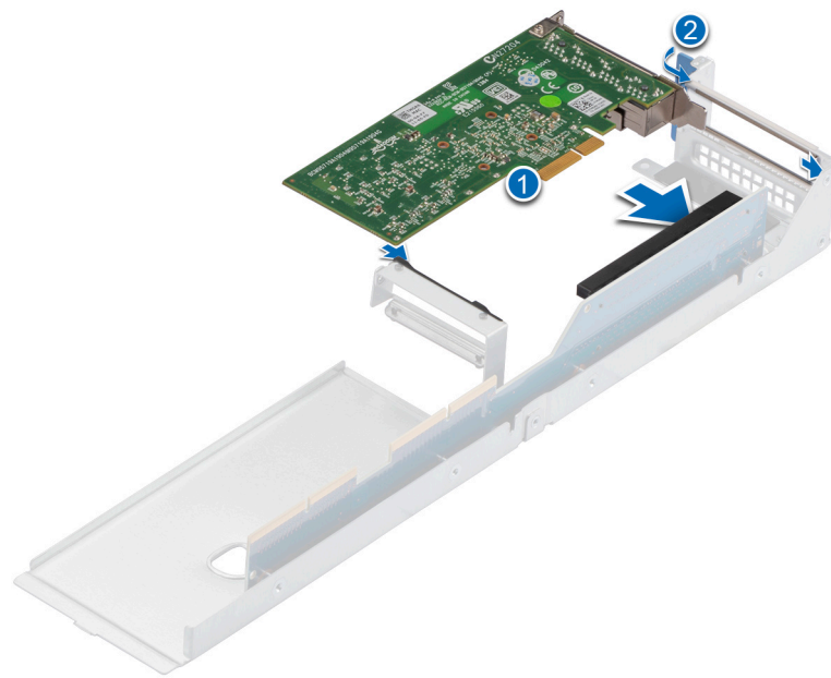
Figure 87. Installation de la carte PCIe demi-hauteur
