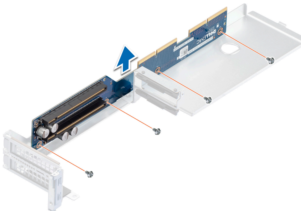
Figure 89. Retrait de la carte de montage
