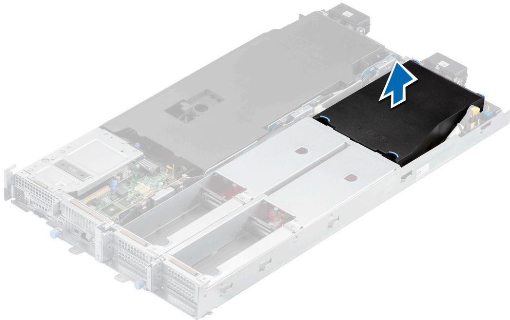
Figure 20. Retrait du carénage à air (configuration pleine largeur, demi-hauteur)
