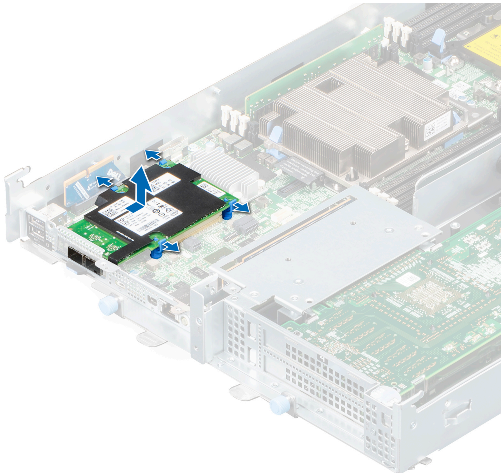
Figure 42. Retrait de la carte OCP
