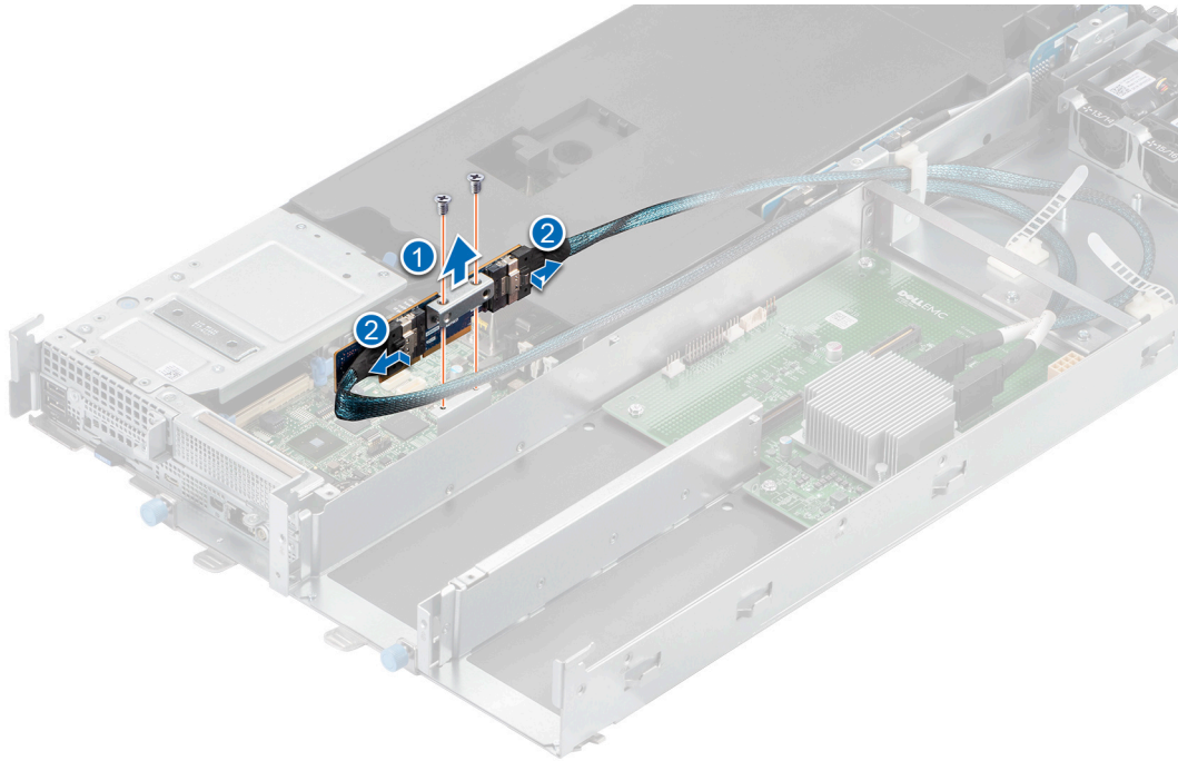
Figure 91. Retrait de la carte de montage principale pour câble
