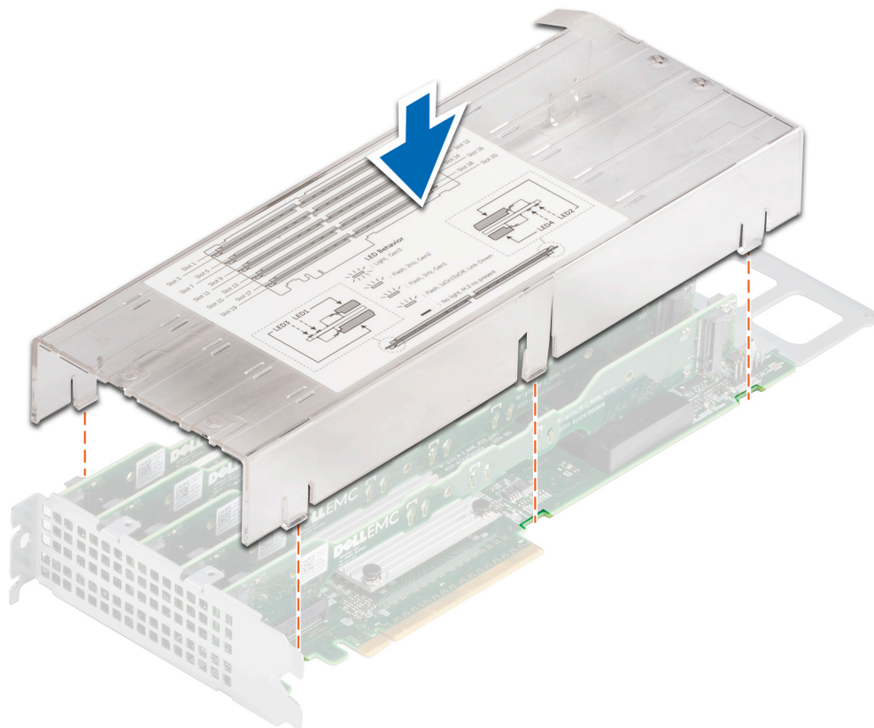
Figure 61. Installation du conduit d'air FE1
