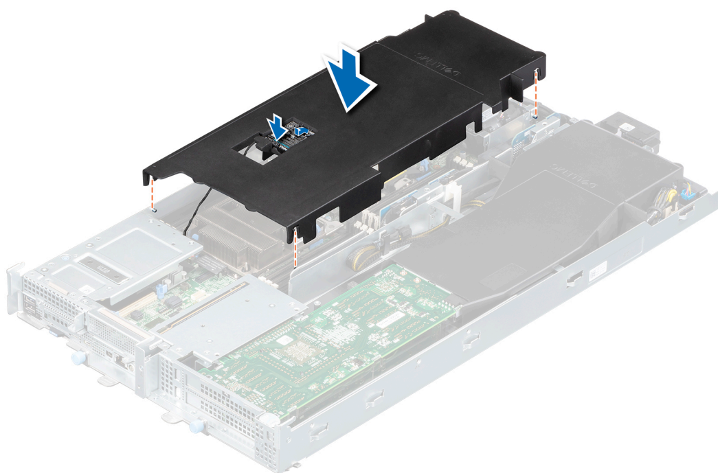
Figure 21. Installation du carénage d'aération
