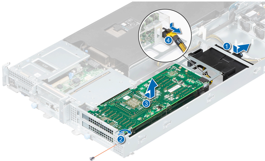
Figure 58. Retrait de la carte FE1
