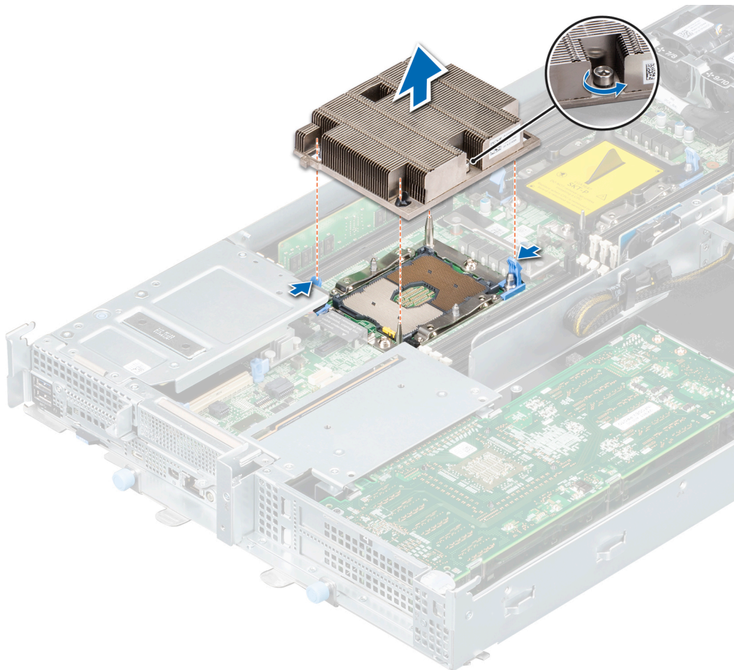
Figure 97. Retrait du module du processeur et du dissipateur de chaleur
