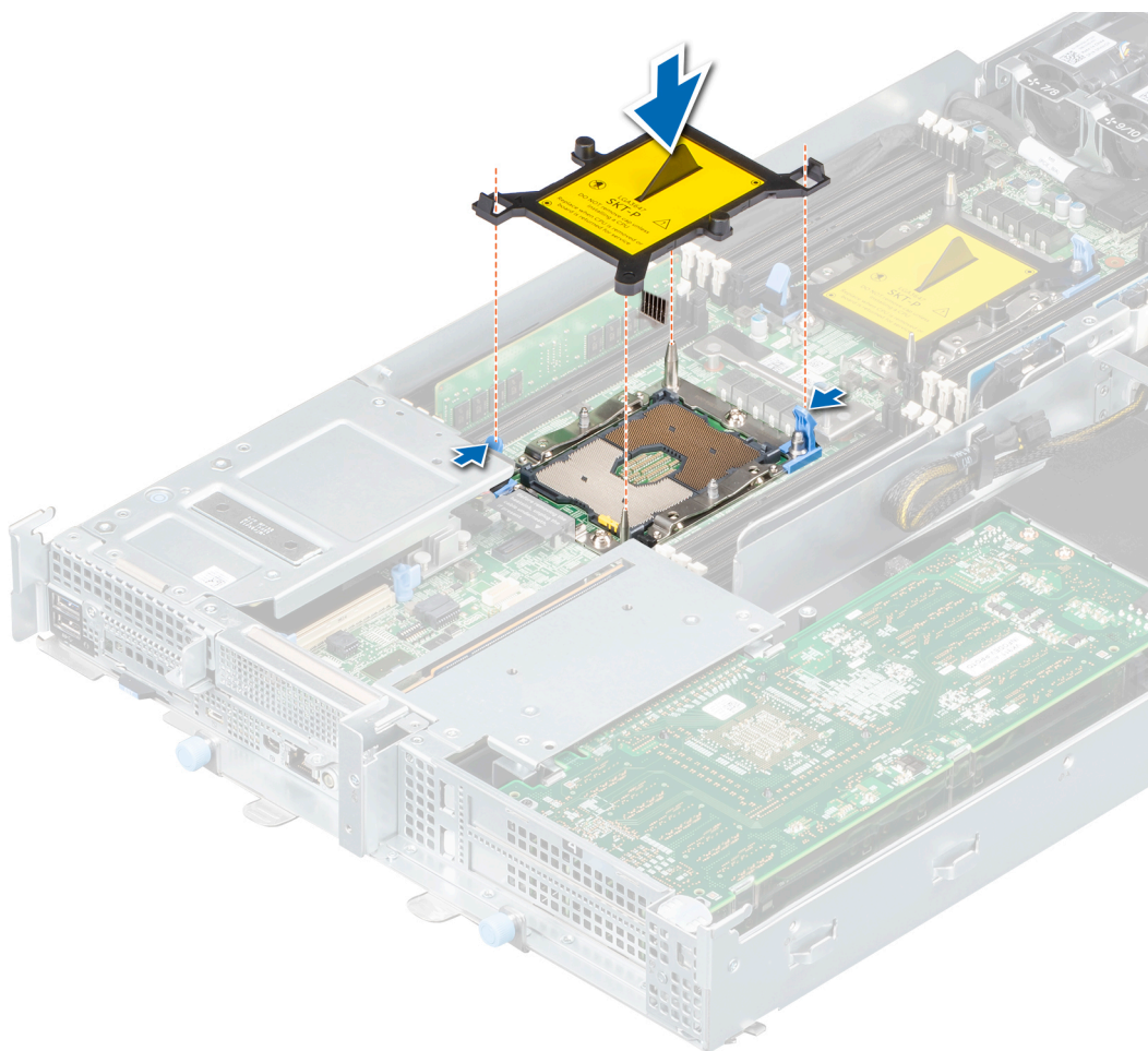
Figure 98. Insertion du cache anti-poussière du processeur
