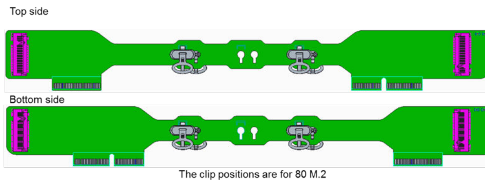
Figure 66. Positions des clips sur la carte de montage pour le format M.2 22 mm x 80 mm
