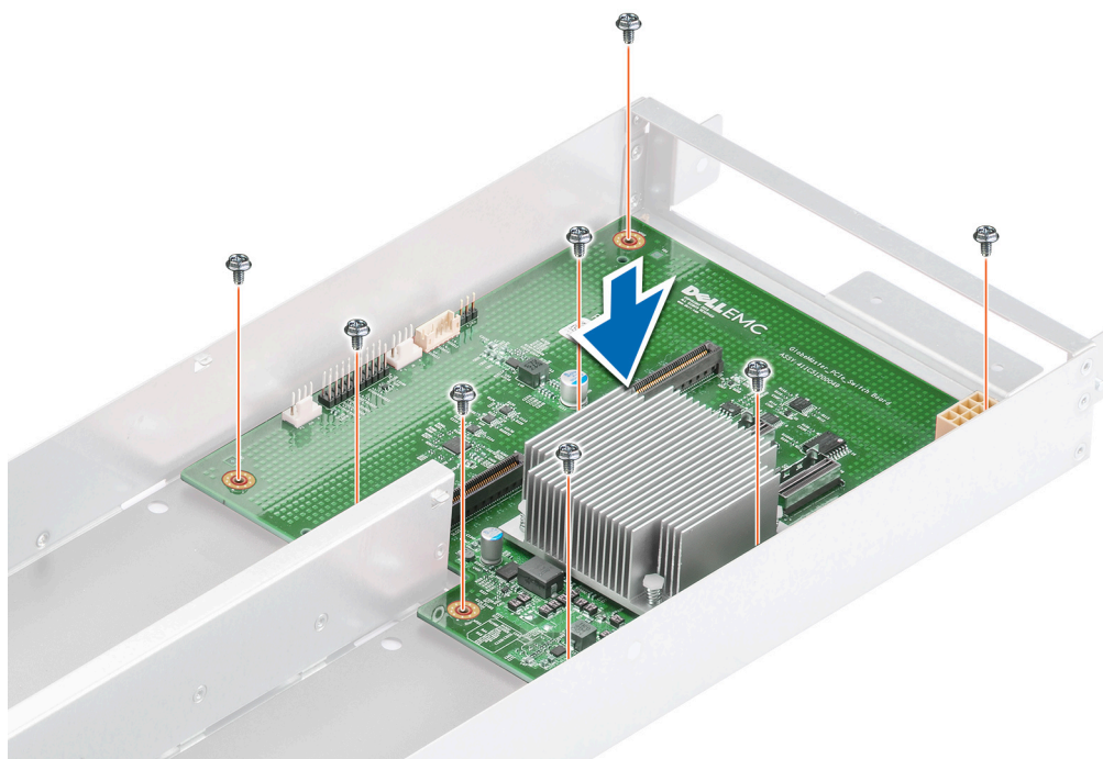
Figure 96. Installation de la carte de commutation PCIe
