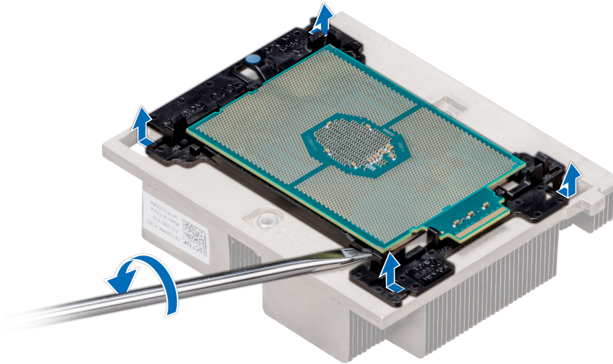
Figure 101. Pliage du support de processeur
