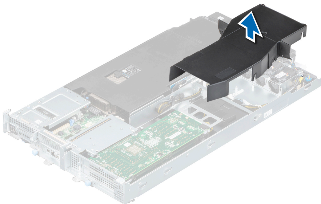
Figure 19. Retrait du carénage à air (configuration pleine largeur, hauteur standard)
