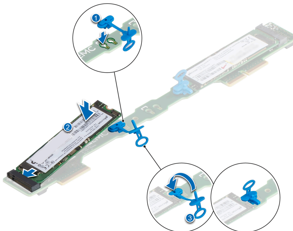
Figure 67. Installation du disque SSD M.2
