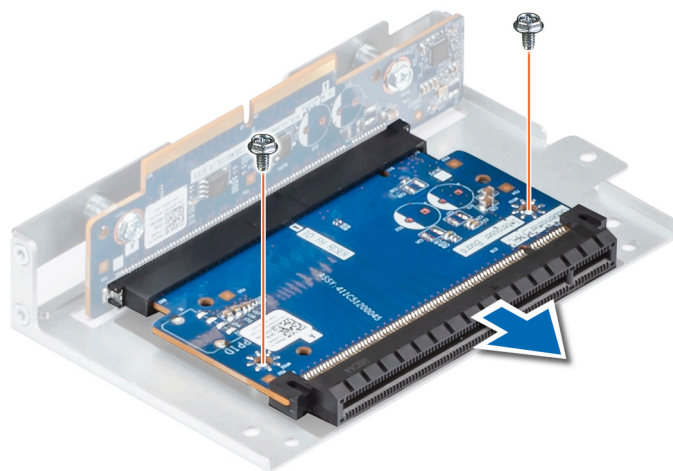
Figure 80. Retrait de la carte intercalaire hauteur standard, pleine longueur
