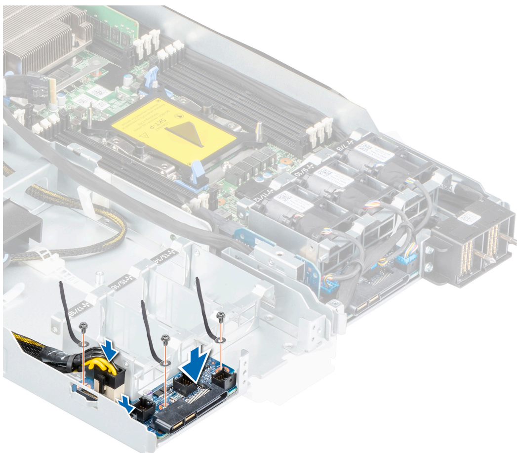
Figure 57. Installation de la carte-pont de la carte mère (2)
