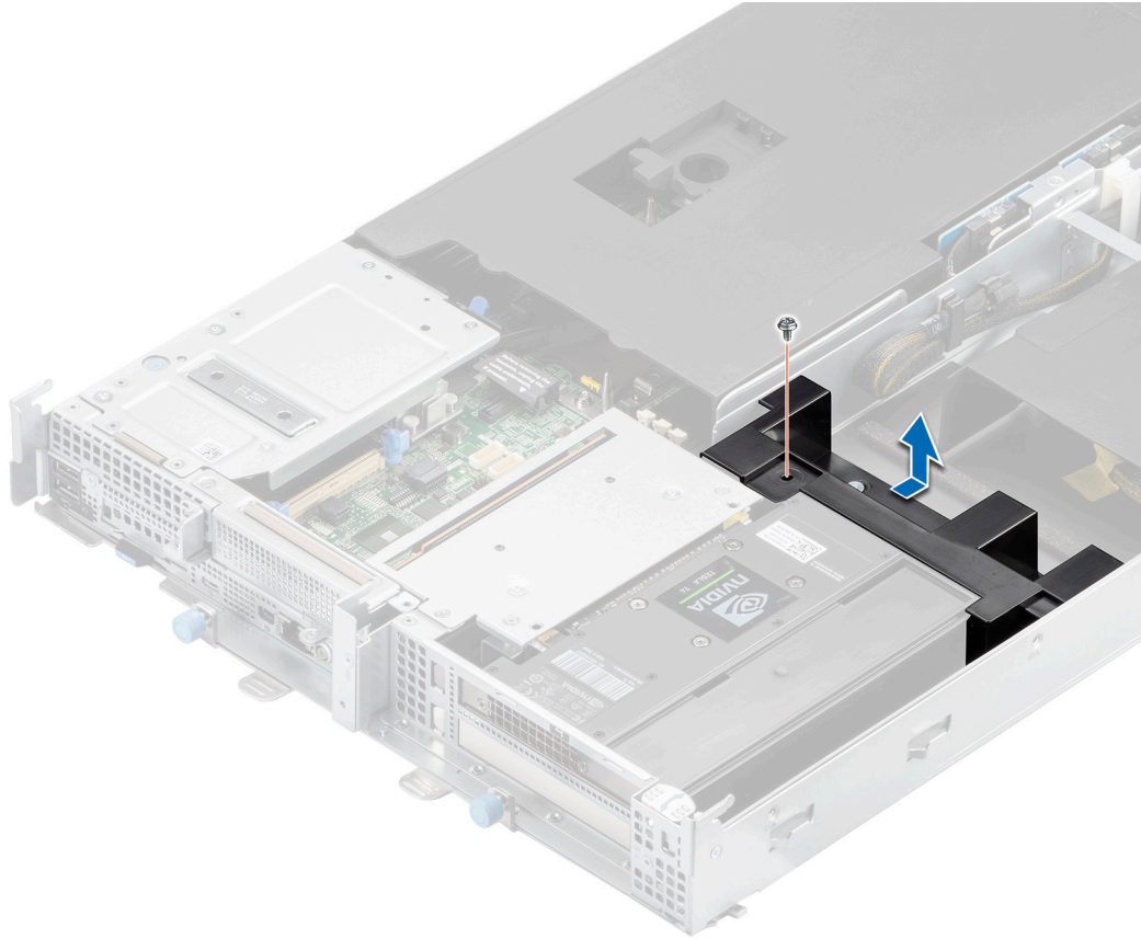
Figure 71. Retrait du déflecteur d'air
