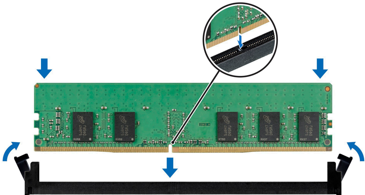
Figure 108. Installation d'une barrette de mémoire
