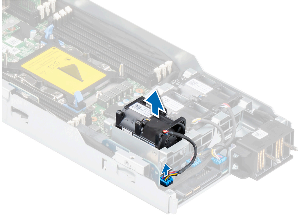
Ilustración 16. Extracción de un ventilador de enfriamiento
