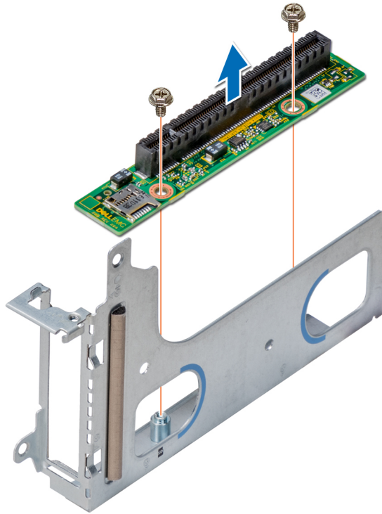
Ilustración 48. Extracción de la placa del soporte vertical x16
