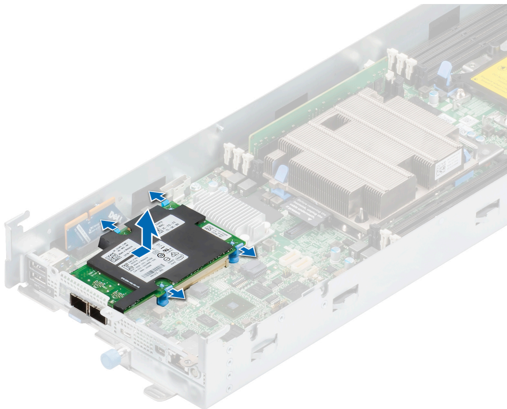
Ilustración 59. Extracción de la tarjeta OCP
