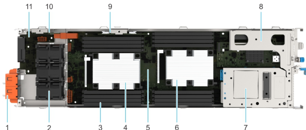
Ilustración 2. Sled de medio ancho en el interior del sistema
