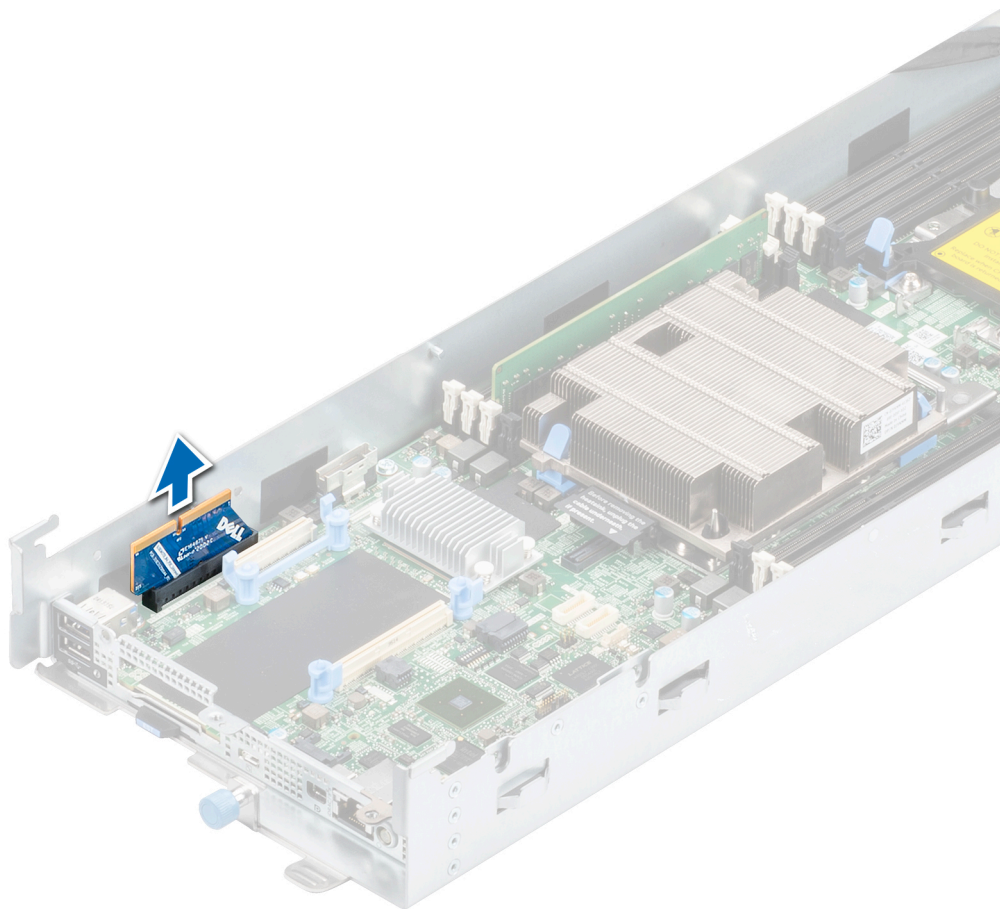
Ilustración 43. Extracción de la placa del soporte vertical de mini-PERC
