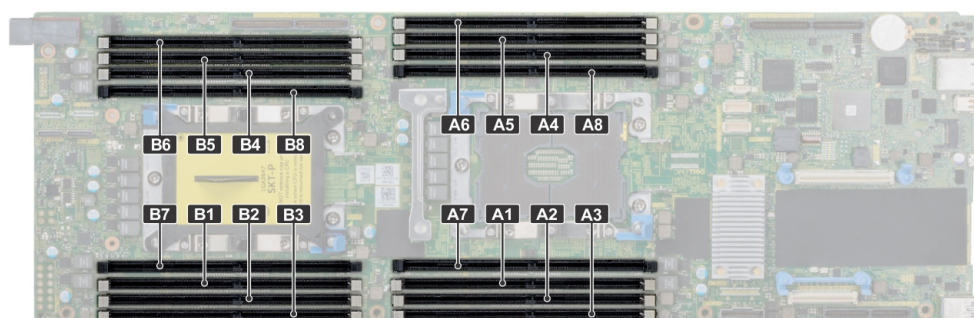
Ilustración 45. Ubicaciones de los conectores de memoria
