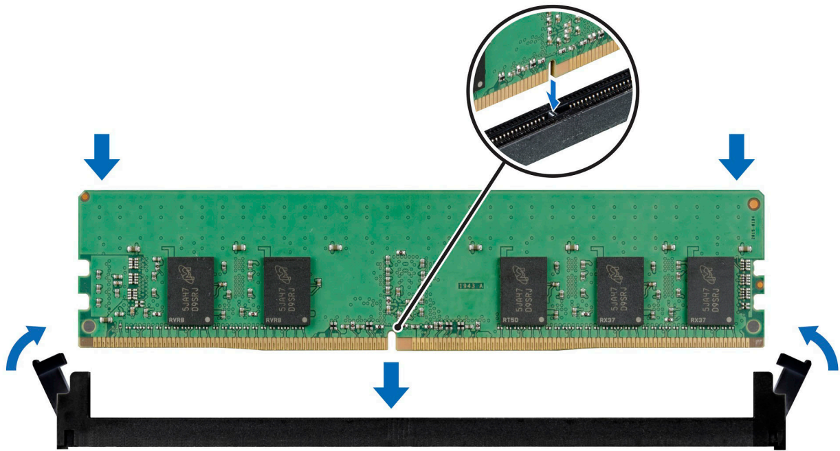
Ilustración 47. Instalación de un módulo de memoria
