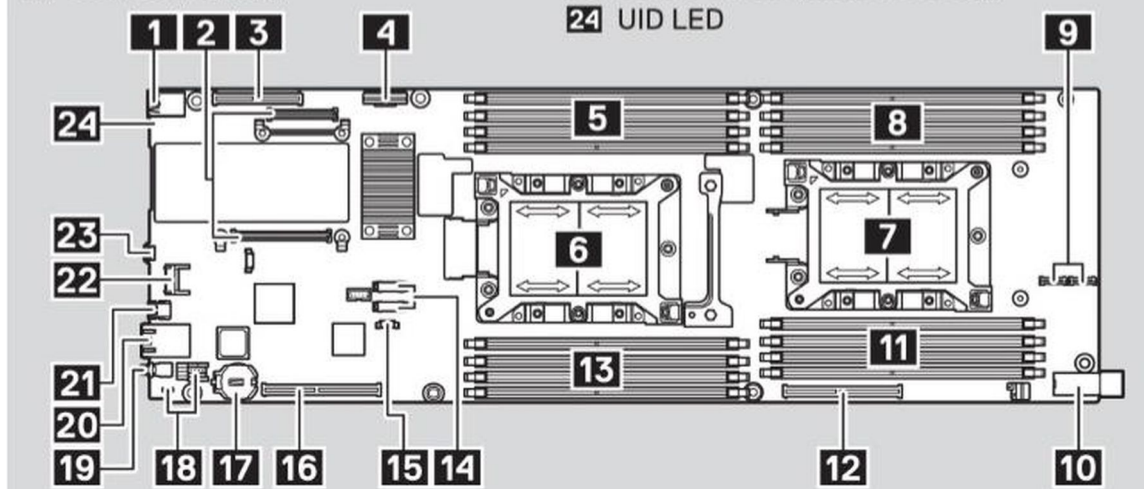
Ilustración 5. Puentes y conectores de la tarjeta madre del sistema
