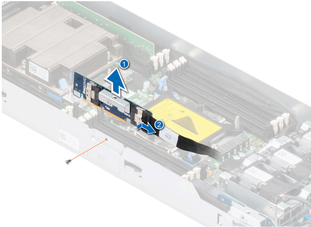
Ilustración 20. Extracción de la placa del soporte vertical M.2
